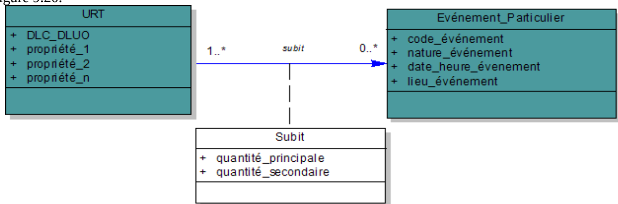
Figure 9.20 – Modèle UML de la classe Événement_Particulier
