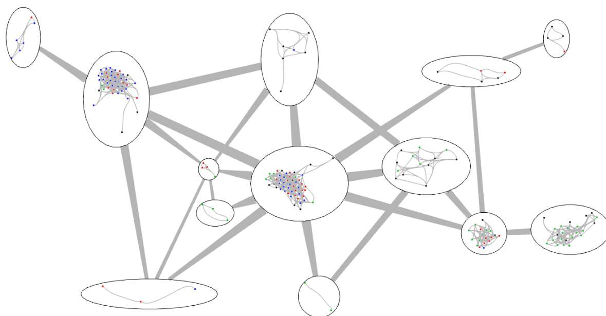
Figure 51 : Dans cette visualisation, qui est une démonstration préliminaire réalisée par Romain Bourqui avec le logiciel Tulip, les fréquences relatives ont été déterminées à partir de photos. 6 facettes de plaquettes ont été analysées dans 3 récifs, pour 3 sites pour chacune des 4 mers régionales (Golfe de Gascogne, méditerranée nord occidentale, Adriatique et Mer Rouge). Les nœuds de ce graphe représentent des facettes de plaques en PVC, et les liens relient les facettes pour chaque pourcentage d'un taxon en commun avec une autre facette. Chaque couleur représente une mer régionale différente. L'intérêt de cette visualisation est de mettre en exergue les clusters les plus importants, où les plaques avec les compositions en taxons les plus similaires sont les plus proches, et les sites des différentes mers sont colorés de manière différente avec des regroupements plus ou moins hétérogènes. La figure a été construite en sélectionnant uniquement des fréquences relatives en commun supérieures à 10%. Lorsque les formes, tailles et/ou couleurs des nœuds correspondant à l'affichage d'une valeur de paramètre de contextes se regroupent dans un cluster, il faut tester la significativité de ces corrélations grâce à des méthodes statistiques propres aux graphes.
