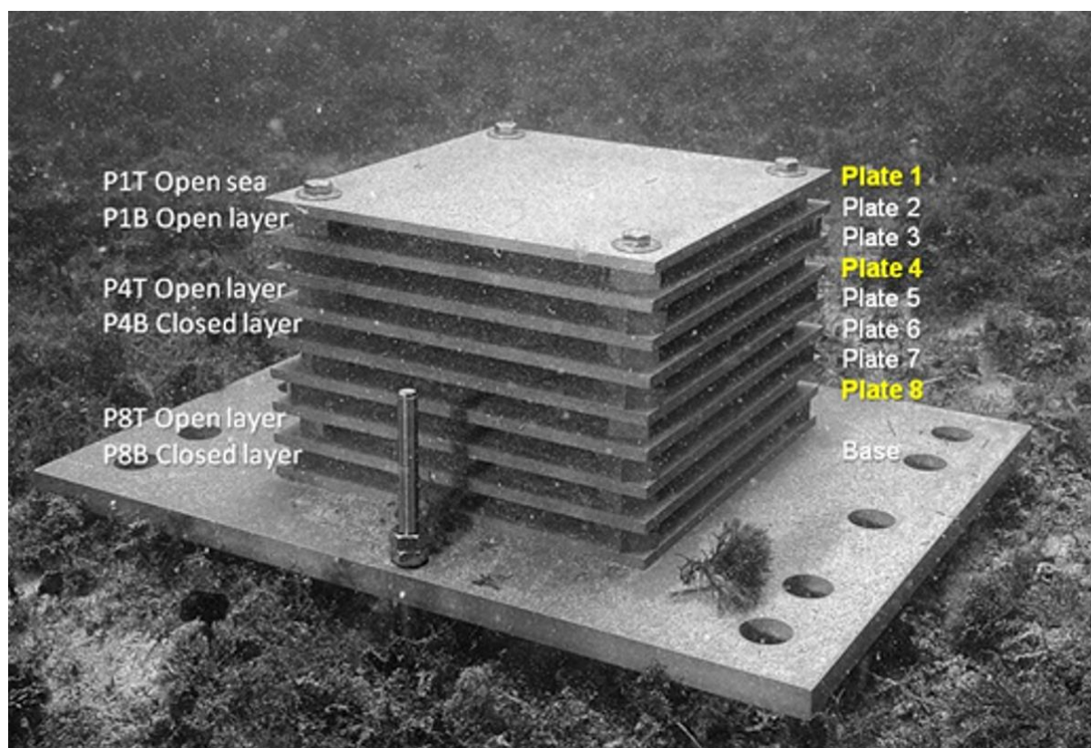
Figure 23 : Un ARMS nouvellement déployé (île de l'Erevine, NW Méditerranée). L'utilisation alternative des espaceurs courts et longs en PVC donne une tour de quatre couches ouvertes et de quatre couches fermées. © photo CNRS / F. Zuberer
