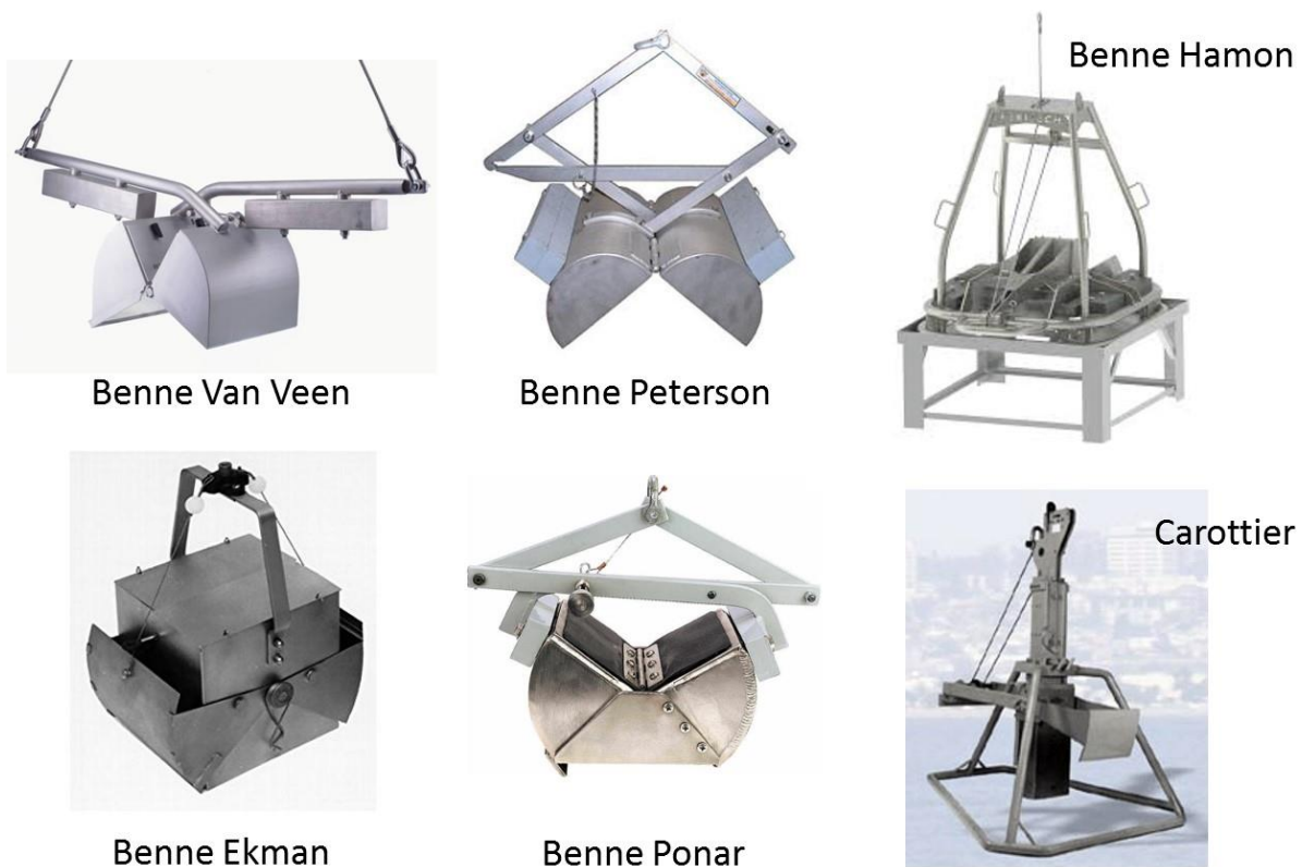
Figure 1_2. Exemples d'engins utilisés pour effectuer des prélèvements quantitatifs.
