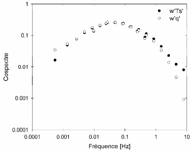
Figure 3 : Distribution en fréquence de cospectres moyens de flux de chaleur sensible ( w'T_s' ) et de flux de chaleur latente ( w'q' ), normalisés par la covariance moyenne, à Lamasquère entre le 12 avril 2006 et le 25 avril 2006 (sol nu).
