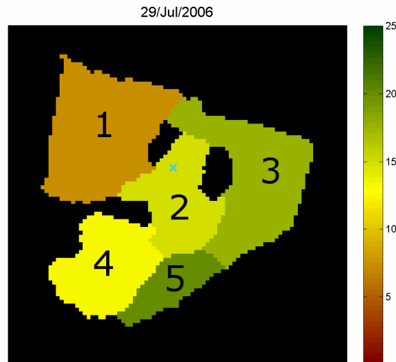
Figure 14 : GEP spatialisée sur les segments composants la parcelle d'Auradé le 29-Juil-2007. Le haut de l'image est orienté au nord et l'échelle est de 100 m pour 1 cm sur la carte. La barre de couleur correspond aux valeurs de GEP exprimées en \text{g C m}^{-2} \text{j}^{-1} . La croix bleue représente l'emplacement du mât de mesure.
