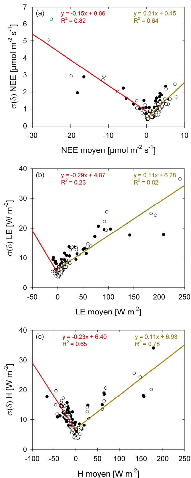
Figure 13 : Erreur aléatoire de la mesure en fonction de la valeur moyenne du flux (vingt classes de flux avec le même nombre de données dans chaque classe) pour (a) le flux net de CO 2 (NEE), (b) le flux de chaleur latente (LE) et (c) le flux de chaleur sensible (H). Les cercles pleins et vides correspondent aux parcelles d'Auradé et de Lamasquère, respectivement. Les traits et notes rouges et vertes correspondent aux droites de régressions et leur coefficient de détermination pour les flux négatifs et positifs, respectivement.
