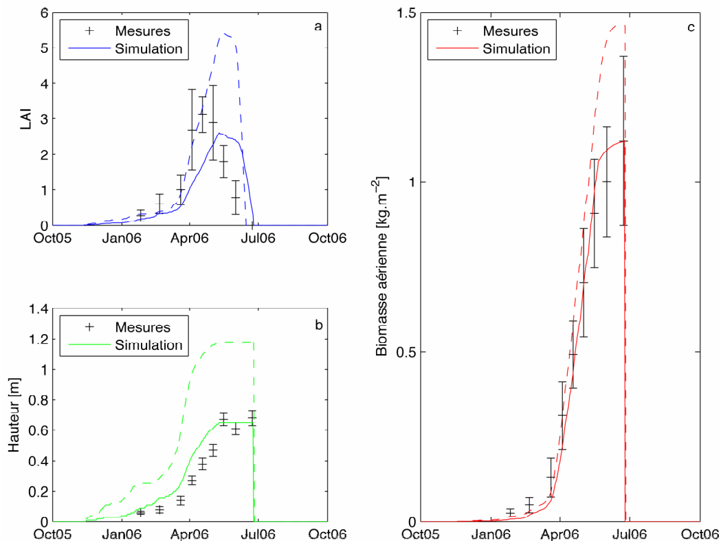
Figure 3 : Simulation des variables biologiques par le modèle STICS, a) la surface foliaire (LAI) exprimée en \text{m}^2 \text{feuilles m}^{-2} \text{sol} , b) la hauteur du couvert en m et c) la biomasse aérienne en \text{kg m}^{-2} pour la culture de blé à Auradé. En pointillé, les simulations avant optimisation des paramètres clés (voir texte).
