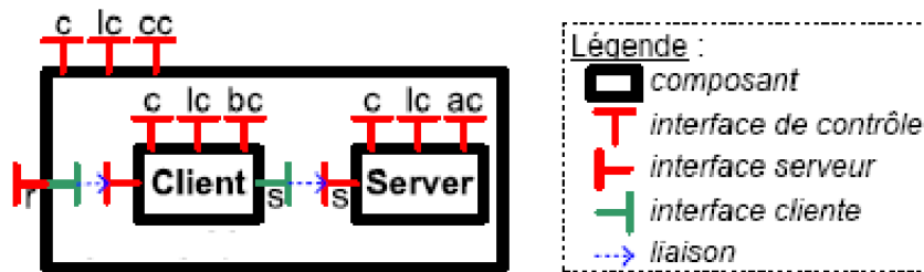
FIGURE A.1 – Modèle à composants Fractal : composant client/serveur
