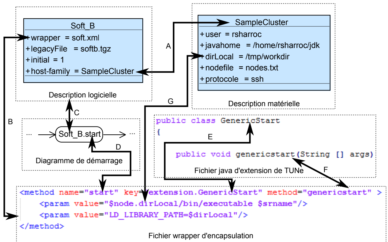
FIGURE 2.13 – Vue globale de la construction d’une gestion autonome avec TUNe
