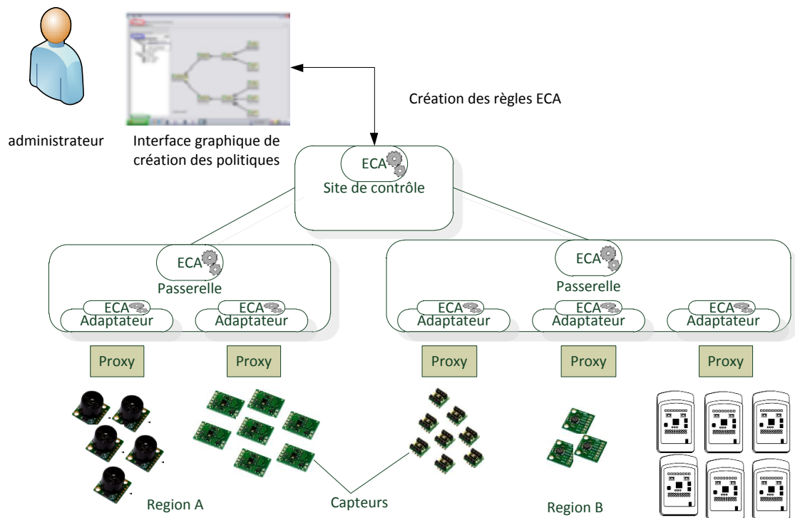
FIGURE 4.1 – Intégration de services ECA dans l'architecture hiérarchique de XSSteaMWare
