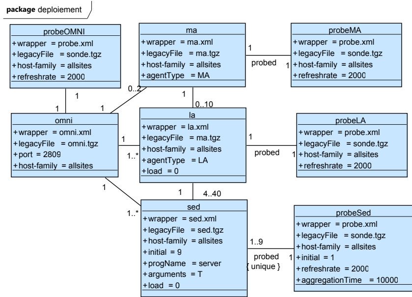
FIGURE 3.5 – SDD utilisé pour le déploiement de DIET, 1 probe d’agrégation pour les SEDs
