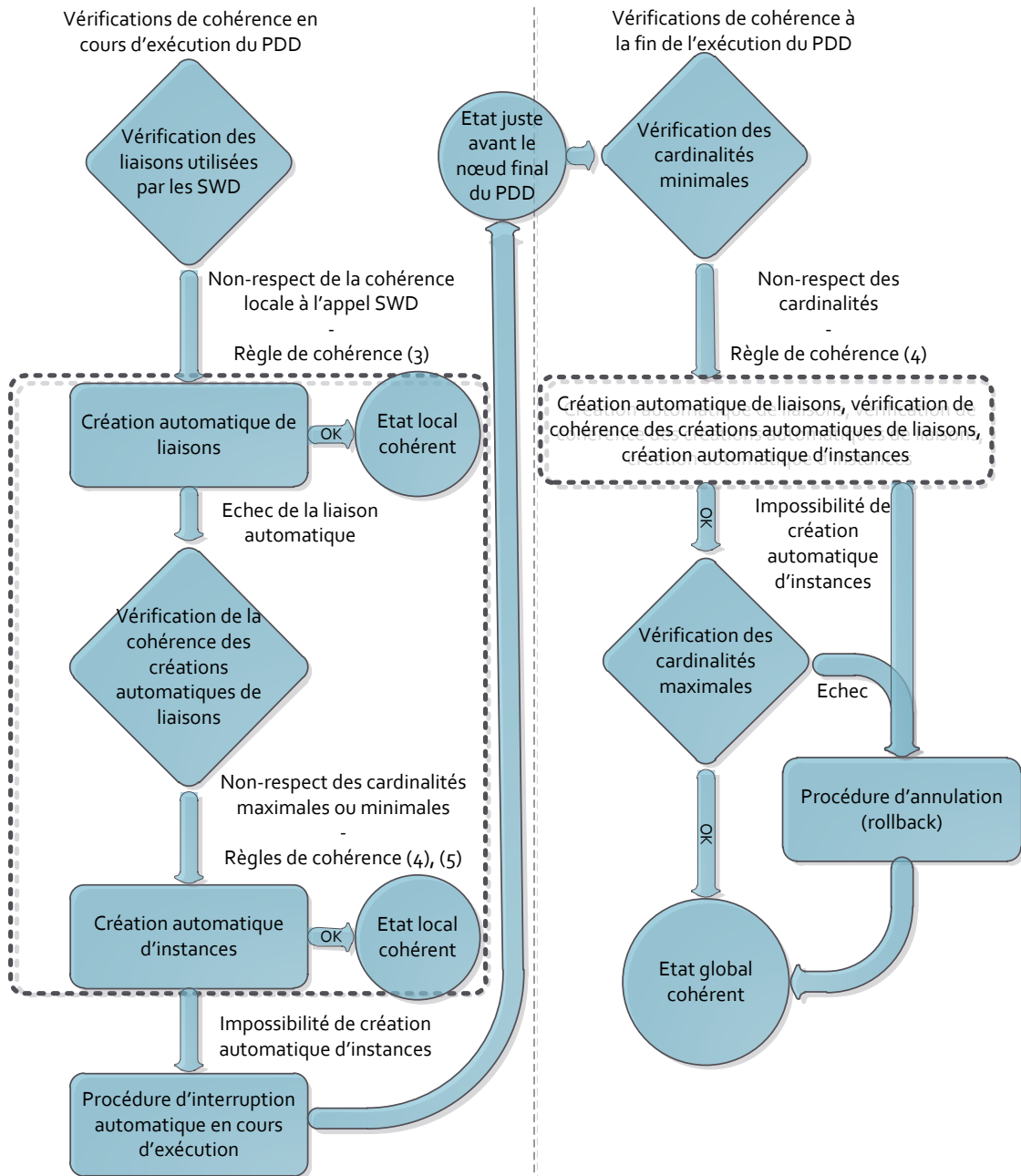
FIGURE 6.10 – Vue globale de la résolution d'incohérences
