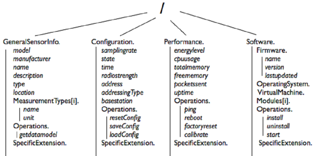
FIGURE 2.3 – Hiérarchie du modèle générique XSStraMWare : le DATAMODEL
