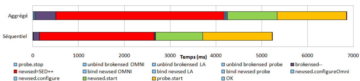
FIGURE 3.10 – Détail du temps de réparation du LA
