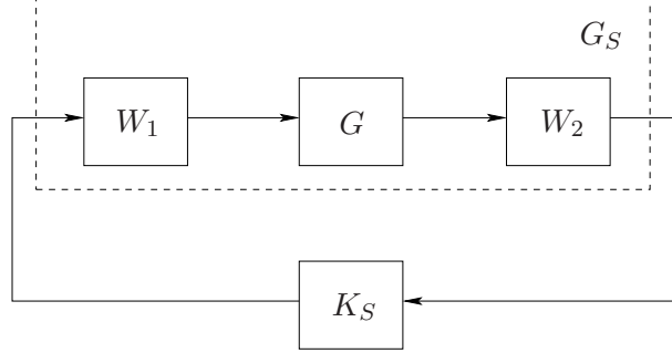
FIG. 4.2 – Schéma LSPD
