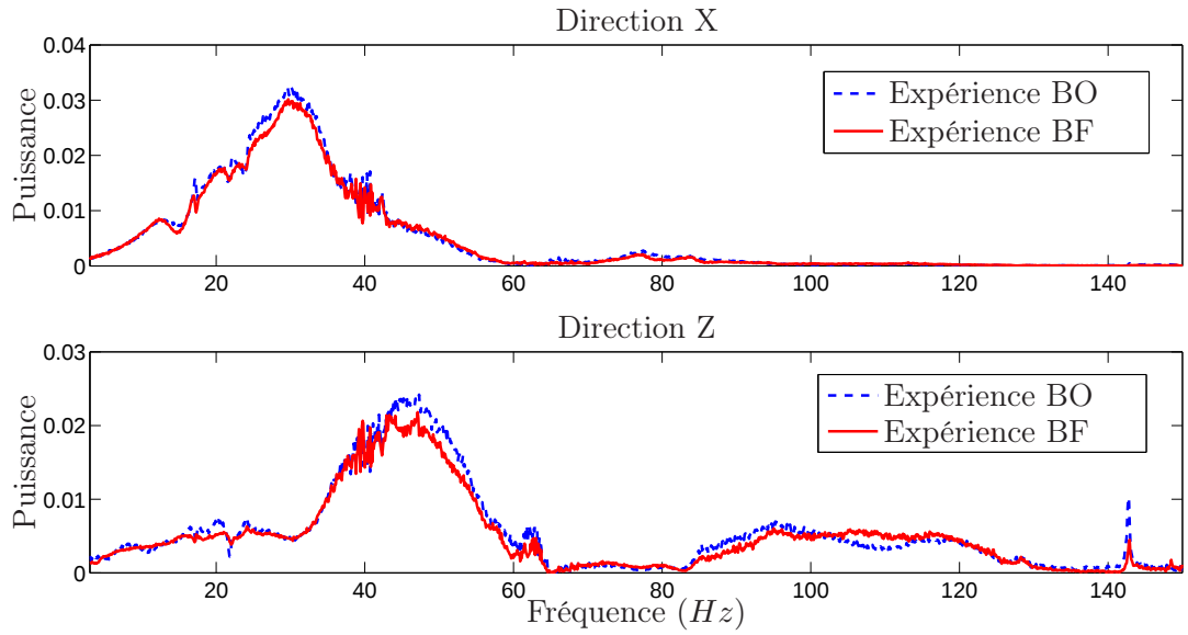
FIG. 3.15 – Résultats expérimentaux - Robot avec 2,5 kg de charge, contrôleur réduit K_{SM_r} - Trajectoire de 18 g dans les directions X et Z - Spectres de puissance
