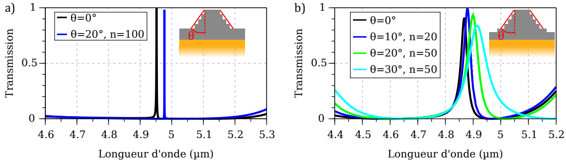
FIGURE 4.4 – Influence de la verticalité des flancs sur la réponse des filtres ZCGs 1D. a) Transmission du filtre ZCG MIR 1D de référence (courbe noire, f = 0.24 ) et d'un filtre de facteur de remplissage f = 0.2 , dont les créniaux ont des flancs inclinés de 20^\circ découpés en 100 niveaux. b) Évolution de la transmission du filtre ZCG MIR 1D doublement corrugué de référence à facteur de remplissage constant ( f = 0.24 ) pour différentes valeurs de l'inclinaison des flancs. Les dimensions communes aux filtres sont les suivantes : d_w = 840 \text{ nm} , d_g = 870 \text{ nm} , \Lambda = 2.703 \mu\text{m} .
