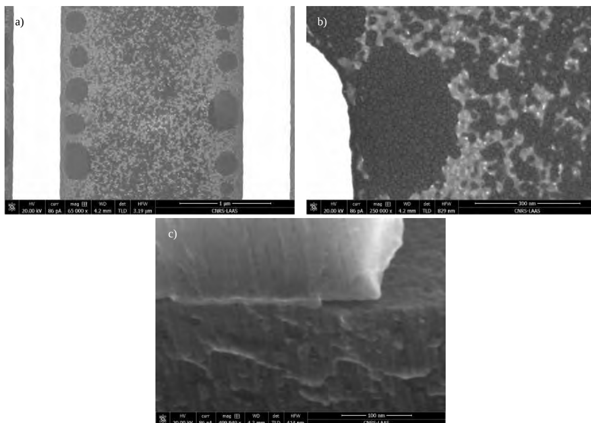
FIGURE 4.31 – Images MEB de l'échantillon surgravé 16 s (voir figures 4.30b, courbe rouge et figure 4.30c) après 2 minutes d'attaque chimique en différents endroits : a) entre deux crêneaux du réseau et b) zoom au niveau d'une zone dégagée de résidus. L'image MEB c) présente le pied d'une dent du réseau clivé ayant subi une attaque chimique de 4 minutes.
