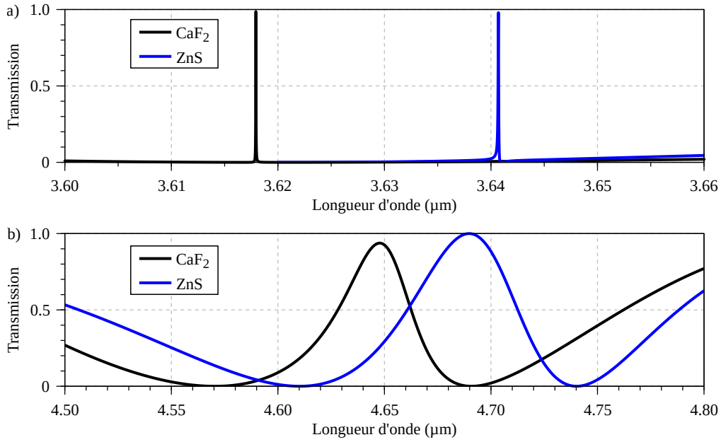
FIGURE 3.27 – a) Spectre en transmission du filtre ZCG TE/TM hautement résonant sur substrat \text{CaF}_2 et \text{ZnS} . Les dimensions du filtre sur substrat \text{CaF}_2 sont : t_s = 0.22 \mu\text{m} , t_r = 0.99 \mu\text{m} , \Lambda = 1.255 \mu\text{m} et f\Lambda = 321 \text{ nm} . L'épaisseur du guide plan pour le filtre de substrat \text{ZnS} est : t_s = 0.194 \mu\text{m} . b) Spectre en transmission du filtre ZCG TE/TM large sur substrat \text{CaF}_2 et \text{ZnS} . Les dimensions du filtre sont : t_s = 0.36 \mu\text{m} , t_r = 0.85 \mu\text{m} , \Lambda = 1.39 \mu\text{m} et f = 0.48 .
