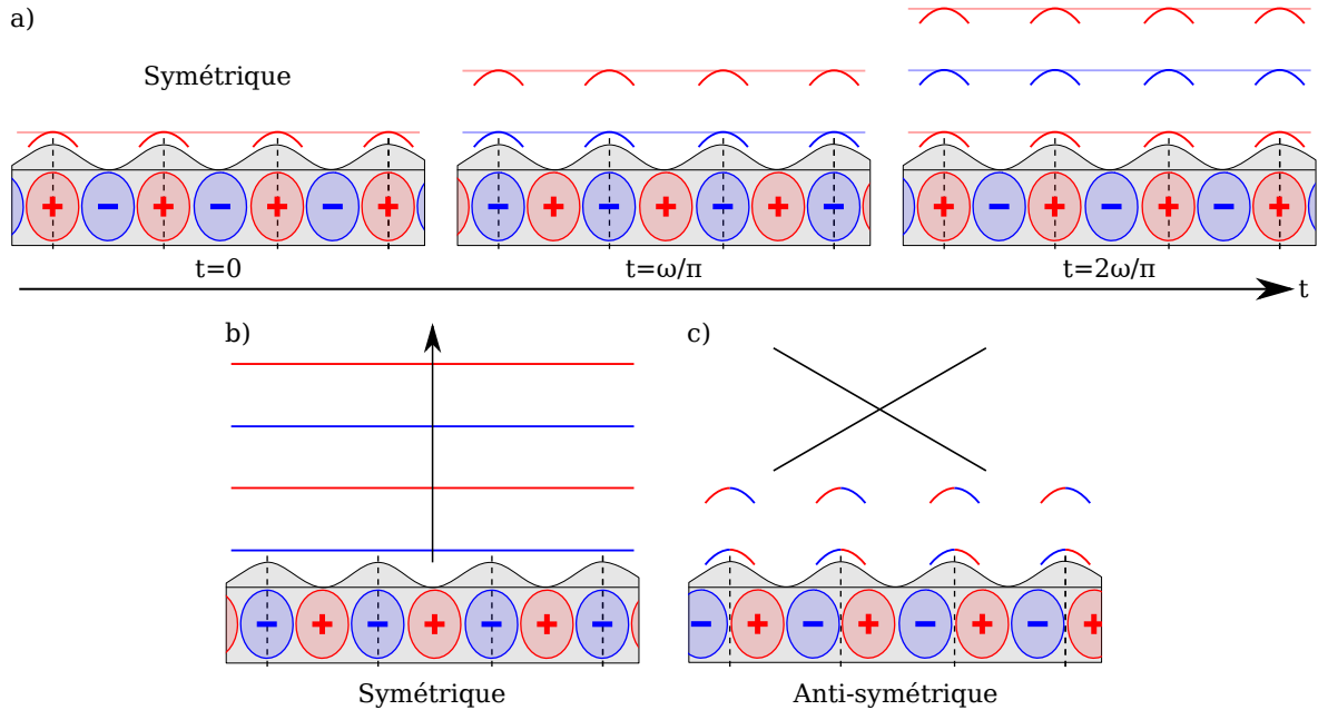
FIGURE 1.22 – a) Illustration de la construction du front d'onde pour le mode symétrique. Représentation schématisée de la forme du front d'onde du champ découplé par le réseau dans le cas b) du mode symétrique et c) du mode anti-symétrique.
