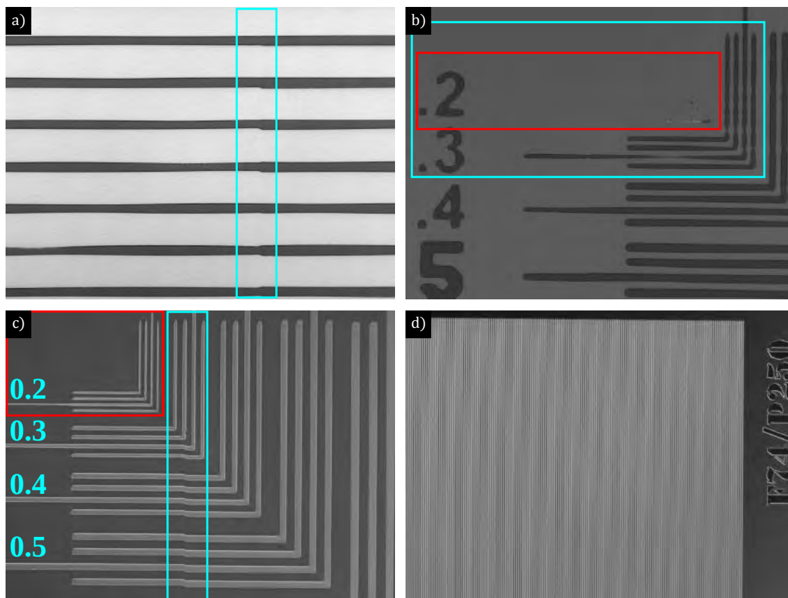
FIGURE C.1 – Images prise au microscope non confocal avec illumination monochromatique de différents réticules utilisés. a) Premier réticule utilisé : les lignes du réseau sont orientées dans la direction de balayage de l'appareil de lithographie laser. Le facteur de remplissage des lignes du réticule est ici de 0.76 (larges bandes de chrome, et petites ouvertures), leur période est de 2.703\text{ }\mu\text{m} . b) Motif de résolution présent à la surface du second réticule. Les chiffres indiqués donnent la largeur des lignes qui est aussi égale à leur espacement, en \mu\text{m} , en unités de champ. Leur taille sur le réticule est donc 5 fois plus grande. Par exemple, « .4 » signifie que les lignes insolées dans la résine avec la réduction de champ mesureront 0.4\text{ }\mu\text{m} . Sur le réticule, elles mesurent en réalité 2\text{ }\mu\text{m} . c) Motif de résolution présent à la surface du troisième et dernier réticule. Les dimensions des lignes ont été ajoutées manuellement. d) Vue d'ensemble sur des lignes de facteur de remplissage égal à 0.74, leur période est de 2.50\text{ }\mu\text{m} .
