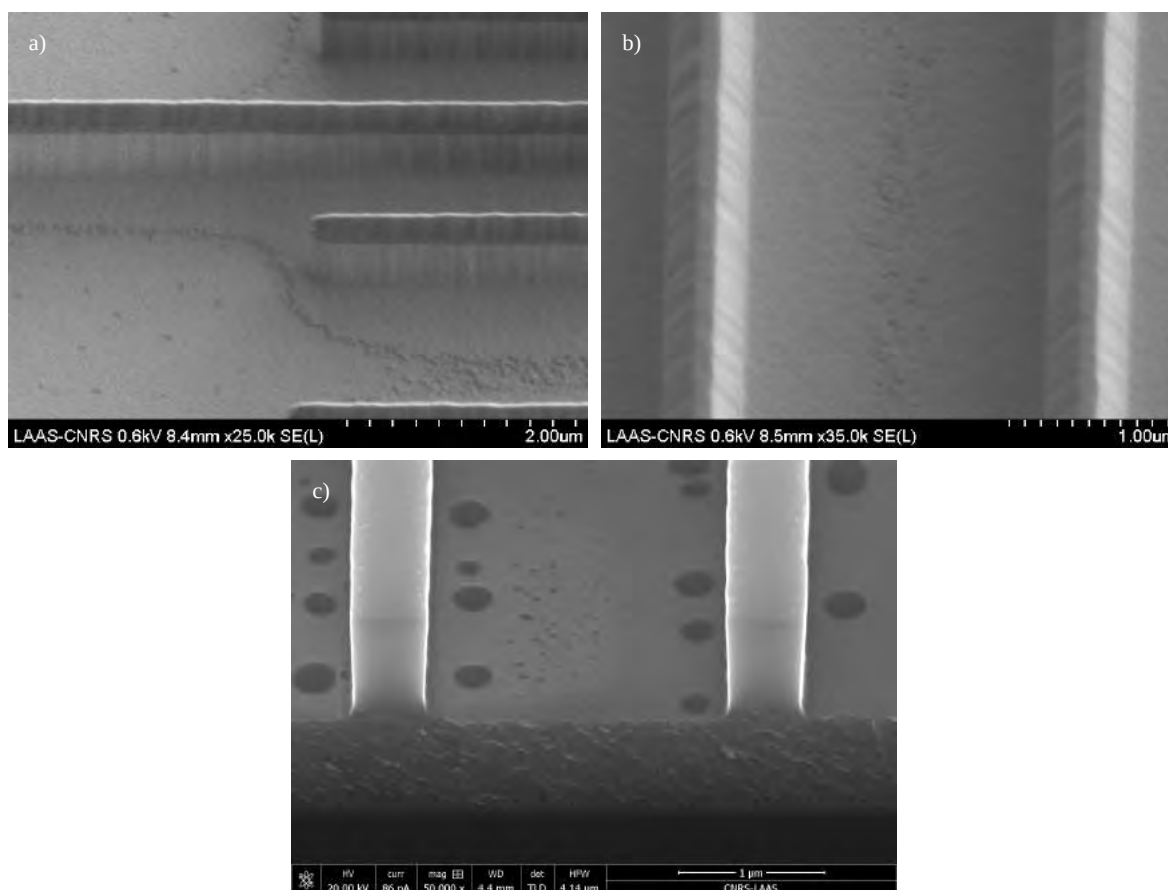
FIGURE 4.30 – Les images a) et b) sont des clichés MEB du réseau dont le suivi DFA est donné par la courbe noire dans la figure 4.29a. Elles correspondent respectivement à a) un bord de motif test et b) une tranchée gravée entre deux créneau du réseau d'un filtre. L'image c) est une vue MEB en coupe de l'échantillon surgravé 12 s, et dont la courbe de suivi DFA est donnée par la courbe bleue de la figure 4.29a.
