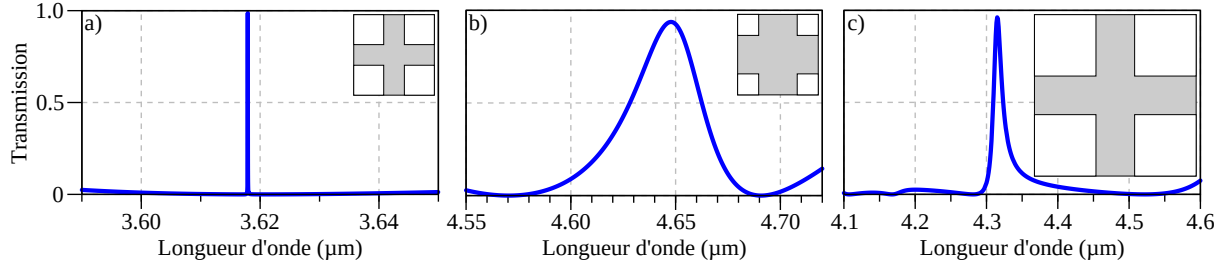
FIGURE 3.30 – Illustration des 3 structures de ZCGs TE/TM caractéristiques obtenues : a) un filtre hautement résonant ( t_s = 0.22 \mu\text{m} , t_r = 0.99 \mu\text{m} , \Lambda = 1.255 \mu\text{m} et f\Lambda = 321 \text{ nm} ), b) un filtre large bande ( t_s = 0.36 \mu\text{m} , t_r = 0.85 \mu\text{m} , \Lambda = 1.39 \mu\text{m} et f = 0.48 ), et c) un filtre multi-résonant ( t_s = 0.36 \mu\text{m} , t_r = 1.2 \mu\text{m} , \Lambda = 2.55 \mu\text{m} et f = 0.24 ). Les encarts dans chaque figure illustrent schématiquement la maille du réseau.
