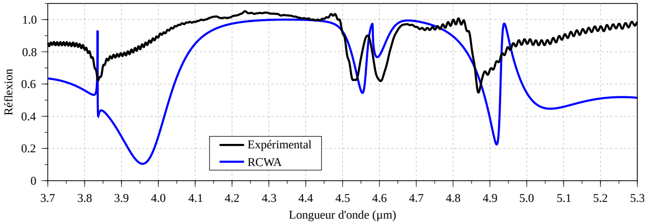
FIGURE 4.35 – Comparaison entre la courbe expérimentale du réseau mesurée en réflexion (courbe noire) et la courbe théorique calculée par RCWA (courbe bleue). Les paramètres géométriques du réseau utilisés pour la simulation sont : d_w = 713 \text{ nm} , d_g = 826 \text{ nm} , h = 122 \text{ nm} , \Lambda = 2.54 \mu\text{m} , f_1 = 0.24 , f_2 = 0.30 , \delta = 47 \text{ nm} . Un faisceau gaussien incident de largeur 40 \mu\text{m} est considéré dans la simulation.
