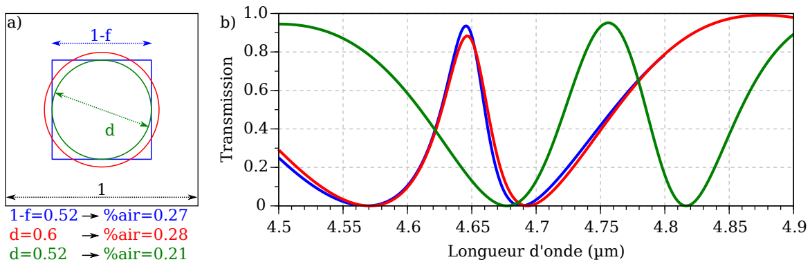
FIGURE 3.23 – Étude comparative de la réponse du filtre ZCG TE/TM large bande selon la forme ronde ou carrée des ouvertures dans le réseau. Les dimensions fixes du filtre sont les suivantes : t_s = 0.36 \mu\text{m} , t_r = 0.85 \mu\text{m} et \Lambda = 1.39 \mu\text{m} .
