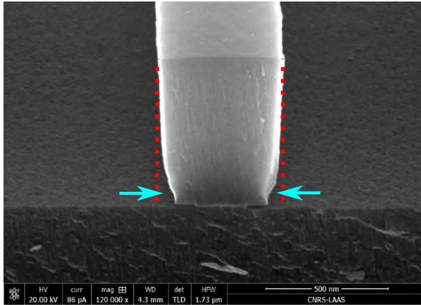
FIGURE 4.21 – Image MEB en coupe de réseaux ayant subi une gravure RIEAN- \text{O}_2 trop longue.
