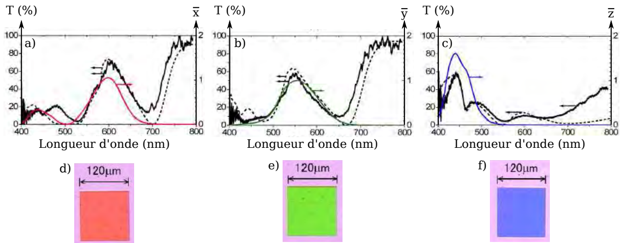
FIGURE 1.38 – Tiré de [144]. Spectres en transmission théoriques (tirets noirs) et expérimentaux (courbe noire) reproduisant les trois fonctions colorimétriques a) rouge ( \bar{x} , courbe rouge), b) verte ( \bar{y} , courbe verte) et c) bleue ( \bar{z} , courbe bleue). Les figures d), e) et f) présentent une photographie des réseaux fabriqués et caractérisés lorsqu'ils sont illuminés en face arrière par un faisceau de lumière blanche. Les paramètres des réseaux (voir figure 1.34, page 45) sont : \Lambda = 400 nm et f\Lambda = 279 nm pour le réseau rouge, \Lambda = 350 nm et f\Lambda = 231 nm pour le réseau vert, et \Lambda = 440 nm et f\Lambda = 177 nm pour le réseau bleu. Le réseau a la même épaisseur pour les 3 filtres : 100 nm.
