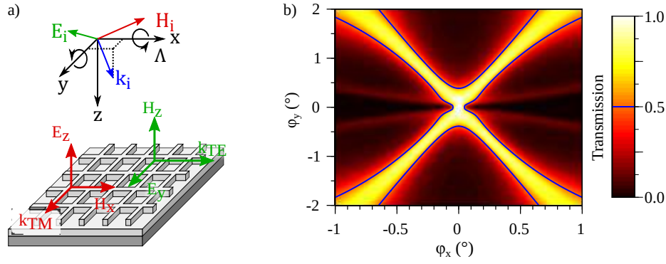
FIGURE 3.16 – a) Illustration des conventions utilisées pour l'étude de la tolérance angulaire. Les angles \phi_x et \phi_y se réfèrent respectivement aux rotations dans le sens trigonométrique autour des axes (Ox) et (Oy). Le champ électrique incident E_i est polarisé TE. b) Cartographie de la transmission T(\phi_x, \phi_y) du filtre à \lambda = 3.61789 \mu\text{m} . La ligne bleue correspond à l'IFWHM du filtre. Les dimensions du filtre sont les suivantes : t_s = 0.22 \mu\text{m} , t_r = 0.99 \mu\text{m} , \Lambda = 1.255 \mu\text{m} et f\Lambda = 321 \text{ nm} .
