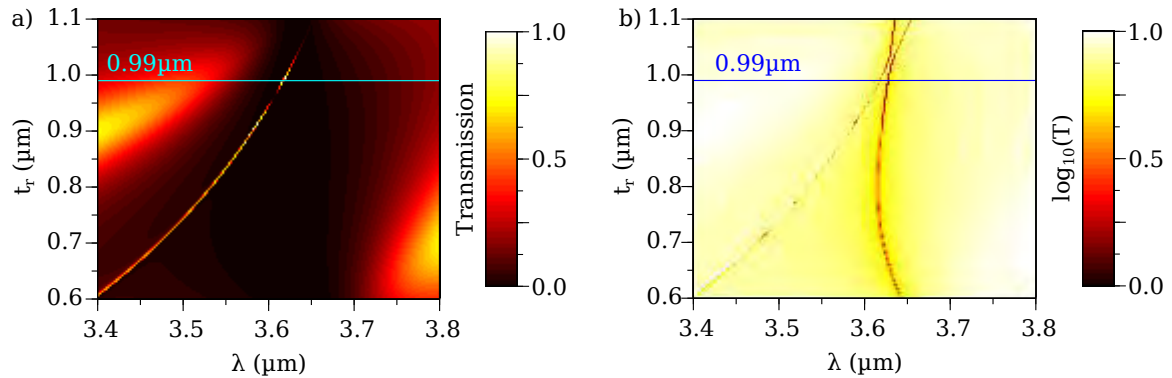
FIGURE 3.13 – Étude paramétrique de la transmission T(\lambda, d_g) à travers une structure de ZCG TE/TM sur une échelle a) linéaire et b) logarithmique. Les paramètres géométriques fixes sont : t_s = 0.22 \mu\text{m} , \Lambda = 1.255 \mu\text{m} et f\Lambda = 321 \text{ nm} .
