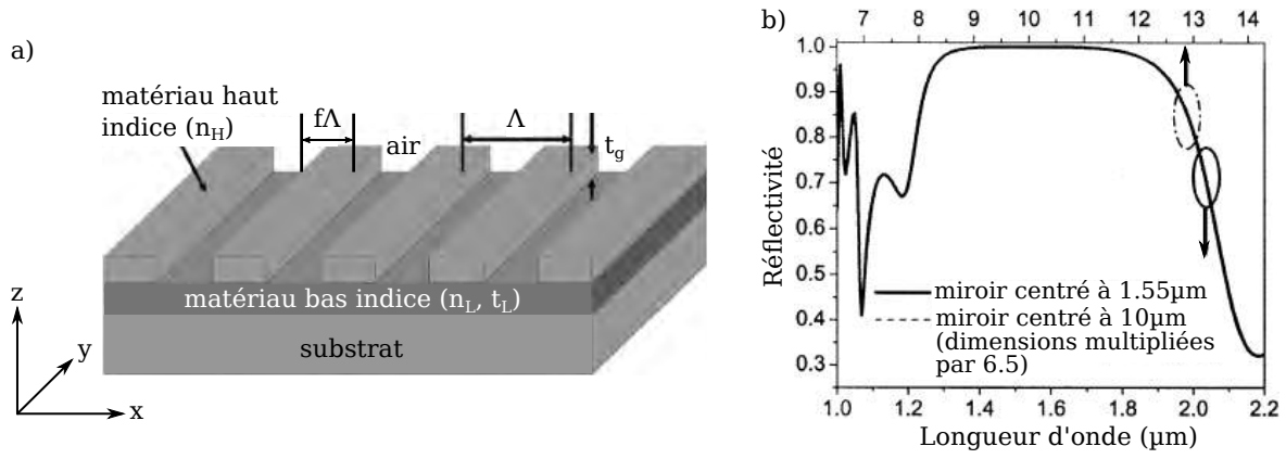
FIGURE 1.34 – Tiré de [125]. a) Schéma de la structure. b) Illustration de l'impact d'un changement d'échelle des dimensions du système sur son spectre. Les dimensions du filtre centré sur 1.55 \mu m sont : \Lambda = 0.7 \mu m , f = 0.75 , t_g = 0.46 \mu m , t_L = 0.9 \mu m , n_H = n_{Si} , n_L = n_{SiO_2} . Les dimensions du filtre centré à 10 \mu m ont été multipliées par 6.5. Le réseau est illuminé sous incidence normale par une onde polarisée TM.
