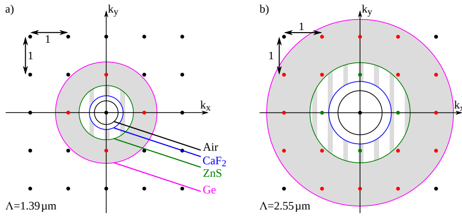
FIGURE 3.29 – Illustration dans l'espace des k des ordres diffractés pouvant intervenir dans le cas d'un filtre résonnant à 4.32 \mu\text{m} ayant une période de a) 1.39 \mu\text{m} et b) 2.55 \mu\text{m} . Les axes sont normalisés à la période du réseau. Les différents cercles ont pour rayon n\Lambda/\lambda , où n est l'indice du matériau considéré, \Lambda est la période du réseau et \lambda est la longueur d'onde du rayonnement incident, fixée à 4.32 \mu\text{m} . Les points rouges indiquent le couplage d'un mode propagatif confiné dans le Ge. Les points verts indiquent le couplage d'un mode pouvant se propager dans le Ge et le ZnS. L'incidence sur le réseau est normale.
