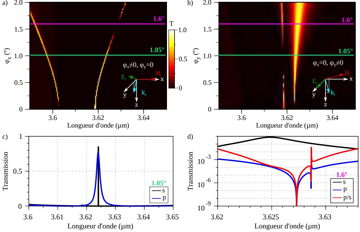
FIGURE B.4 – Les figures a) et b) présentent respectivement la cartographie en transmission T(\lambda, \varphi_x) sur une échelle linéaire du filtre TE/TM hautement résonant sous incidence pseudo-classique a) p et b) s. c) Extraction du spectre du filtre pour les deux états de polarisation p et s pour une incidence de 1.05^\circ illustrant un comportement insensible à la polarisation. d) Même principe, pour une incidence de 1.6^\circ , illustrant un comportement de type polariseur. Les dimensions du filtre sont les suivantes : t_s = 0.22 \mu\text{m} , t_r = 0.99 \mu\text{m} , \Lambda = 1.255 \mu\text{m} et f\Lambda = 321 \text{ nm} .
