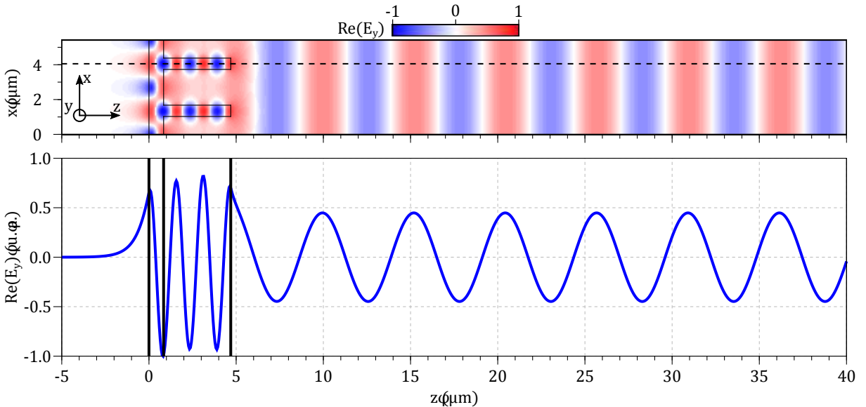
FIGURE 2.16 – a) Cartographie de la partie réelle du champ E_y dans le plan (Oxz) sur deux périodes du filtre de dimensions d_g = 3.85\text{ }\mu\text{m} , d_w = 0.84\text{ }\mu\text{m} , \Lambda = 2.703\text{ }\mu\text{m} et f = 0.24 à la longueur d'onde du pôle du couplage C_1^{(1)} : 5.24\text{ }\mu\text{m} . b) Évolution de la partie réelle du champ E_y extraits de la cartographie a) à l'abscisse indiquée par la ligne en tirets noirs.
