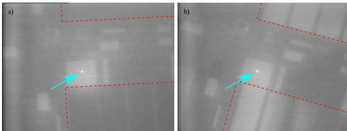
FIGURE 4.23 – Capture d'écran du moniteur de suivi du pointage laser a) avant ouverture du BARC et b) après ouverture du BARC. Le spot laser, indiqué par une flèche bleue, est au centre du motif de suivi DFA dédié, apparaissant comme un carré gris clair. Les zones structurées correspondant aux réseaux des filtres sont délimitées par des lignes en pointillés rouges.
