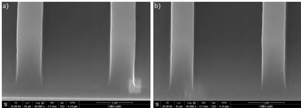
FIGURE C.2 – Vue MEB en coupe sous une incidence de 52^\circ de motifs insolés sur wafer 6 pouces dans différentes conditions : (a) Dose égale à 1050\text{ J}\cdot\text{m}^{-2} et focus de -0.2\text{ }\mu\text{m} , b) dose égale à 1050\text{ J}\cdot\text{m}^{-2} et focus de -0.3\text{ }\mu\text{m} . La zone plus claire dans le coin inférieur droit de l'image a) correspond à la zone de mise au point du MEB.
