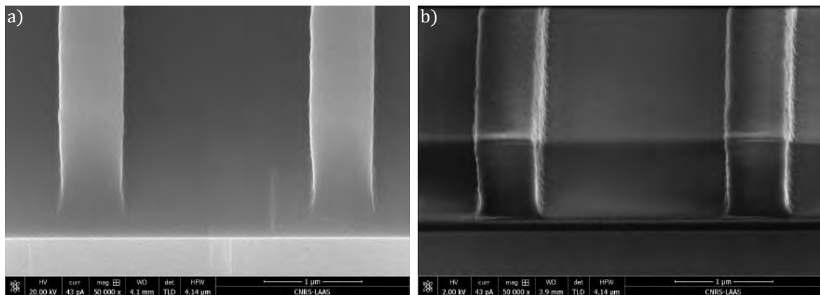
FIGURE C.3 – Vue MEB en coupe de motifs insolés sur wafer 6 pouces dans les mêmes conditions d'exposition (Dose égale à 1100\text{ J}/\text{m}^2 et focus de -0.2\text{ }\mu\text{m} ), mais pour différents réglages du MEB (a) V_{\text{acc}} = 20\text{ kV} , I = 86\text{ pA} , et b) V_{\text{acc}} = 2\text{ kV} , I = 43\text{ pA}
