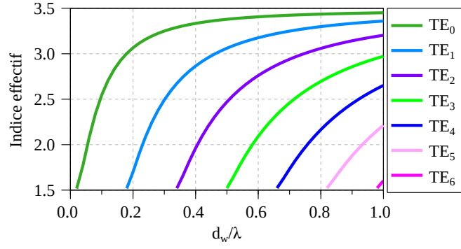
FIGURE 2.5 – Évolution de l'indice effectif des modes d'un guide d'onde plan en silicium ( n_{\text{Si}} = 3.48 ) sur un substrat de silice ( n_{\text{SiO}_2} = 1.51 ) avec l'épaisseur d_w du guide normalisée à la longueur d'onde \lambda .
