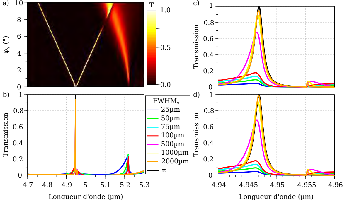
FIGURE A.3 – a) Cartographie de la transmission T(\lambda, \phi_y) du filtre en fonction de la longueur d'onde du rayonnement incident et de l'angle d'incidence \phi_y pour le filtre ZCG MIR de référence. Une rotation supplémentaire d'angle \phi_x = 10^\circ est introduite. Le spectre du filtre est calculé pour différentes tailles de faisceau a) sur une gamme spectrale large, b) au voisinage du pic de transmission, et c) au voisinage du pic de transmission après correction de l'erreur de normalisation. Les dimensions géométriques du filtre sont les suivantes : d_w = 0.84 \mu\text{m} , d_g = 0.87 \mu\text{m} , \Lambda = 2.703 \mu\text{m} et f = 0.24 .
