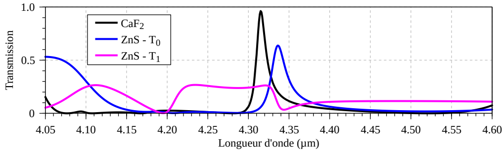
FIGURE 3.28 – Spectre en transmission du filtre ZCG TE/TM couplé par l'ordre 2 du réseau sur substrat \text{CaF}_2 et \text{ZnS} . Les dimensions du filtre sont : t_s = 0.36 \mu\text{m} , t_r = 1.2 \mu\text{m} , \Lambda = 2.55 \mu\text{m} et f = 0.24 .
