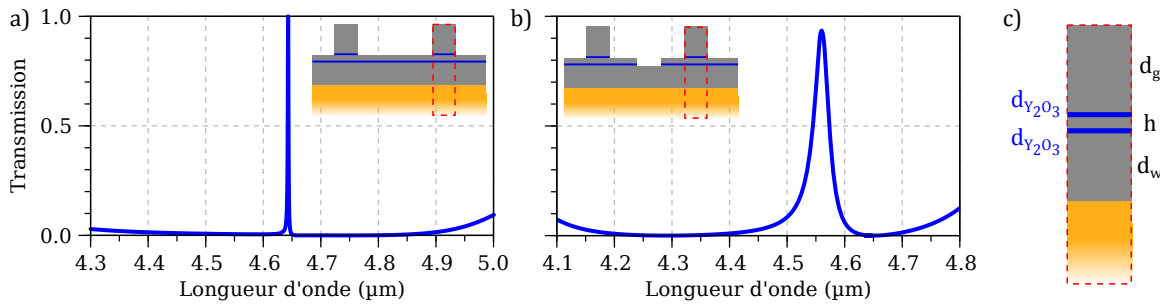
FIGURE 4.20 – Introduction de couches d’arrêt en \text{Y}_2\text{O}_3 dans les structures de ZCG 1D MIR de référence a) simplement et b) doublement corrugués. c) Zoom sur l’empilement de couches minces. Les dimensions des filtres sont les suivantes : d_w = 682 \text{ nm} , h = 100 \text{ nm} , d_g = 820 \text{ nm} , d_{\text{Y}_2\text{O}_3} = 10 \text{ nm} , \Lambda = 2.54 \mu\text{m} , f = 0.24 . 10 harmoniques sont utilisées pour les simulations.
