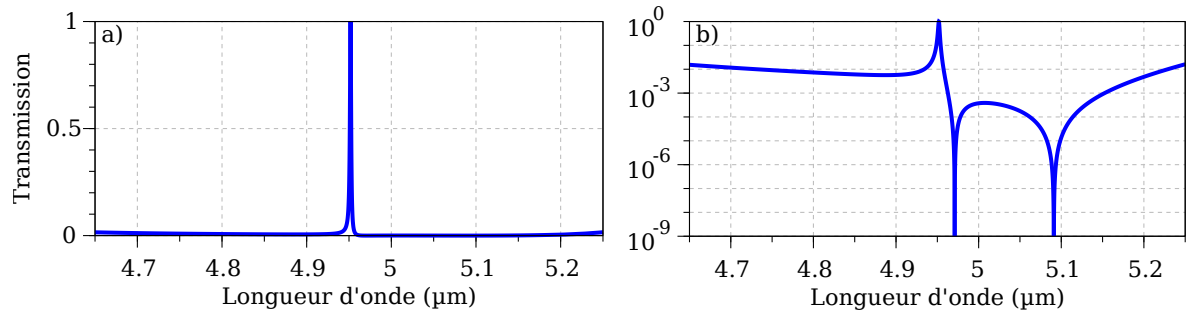
FIGURE 2.12 – Courbe de transmission sur une échelle a) linéaire et b) logarithmique d'un filtre ZCG de transmission proche de 100% dans le moyen infrarouge. Les dimensions du filtre sont les suivantes : d_w = 0.84 \mu\text{m} , d_g = 0.87 \mu\text{m} , \Lambda = 2.703 \mu\text{m} et f = 0.24 .
