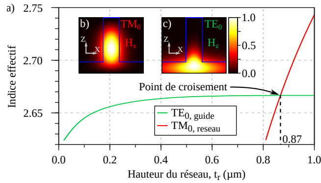
FIGURE 3.12 – a) Indice effectif des modes TE (courbe verte) et TM (courbe rouge) en fonction de l'épaisseur des créniaux du réseau t_r . Dans les encarts b) et c) sont respectivement présentés le carré de l'amplitude des composantes x et y du champ magnétique dans une période du réseau pour t_r = 0.87 \mu\text{m} (point de croisement des courbes de dispersion). Le calcul est effectué à \lambda = 3.6179 \mu\text{m} . À cette longueur d'onde, les indices des matériaux sont les suivants : n_{\text{Ge}} = 4.713 et n_{\text{CaF}_2} = 1.413 . Les dimensions fixes du filtre sont les suivantes : t_s = 0.22 \mu\text{m} , \Lambda = 1.255 \mu\text{m} et f\Lambda = 321.3 \text{ nm} .
