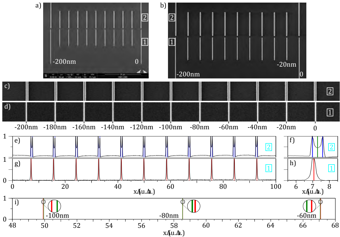
FIGURE 4.9 – Illustration de la méthode de mesure du désalignement entre les niveaux à partir de l'image MEB d'un vernier de résolution 20 nm orienté dans la direction x . Le niveau 1 est le niveau gravé, le niveau 2 est un niveau de résine. Le décalage mesuré correspond à la position relative du second niveau par rapport au premier niveau. Le désalignement entre les deux niveaux est estimé à -80 \pm 20 nm.
