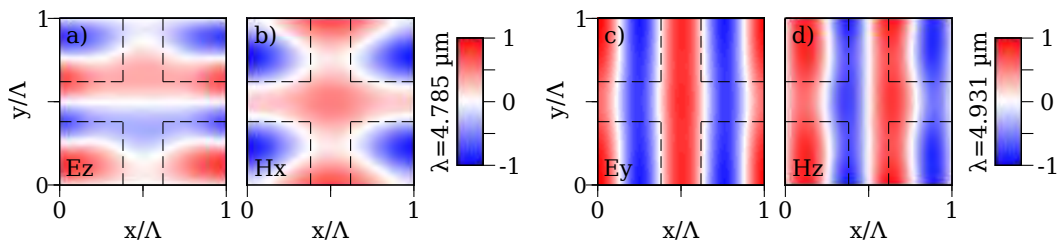
FIGURE 3.9 – Partie réelle des composantes selon z des champs \vec{E} et \vec{H} dans le plan (Oxy) du guide de cote z = 0.42 \mu\text{m} sur une période du réseau aux longueurs d'ondes respectives des deux résonances de la figure 3.8f : 4.785 et 4.931 \mu\text{m} . Les données sont normalisées au maximum de la partie réelle du champ associé dans le volume de la structure. Le champ \vec{E}_i est orienté selon y .
