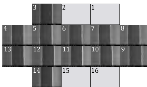
FIGURE 4.18 – Cartographie MEB sous incidence normale des réseaux insolés du second niveau de photolithographie. La bande sombre dans chaque motif correspond à l'ouverture dans la couche d'ECI. Les conditions d'insolation et de développement sont les conditions standards. Le numéro indiqué sur chaque image définit l'ordre d'insolation tel qu'effectué par le stepper. Aucun cliché n'a été pris au niveau des motifs non conformes.
