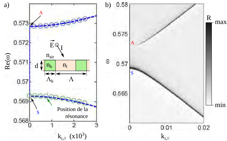
FIGURE 1.23 – Tiré de [92]. a) Courbe de dispersion donnant la partie réelle de la pulsation en fonction de la composante tangentielle du vecteur d'onde incident pour un réseau 1D suspendu dans l'air dont la structure est illustrée en encart. b) Cartographie de l'efficacité de réflexion en fonction de la pulsation de l'onde incidente et de la norme du projeté du vecteur d'onde incident. Les paramètres de la structure considérée sont : n_h = 2.05 , n_l = 1.97 , \Lambda_h/\Lambda = 0.4 , \Lambda = 1 \mu m , d = 0.5 \mu m . L'onde incidente est polarisée TE, l'indice de l'air est égal à 1.
