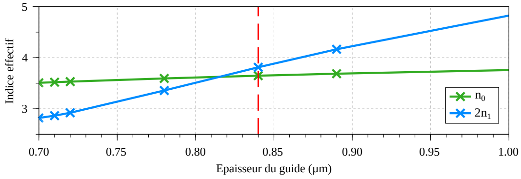
FIGURE 2.9 – Détermination graphique de l'épaisseur du guide : le point de fonctionnement optimal, indiqué par les tirets rouges, se situe légèrement au-delà du point de croisement où n_0 = 2n_1 .
