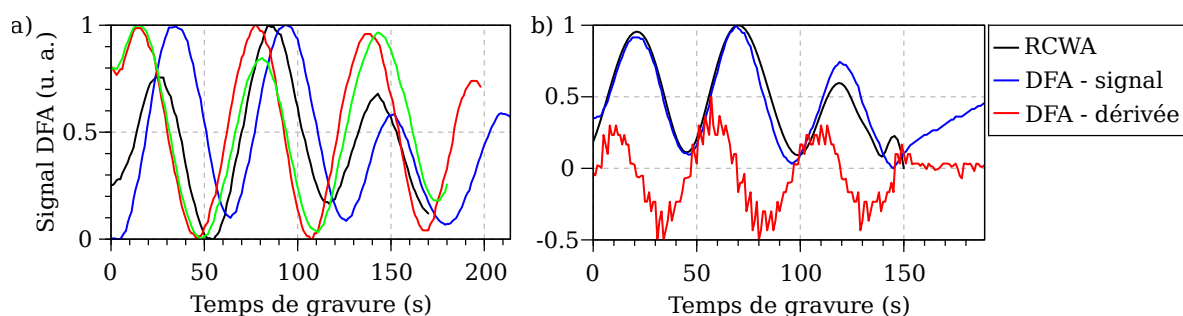
FIGURE 4.22 – Suivi DFA de la gravure dans un réseau. a) Courbes expérimentales de la gravure de substrats de Si ayant subi des étapes de photolithographie identiques. b) Comparaison entre des données de suivi DFA théoriques (courbe noire) et expérimentales (courbes bleues et rouge) de la gravure d'un empilement de couches minces de Ge avec couches d'arrêt.
