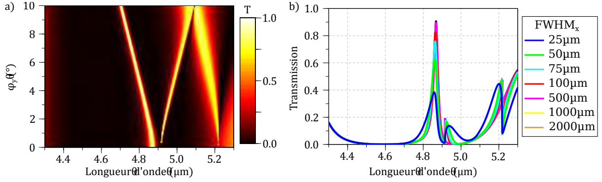
FIGURE 2.30 – a) Cartographie de la transmission T(\lambda, \phi_y) du filtre ZCG MIR doublement corrugué de référence en fonction de la longueur d'onde du rayonnement incident et de l'angle d'incidence \phi_y . b) Spectre du filtre calculé pour différentes tailles de faisceau. Les dimensions géométriques du filtre sont les suivantes : d_w = 0.84 \mu\text{m} , d_g = 0.87 \mu\text{m} , h = -0.1 \mu\text{m} , \Lambda = 2.703 \mu\text{m} et f = 0.24 .
