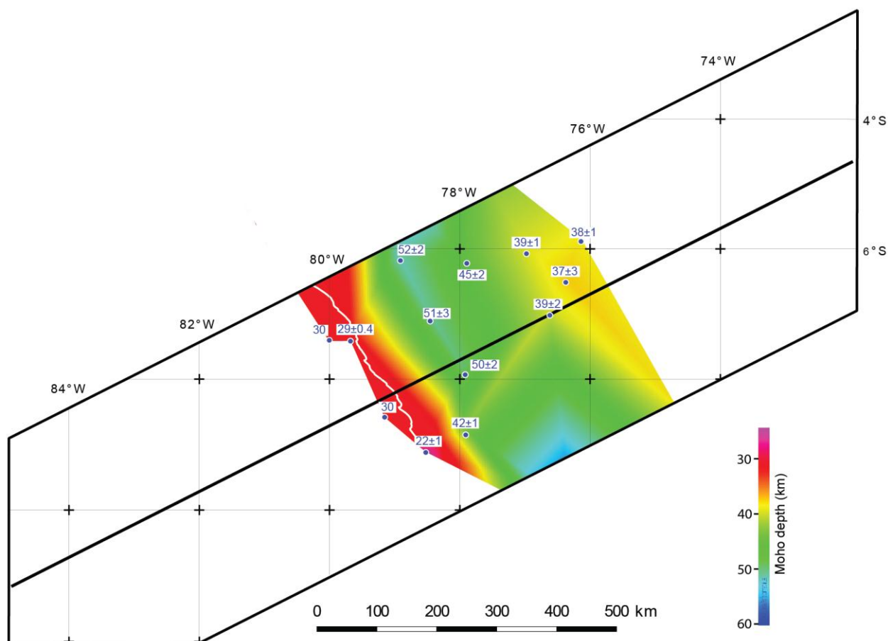
Figure III-4 : Carte des profondeurs du Moho, calculées par interpolation des analyses de fonction récepteur (Condori et al., 2017) et de la sismique réfraction (Hussong et al., 1976).
