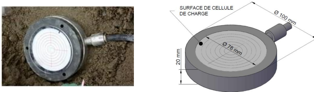
Figure 28 : Jauge de contrainte électrique typique
