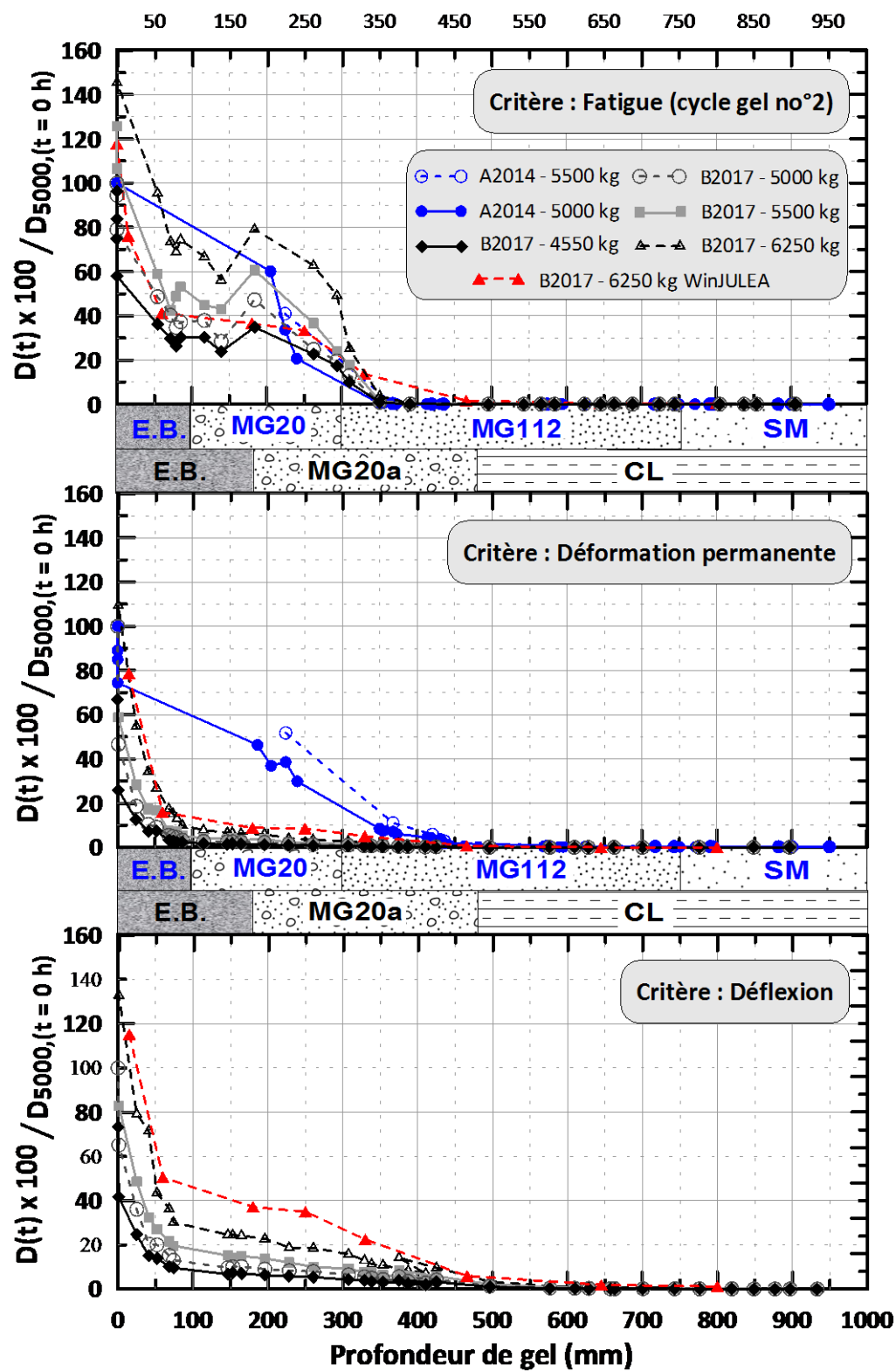
Figure 76 : Analyse des dommages relatifs selon les critères de fatigue, déformation permanente et déflexion pour les chaussées A 2014 et B 2017
