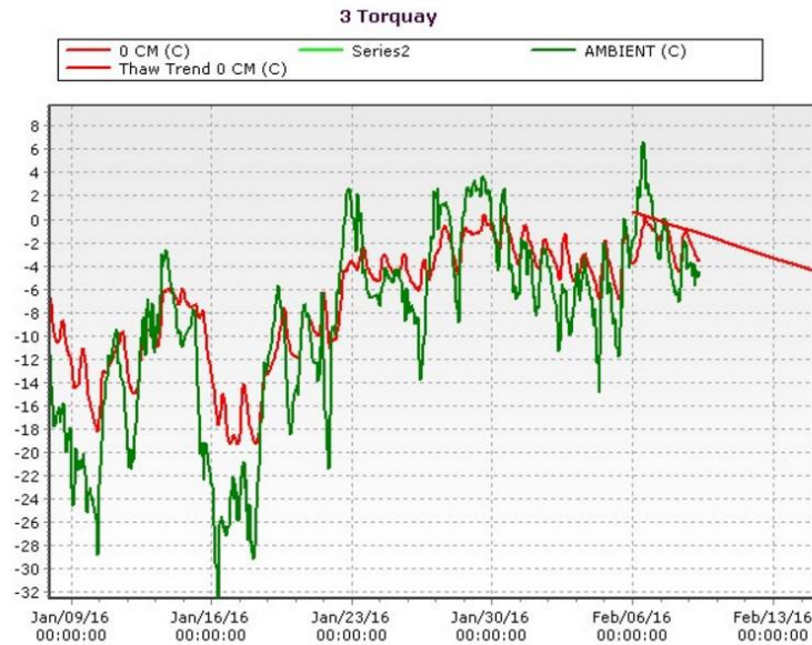
Figure 22 : Température de l'air et de la surface du pavage à la station Torquay (http://data.lakewood.com/livedata/saskHighways/torquay/)
