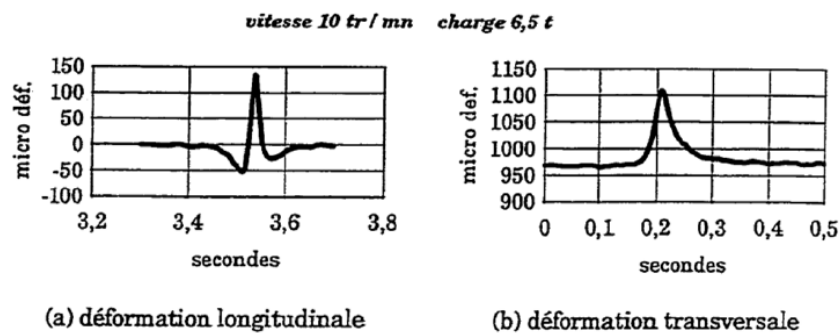
Figure 4 : Déformations transversales et longitudinales mesurées dans une couche d'enrobé sous le passage d'une roue (Doucet, 1999)
