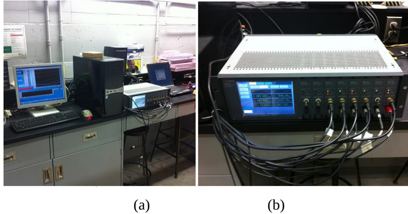
Figure 33 : (a) Systèmes d’acquisitions National Instruments (électrique et optique) et (b) système d’acquisition de données optique ProSens PSC-D
