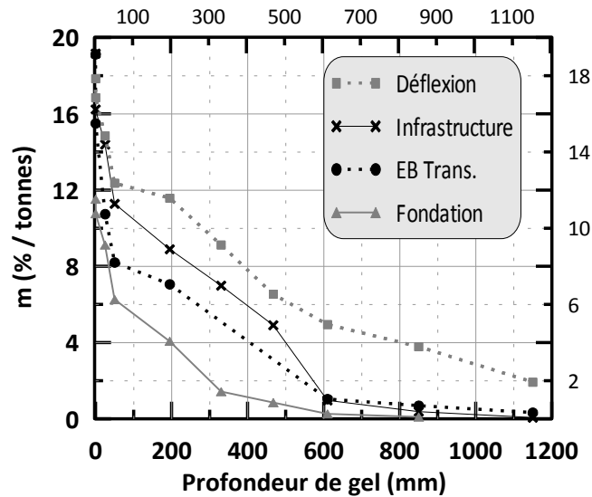
Figure 58 : Relation entre la pente m selon la profondeur de gel
