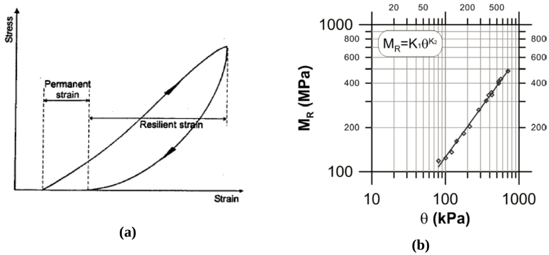
Figure 6 : (a) Relation contraintes/déformations d'un matériau granulaire (Extrait de Lekarp et coll. (2000a) (b) Variation du M_R d'un matériau granulaire selon les contraintes totales ( \theta ), (Extrait de Bilodeau & Doré (2013)
