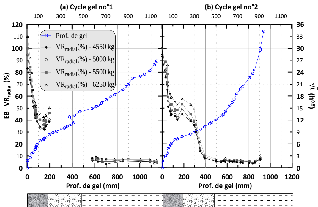
Figure 54 : Déformations transversales à la base de l'enrobé bitumineux pour le cycle de gel no°1 (a) et no°2 (b)
