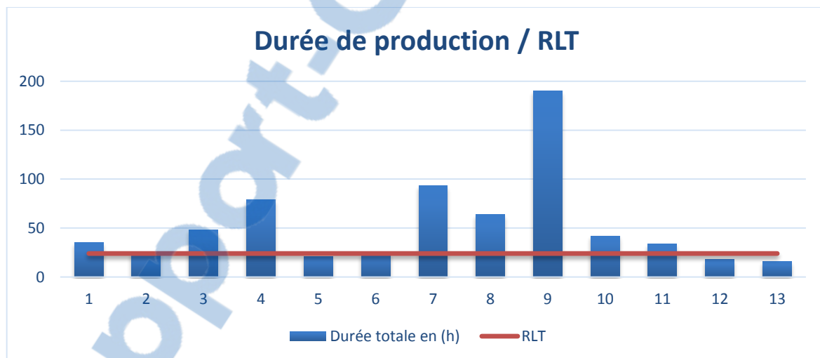
Figure 42 Étude capacitaire par machine twist
