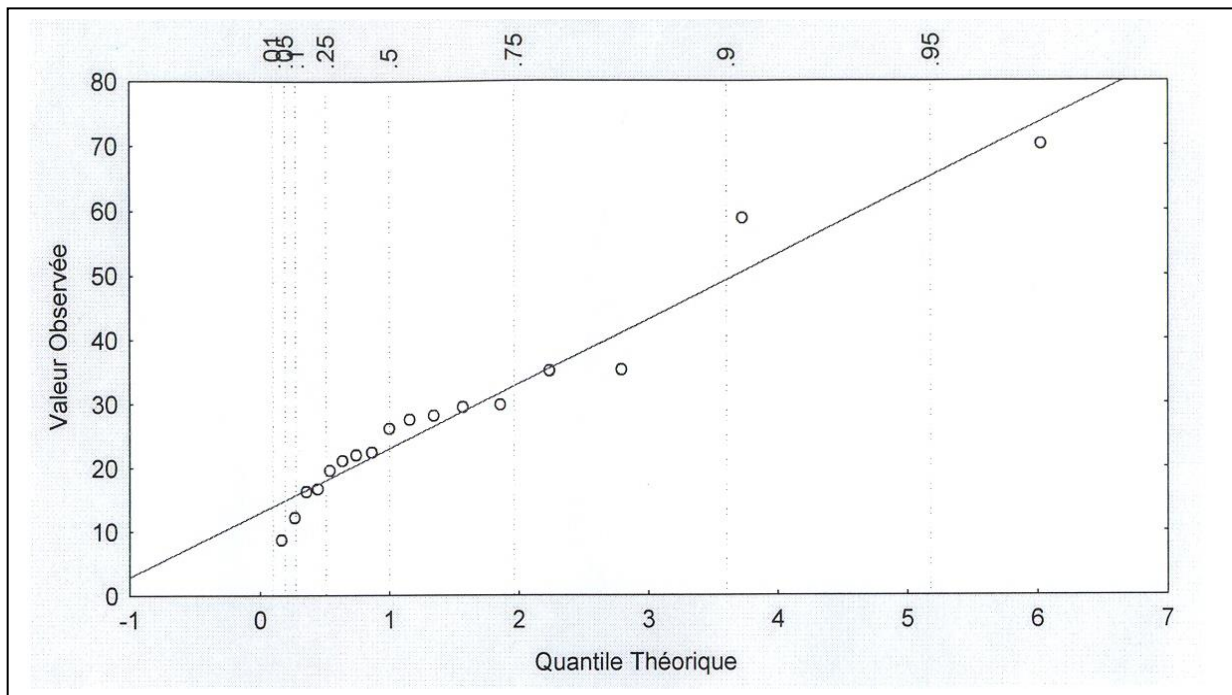
Figure N°32 : Distribution de la loi « log normale » des débits dérivables sur la prise de la Tafna (1981-1997) « Y = 12,933 + 10,078X + \zeta »
