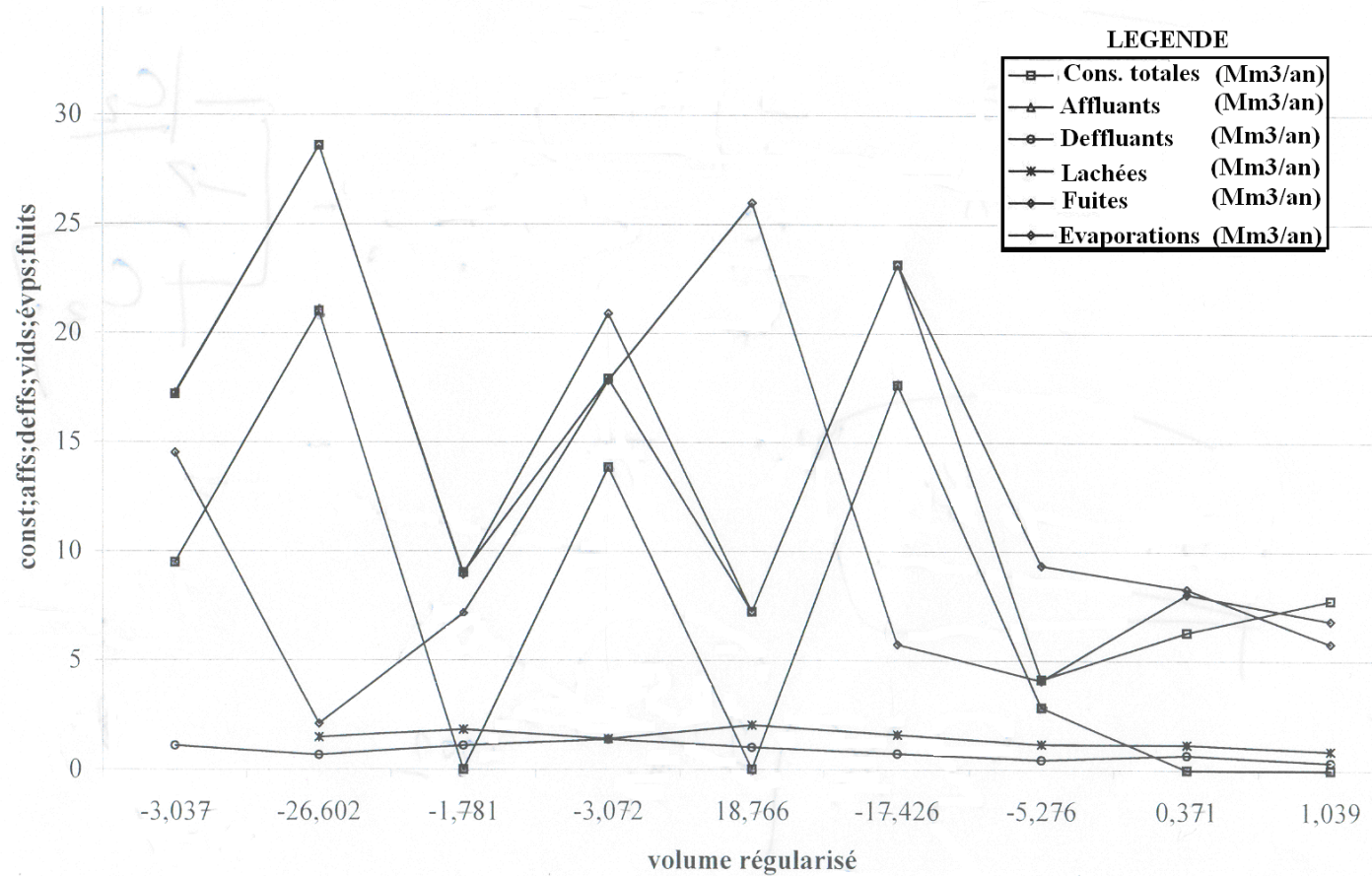
Figure N° 23: volume régularisé barrage sidi abdelli (1991-1999) (Mm3/an)
