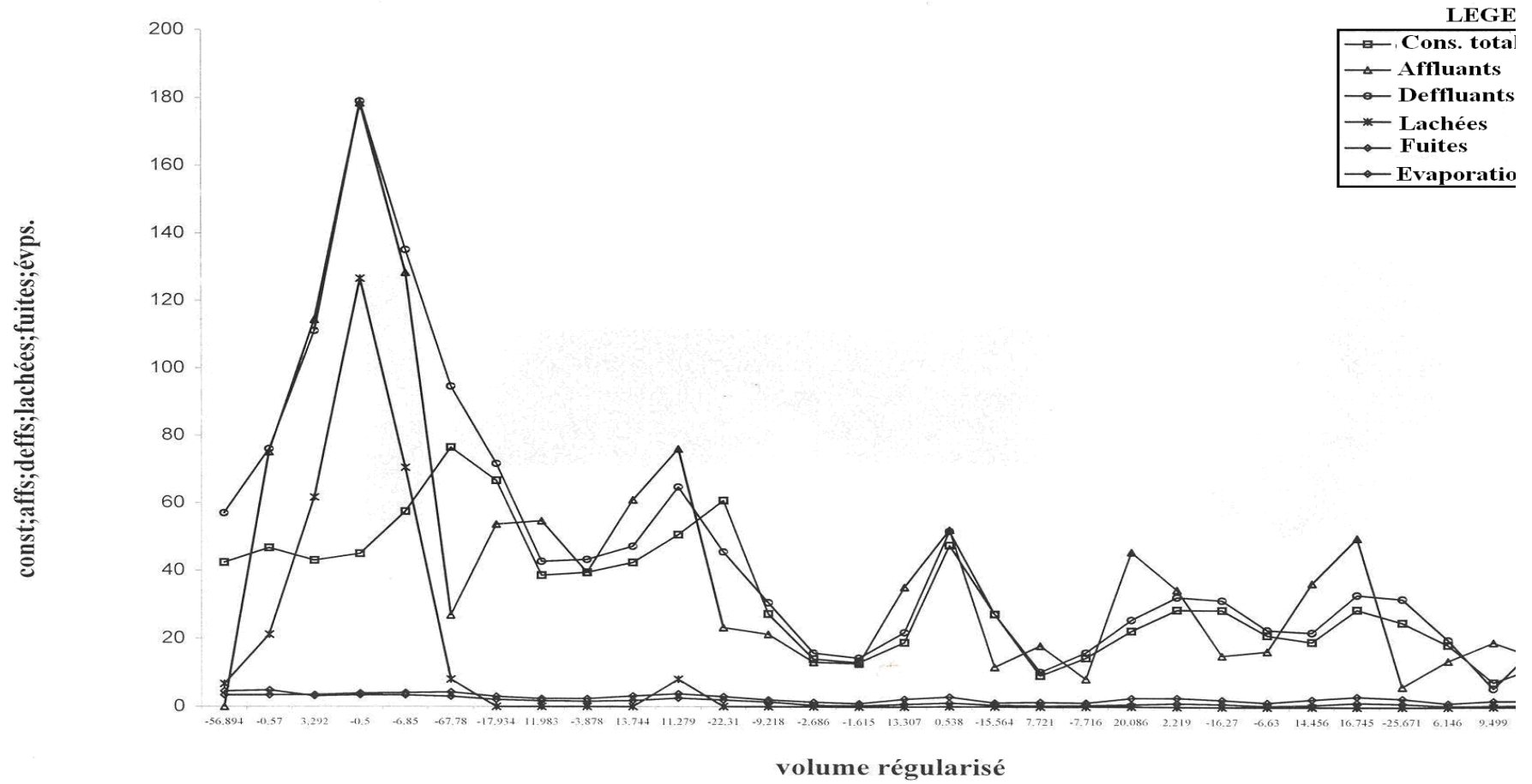
Figure 21 : volume régularisé barrage beni bahdel(1970-1999) (Mm3/an)
