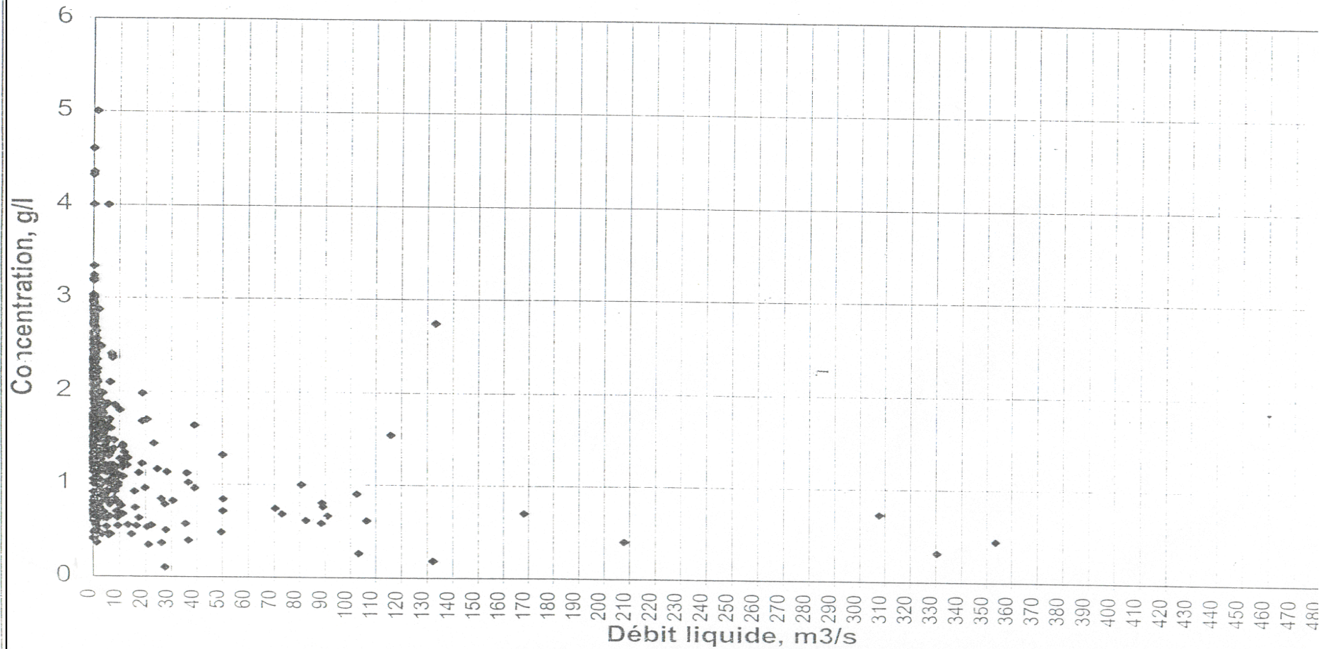
Figure 35 : Ts en fonction du débit liquide dans l'oued TAFNA à la Pierre du chat, Algérie, de 09/1977 à 05/1991
