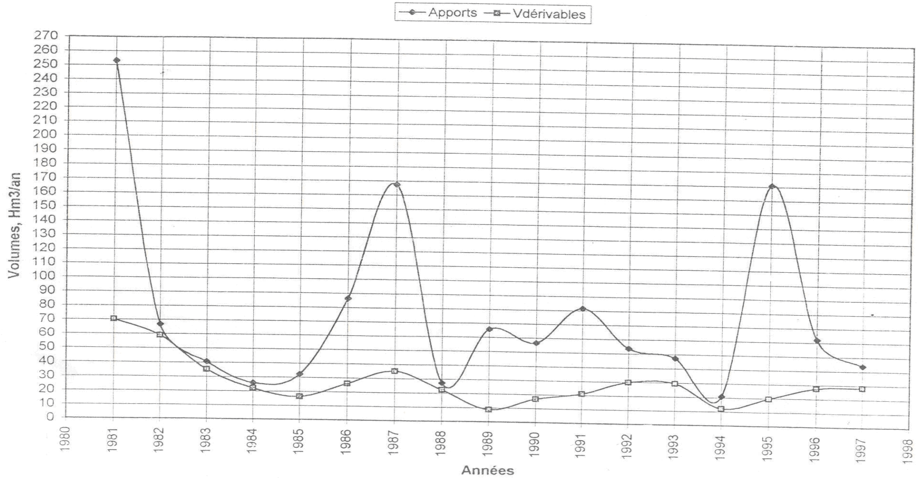
Figure 38 : Apports à la pierre du chat et Volumes annuels dérivables sur la TAFNA
