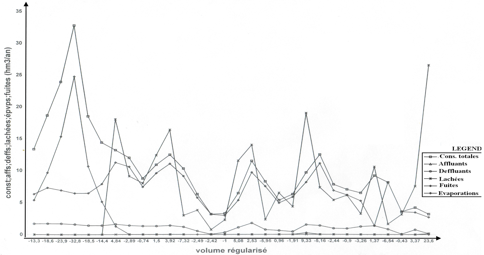
Figure 22 : volume régularisée barrage meffrouche(1970-1999) (Mm3/an)
