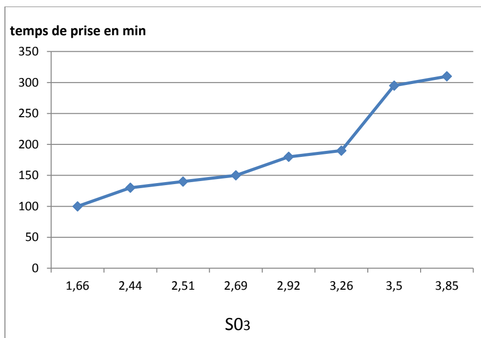
Figure 25: Courbe de l'évolution de la prise initiale (en min) en fonction du pourcentage en SO 3
