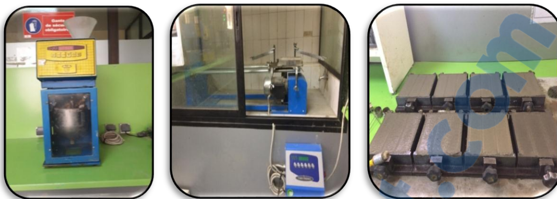
Figure 20 : malaxeur/ table à choc/ moules
