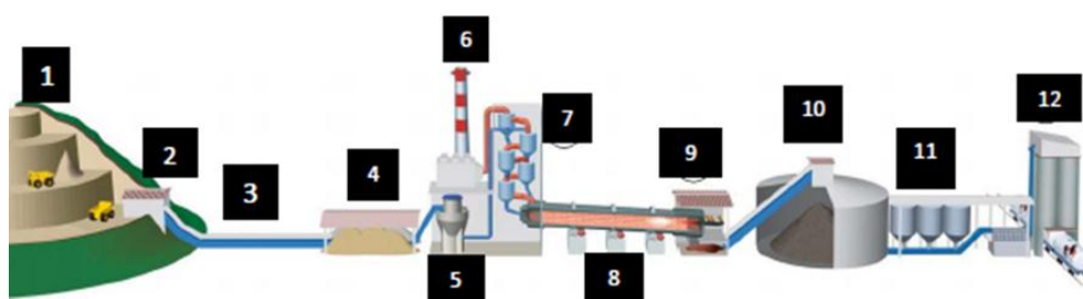
Figure 2 : Schéma simplifié du procédé industriel de production du ciment
