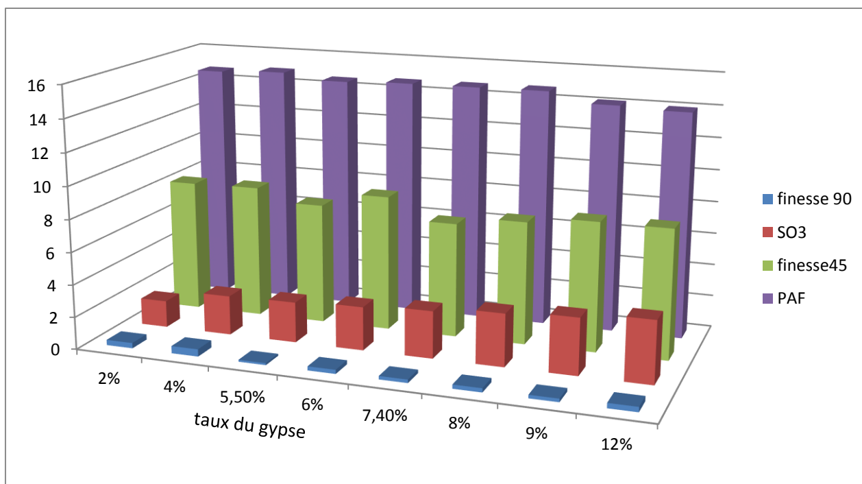
Figure 24: résultats des analyses chimiques du ciment en fonction de la variation du taux de gypse
