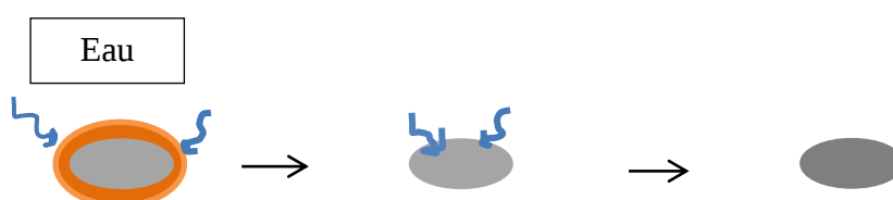
Figure 26: Schéma simplifié illustrant la prise après contact du ciment avec l'ajout du gypse et de l'eau
