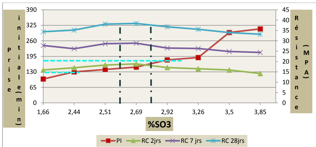
Figure 28: Résistances à la compression à 2j, 7j et 28j et le temps de prise du ciment en fonction du %SO 3
