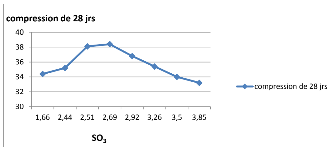
Figure 27:Résultats de la compression de 28 jours en fonction du % en SO 3
