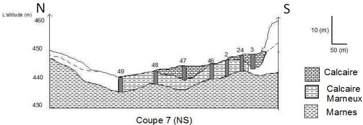
Figure 1 : Coupe 7 avec l'orientation (NS)
