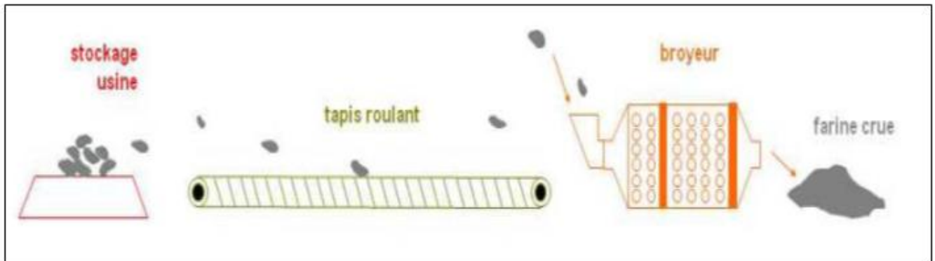
➤ Figure 10 : Description du broyage du cru (Compte rendu de la mission à la société de ciments Artificiels de Meknès CADEM –avril 1988 .)
