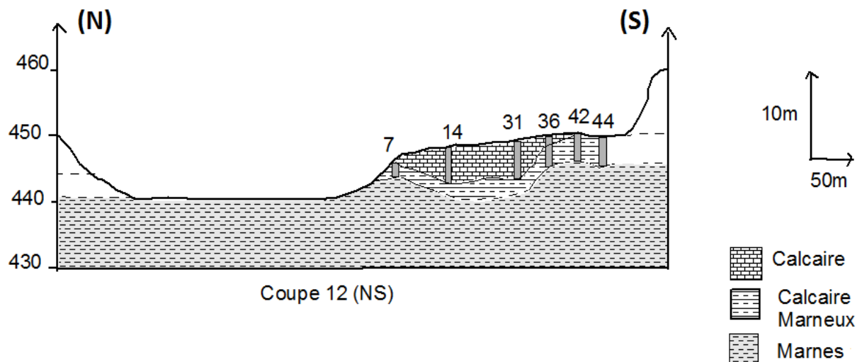
Figure6 : Coupe 12 avec l'orientation (NS).
