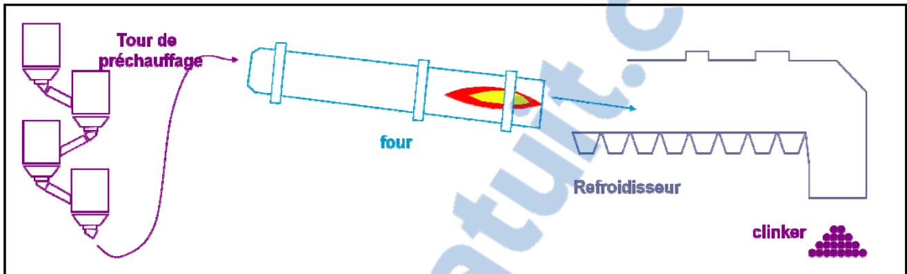
Figure 12 : Description de la ligne de cuisson (Compte rendu de la mission à la société de ciments Artificiels de Meknès CADEM –avril 1988.)
