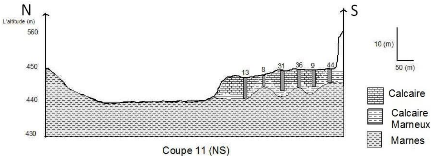
Figure 5: Coupe 11 avec l'orientation (NS)
