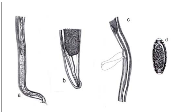
Fig. 2: Capillaria plica
