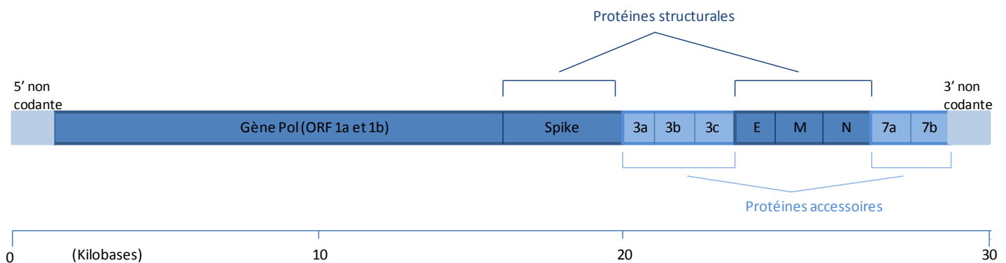
Figure 2 : Organisation du génome des coronavirus félins (BROWN et al. , 2009)
