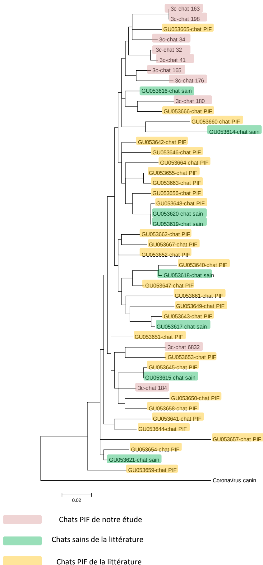
Figure 14 : Arbre monophylétique de probabilité maximale pour la protéine issue du gène 3c
