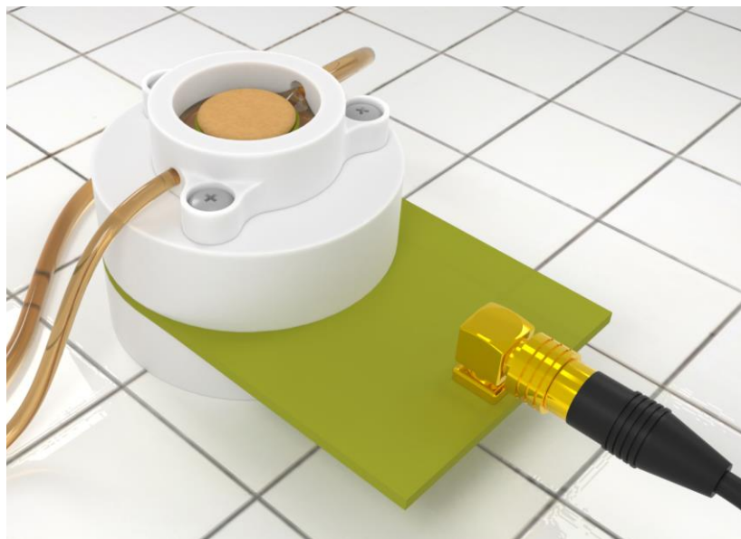
Figure LXXXVI Visuel du biocapteur ex vivo
