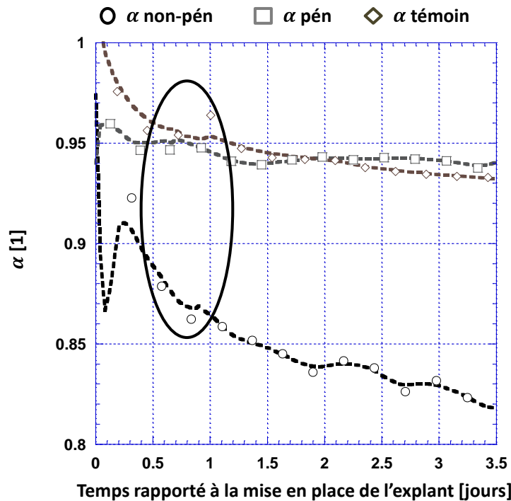
Figure LXXIX Évolutions du coefficient de structure pour les bornes de l'attribut péné rant par rapport à un explant type, l'instant de traitement est encerclé en noir
