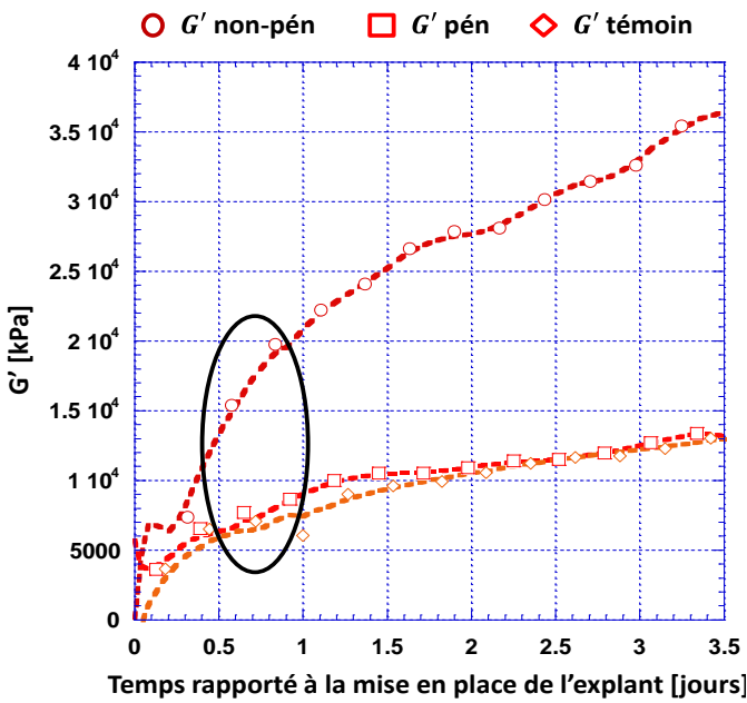
Figure LXXVII Évolutions du module élastique pour les bornes de l'attribut péné rant par rapport à un explant type, l'instant de traitement est encerclé en noir
