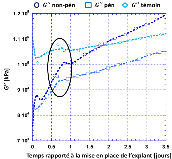
Figure LXXVIII Évolutions du module visqueux pour les bornes de l'attribut péné rant par rapport à un explant type, l'instant de traitement est encerclé en noir
