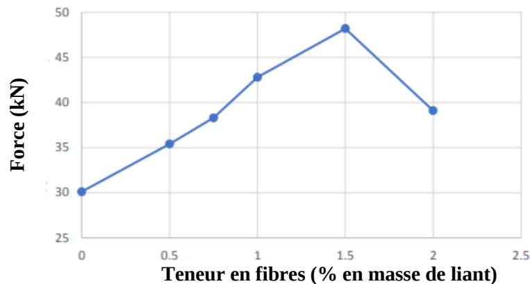
Figure I-27: Capacité portante maximale en flexion en fonction du dosage de fibres de polypropylène (Orouji et al., 2021)
