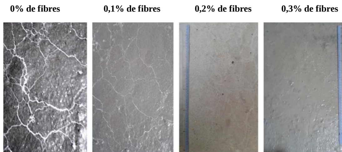
Figure I-23: Comparaison de la fissuration due au retrait plastique entre une formulation cimentaire non fibrée et des formulations renforcées par plusieurs dosages en fibres de polypropylène (Sadiqul Islam and Gupta, 2016)
