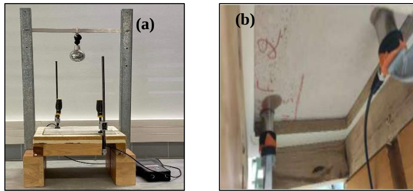
Figure V-4: Principe de mesure de la vitesse de la propagation des ondes ultrasonores (a) vue de face et (b) vue de dessous
