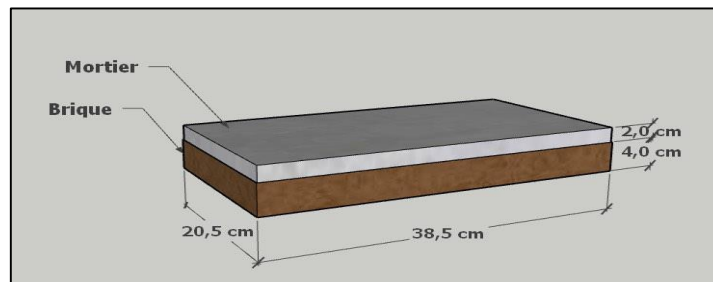
Figure IV-14: Dimensions de la brique et du rechargement en mortier
