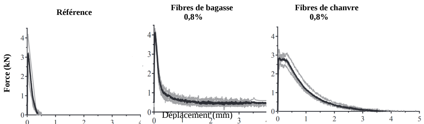
Figure I-35: Courbes Force – Déplacement en flexion 3 points (Ruano et al., 2020)
