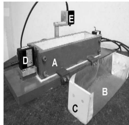
Figure III-14: Dispositif de mesure des déformations plastiques : moule 7x7x28 cm (A), enveloppe (B+C), capteurs laser (D et E) (Turcry, 2004)
