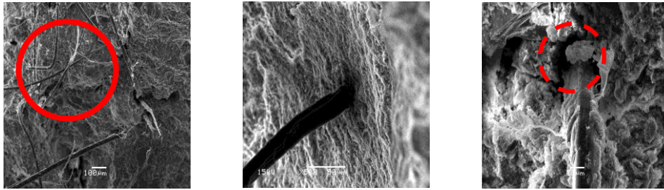
Figure V-27: Analyse MEB du mortier pouzzolanique à 28 jours avec plusieurs grossissements
