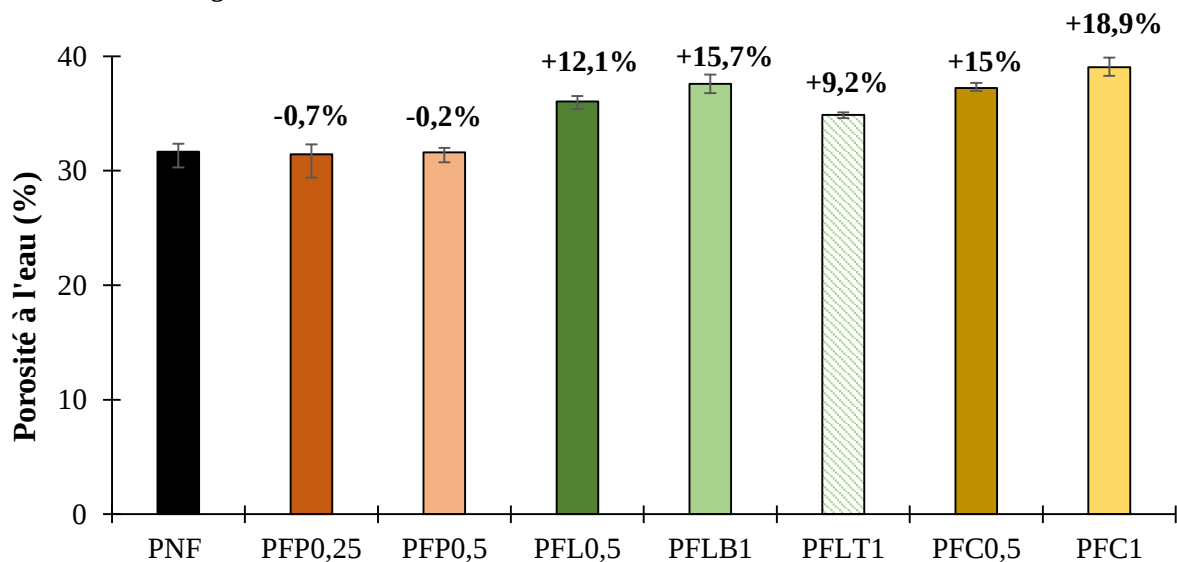
Figure V-22: Porosité accessible à l'eau des formulations cimentaires
