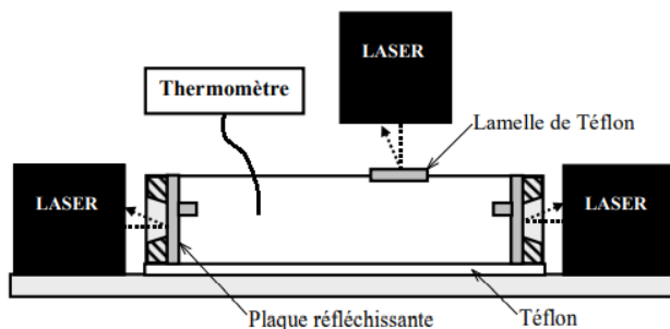
Figure III-13: Dispositif de mesure des déformations plastiques (Turcry, 2004)
