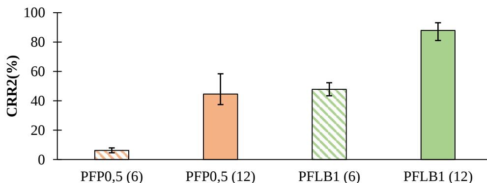
Figure IV-20: Comparaison du CRR2 des formulations pouzzolaniques avec une longueur de fibres de 6 et 12 mm.
