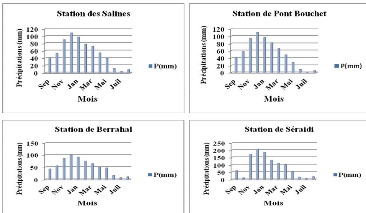
Fig.16: Précipitations moyennes mensuelles interannuelles pour les 04 stations (Les Salines, Pont Bouchet, Berrahal et Seraïdi)
