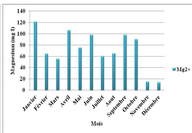
Fig. 67: Evolution mensuelle de magnésium (Barrage Mexa, année 2017)
