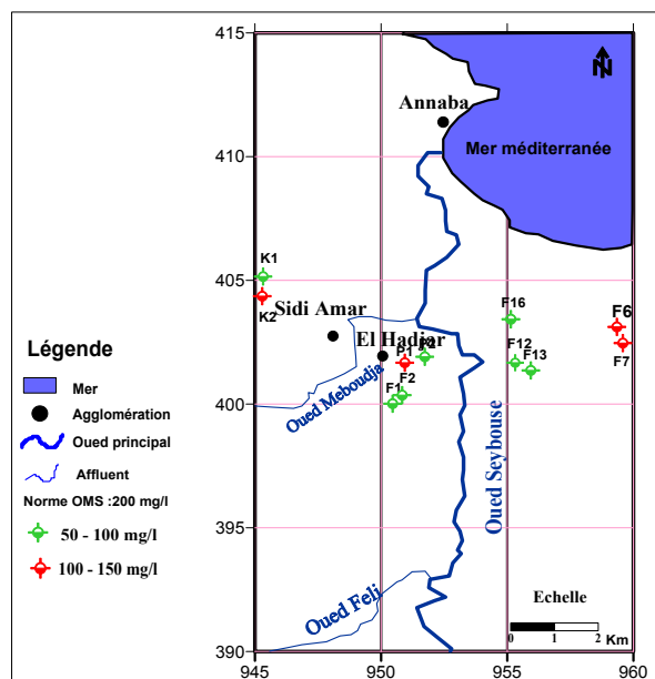
Fig. 45 : Carte de la distribution spatiale de magnésium (Forages et puits, Septembre 2017)
