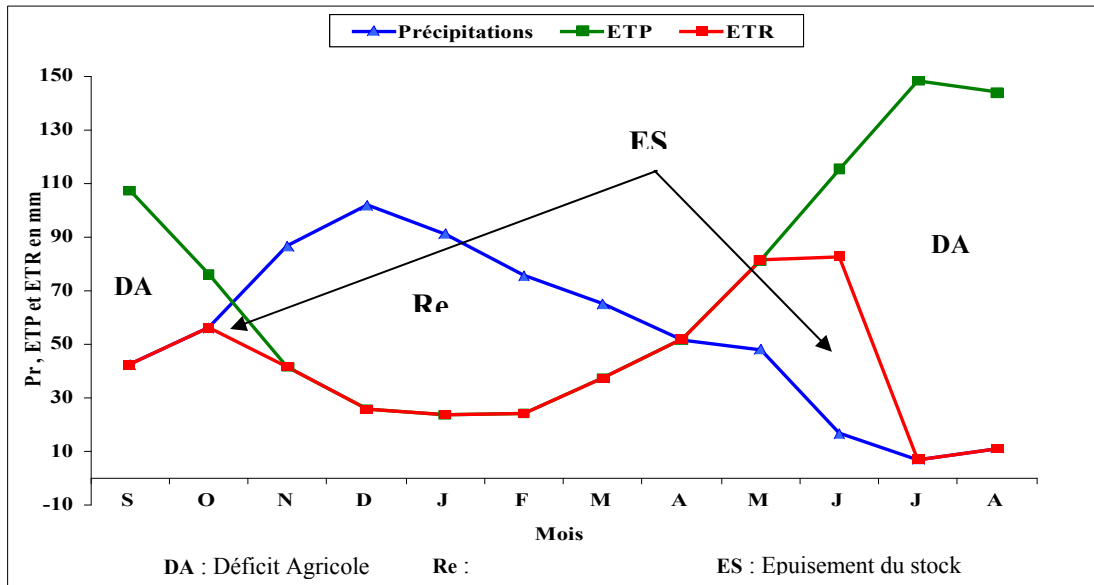
Fig. 29: Représentation graphique du bilan hydrique selon THORNTHWAITE, Station de Berrahal, période (1985-2012)
