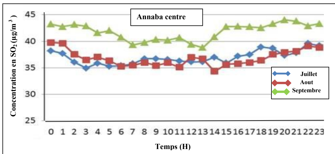
Fig. 108: Moyennes horaires des concentrations en dioxyde de soufre enregistrées en juillet, août et septembre (années 2012, 2013 et 2014) pour la station d'Annaba ville
