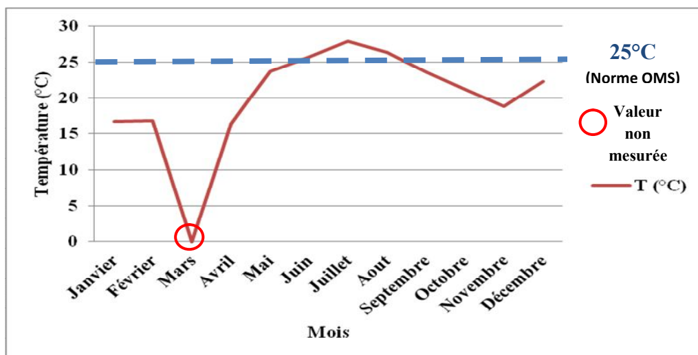
Fig. 61: Variations mensuelles des températures (Eaux de barrage Mexa, année 2017)
