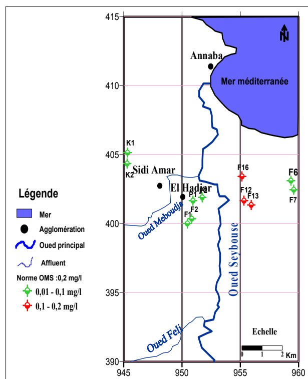
Fig. 52: Carte de la distribution spatiale des nitrites
