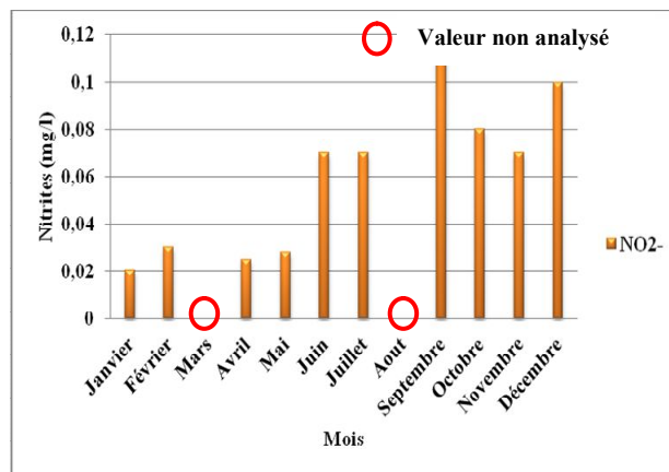
Fig. 71: Evolution mensuelle des nitrites (Barrage Mexa, année 2017)
