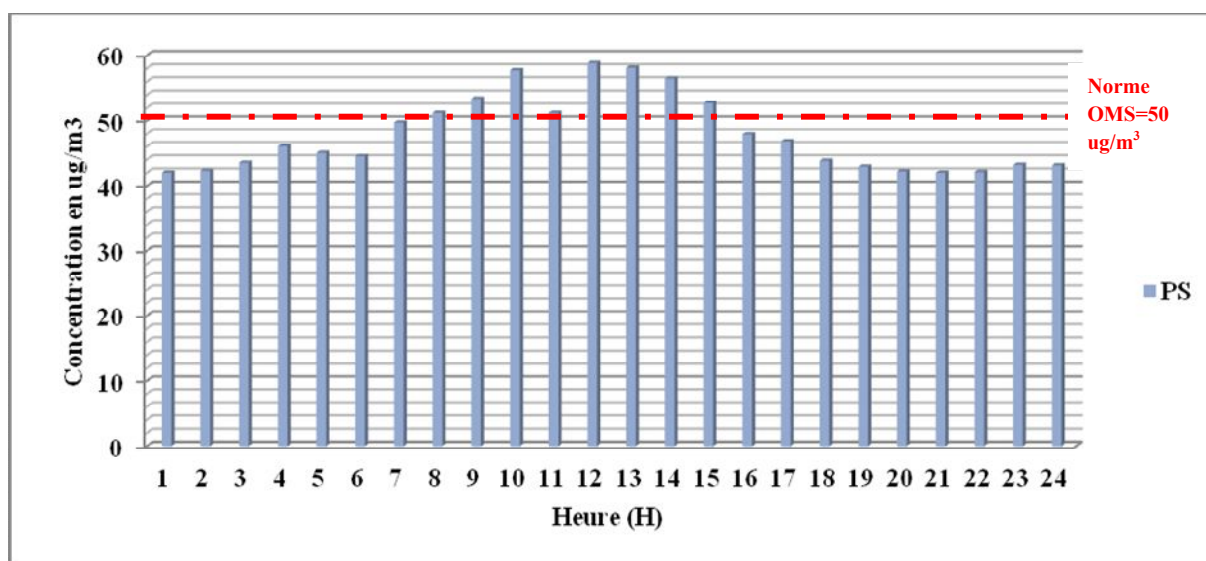
Fig. 100. Moyennes horaires des concentrations en poussières enregistrées en juillet, août et septembre (années 2012, 2013 et 2014) pour la station d'Annaba ville
