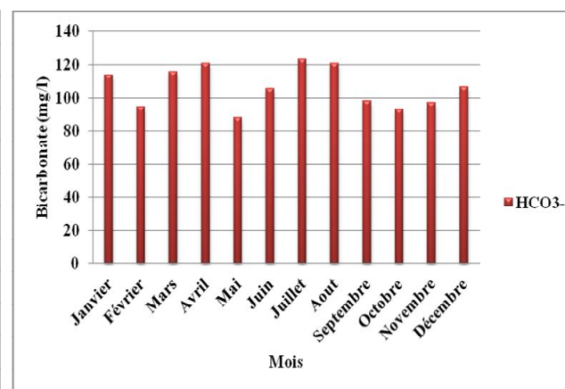
Fig. 69: Evolution mensuelle des bicarbonates (Barrage Mexa, année 2017)
