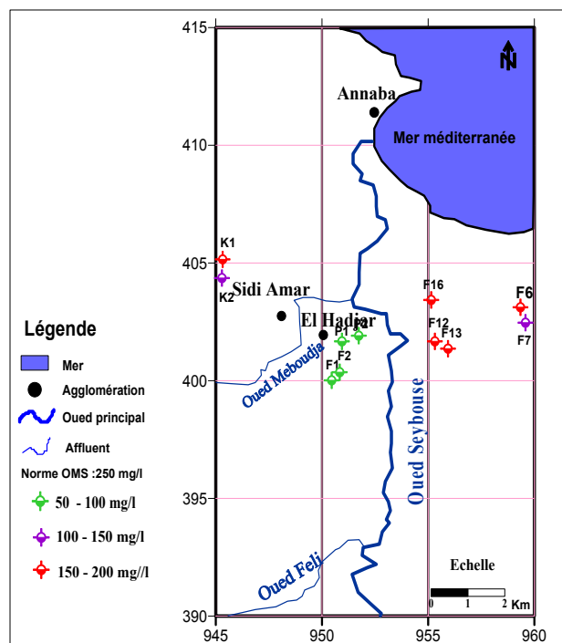
Fig. 49 : Carte de la distribution spatiale des sulfates (forages et puits, Septembre 2017)
