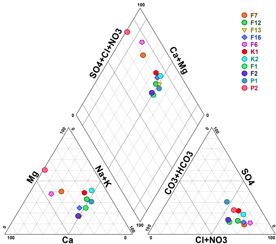
Fig. 56: Représentation de diagramme de Piper (Forages et puits, Septembre 2017)
