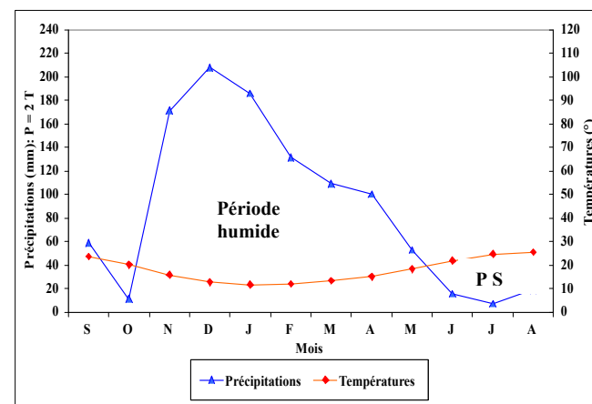
Fig.24 : Diagramme ombrothermique de la station de Seraïdi
