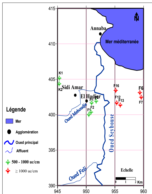
Fig. 41 : Carte de la distribution spatiale de la CE (Forages et puits, Septembre 2017)
