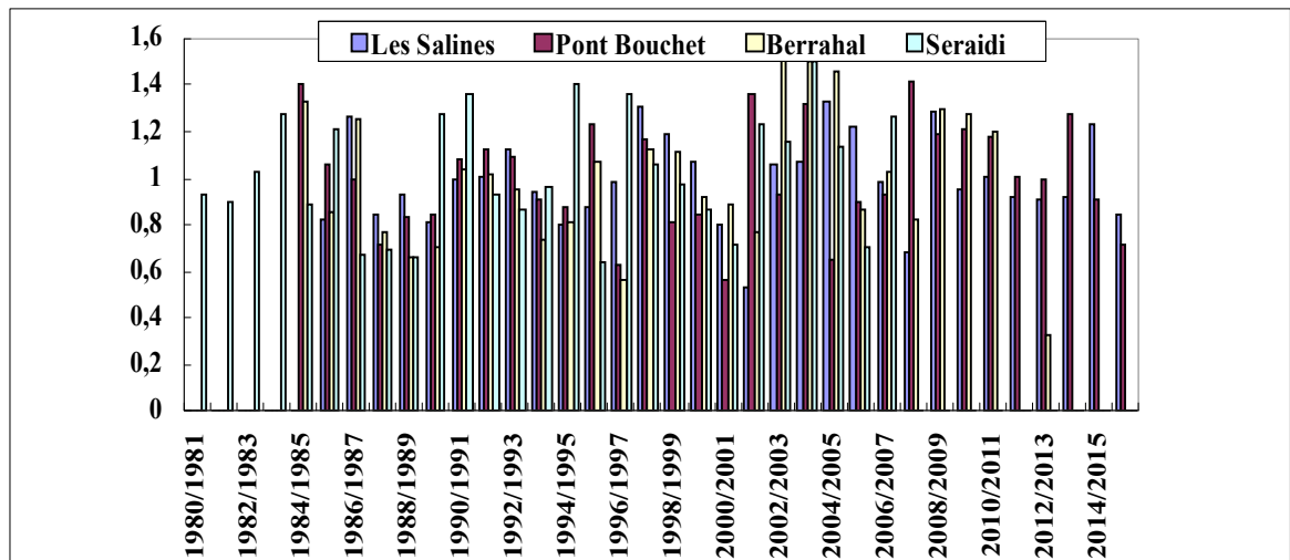
Fig.19: Les variations du coefficient pluviométrique pour les 04 stations (Les Salines, Pont Bouchet, Berrahal et Seraïdi) durant des périodes différentes.
