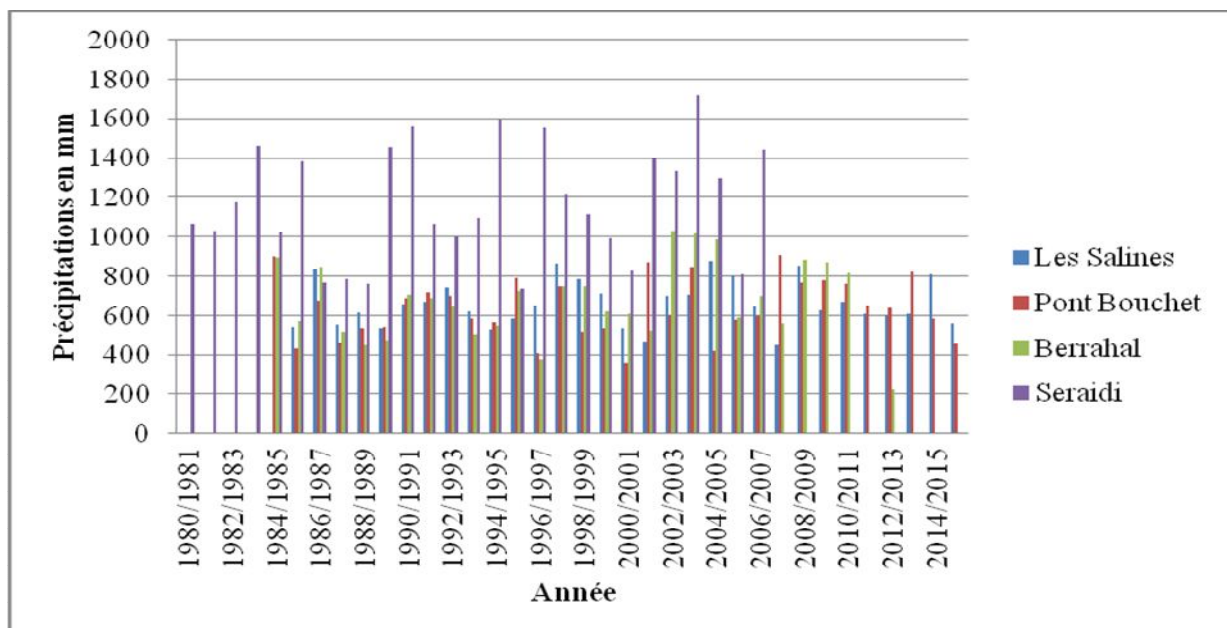
Fig.17: Précipitations moyennes inter- annuelles pour les 04 stations (Les Salines, Pont Bouchet, Berrahal et Séraïdi)
