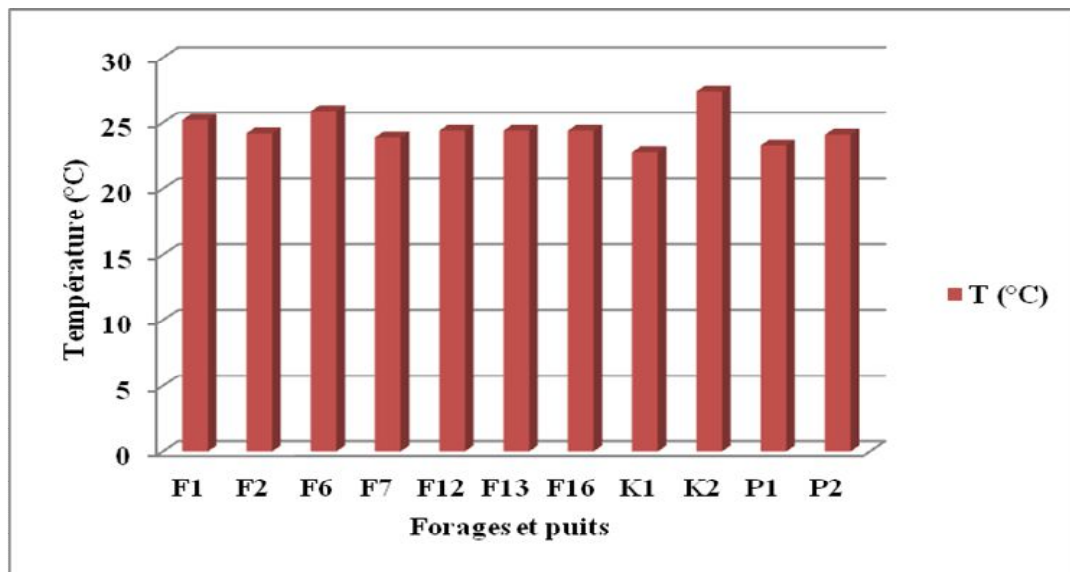
Fig. 38: Variation de la température dans les forages et puits (Sept. 2017)
