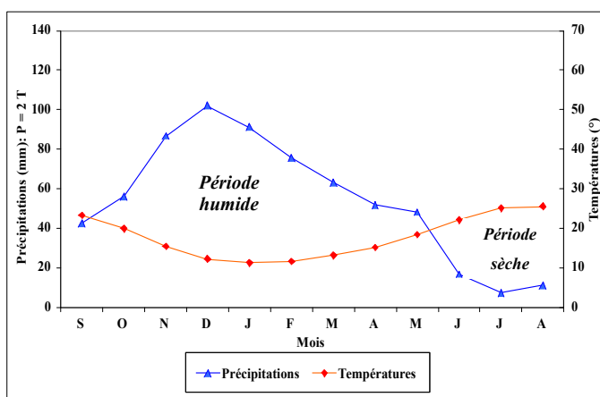
Fig.23 : Diagramme ombrothermique de la station de Berrahal
