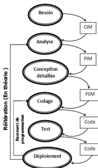
Figure 4.6. Processus de développement MDA [Mes 06]
