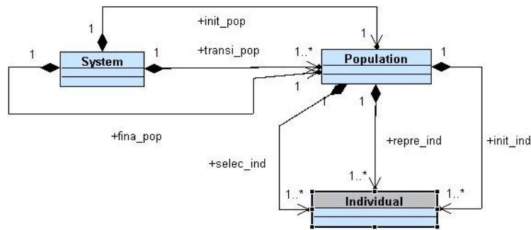
Figure 6.4. Représentation du modèle du voyageur de commerce (TSM)
