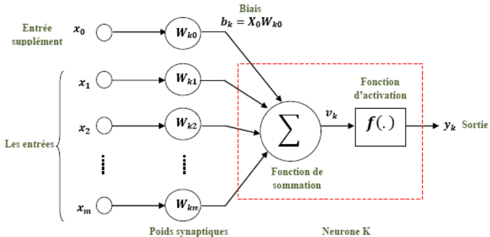
Figure 3.19. Neurone formel avec entrée supplémentaire
