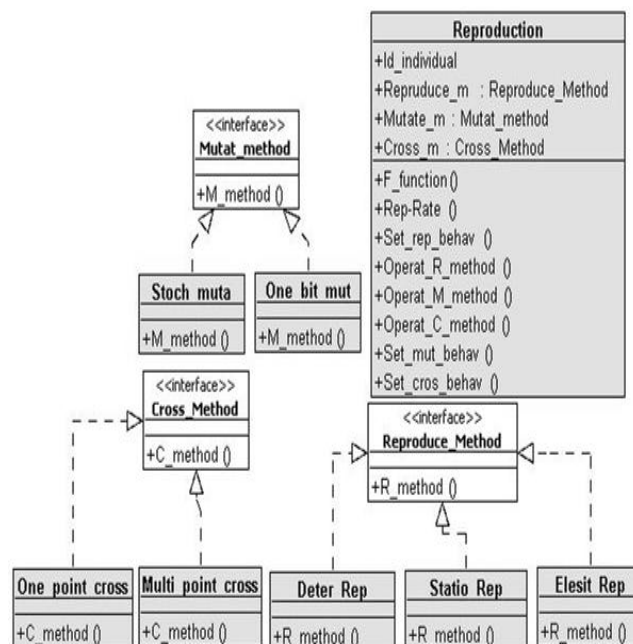
Figure 5.19. Vue du méta modèle de la reproduction
