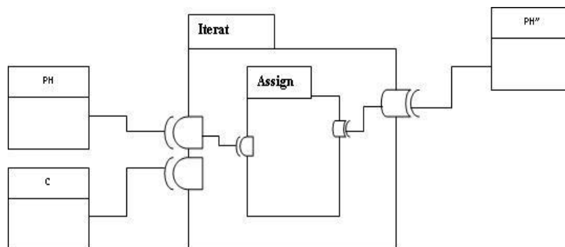
Figure 5.5. Représentation semi formelle des composants iterat et assign
