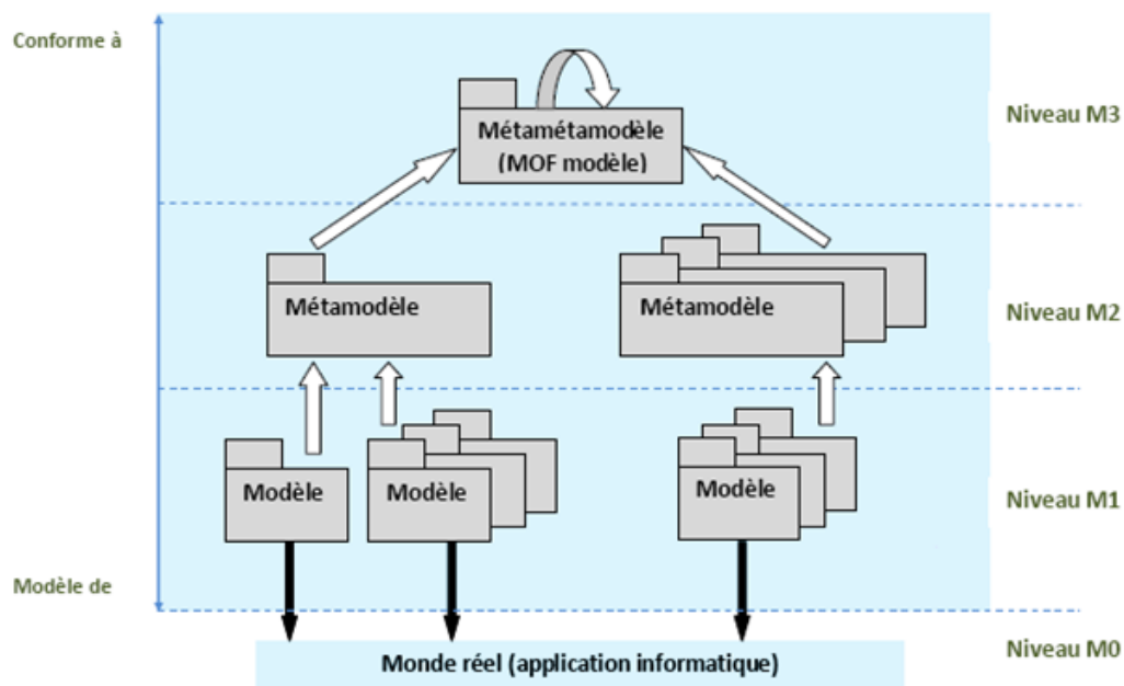
Figure 4.3. L'architecture à quatre niveaux de MDA
