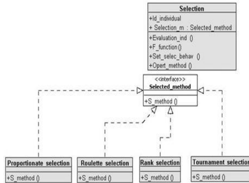
Figure 5.17. Vue du méta modèle de la sélection
