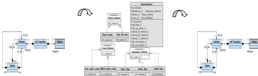
Figure 6.13. Représentation de la transformation reproduce de CLONCLAS.
