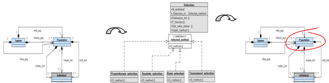
Figure 6.6. Représentation de la transformation de sélection du modèle TSM
