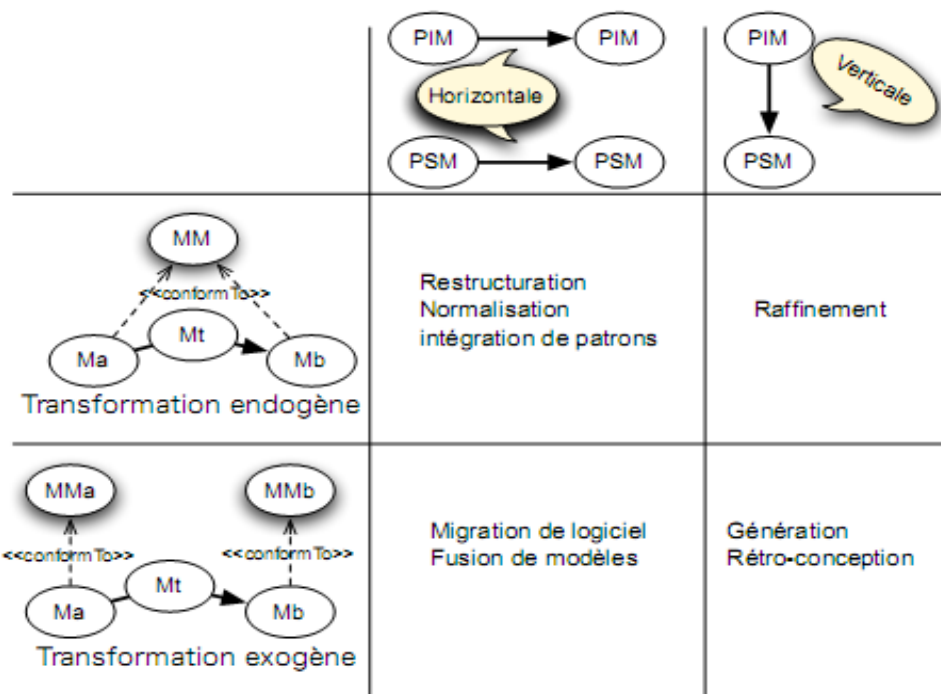
Figure 4.9. Types de transformation et leurs principales utilisations
