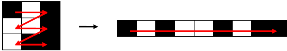
Figure 6.9. Image binaire → vecteur
