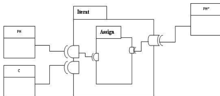
Figure 5.7. Représentation semi formelle des composants iterat et assign de la phylogénèse
