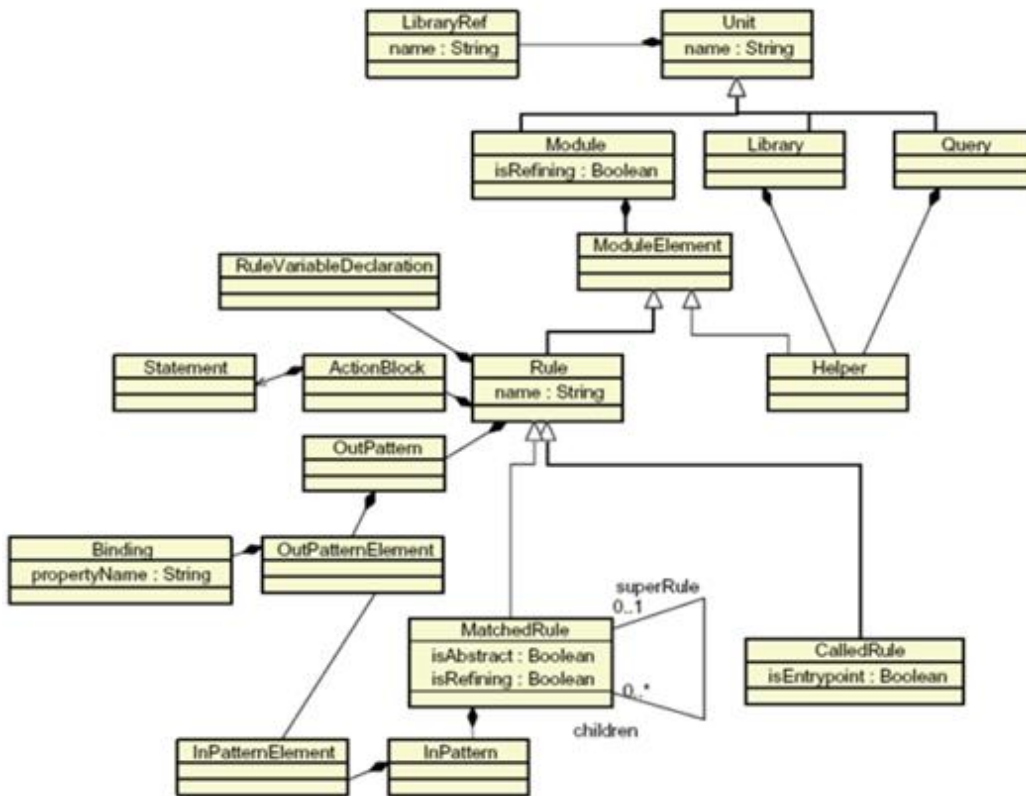
Figure 4.11. Métamodèle ATL simplifié
