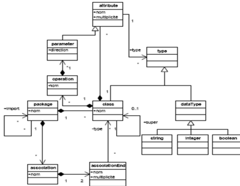
Figure 4.4. MOF (v1.4) sous forme de diagramme de classe [Bla 05].
