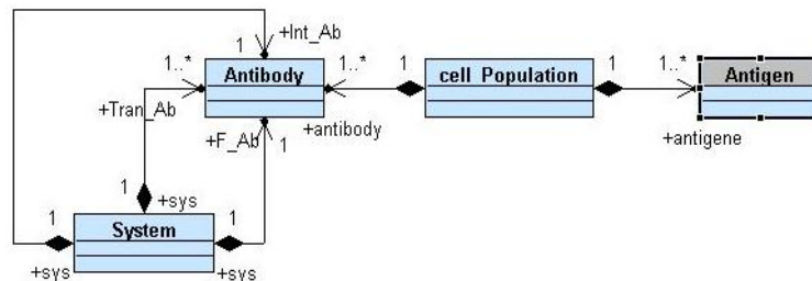
Figure 6.10. Représentation du modèle CLONCLAS
