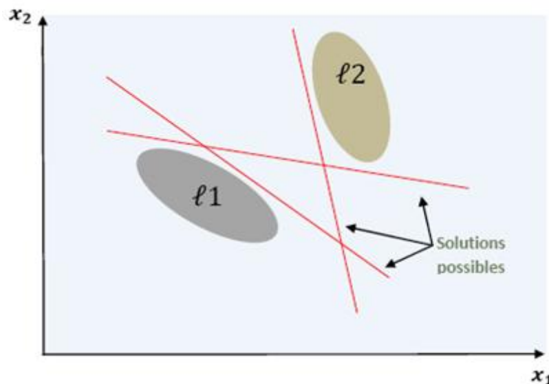
Figure 3.24. Exemple de solutions possibles de la règle du perceptron
