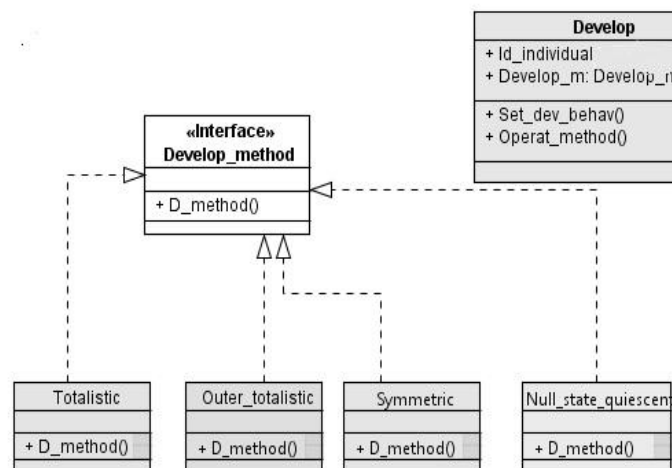
Figure 5.16. Vue du méta modèle de la développement
