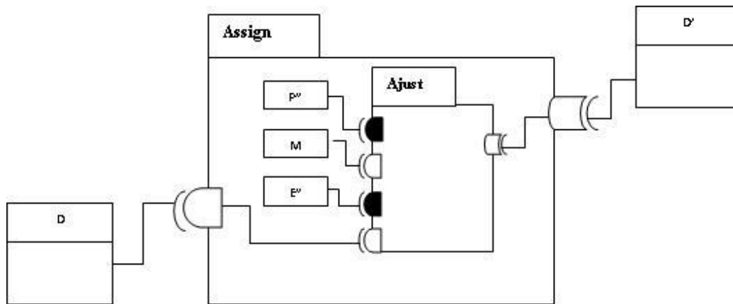
Figure 5.12. Représentation semi formelle des composants assign et Ajust
