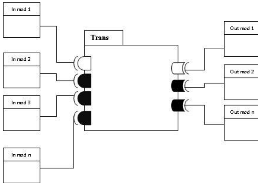
Figure 5.4. Représentation semi formelle de l'unité architecturale
