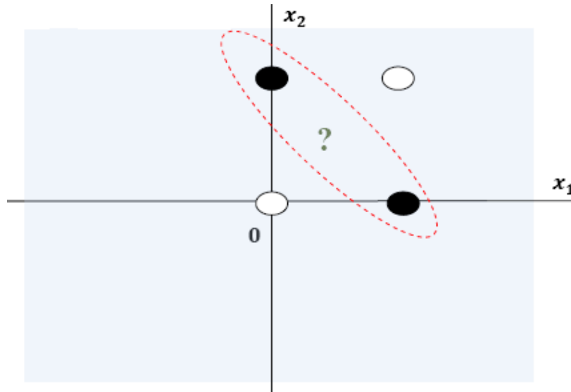
Figure 3.25. Problème du XOR
