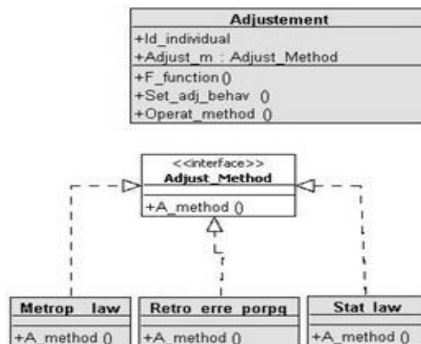
Figure 5.18. Vue du méta modèle de l'ajustement
