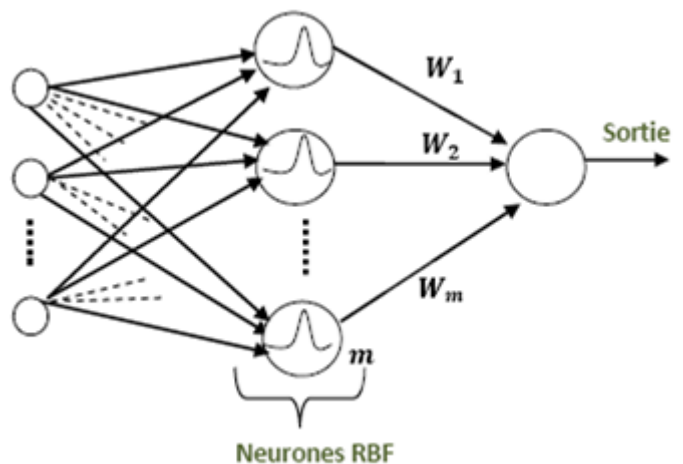
Figure 3.26. Réseau RBF
