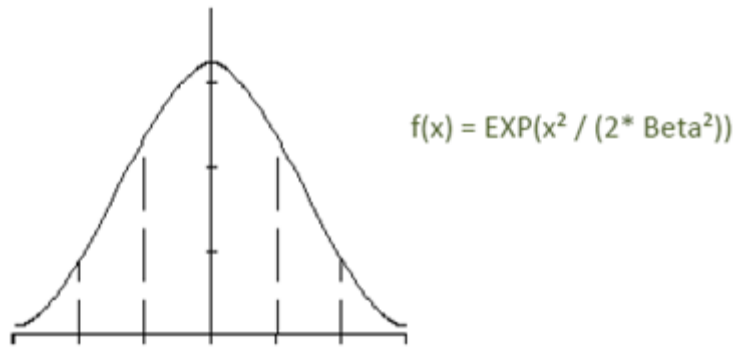
Figure 3.27. Fonction gaussienne
