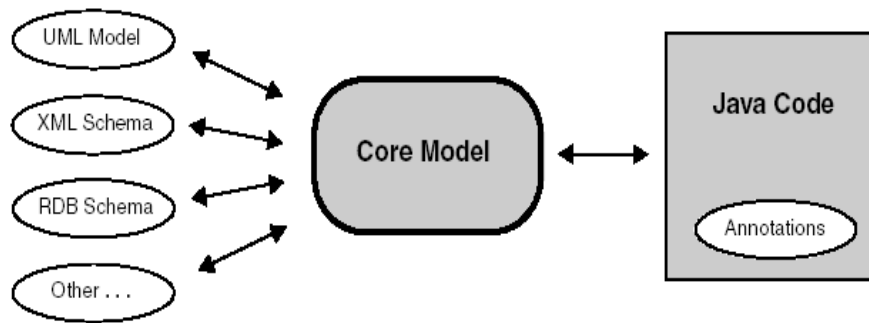
Figure 4.12. Organisation générale d'EMF [Bud 04]
