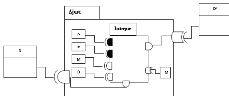
Figure 5.13. Représentation semi formelle des composants Ajust et Interpret
