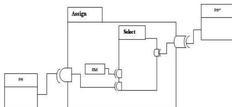
Figure 5.8. Représentation semi formelle des composants assign et select
