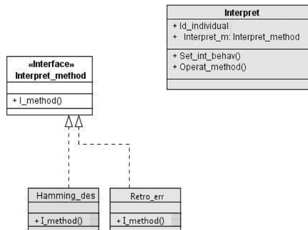
Figure 5.20. Vue du meta modele de l'interpretation
