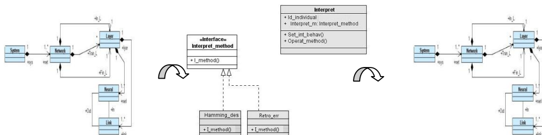
Figure 6.19. Représentation de la transformation d'interprétation d'un afficheur à sept segments
