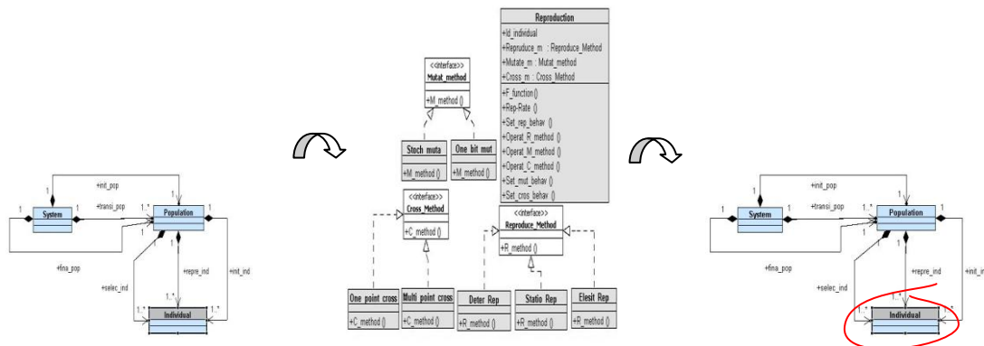
Figure 6.5. Représentation de la transformation de reproduction du modèle TSM
