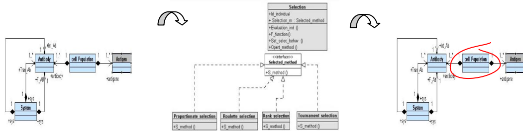
Figure 6.12. Représentation de la transformation de sélection de CLONCLAS
