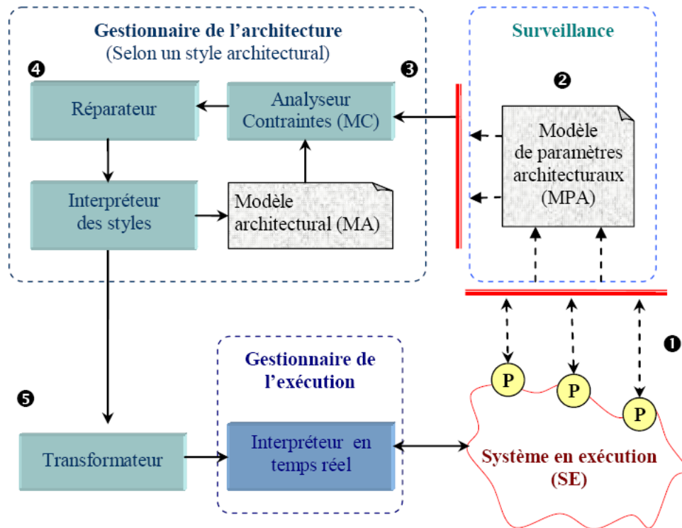
Figure 6.20. Principe de l'approche Rainbow [Mes 06]
