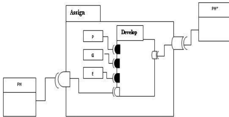
Figure 5.6. Représentation semi formelle des composants assign et develop
