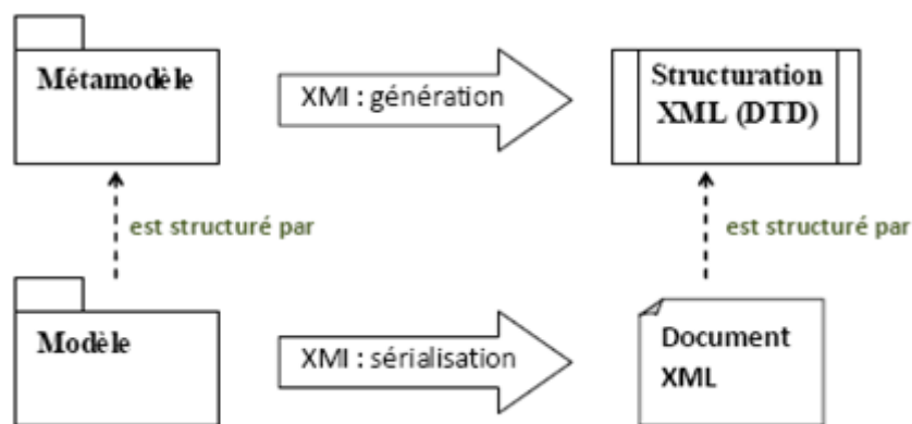
Figure 4.5. XMI et la structuration de balises XML [Bla 05]
