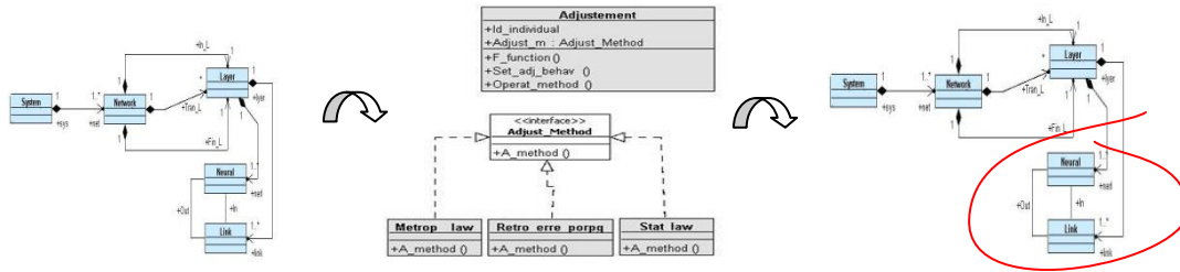
Figure 6.18. Représentation de la transformation d'ajustement d'un afficheur à sept segments
