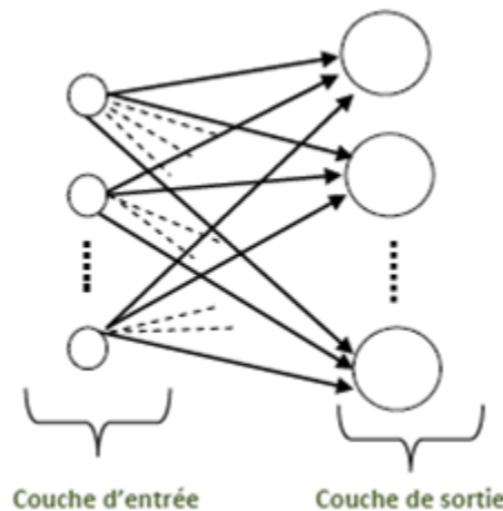
Figure 3.21. Réseau à une couche.
