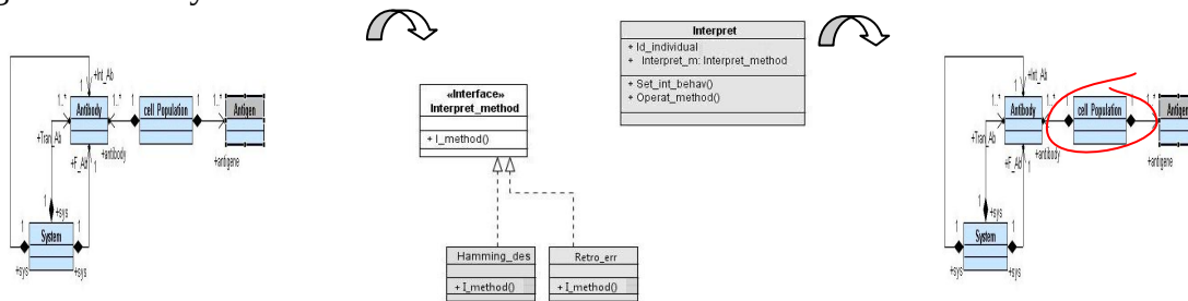
Figure 6.11. Représentation de la transformation d'interprétation de CLONCLAS
