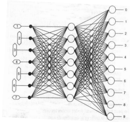
Figure 6.15. Réseau de reconnaissance de l'afficheur à sept segments
