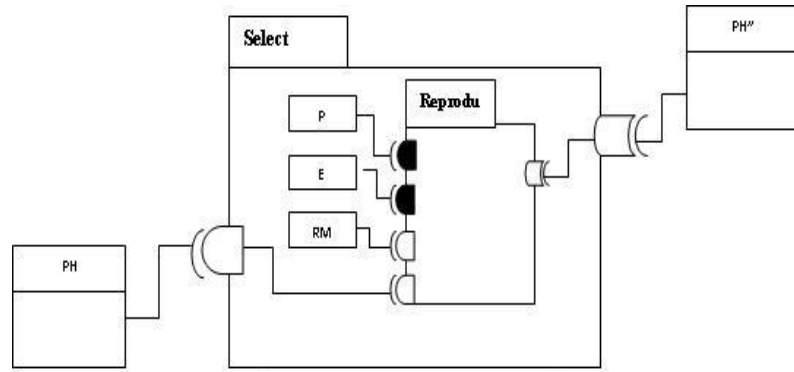
Figure 5.9. Représentation semi formelle des composants select et reproduce
