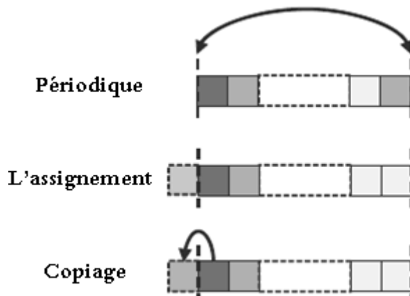
Figure 3.7. Les principales méthodes d'élimination de frontières sur un espace d'une dimension
