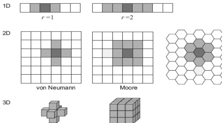
Figure 3.6. Quelques types de voisinage pour des représentations à une, deux et trois dimensions.
