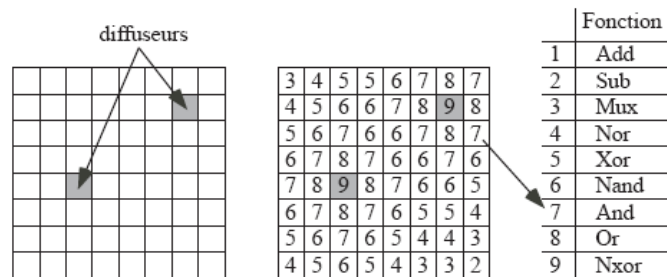
Figure 5.1. Gradient chimique propagé par le codage morphogénétique. La fonctionnalité de la cellule est ensuite définie par une table, qui constitue une partie du génome [Tho 05]
