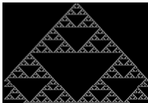
Figure 3.9. Exemple d'automate à une dimension (Triangle de Pascal) [Ren 00].
