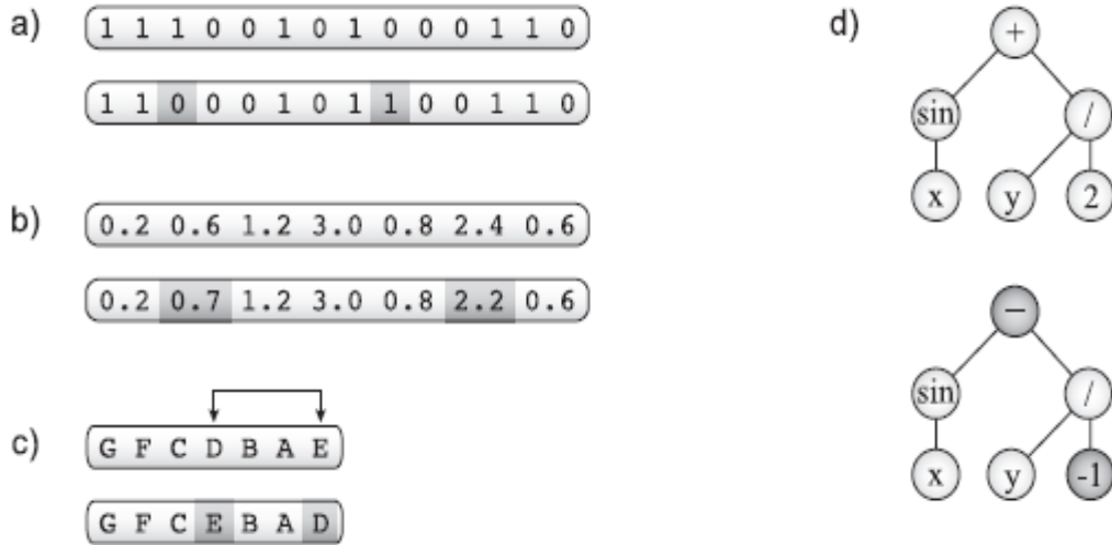
Figure 3.16. Représentation des opérations de mutation a) mutation des valeurs binaires, b) mutation des valeurs réelles, c) mutation pour les séquences, d) mutation pour la représentation en arbre.
