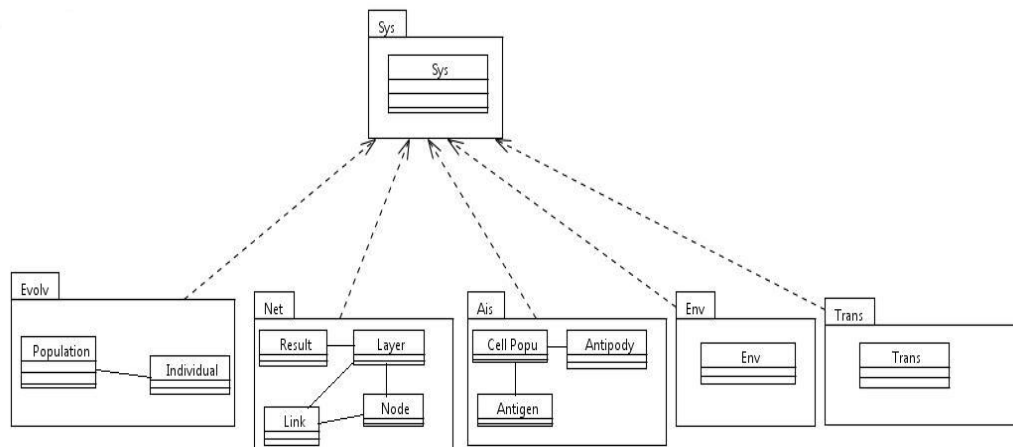
Figure6.23. Description du meta modele notre simulateur
