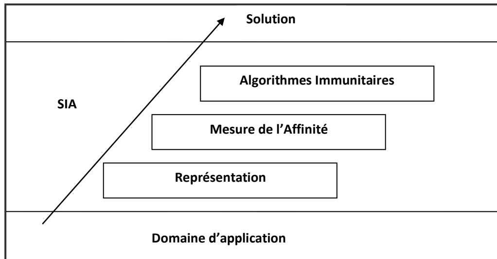
Figure 3.33. Un framework de SIA pour l'ingénierie et sa structure multi niveau [Dec 03]
