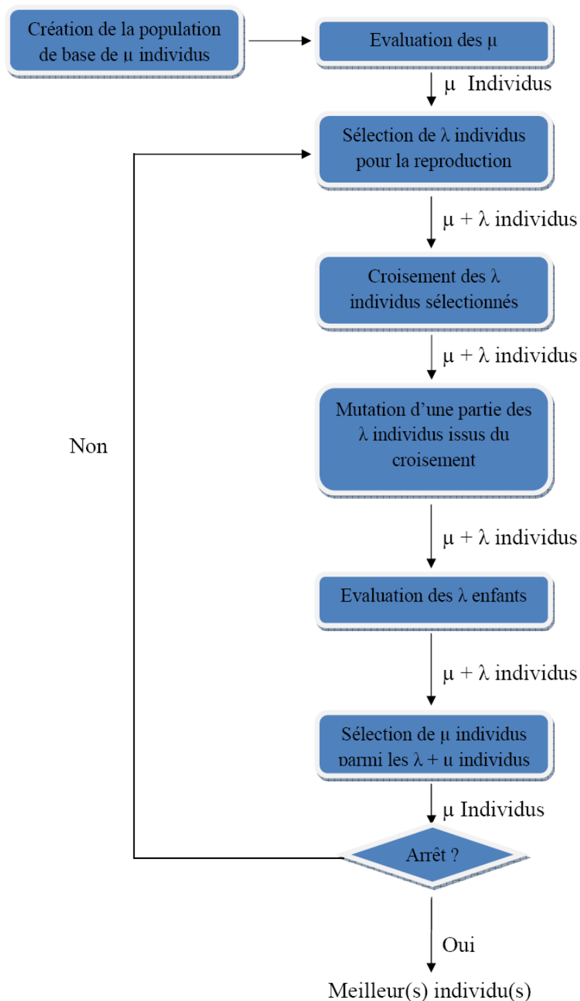
Figure 3.12. Schéma type d'un algorithme évolutionnaire [Lam 09].
