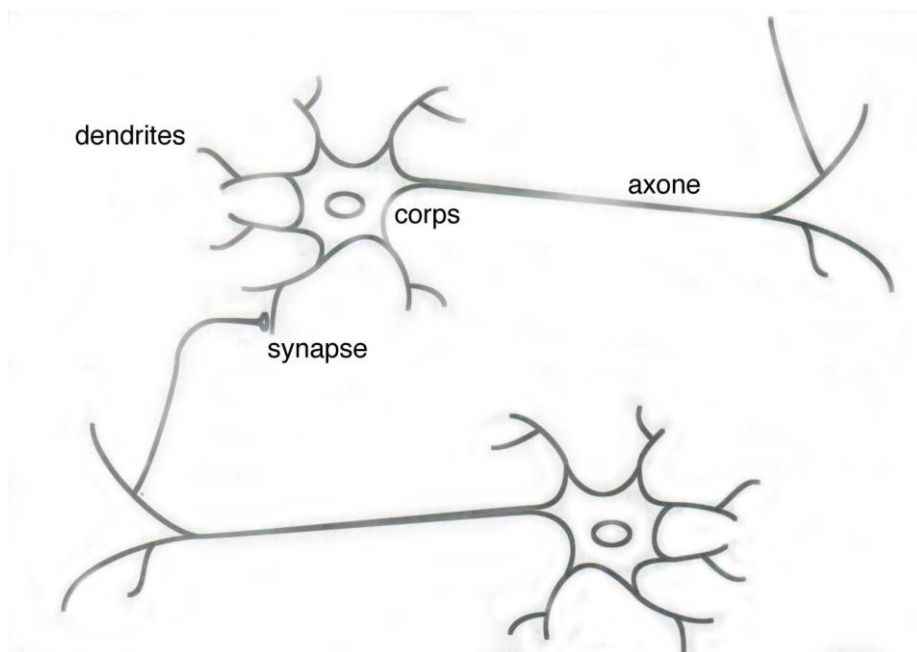
Figure 3.17. Neurone biologique.
