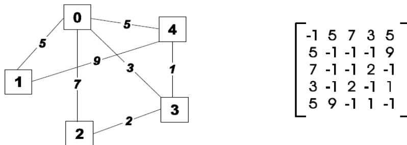
Figure 6.2. Représentation mathématique du voyageur de commerce
