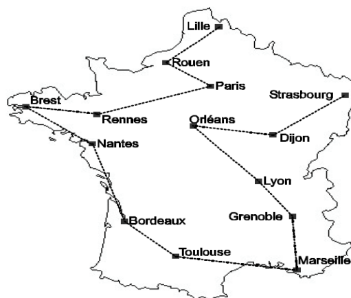
Figure 6.1. Représentation du problème du voyageur de commerce
