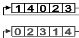
Figure 6.3. Représentation d'une tournée
