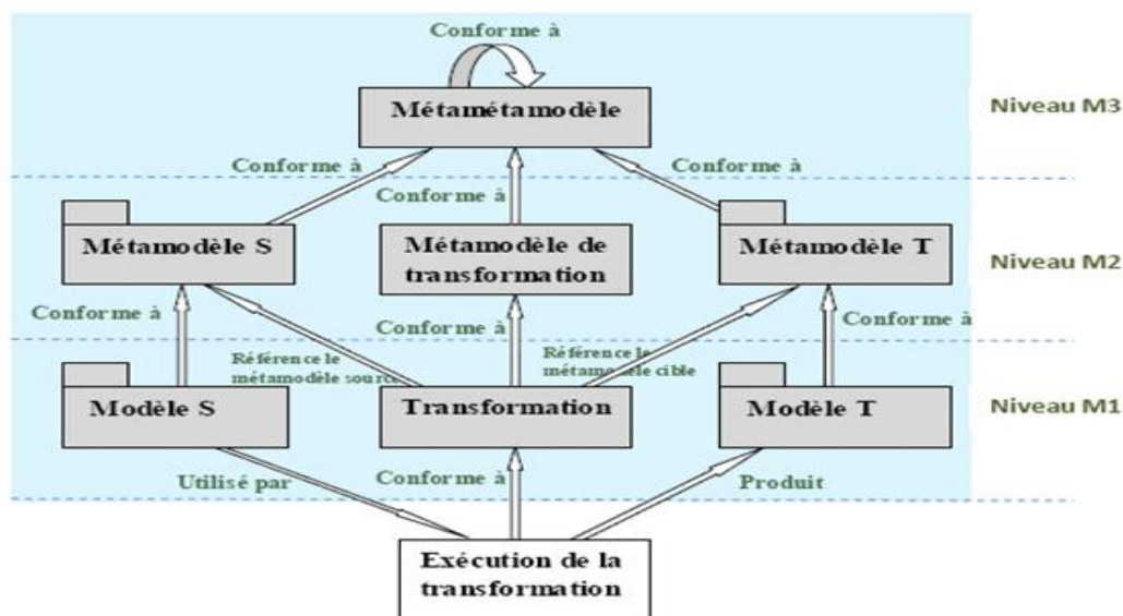
Figure 4.8. Les Niveaux méta de la transformation de modèles
