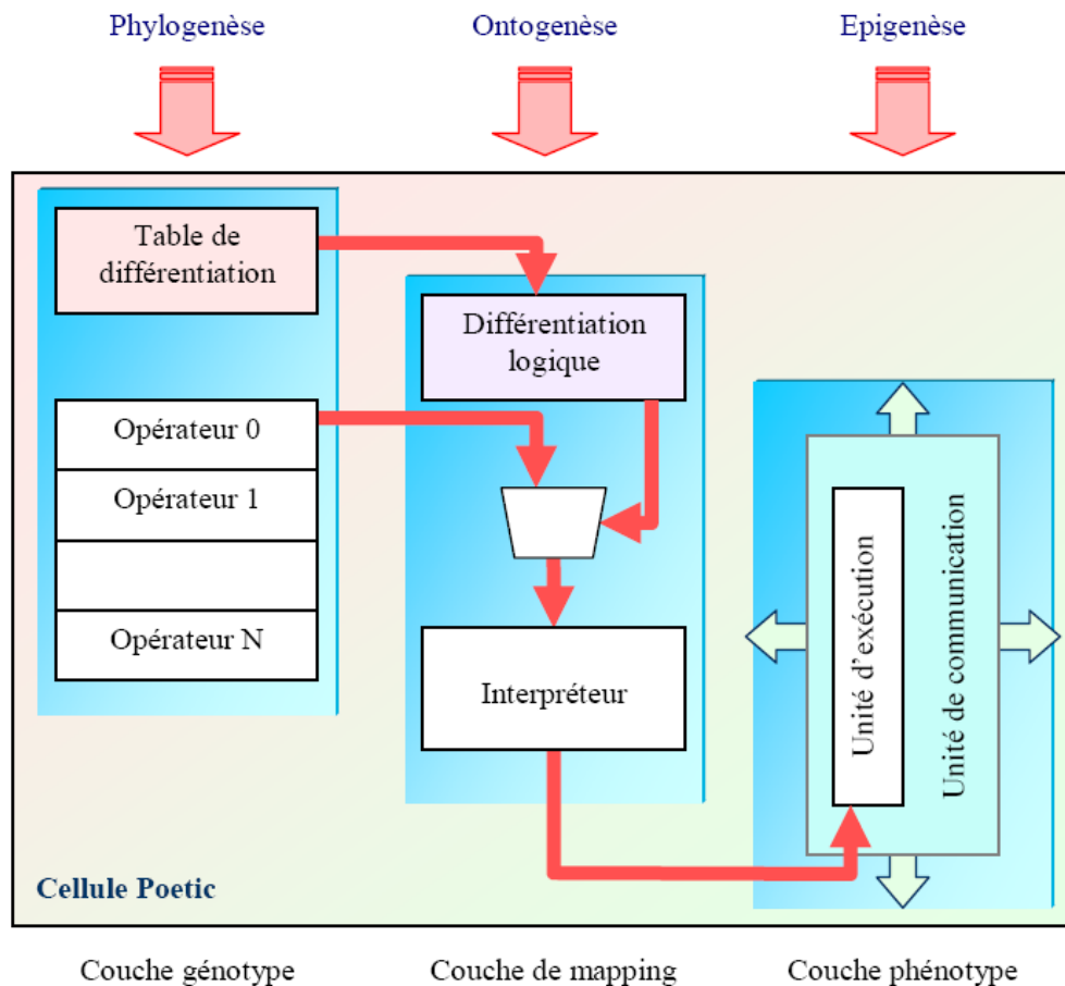
Figure 6.21. Les couches composant une cellule Poetic [Mes 06]
