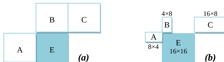
Figure 2.25 : Macroblocs en cours et de voisinage avec des tailles différentes.
