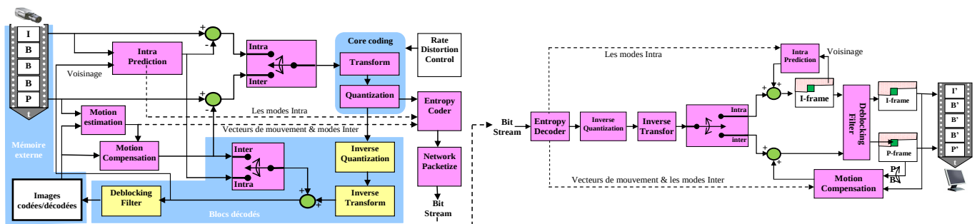
Figure 5.1. Traitement des macroblocs dans un Encodeur/Décodeur H.264/AVC.
