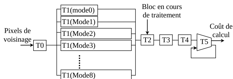
Figure 5.8. Réalisation en série (en pipeline) des tâches dans le module Intra4×4.
