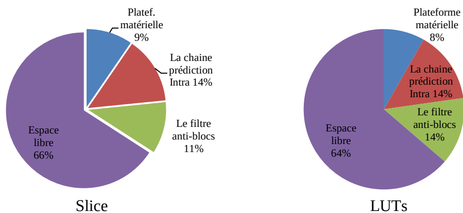
Figure 6.13. Taux d'utilisation des ressources matérielles de l'encodeur H.264/AVC.
