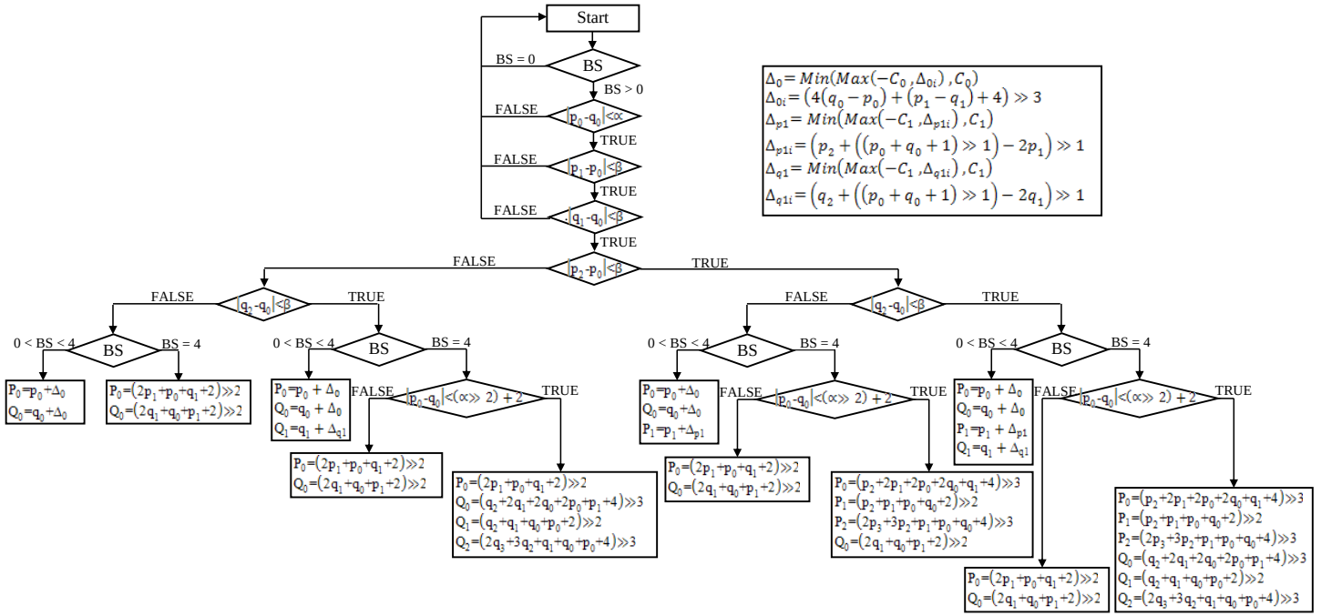
Figure 2.22 : L'organigramme du filtre anti-blocs utilisé dans H.264 [63].
