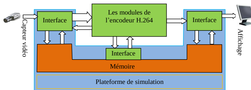
Figure 4.9. Plateforme de traitement vidéo pour l'encodeur H.264.
