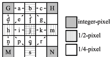
Figure 2.16 : Filtre sous-pixélique de luminance H.264.
