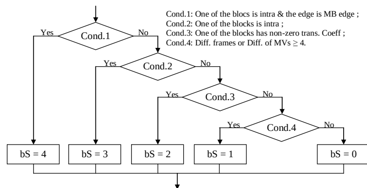
Figure 5.18. Organigramme de calcul des valeurs de BS.
