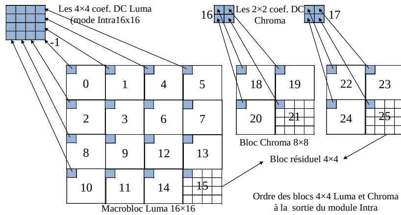
Figure 2.23 : Ordre de transmission des blocs à l'encodeur entropique dans le mode Intra.
