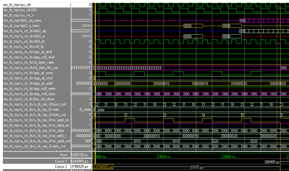
Figure 4.8. Temps de réponse global du contrôleur en mode d'écriture.
