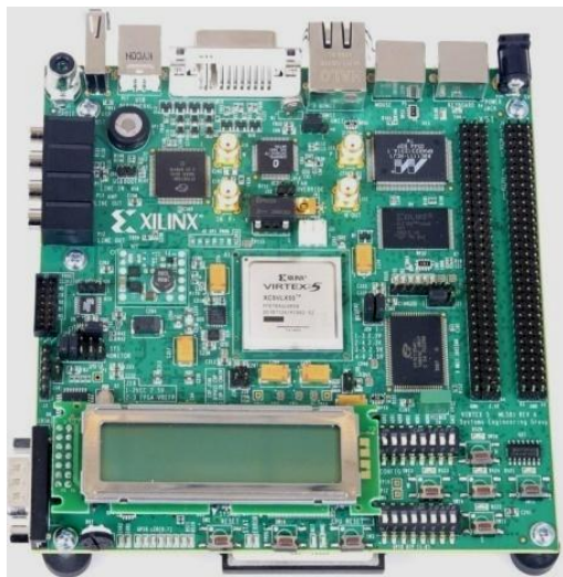
Figure 4.1. La carte Virtex5-ML501 de Xilinx [80].
