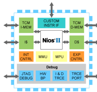
Figure 1.10. Les processeurs NIOS et NIOS-II de Altera
