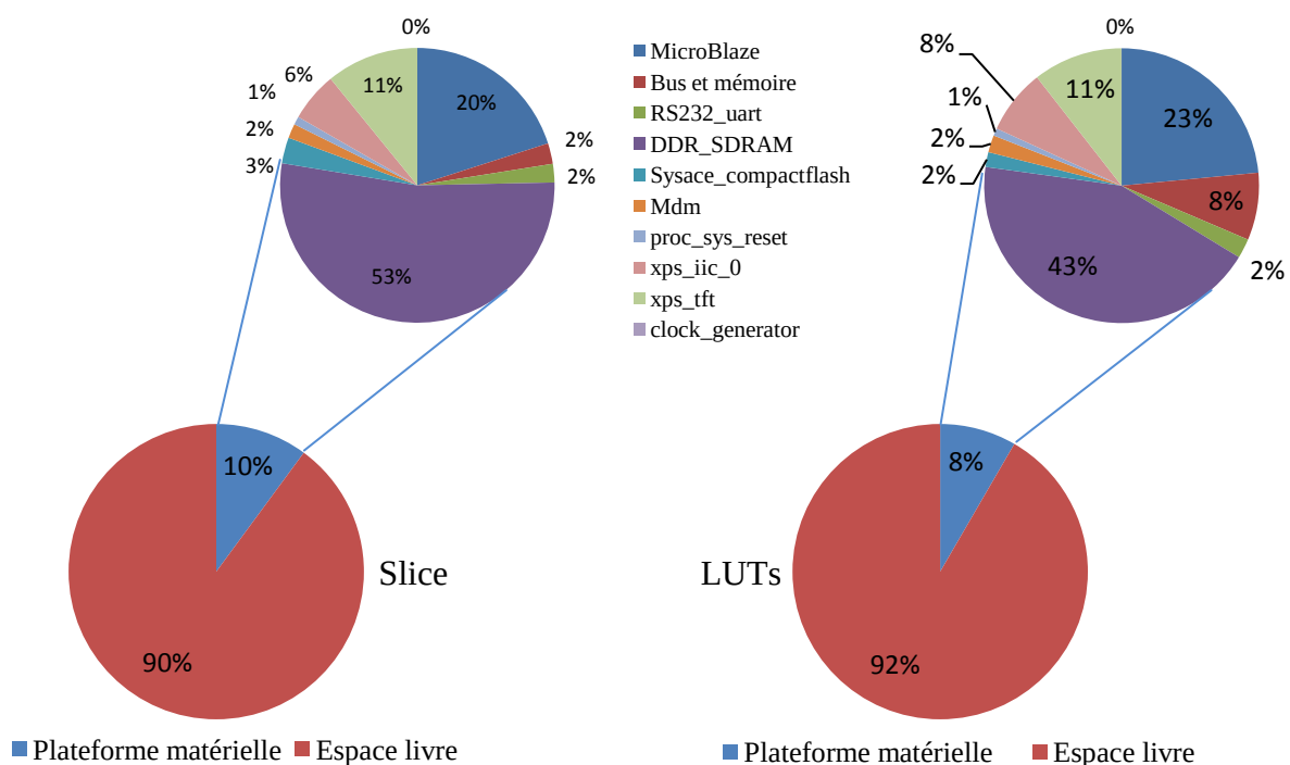
Figure 6.9. Taux d'utilisation des ressources matérielles de la plateforme de traitement.
