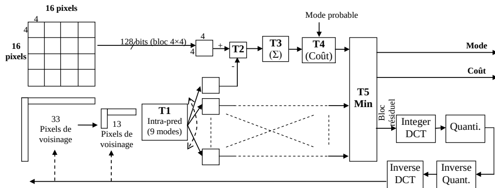
Figure 5.7. Architecture matérielle proposée pour le module Intra4×4.
