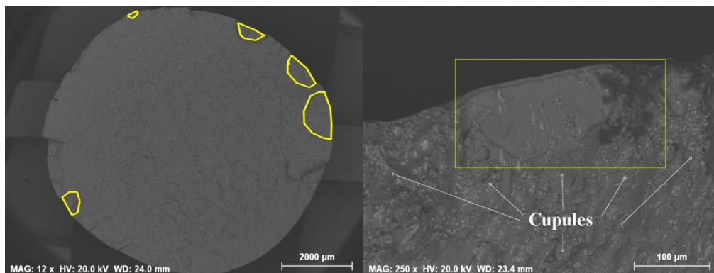
Figure III. 27 : Sites de propagation de fissures d'une éprouvette imprégnée, \sigma^{alt}=130 MPa et R_\sigma=0.1
