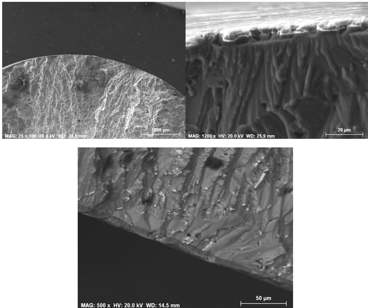
Figure III. 40 : Faciès de rupture d'une éprouvette imprégnée, \tau^{\text{alt}} = 150 \text{ MPa} , R_\tau = -1 et R_a = 0.8 \text{ µm}
