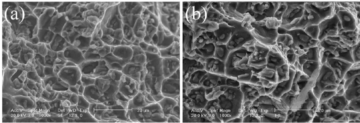
Figure I. 21 : Faciès de rupture de deux éprouvettes testées, respectivement à déformation imposée; (a) 0.5% et (b) 0.8%, T=200°C [37]
