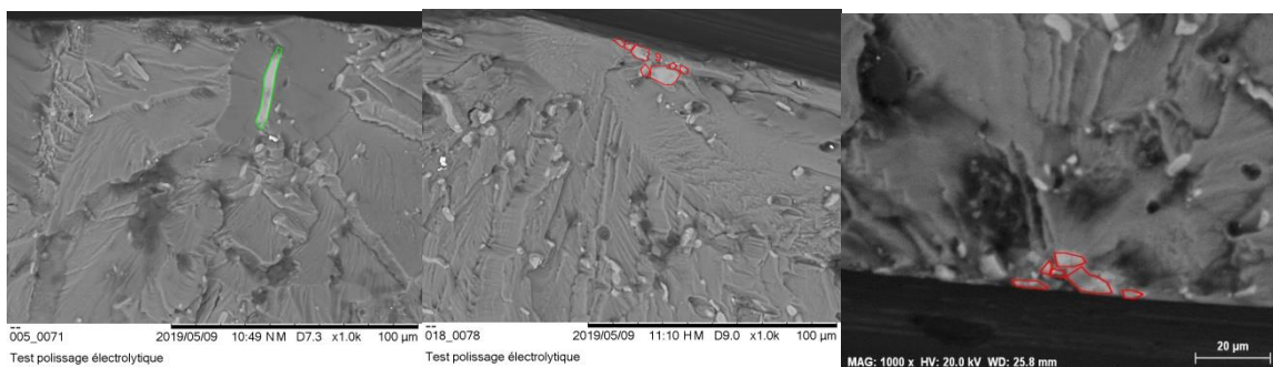
Figure III. 13 : Faciès de rupture d'éprouvettes testée en traction cyclique, R_o=0.1 , \sigma^{\text{alt}}=100 \text{ MPa} , pour des rugosités de a) 0.8 \mu\text{m} , b) 3.2 \mu\text{m} , c) 6.3 \mu\text{m}
