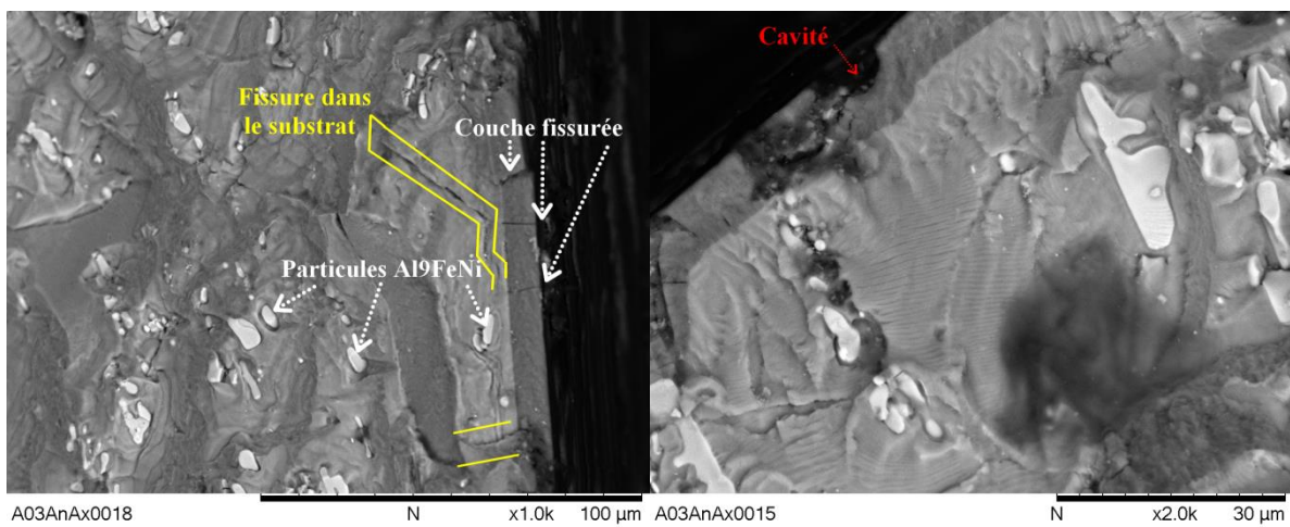
Figure III. 24 : Sites d'amorçage de fissures d'une éprouvette anodisée, \sigma^{\text{alt}}=100 MPa et R_\sigma=0.1
