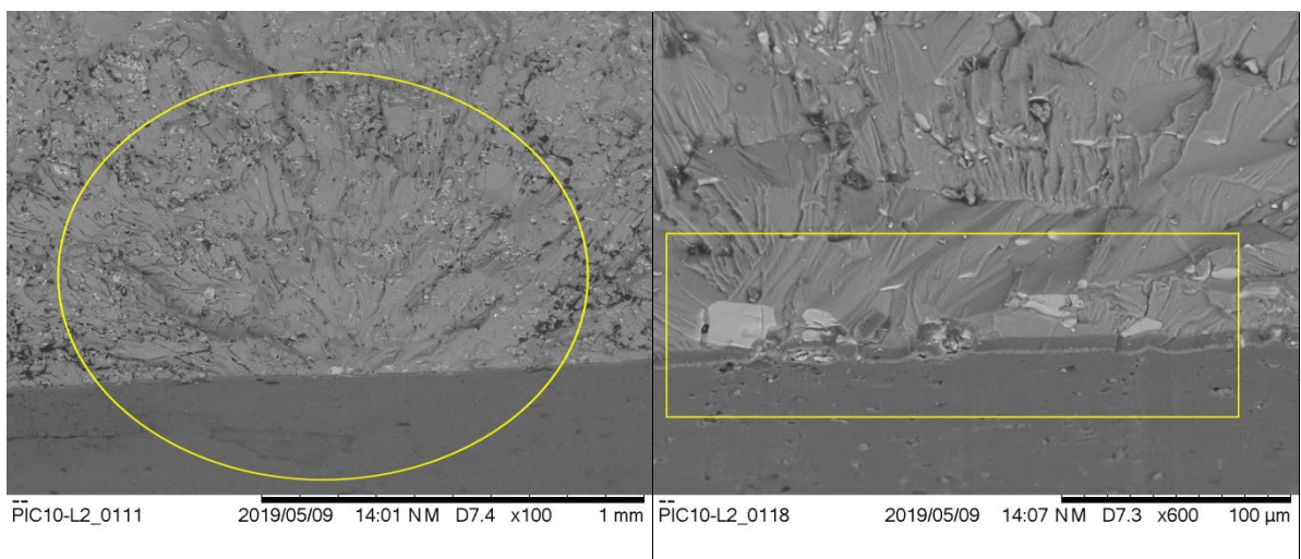
Figure III. 48 : Zones d'amorçage d'une éprouvette colmatée, \sigma_{\theta\theta}^{\text{alt}} = 117.7 \text{ MPa} , R_{\sigma p} = 0.1 et R_a = 0.8 \mu\text{m}
