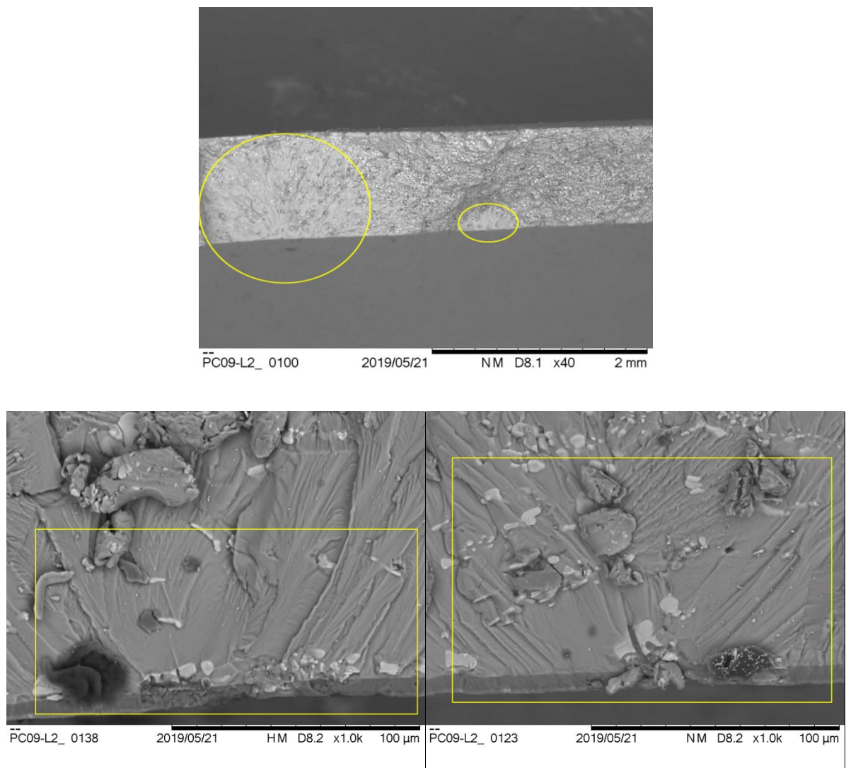
Figure III. 50 : Zones d'amorçage d'une éprouvette colmatée, \sigma_{00}^{alt} = 85 \text{ MPa} , R_{\sigma p} = 0.1 et R_a = 0.8 \text{ μm}
