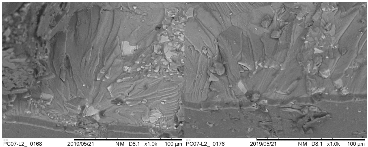
Figure III. 47 : Zones d'amorçage d'une éprouvette colmatée, \sigma_{\theta\theta}^{\text{alt}} = 144 \text{ MPa} , R_{\sigma p} = 0.1 et R_a = 0.8 \mu\text{m}
