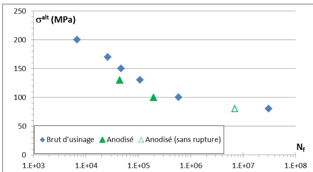
Figure III. 22 : Courbe de fatigue en traction cyclique sur éprouvettes anodisées et brutes d'usinage ( R_\sigma=0.1 et R_a=0.8 \mu m )
