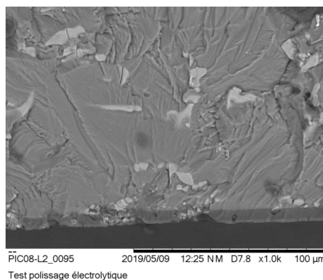
Figure III. 49 : Zones d'amorçage d'une éprouvette colmatée, \sigma_{\theta\theta}^{\text{alt}} = 98 \text{ MPa} , R_{\sigma p} = 0.1 et R_a = 0.8 \mu\text{m}
