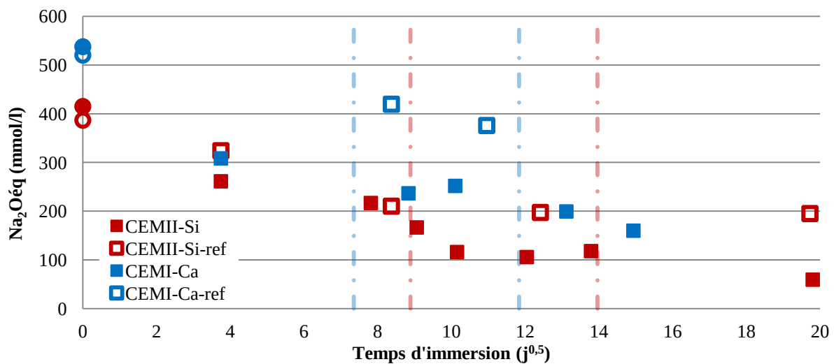
Figure III-22: Evolution de la teneur en alcalins équivalent dans la solution interstitielle des bétons CEMII-RSI-Si et CEMI-RSI-Ca
