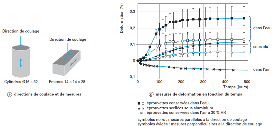
Figure I-33: Epreuves cylindrique et prismatique (a) et mesures de déformations (b)
