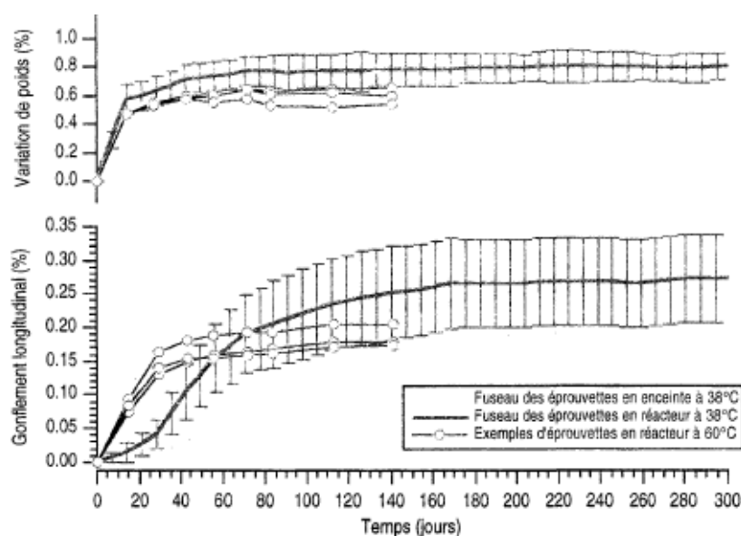
Figure I-43: Influence de la température sur la cinétique des déformations (Larive, 1997)
