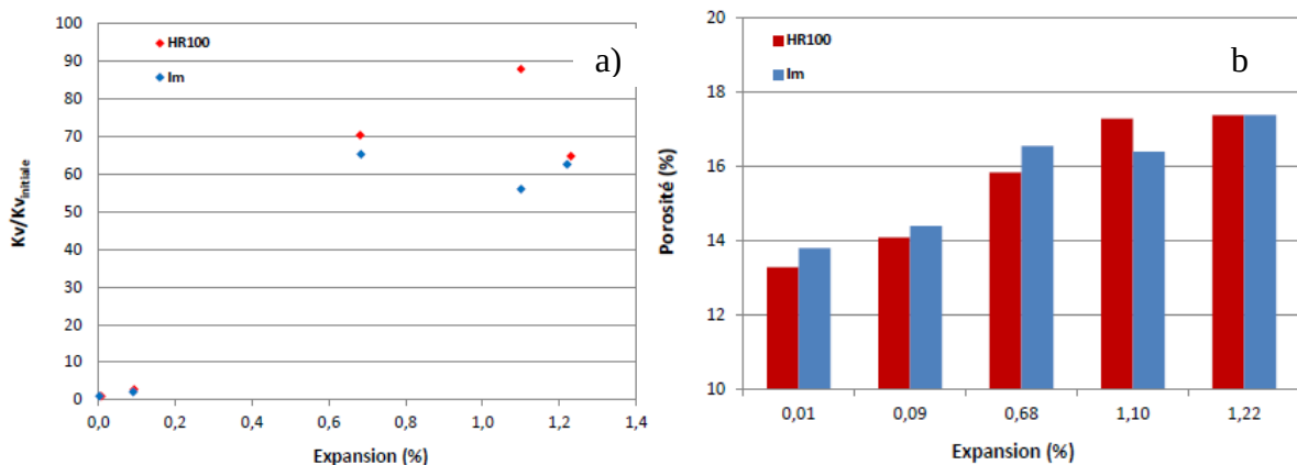
Figure I-51: Evolution du rapport d'accroissement de la perméabilité intrinsèque (a) et de la porosité (b) en fonction de l'expansion provoquée par la RSI (Al Shamaa, 2012)
