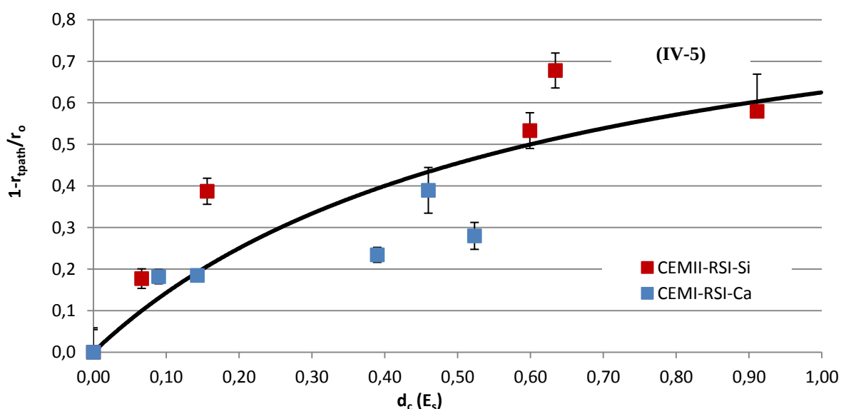
Figure IV-4 : Corrélation entre le rapport de résistivité électrique et l'endommagement par RSI mesuré par le module statique (bétons CEMII-RSI-Si et CEMI-RSI-Ca )
