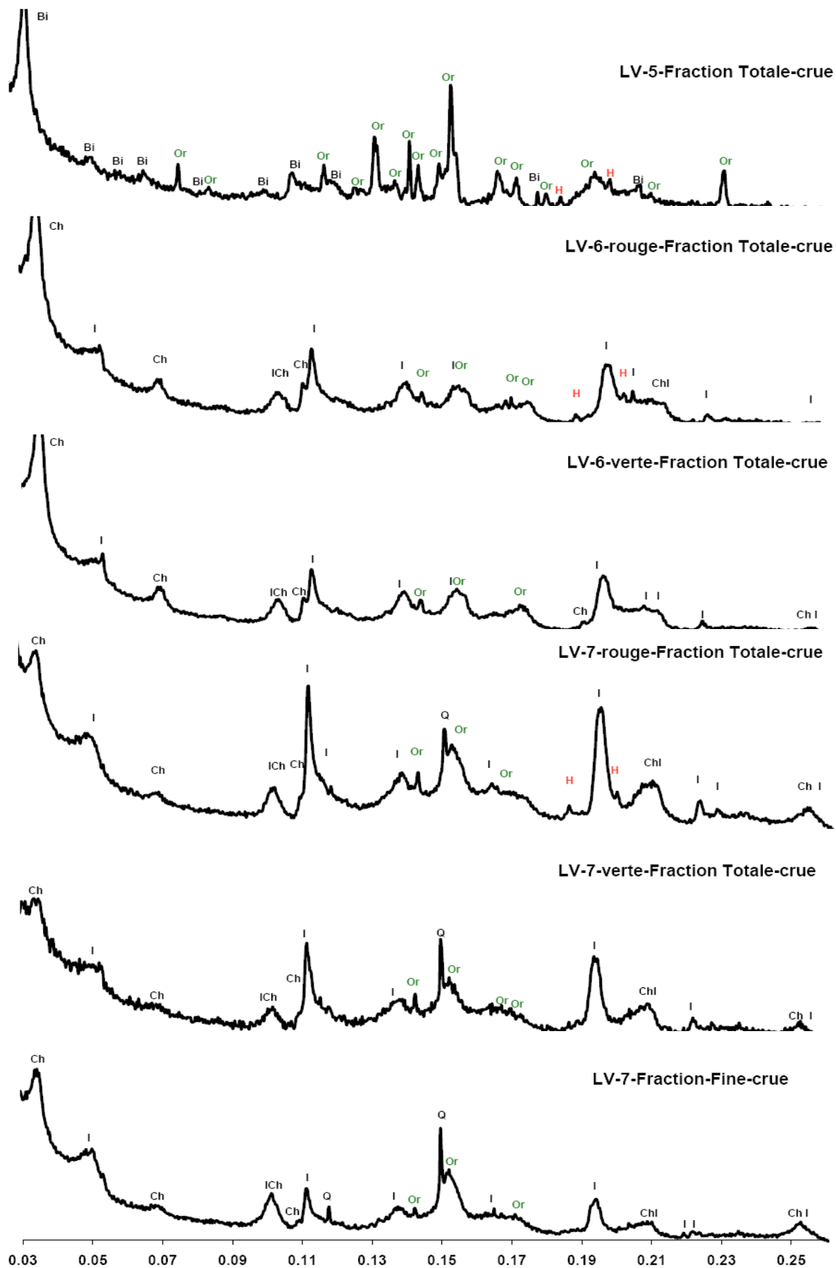
Figure II.C.3a : Diagrammes de diffraction des rayons X, I = f(\sin\theta/\lambda) (Longueur d'onde : \lambda_{CuK\alpha} ), réalisés au CEMES pour les fractions totales et fines des prélèvements LV-5 , LV-6 et LV-7 (Q : quartz, I : Illite, Cl : Chlorite, Or : Orthose, Bi : Biotite, H : Hématite).
