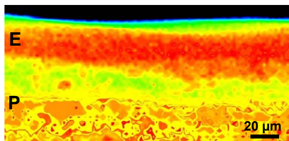
Carte Fluorescence X : Fe
