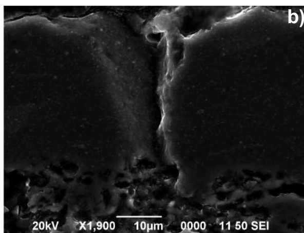
Figure III.C.6 : Engobe de l'échantillon d'Espalion (ESP05-09) observé par MEB en mode BES (électrons rétrodiffusés), après un très léger polissage de surface (a). Coupe transversale polie d'un fragment de sigillée attribuée à l'atelier d'Espalion (ESP-05-49), observée par MEB en mode électrons secondaires (b).
