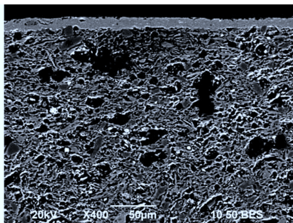
Engobe Noir-recuit-1060°C
