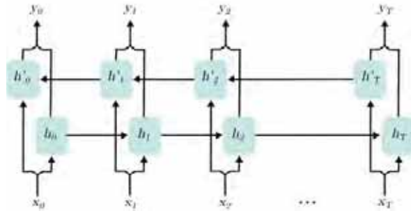
FIGURE 5.2 – Fonctionnement d'un RNN bi-directionnel, version déroulée
