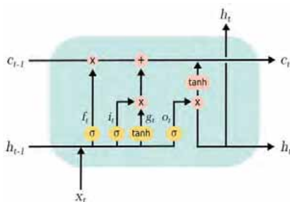
FIGURE 5.3 – Cellule de réseau LSTM
