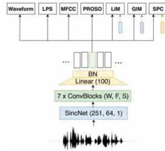
FIGURE 3.4 – Architecture du modèle PASE, tirée de [Pascual 2019]
