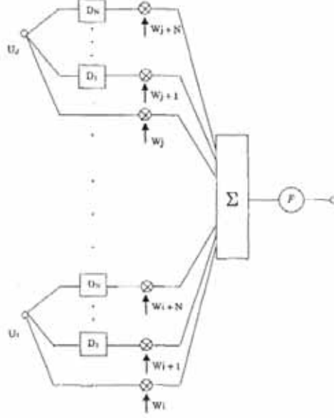
FIGURE 3.6 – Schéma d'une unité de réseau de neurones à délais temporels, tiré de [Waibel 1989]
