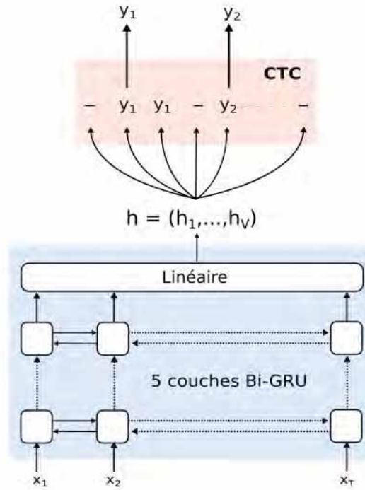
FIGURE 5.7 – Architecture du modèle RNN-CTC
