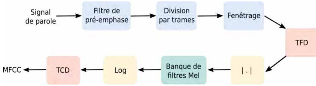
FIGURE 3.1 – Procédure d'extraction des MFCC
