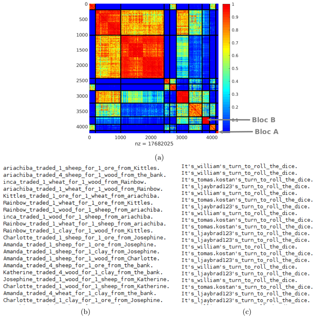
FIGURE 3.20 : (a) : Matrice affinité en sortie de FC1 et sa structure par blocs retournée par l'algorithme SC pour 10 classes. (b) : Quelques exemples des EDUs du bloc A de la Figure (a). (c) : Quelques exemples des EDUs du bloc B de la Figure (a).
