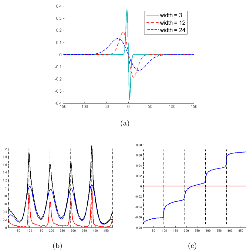
FIGURE 2.4 : (a) Le filtre pour différentes tailles de fenêtre glissante. (b) et (c) Détection des paliers.
