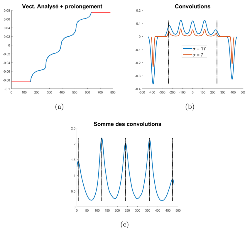
FIGURE 2.8 : (a) : Troisième vecteur singulier gauche de la matrice rbsb480 issue de [3] doublement stochastique avec prolongation (en rouge). (b) : Produits de convolution avec le filtre pour deux \sigma différents. (c) : Somme des deux produits de convolution. En pointillés noirs, les maxima détectés par le filtre.
