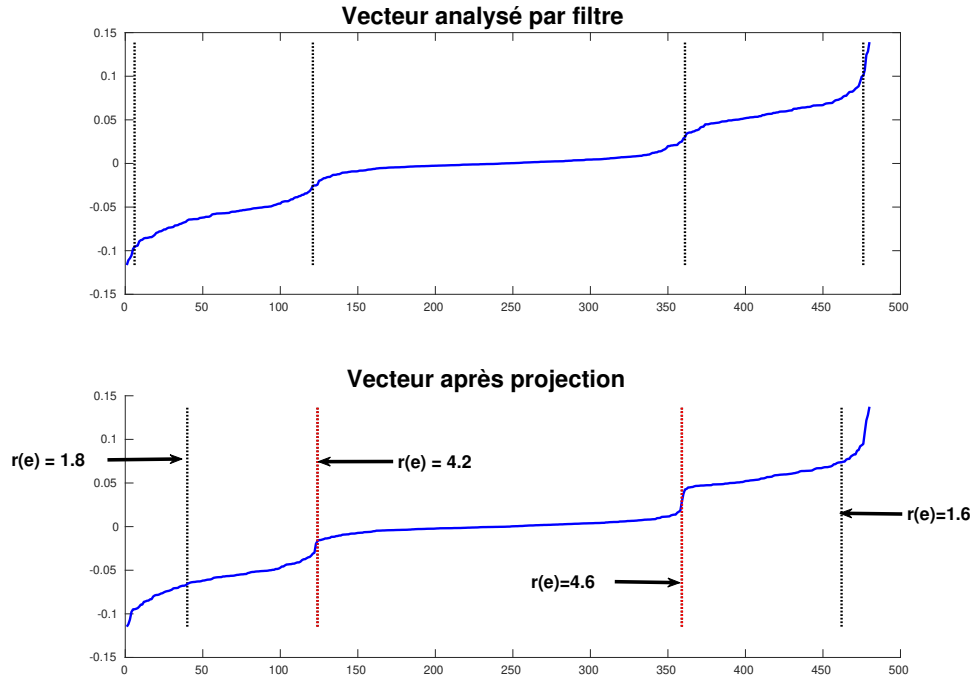
FIGURE 2.23 : Processus de détection des arêtes par projections : en haut : un vecteur singulier gauche de la matrice \mathbf{rbsb480} , les traits pointillés noirs représentent les arêtes retournées par le filtre de Canny appliqué à ce vecteur. En bas : le vecteur résultant du processus de projections itératif. Les arêtes conservées après analyse de leur SNR sont affichées en rouge. Le SNR de chaque arête est précisé.
