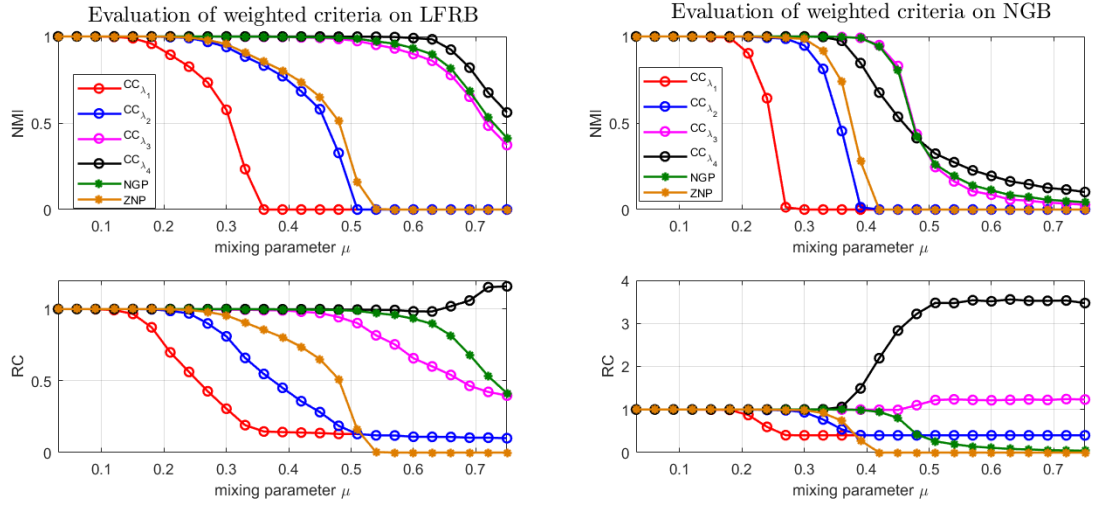
FIGURE 1.16 : NMI et RC pour les critères pondérés, sur LFRBenchmark (à gauche) et NGBenchmark (à droite).
