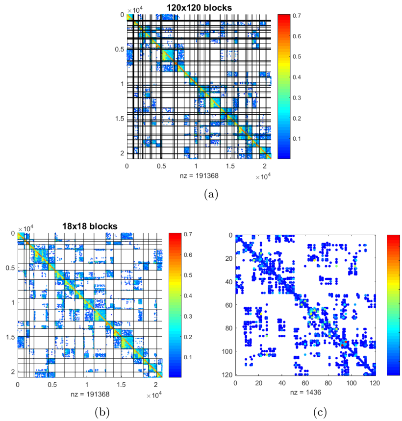
FIGURE 3.11 : Matrice Ill_Stokes . (a) : Le partitionnement de la matrice après avoir ramené les éléments dominants sur sa diagonale. La matrice possède alors 120 blocs diagonaux. (b) : Le partitionnement de la matrice obtenu après application du processus de fusion symétrique sur le partitionnement présenté en (a). (c) : Matrice condensée 120 \times 120 construite à partir de la matrice et de son partitionnement présenté en (a).
