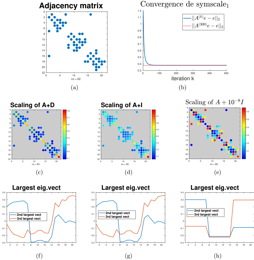
FIGURE 2.3 : L'ajout d'éléments non nuls sur la diagonale de la matrice traitée est parfois nécessaire pour assurer l'existence d'un équilibrage doublement stochastique. Ici, la matrice affichée en (a) est à diagonale vide, et les algorithmes d'équilibrage ne permettent pas de mettre cette matrice sous forme doublement stochastique, comme le montre la courbe d'erreur en fonction des itérations de l'algorithme symscale1 , en (b). Nous proposons trois façons d'assurer la bi-irréductibilité de cette matrice en remplissant sa diagonale : avec le degré du noeud concerné – cf (c) –, avec 1 – cf (d) –, avec 10^{-8} – cf (e). En dessous de ces matrices sont affichés leur deuxième et troisième vecteurs propres dominants. On observe que l'aspect constant par morceaux est évident pour la matrice (e), ce qui n'est pas le cas des matrices (c) et (d).
