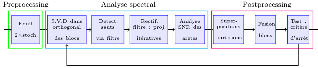
FIGURE 2.32 : Fonctionnement global de notre algorithme spectral.
