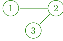
FIGURE 1.10 : A gauche : un graphe simple. A droite : le graphe aléatoire ayant le même nombre d'arêtes que le graphe de gauche, et une distribution uniforme des degrés. La distribution des degrés est donné au dessus des deux graphes.
