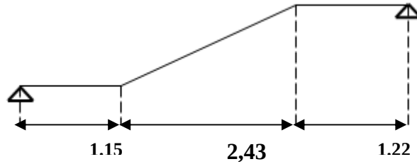
Figure IV-2 : Schéma statique de l'escalier
