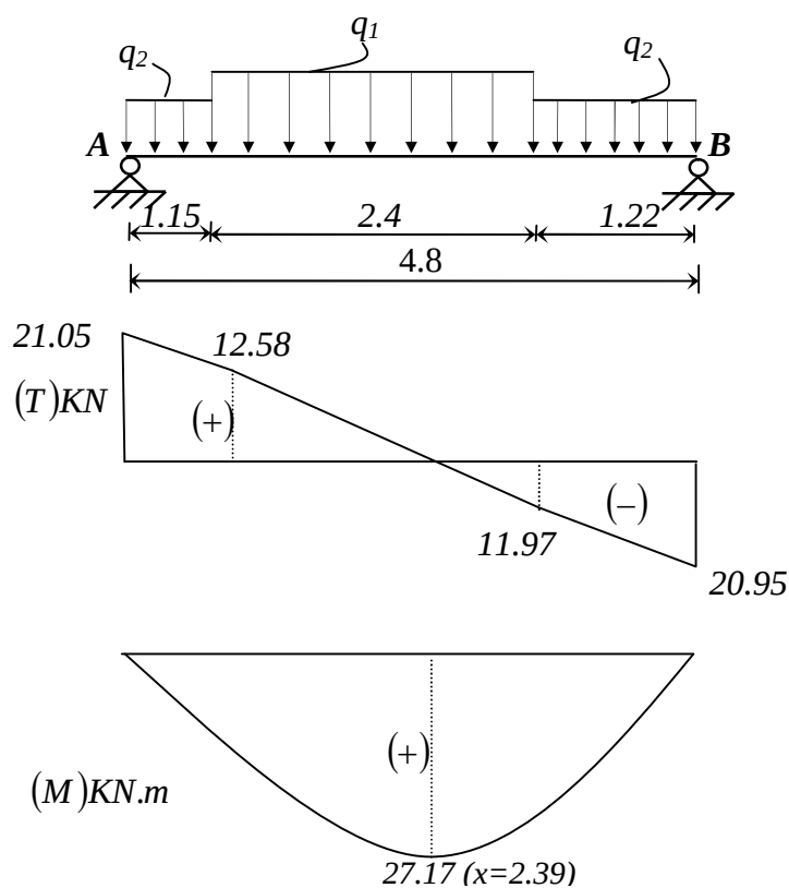
Fig IV-5 Diagrammes des sollicitations
