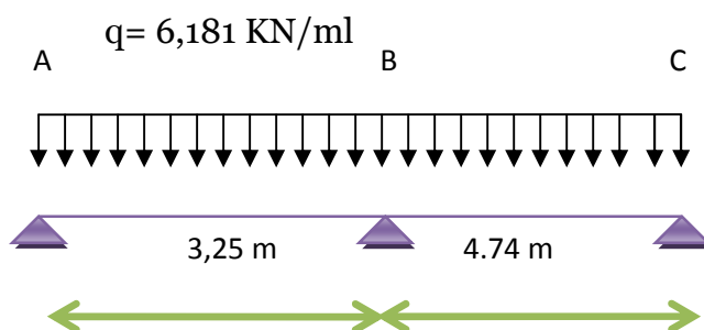
Figure III.7 schéma statique des poutrelles.
