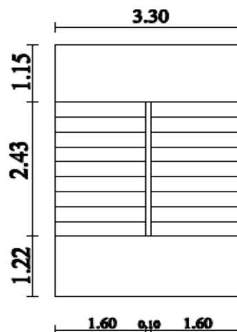
Vue en plan des escaliers
