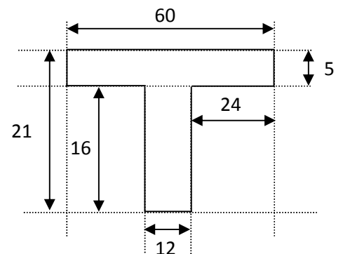
Figure III.1 Schéma de poutrelle.
