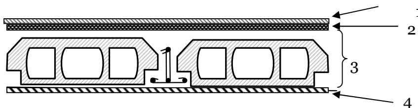
Figure II.3 détail des constituants du plancher d'étage courant
