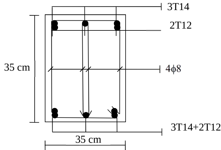
Figure VI.6 Schéma de ferrailage de la poutre secondaire
