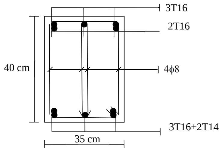
Figure VI.5 Schéma de ferrailage de la poutre principale
