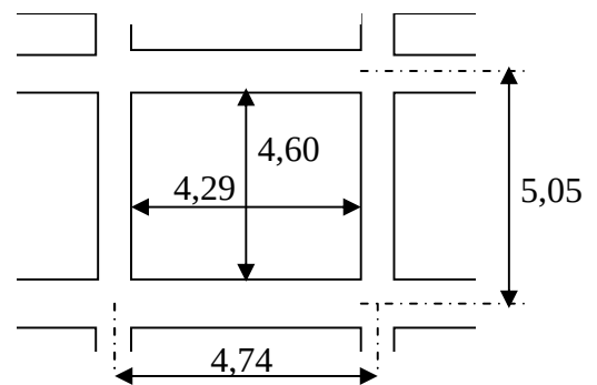
Figure VII.2 schéma du radier
