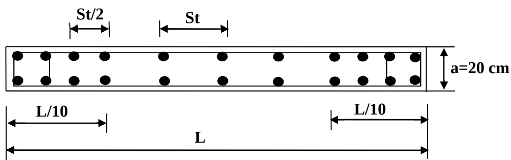
Figure VI.9 Disposition des armatures verticales dans les voiles
