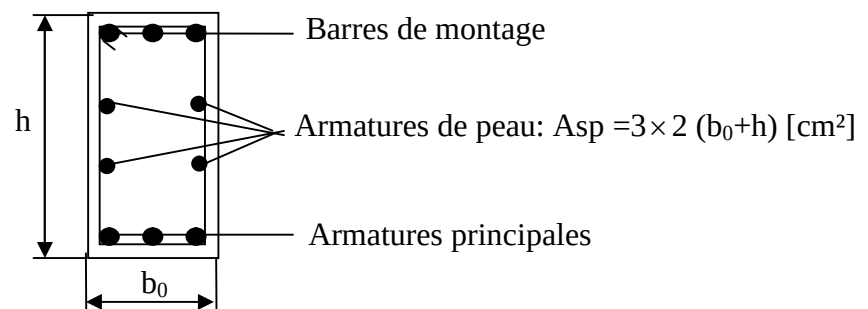
Figure VII.5 Répartition armatures dans les poutres
