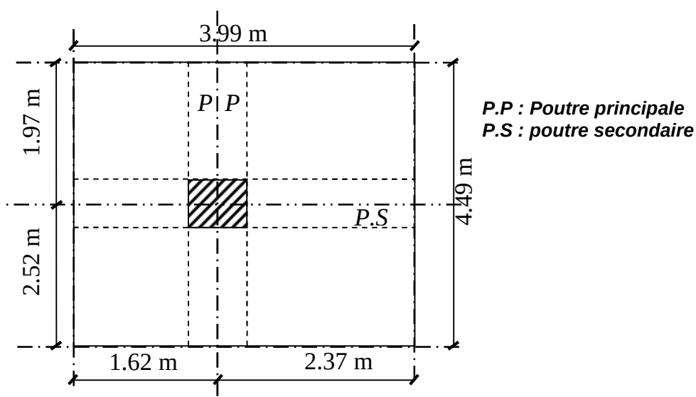
Figure II.6 Section afférente d'un poteau sollicité.
