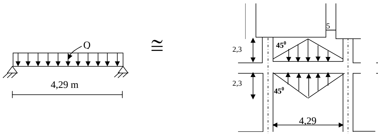
Figure VII.4 Répartition des charges sur les poutres
