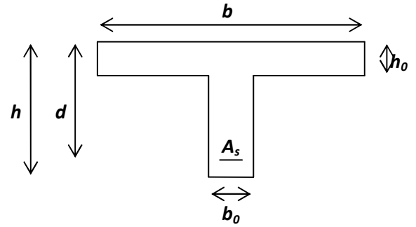
Figure III.12 Dimensions des poutrelles
