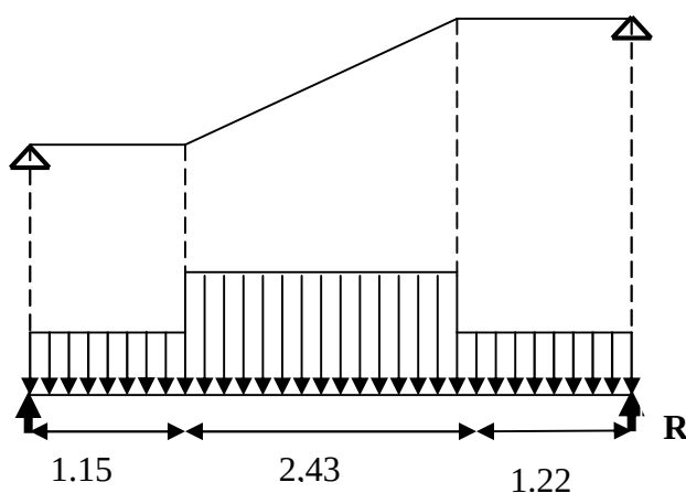
Figure IV.2 Schéma statique de l'escalier
