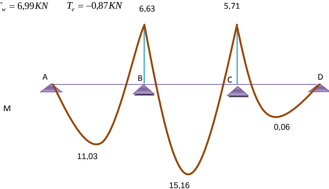
Figure III.3 Diagramme des moments fléchissants
