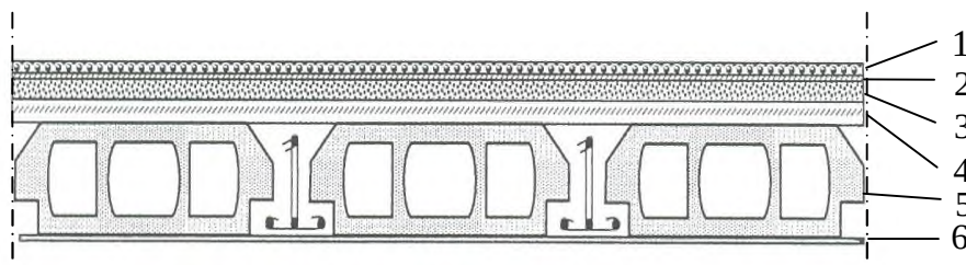
Figure II.2 détail des constituants du plancher terrasse inaccessible.
