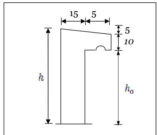
Fig. IV .10: Coupe de l'acrotère
