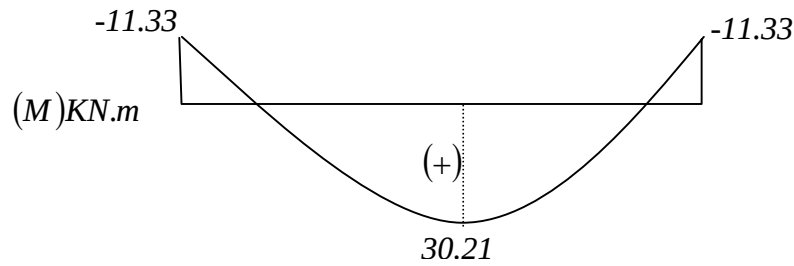
Fig IV. 4 Diagramme des moments retenus
