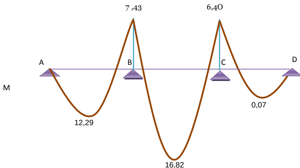
Figure III.5 Diagramme des moments fléchissant, M [KN.m]
