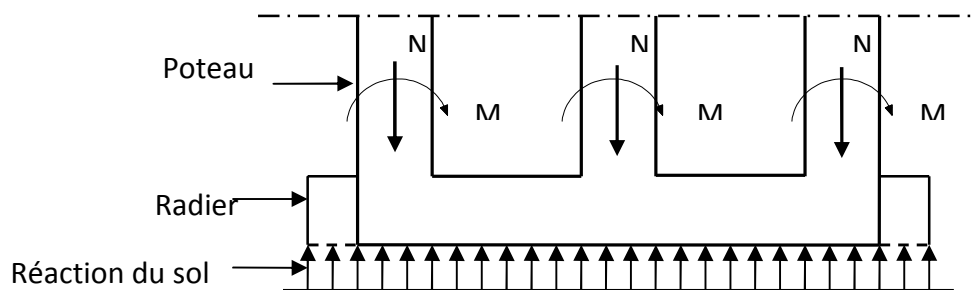
Figure VII.1 Schéma du Radier
