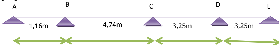
Figure.III.2 schéma statique des poutrelles.
