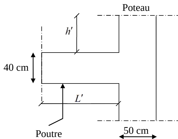
Figure VI.3 Schéma de la zone nodale.
