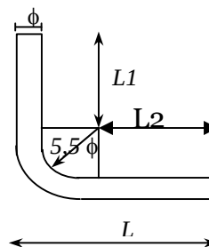
Figure III.13 Schéma de l'ancrage
