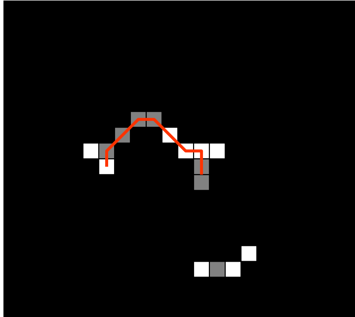
Figure 5 : chaînage des points de contour
