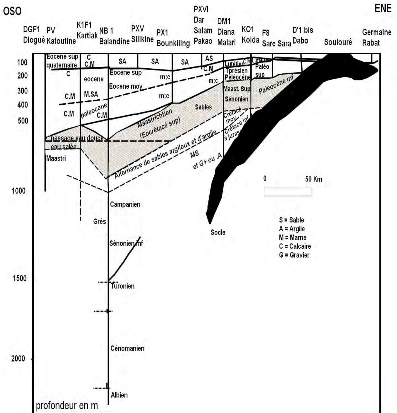
Figure 10 : Coupe géologique du bassin sédimentaire casamançais (Lepriol, 1983), modifié
