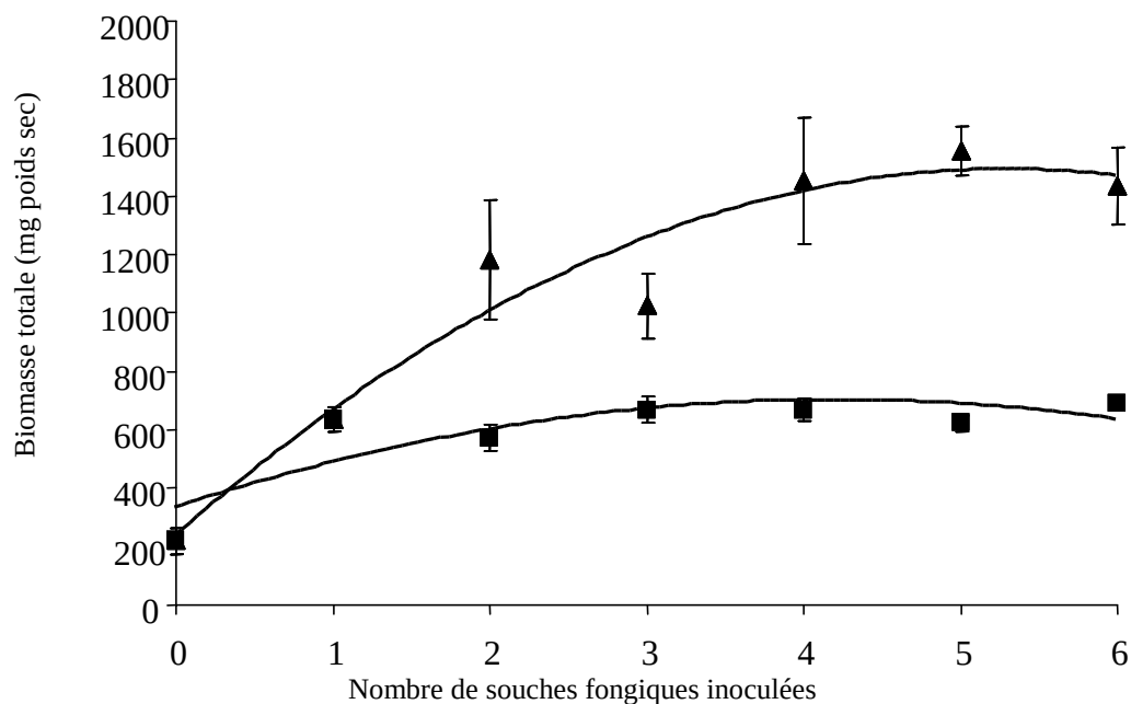
Figure 4 : Comparaison de l'effet théorique de l'inoculation fongique sur la biomasse totale des plants versus l'effet mesuré dans l'expérience en serre après 4 mois de culture. ■ : Biomasse totale théorique ; ▲ : Biomasse totale mesurée
