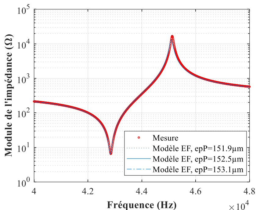
Figure 2.13 : Effet de l'incertitude de l'épaisseur sur l'impédance d'une couche PZT-LL 2 .
