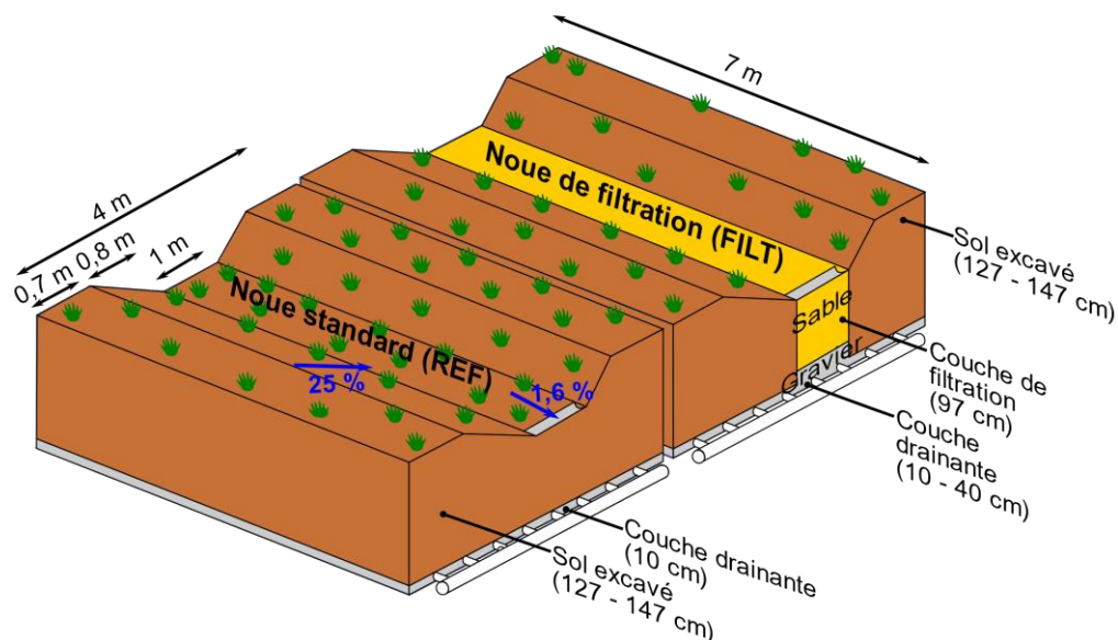
Figure 3.2. Schéma conceptuel des noues pilotes (les épaisseurs de sol indiquées correspondent aux épaisseurs initiales, avant tassement naturel)
