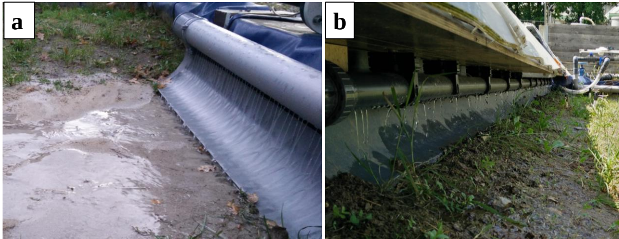
Figure 3.25. Détails des deux modalités d'injection d'eau, en fonctionnement. a. Injection d'eau en tête de noue de filtration. b. Injection d'eau latérale dans une noue
