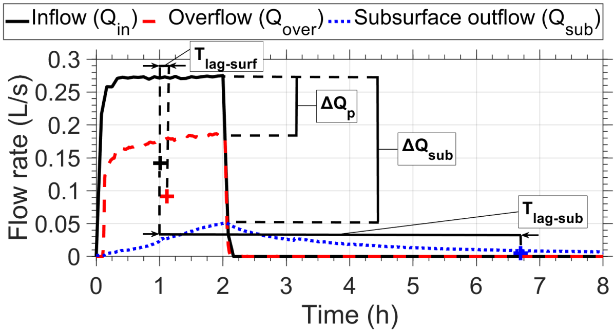
Figure 4.2. Hydrogrammes et indicateurs associés pour estimer les performances hydrologiques des noues
