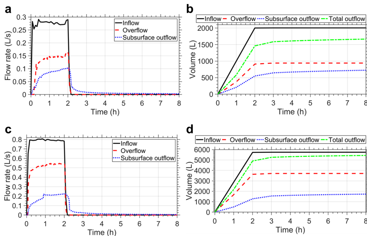
Figure 4.6. Réponses hydrauliques types de la noue standard observées suite à des alimentations latérales (hydrogrammes – volumes cumulés). a – b. Alimentation 0,27 L/s latérale (27/06/2018). c – d. Alimentation 0,8 L/s latérale (03/05/2018)
