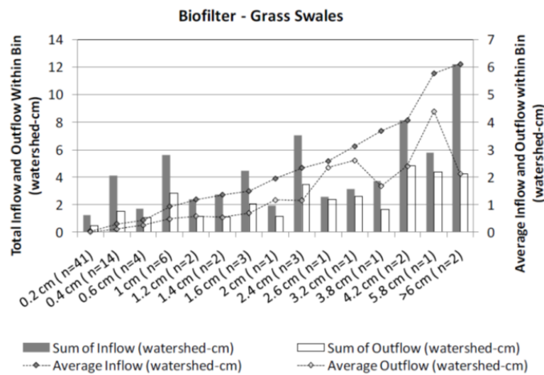
Figure 1.21. Performances hydrologiques des noues référencées dans l'ISBD (extrait de Poresky et al. (2011))
