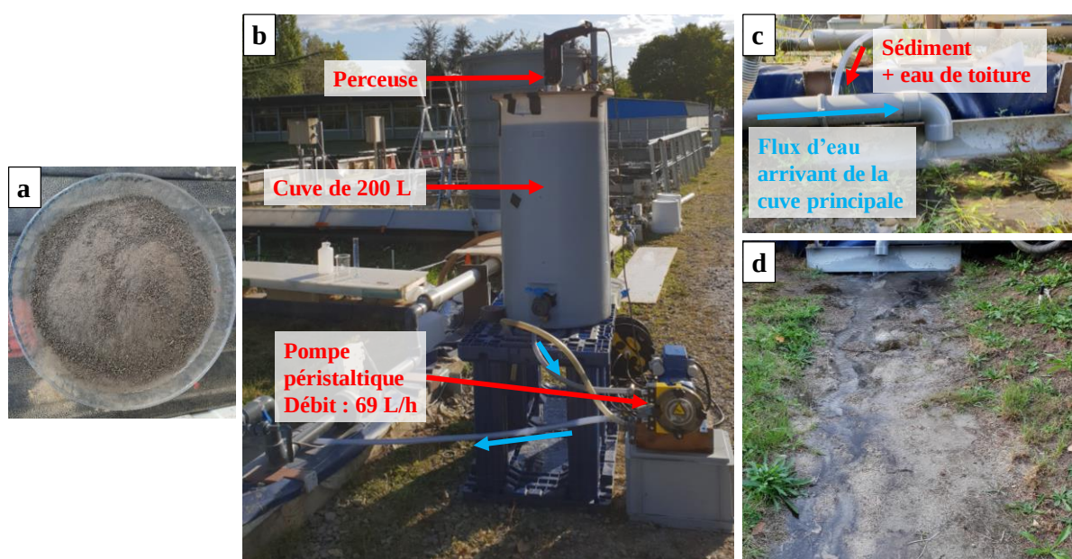
Figure 3.32. Détails d'un essai avec eaux dopées en MES. a. Sédiments injectés dans la cuve. b. Dispositif de dopage des eaux en MES. c. Zone de mélange des flux provenant des 2 cuves. d. Injection d'eau dopée en MES dans la noue de filtration
