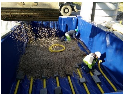
Figure 3.3. Etape de pose des 8 drains annelés (diamètre 80 mm) en fond d'ouvrage (au sein d'une couche de 10 cm de gravier) ; les drains sont posés directement sur la géomembrane
