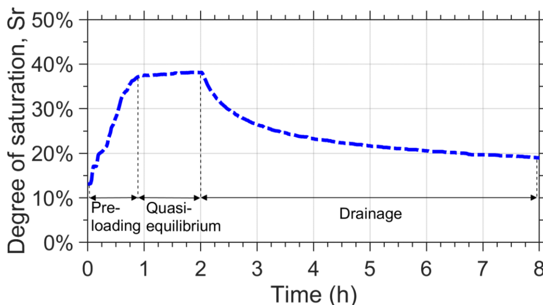
Figure 4.27. Evolution type de l'état de saturation de la noue de filtration en trois phases
