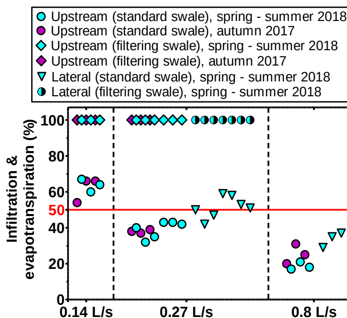
Figure 4.33. Evolution de la proportion d'eau infiltrée dans les noues pilotes suivant cinq conditions d'alimentation ; les résultats des deux périodes de tests (automne 2017 et printemps-été 2018) sont différenciés par des couleurs différentes (violet et cyan)
