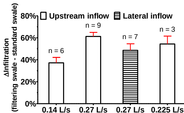
Figure 4.34. Evolution des écarts entre les proportions d'eau infiltrée dans la noue de filtration et dans la noue standard suivant quatre conditions d'alimentation (écarts-types représentés par les barres rouges)
