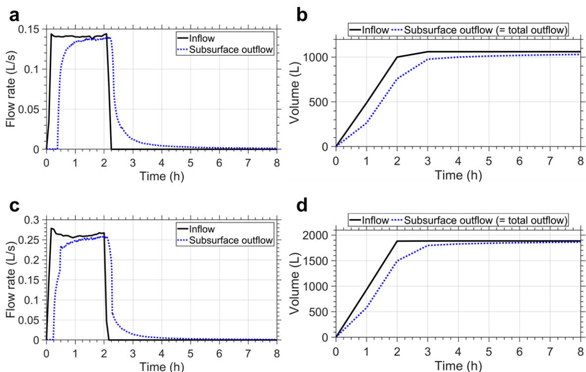
Figure 4.18. Réponses hydrauliques types de la noue de filtration observées en novembre/décembre 2017 (a, c : hydrogrammes - b, d : volumes cumulés). a - b, 0,14 L/s en tête (18/12/2017). c - d, 0,27 L/s en tête (27/11/2017)
