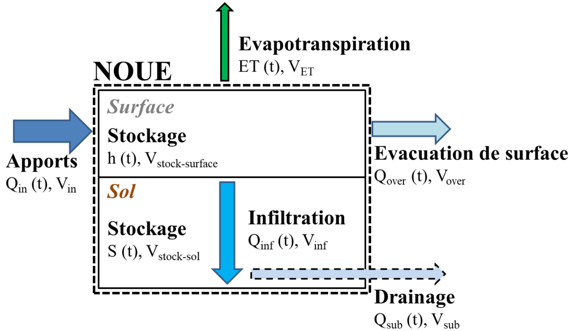
Figure 1.14. Bilan des flux hydriques consécutifs à un évènement de ruissellement en entrée de noue
