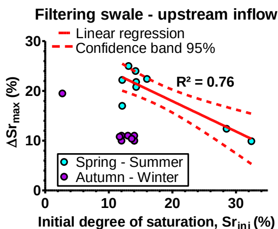
Figure 4.30. Evolutions de l'augmentation maximale du degré de saturation de la partie centrale de la noue de filtration en fonction de son degré de saturation initial (alimentation en tête) et régressions linéaires correspondantes (les résultats des alimentations sur la période automne – hiver 2017 n'ont pas été incorporés à la régression linéaire)
