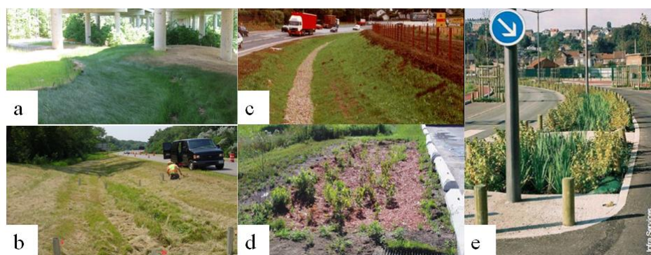
Figure 1.1. Diversité de la couverture d'une noue. a noue enherbée (Luell, 2011). b noue enherbée (Ahmed et al., 2014a). c noue doté d'un lit central empierré (Jefferies, 2004). d noue plantée recouverte d'un paillis (Toronto and Region Conservation Authority, 2008). e noue plantée (Infra Services - Conseil Général Hauts-de-Seine (2010))
