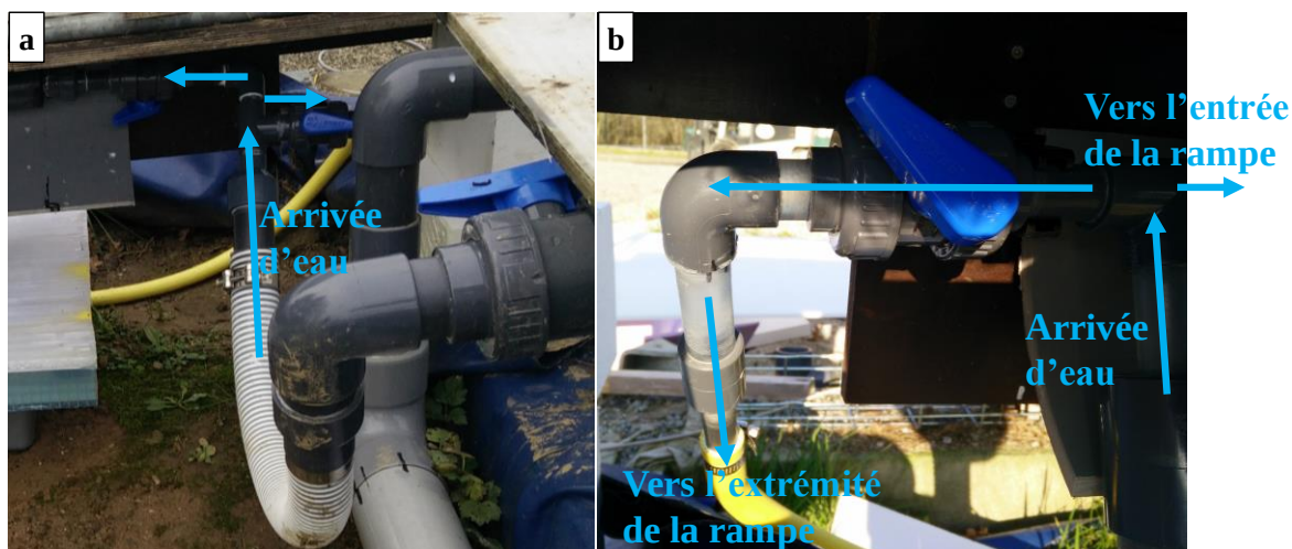
Figure 3.27. Dispositif de répartition du flux entrant entre les deux extrémités du tuyau d'alimentation latérale. a. Vue d'ensemble du dispositif de répartition du flux. b. Zoom sur une vanne de réglage de la répartition du flux
