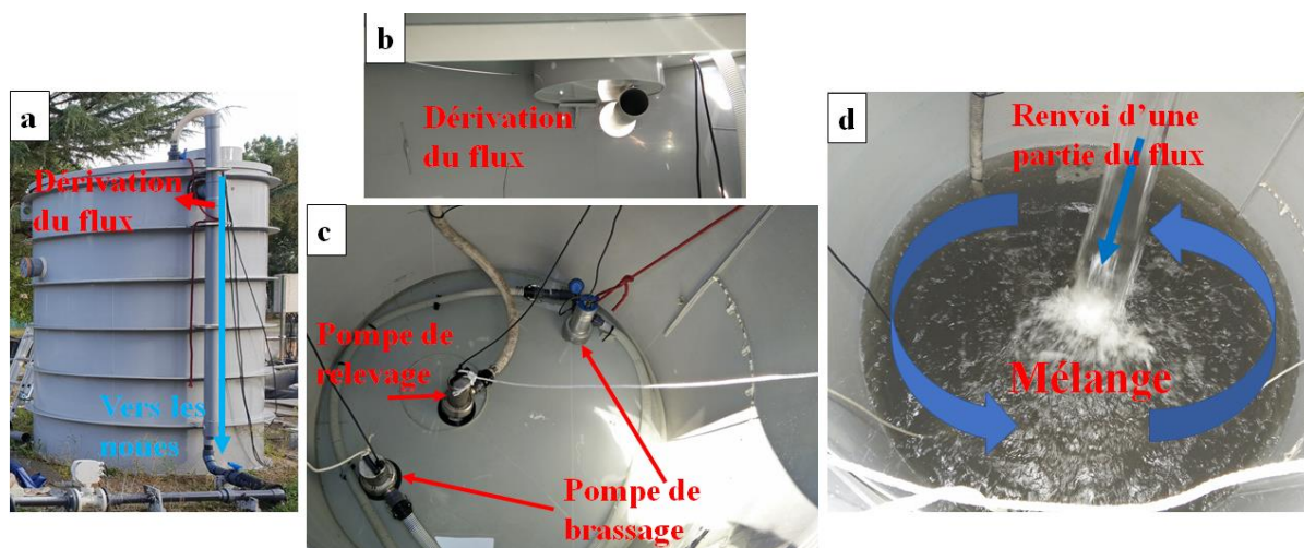
Figure 3.23. Caractéristiques de la cuve principale d'injection des eaux pluviales (volume \sim 7 \text{ m}^3 ). a. Extérieur de la cuve et du dispositif de dérivation du flux d'eau. b. Dispositif de dérivation du flux d'eau depuis l'intérieur de la cuve. c. Pompes de relevage et de brassage des eaux (intérieur de la cuve). d. Intérieur de la cuve lors d'une simulation d'évènement sur le pilote (mélange des eaux en continu)
