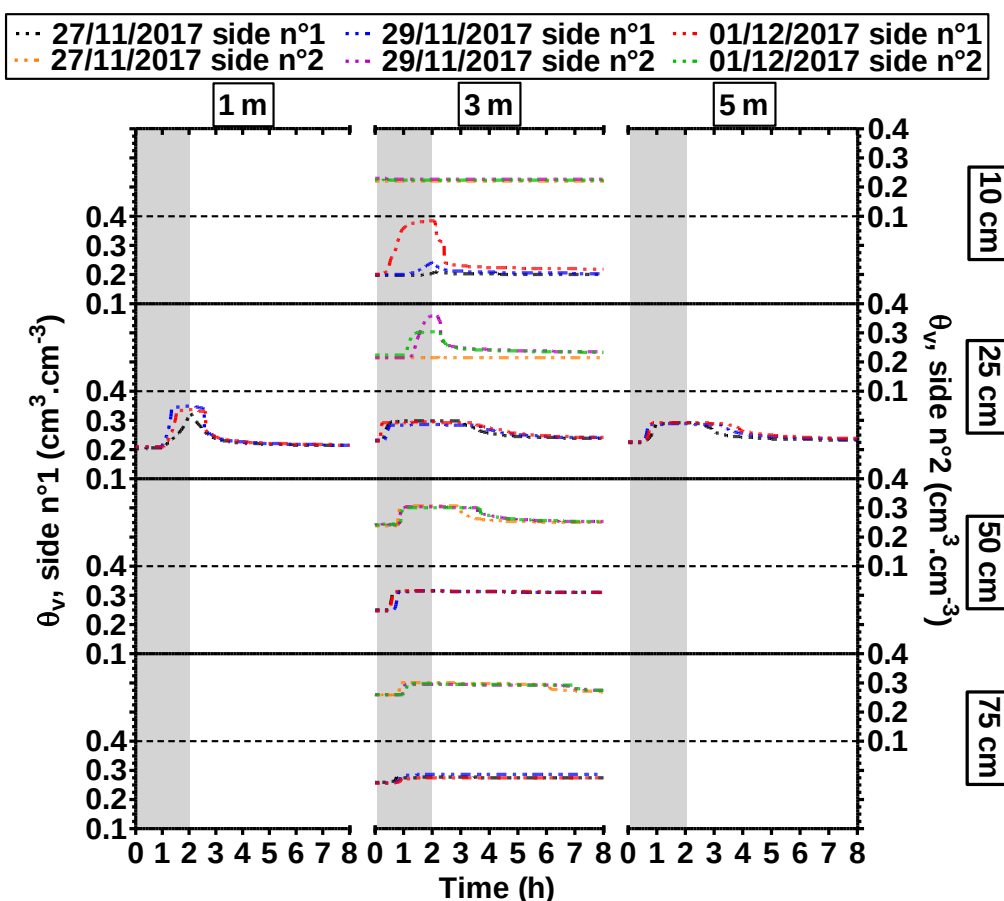
Figure 4.10. Evolutions types de \theta_v au sein des talus (side n°1 = talus pouvant être alimenté latéralement) de la noue standard lors d'alimentations (en gris sur la Figure) en tête à 0,27 L/s (3 positions par rapport à l'amont – 1, 3 et 5 m – et 4 profondeurs par rapport à la surface du fond de la noue – 10, 25, 50 et 75 cm)
