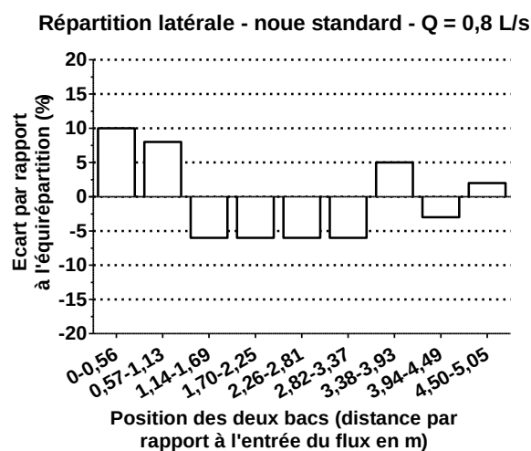
Figure 3.31. Caractérisation de l'uniformité de la répartition de l'eau lors d'une injection latérale (0,8 L/s)
