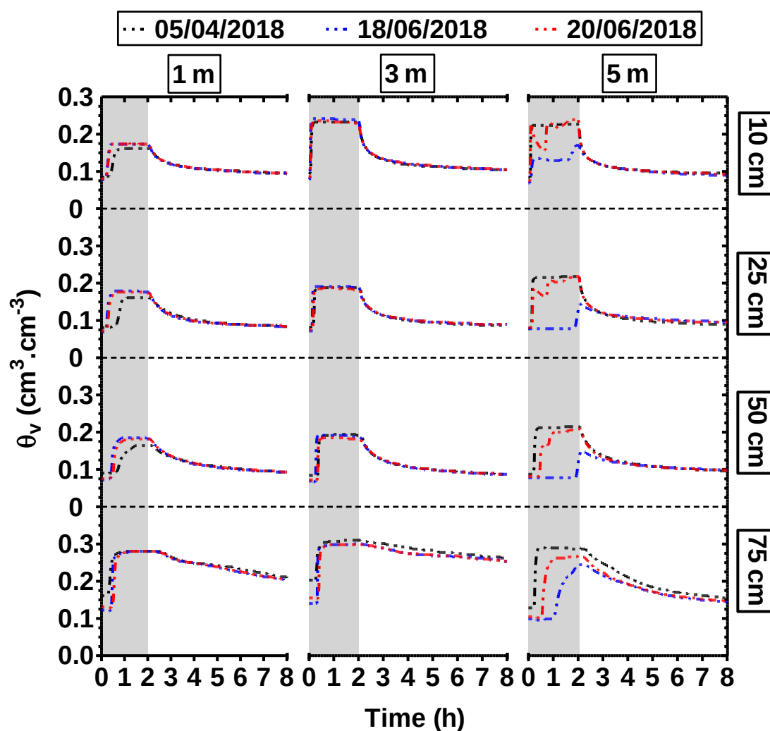
Figure 4.24. Evolutions types de la teneur en eau volumique \theta_v au sein de la partie centrale de la noue de filtration lors d'alimentations (en gris sur la Figure) en tête à 0,27 L/s (3 positions par rapport à l'amont – 1, 3 et 5 m – et 4 profondeurs – 10, 25, 50 et 75 cm)
