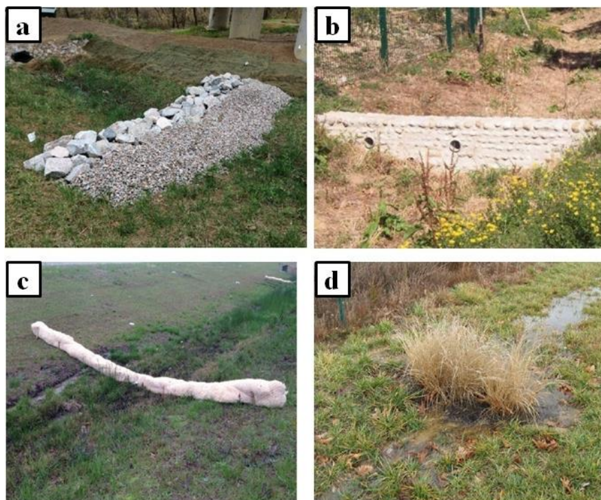
Figure 1.11. Exemples de configurations de cloisons pouvant être aménagées dans une noue. a. cloison construite avec des roches (photographie extraite de Powell (2015)). b. cloison empierrée avec orifices de régulation du débit (crédit photo : conseil général des Hauts de Seine). c. cloison filtrante (photographie extraite de Powell (2015)). d. cloison végétalisée (photographie extraite de Jamil (2009))
