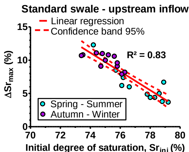
Figure 4.15. Evolutions de l'augmentation maximale du degré de saturation de la partie centrale de la noue standard en fonction de son degré de saturation initial (alimentation en tête) et régressions linéaires correspondantes
