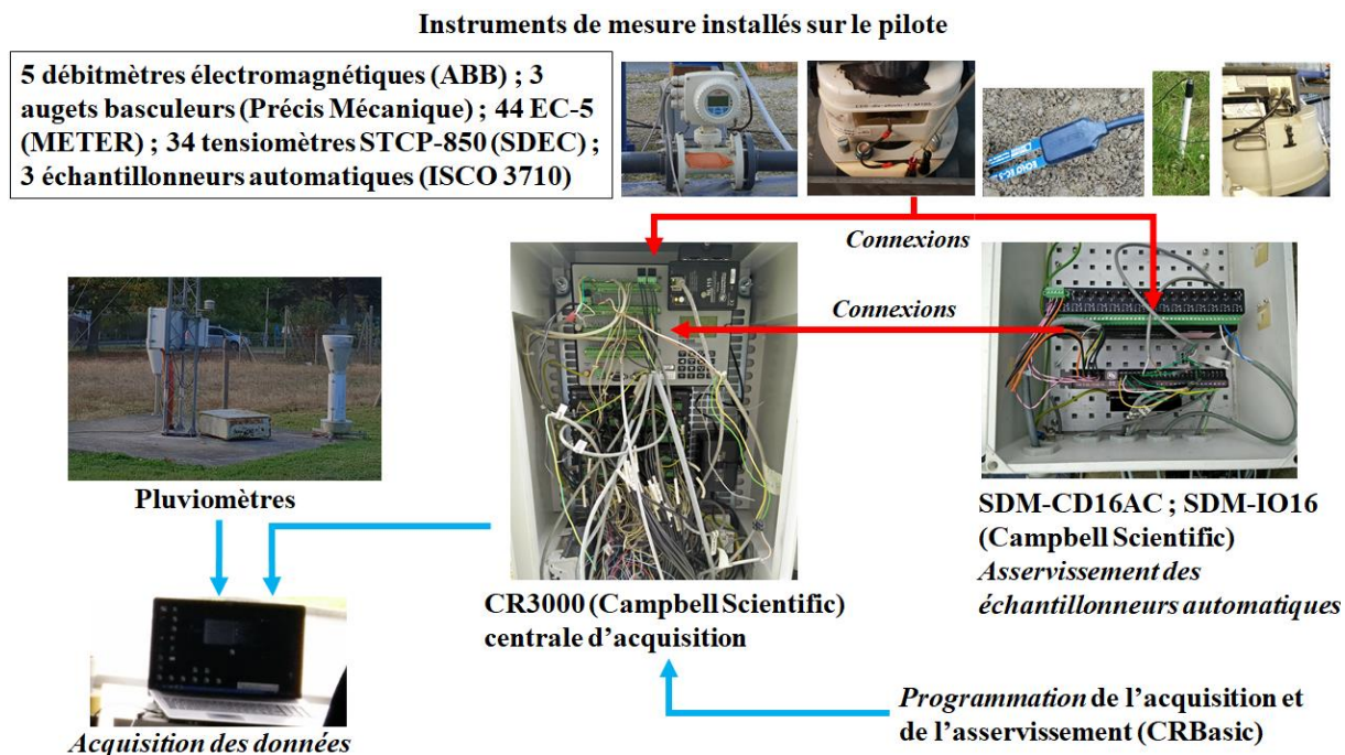
Figure 3.33. Instrumentation du pilote
