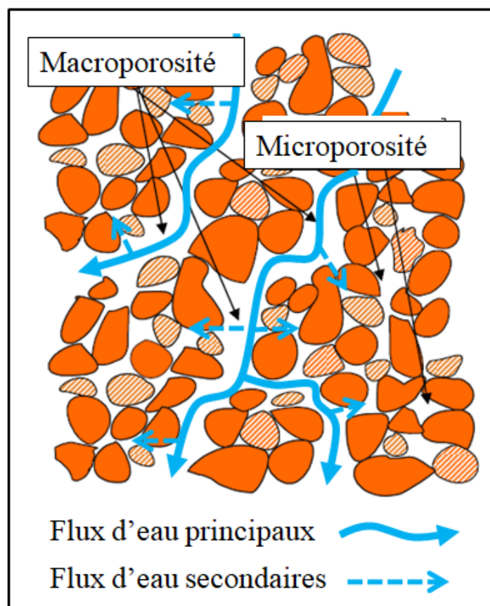
Figure 1.5. Structure d'un sol en termes de porosité et schématisation des écoulements (schéma adapté de Lassabatere (2002))
