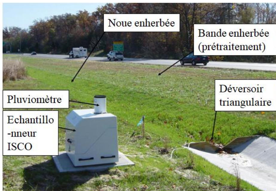
Figure 1.10. Bande enherbée végétalisée aménagée en amont d'une noue enherbée de bord de route (photographie extraite et traduite de Davis et al. (2012))
