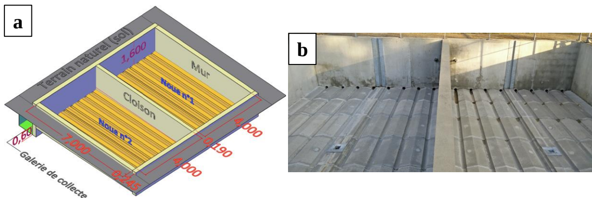
Figure 3.1. Dispositif d'essai de la plateforme Aquasim (CSTB Nantes) dans lequel ont été aménagées les noues. a. Schéma du dispositif d'essai (dimensions en mètre). b. Dispositif d'essai en septembre 2016
