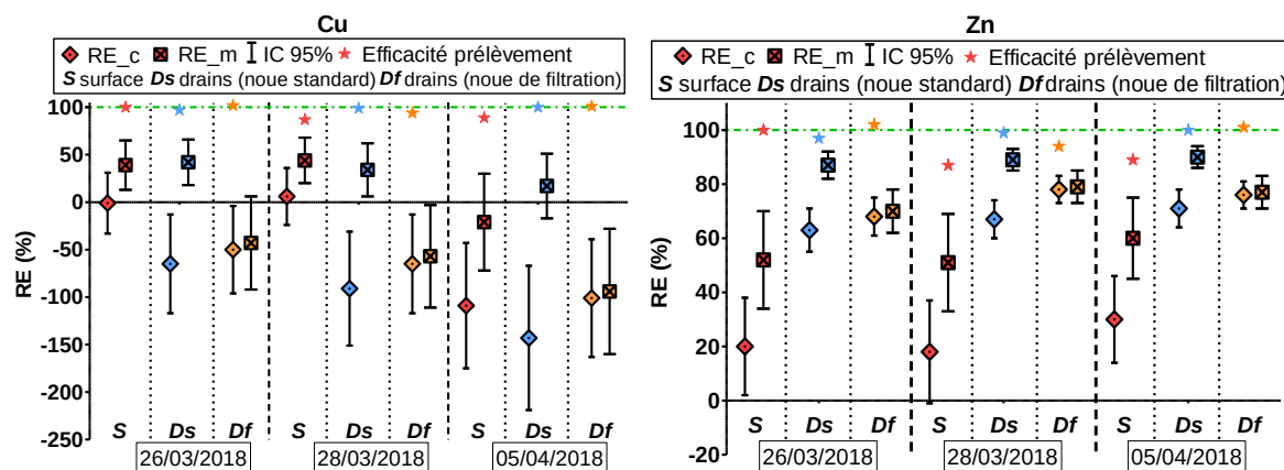
Figure 3.40. Evaluation de la reproductibilité des indicateurs de performances épuratoires pour Cu et Zn
