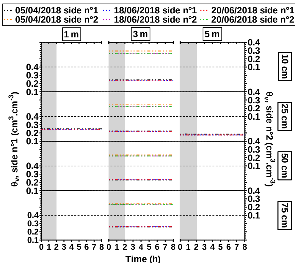
Figure 4.25. Evolutions types de \theta_v au sein des talus (side n°1 = talus pouvant être alimenté latéralement) de la noue de filtration lors d'alimentations (en gris sur la Figure) en tête à 0,27 L/s (3 positions par rapport à l'amont – 1, 3 et 5 m – et 4 profondeurs par rapport à la surface du fond de la noue – 10, 25, 50 et 75 cm)
