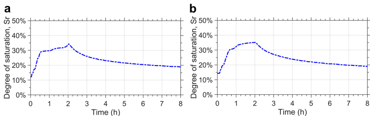
Figure 4.28. Evolutions types des degrés de saturation de la partie centrale de la noue de filtration (alimentations en tête). a. 0,14 L/s. b. 0,27 L/s
