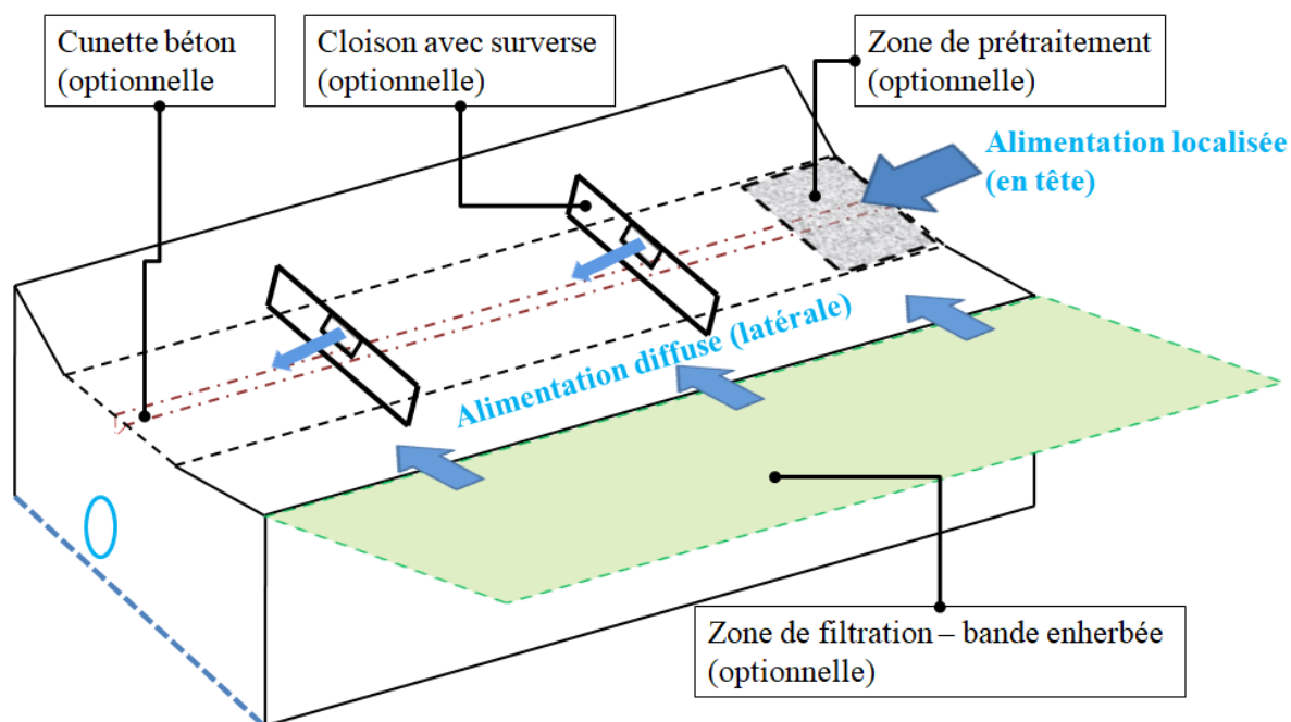
Figure 1.8. Configurations optionnelles sur une noue pour améliorer ses performances hydrologiques et épuratoires ou préserver sa durée de vie (limiter l'érosion)
