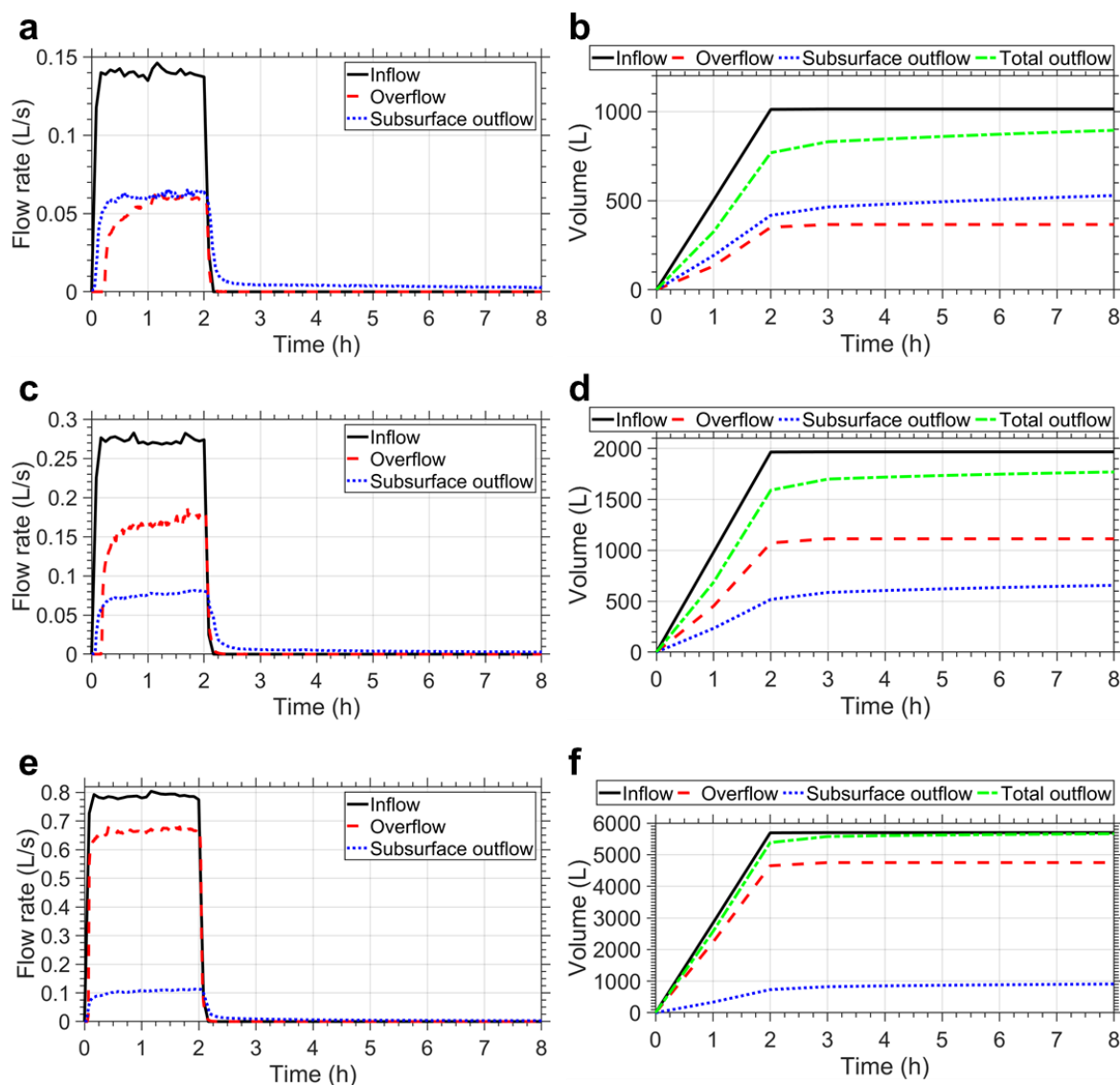
Figure 4.5. Réponses hydrauliques types de la noue standard observées entre mars et juin 2018 (a, c, e : hydrogrammes – b, d, f : volumes cumulés). a - b. Alimentation 0,14 L/s en tête (18/04/2018). c - d. Alimentation 0,27 L/s en tête 18/06/2018). e - f. Alimentation 0,8 L/s en tête (14/05/2018)
