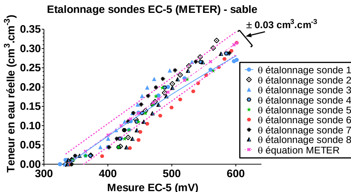
Figure 3.36. Résultats des courbes d'étalonnage de 8 sondes EC-5 et comparaison avec la droite d'étalonnage donnée par le constructeur (incertitude de \pm 0,03 \text{ cm}^3.\text{cm}^{-3} )
