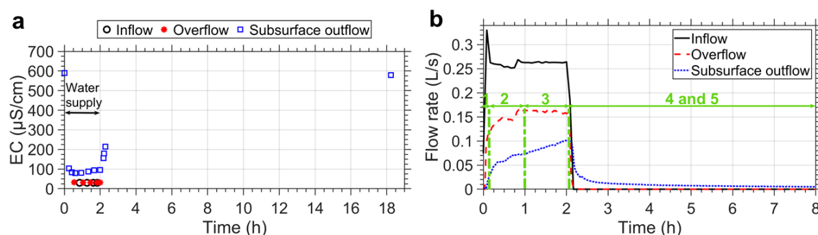
Figure 4.8. Evolution de la conductivité électrique EC à l'entrée et aux sorties de la noue standard (alimentation 0,27 L/s latérale – 20/03/2018). a. Evolution de EC. b. Hydrogrammes avec les différentes phases d'évolution de la conductivité électrique en sortie de drains (en vert)
