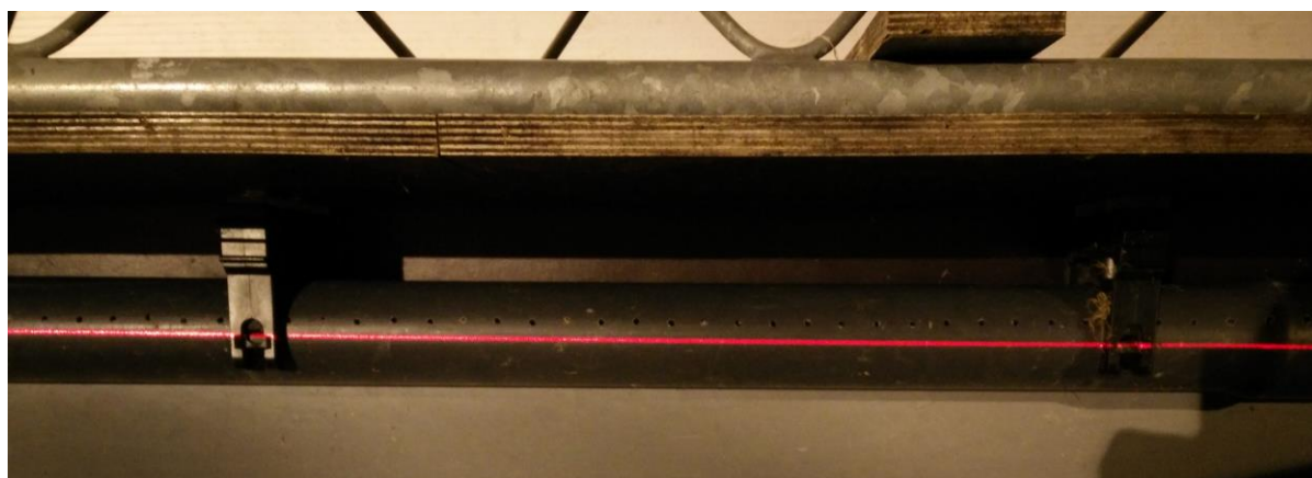
Figure 3.28. Photographie du réglage de la planéité des trous d'une rampe latérale à l'aide d'un laser
