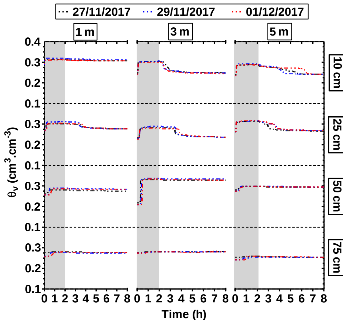
Figure 4.9. Evolutions types de la teneur en eau volumique \theta_v au sein de la partie centrale de la noue standard lors d'alimentations (en gris sur la Figure) en tête à 0,27 L/s (3 positions par rapport à l'amont – 1, 3 et 5 m – et 4 profondeurs – 10, 25, 50 et 75 cm)
