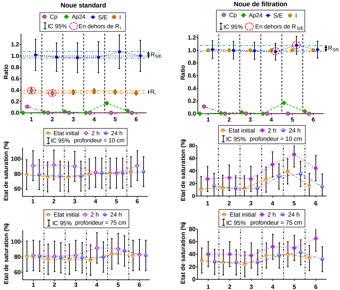
Figure 3.39. Evaluation de la reproductibilité du fonctionnement hydraulique des deux noues lors des six essais simulés (5,4 mm/h pendant 2 h). Les numéros en abscisse indiquent des dates de tests sur le pilote (1 : 27/11/2017, 2 : 29/11/2017, 3 : 01/12/2017, 4 : 26/03/2018, 5 : 28/03/2018, 6 : 05/04/2018)
