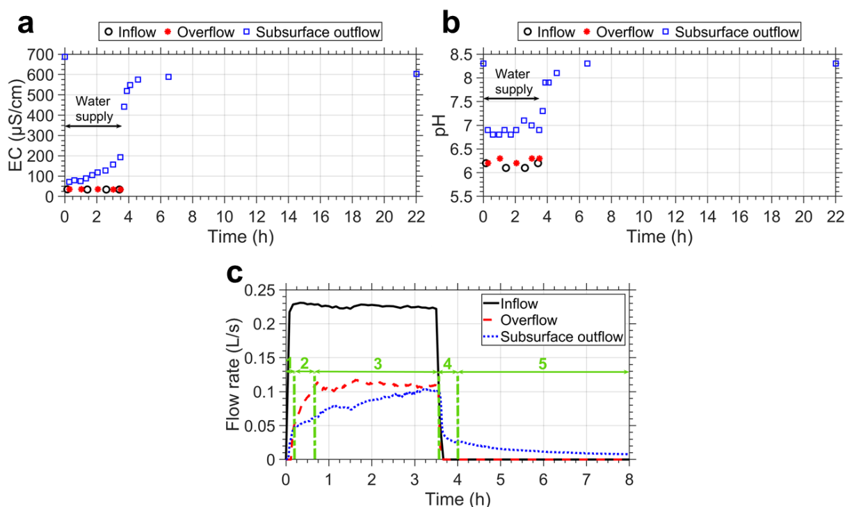
Figure 4.7. Evolution de la conductivité électrique EC et du pH à l'entrée et aux sorties de la noue standard (alimentation 0,225 L/s – 30/01/2018). a. Evolution de EC. b. Evolution du pH. c. Hydrogrammes avec les différentes phases d'évolution de la conductivité électrique en sortie de drains (en vert)
