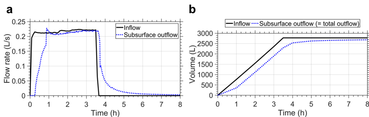
Figure 4.19. Réponse hydraulique type de la noue de filtration à un évènement spécial (a : hydrogrammes - b : volumes cumulés). a - b, 0,225 L/s en tête (30/01/2018)
