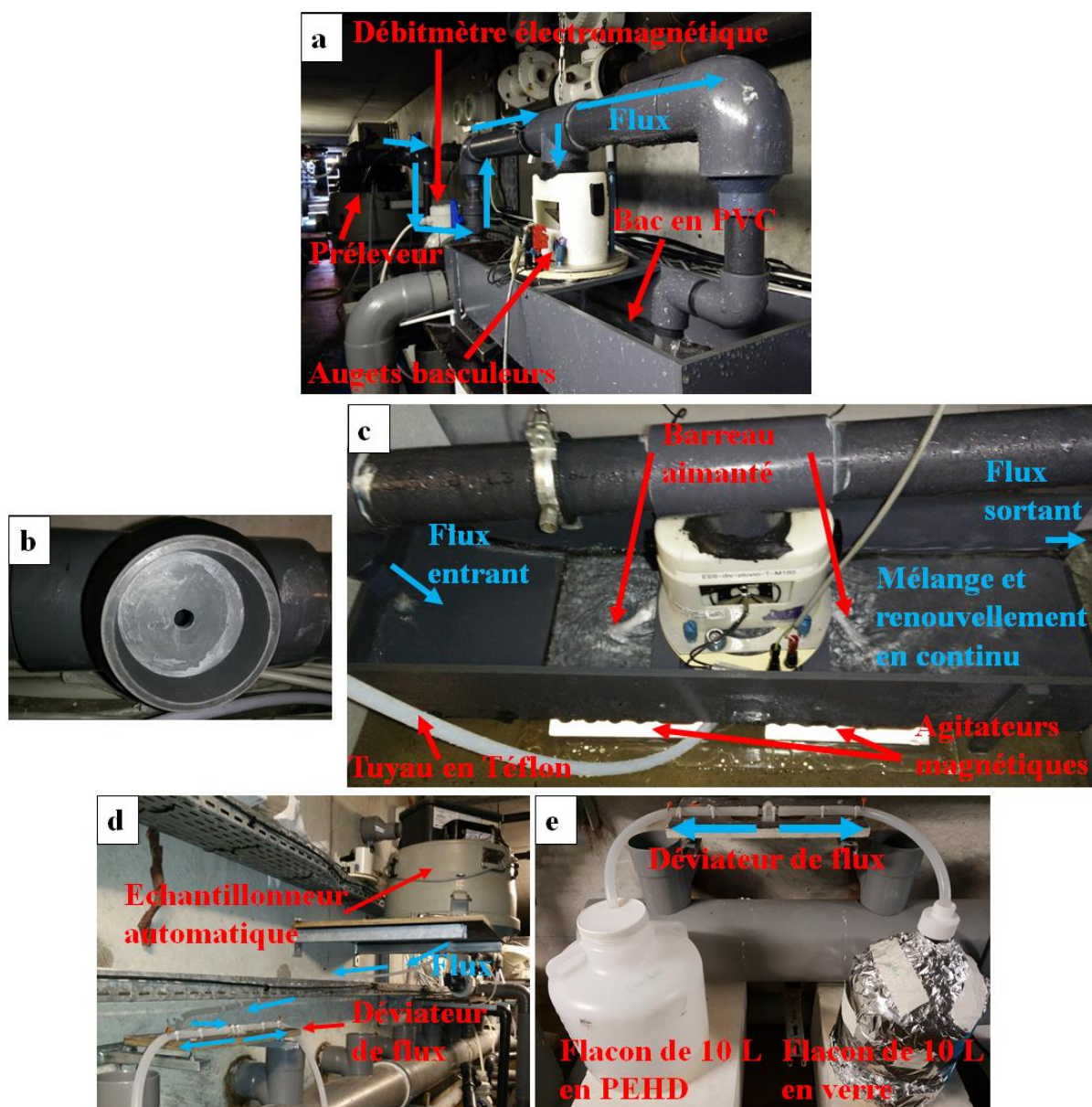
Figure 3.34. Caractéristiques du dispositif de mesure des débits/volumes sortant d'une noue (un dispositif par sortie instrumentée) et du système associé de prélèvement automatisé des eaux. a. Vue d'ensemble du système. b.
