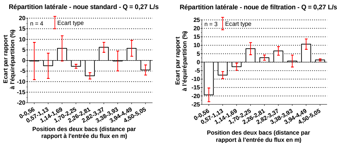
Figure 3.30. Caractérisation de l'uniformité de la répartition de l'eau lors d'une injection latérale (0,27 L/s)
