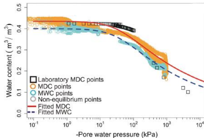
Figure 1.19. Reconstruction d'une courbe h(\theta) à partir de mesures terrain par des sondes de teneur en eau et des tensiomètres (figure extraite de Bordoni et al. (2017))
