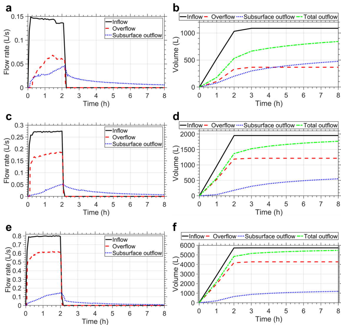
Figure 4.3. Réponses hydrauliques types de la noue standard observées en novembre/décembre 2017 (a, c, e : hydrogrammes – b, d, f : volumes cumulés). a - b. Alimentation 0,14 L/s en tête (18/12/2017). c - d. Alimentation 0,27 L/s en tête (27/11/2017). e - f. Alimentation 0,8 L/s en tête (12/12/2017)
