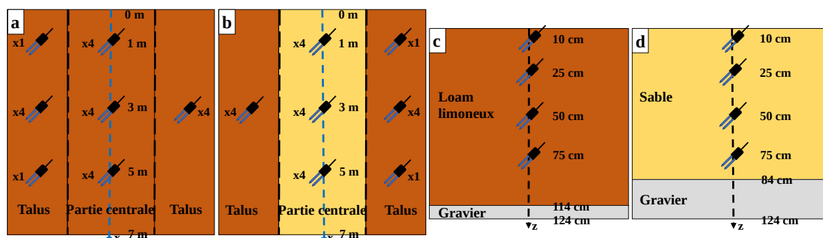
Figure 3.35. Emplacements des sondes de teneur en eau EC-5. a. Positions dans la noue standard (profil en long). b. Positions dans la noue de filtration (profil en long). c. Positions dans la partie centrale de la noue standard (profil en travers). d. Positions dans la partie centrale de la noue de filtration (profil en travers). Les EC-5 dans les talus sont enfouies aux mêmes profondeurs que dans la partie centrale, exceptés les profils verticaux à une sonde (enfouie à 25 cm de profondeur)
