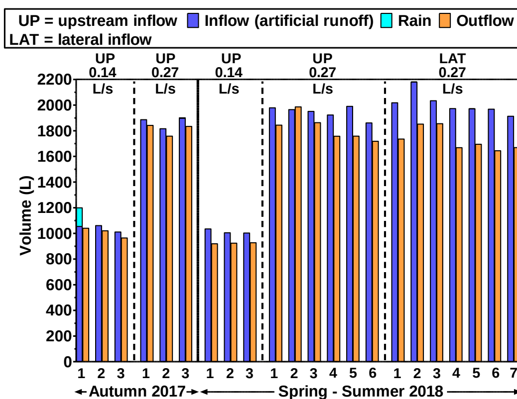
Figure 4.32. Bilans volumiques pour les alimentations en eau de 2 h sur la noue de filtration
