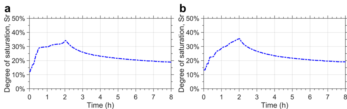
Figure 4.29. Evolutions types des degrés de saturation de la partie centrale de la noue de filtration consécutives à des alimentations en tête et latérale. a. Alimentation 0,27 L/s en tête. b. Alimentation 0,27 L/s latérale.
