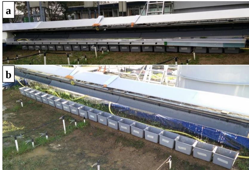
Figure 3.29. Réalisation d'une cartographie de la répartition du flux d'eau sur 5,5 m. a. Couverture des bacs avant d'atteindre un régime hydraulique permanent dans la canalisation. b. Remplissage des bacs avant pesée
