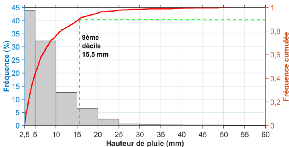
Figure 3.19. Distribution statistique des évènements pluvieux classés par hauteur de pluie \geq 2,5 mm
