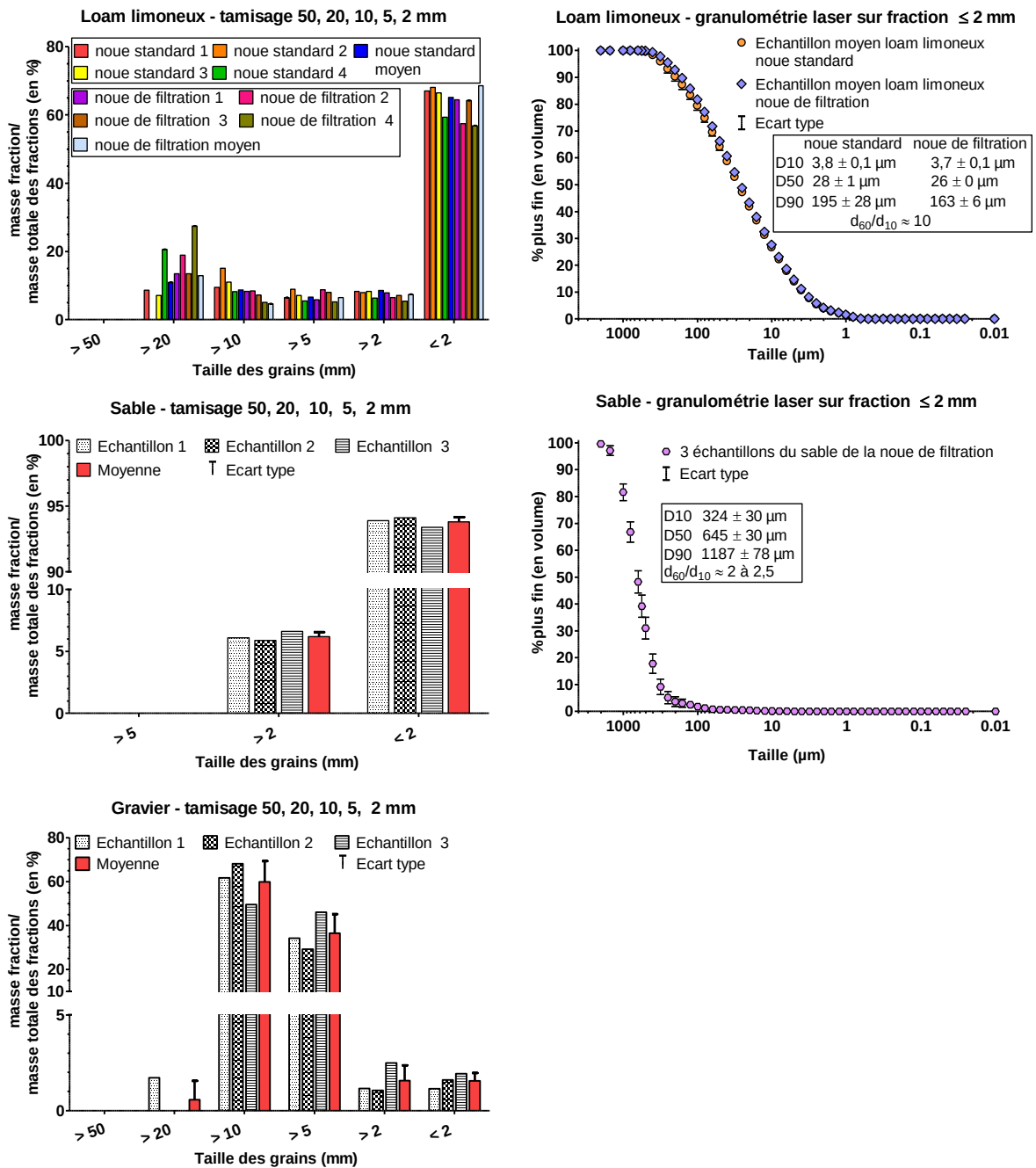
Figure 3.13. Granulométrie (tamis et laser) des matériaux utilisés pour la construction des noues pilotes ; D10, D50 et D90 sont les bornes supérieures respectives des tailles des 10, 50 et 90% des particules les plus fines
