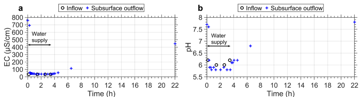
Figure 4.22. Evolution de la conductivité électrique EC et du pH à l'entrée et aux sorties de la noue de filtration (alimentation 0,225 L/s). a. Evolution de EC. b. Evolution du pH
