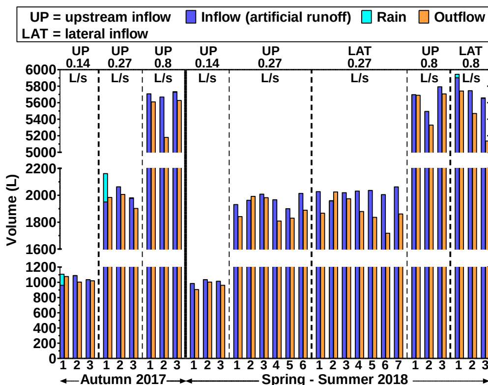
Figure 4.17. Bilans volumiques pour les alimentations en eau de 2 h sur la noue standard
