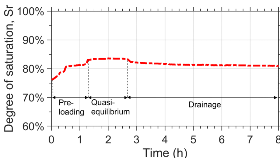
Figure 4.12. Evolution type de l'état de saturation de la partie centrale de la noue standard
