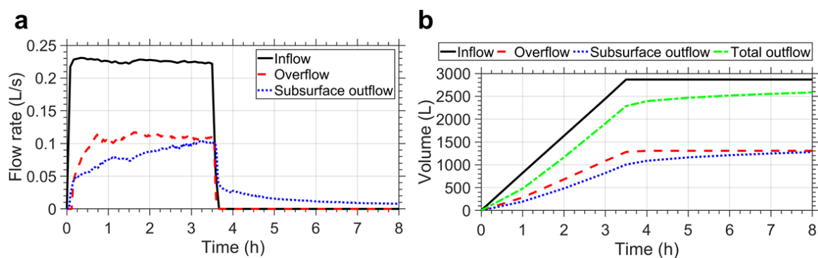
Figure 4.4. Réponse hydraulique type de la noue standard à un évènement spécial (a : hydrogrammes – b : volumes cumulés). a - b. Alimentation 0,225 L/s (30/01/2018)
