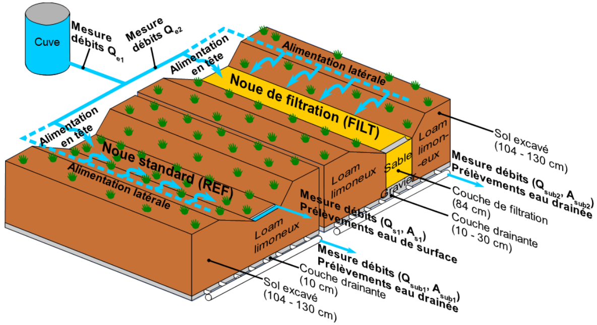
Figure 3.37. Schéma du pilote aménagé au CSTB. Les débits mesurés par les DEM et les augets présentent respectivement les préfixes Q et A
