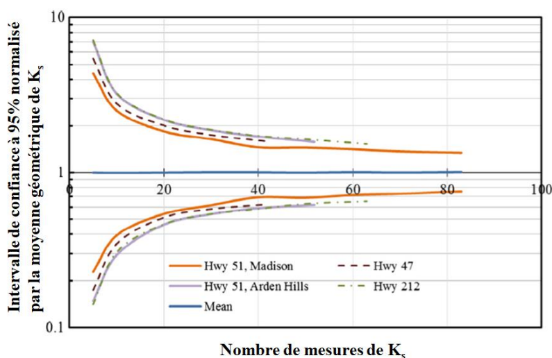
Figure 1.17. Evolution de l'IC95 normalisé par la moyenne géométrique de K_s en fonction du nombre de mesures de K_s dans 4 noues (figure extraite de Ahmed et al. (2015))
