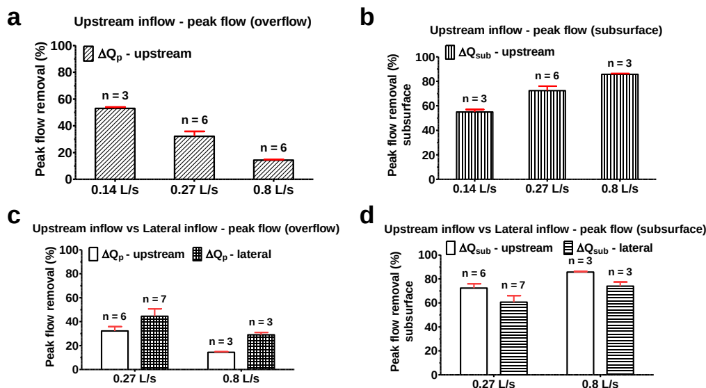
Figure 4.16. Abattements du débit de pointe par la noue standard (alimentations en eau de 2 h). a – b. \Delta Q_p – \Delta Q_{sub} (alimentations en tête). c – d. Comparaison entre les \Delta Q_p – \Delta Q_{sub} observés lors d’alimentations en tête et latérale. Les barres rouges représentent les écarts-types
