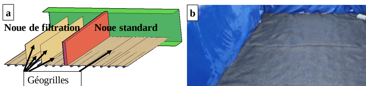
Figure 3.7. Géogrilles utilisées aux interfaces entre les différents types de matériaux (mailles de 500 µm).
