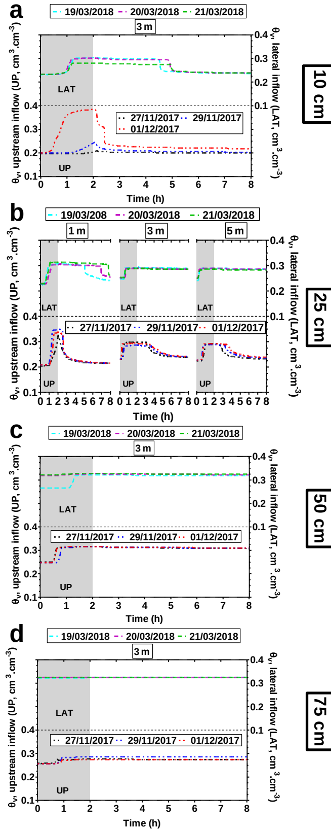
Figure 4.11. Evolutions types de \theta_v au sein du talus de la noue standard pouvant être alimenté latéralement, suite à des alimentations (en gris sur la Figure) en tête (UP) et latérale (LAT) à 0,27 L/s (3 positions par rapport à l'amont – 1, 3 et 5 m). a – d. Profondeurs par rapport à la surface du fond de la noue (10, 25, 50 et 75 cm)
