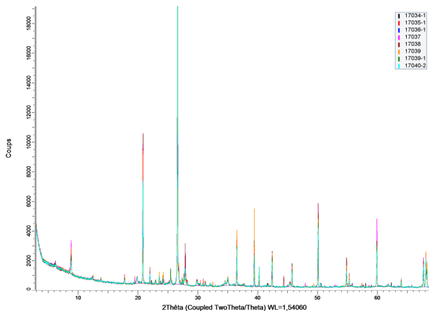
Figure 3.14. Diffractogramme de 8 échantillons du loam limoneux des noues ; ordonnées et abscisses : comptage du détecteur et angle de Bragg pour une longueur d'onde de 1,5406 Å
