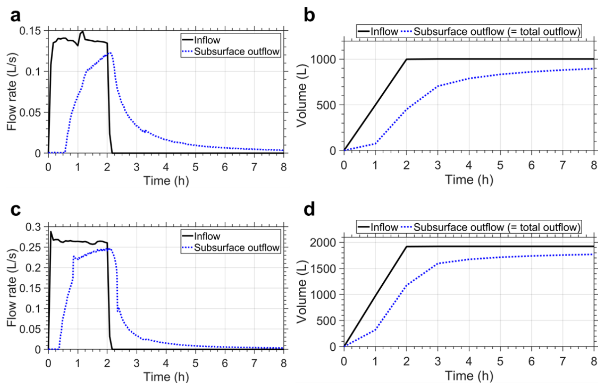
Figure 4.20. Réponses hydrauliques types de la noue de filtration observées entre mars et juin 2018 (a, c : hydrogrammes – b, d : volumes cumulés). a - b, 0,14 L/s en tête (18/04/2018). c - d, 0,27 L/s en tête (18/06/2018)
