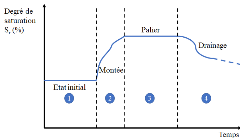
Figure 1.18. Evolution du degré de saturation du massif d'une noue lors d'un événement pluvieux (d'après les résultats de Monrabal-Martinez et al. (2018))
