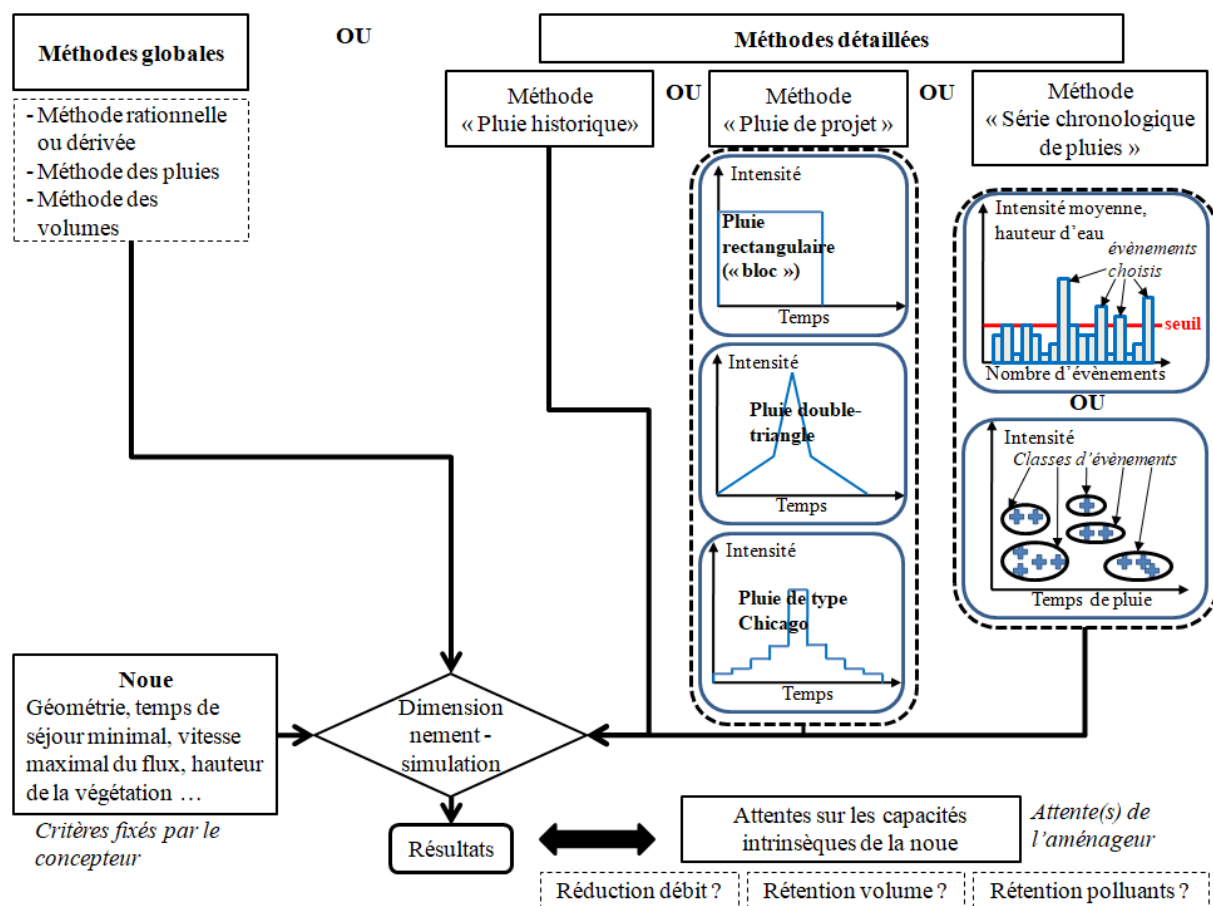
Figure 1.13. Diagramme résumant les méthodes de dimensionnement d'une noue
