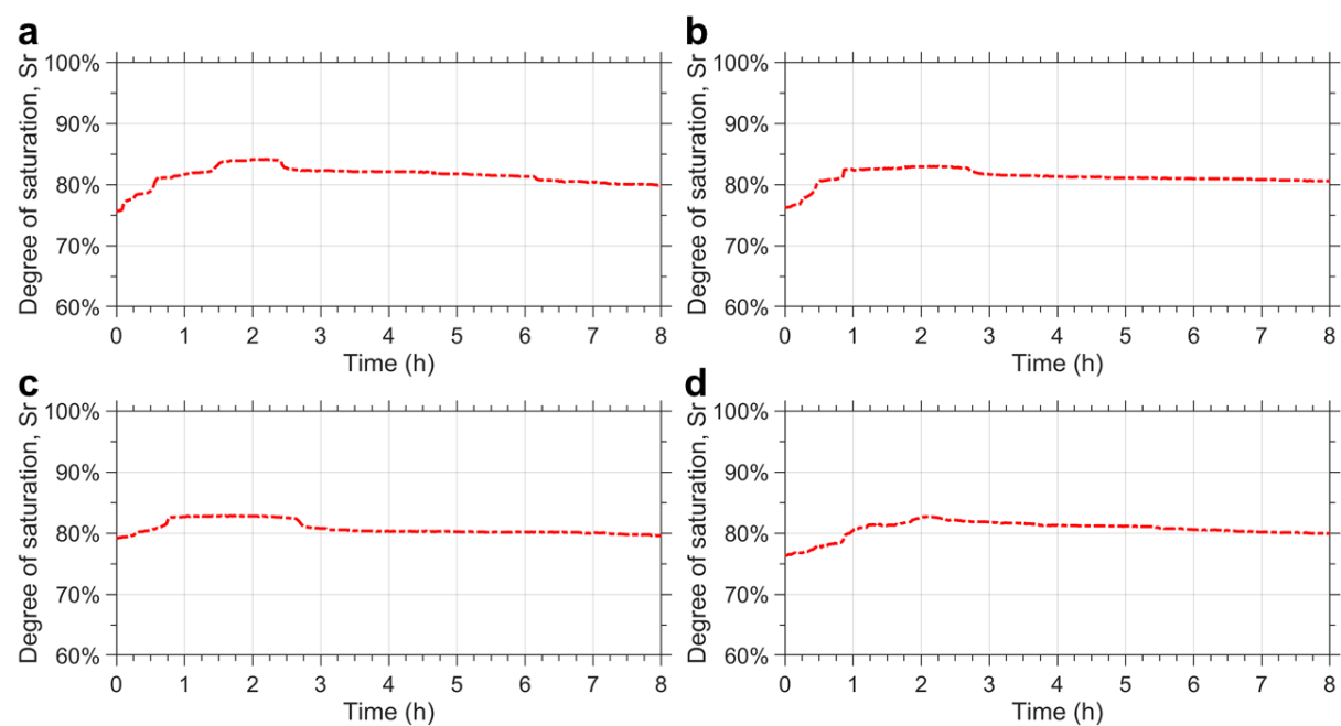
Figure 4.14. Evolutions types des S_r de la noue standard consécutives à des alimentations en tête et latérale. a - b. Alimentation 0,27 L/s en tête - latérale. c - d. Alimentation 0,8 L/s en tête - latérale.
