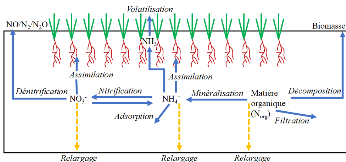
Figure 1.28. Schéma présentant les processus de rétention, de dégradation et de remobilisation des substances azotées au sein de la matrice sol
