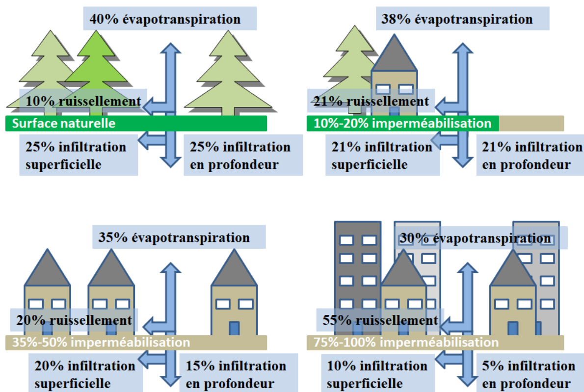
Figure I.1 Evolution des composantes du bilan hydrologique en fonction du taux d'imperméabilisation des sols (d'après Arnold and Gibbons (1996))
