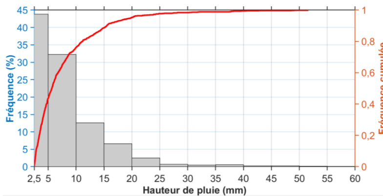
Figure 3.17. Distribution statistique des hauteurs de pluie pour les évènements pluvieux \geq 2,5 mm
