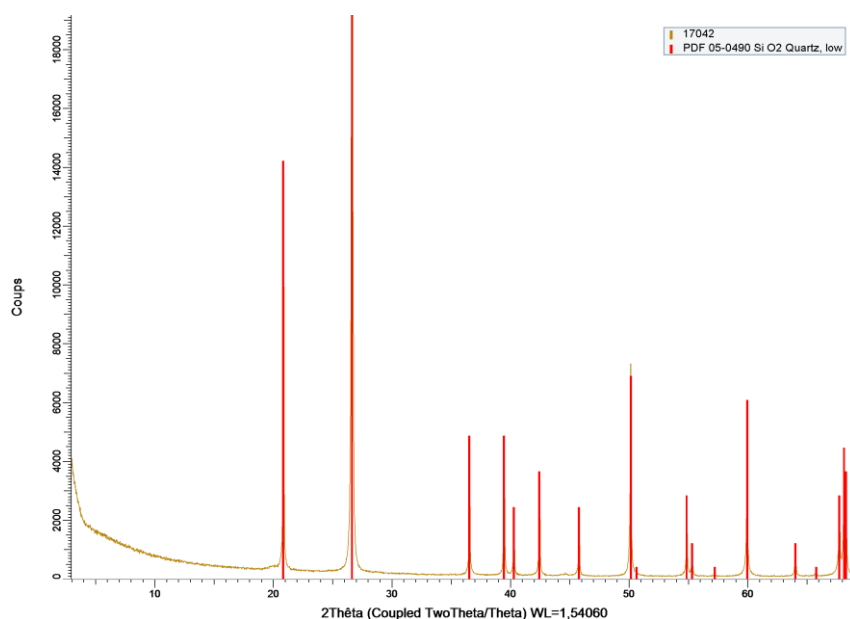
Figure 3.15. Comparaison du diffractogramme type d'un quartz avec celui du gravier des noues (diffractogramme du sable des noues identique) ; ordonnées et abscisses : voir Figure 3.14
