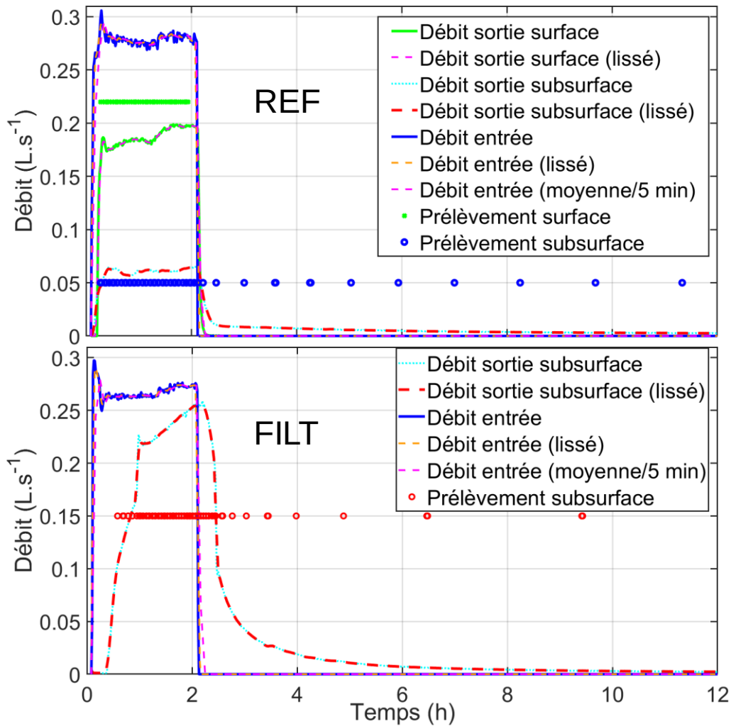
Figure 3.38. Réponses hydrauliques des noues standard REF et de filtration FILT ; les préleveurs sont déclenchés tous les 29 L (surface REF), 17 L (subsurface REF) et 47 L (subsurface FILT)
