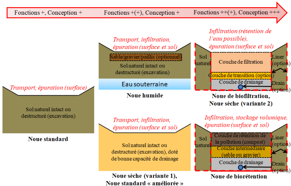
Figure 1.7. Bilan schématique des fonctions et conceptions des principaux types de noues. La diversité des fonctions et le degré de complexité de la conception de la noue sont indiqués par le nombre de +
