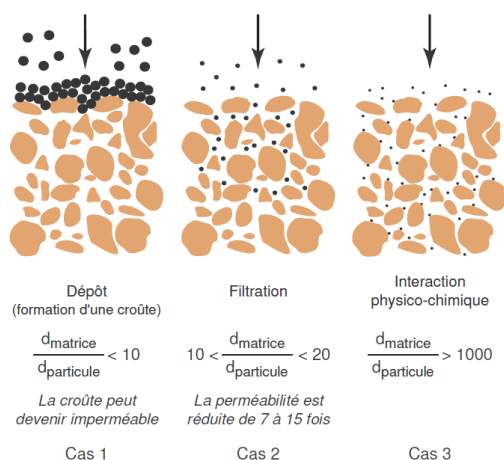
Figure 1.27. Processus de piégeage des particules au sein d'un sol en fonction de la taille des particules et conséquences sur la perméabilité du massif (extrait de Durin (2006))
