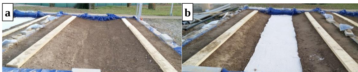
Figure 3.8. Noues pilotes juste après leur construction (décembre 2016). a. Noue standard. b. Noue de filtration
