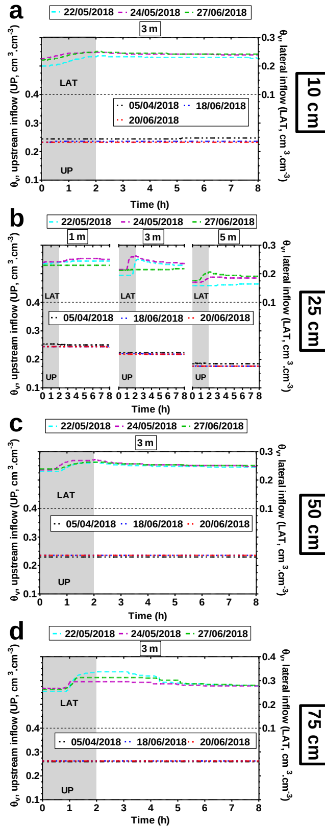
Figure 4.26. Evolutions types de \theta_v au sein du talus de la noue de filtration pouvant être alimenté latéralement, suite à des alimentations (en gris sur la Figure) en tête (UP) et latérale (LAT) à 0,27 L/s (3 positions par rapport à l'amont – 1, 3 et 5 m). a – d. Profondeurs par rapport à la surface du fond de la noue (10, 25, 50 et 75 cm)
