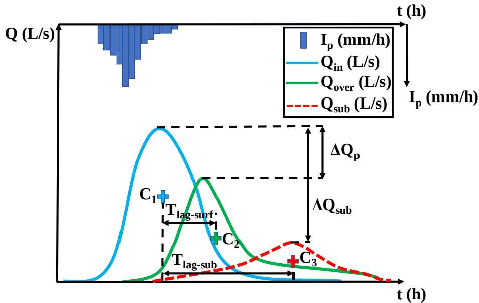
Figure 1.20. Hyétogramme de pluie (intensité de pluie I_p en mm/h) et hydrogrammes associés (débit d'entrée Q_{in} , débits de sortie Q_{over} et Q_{sub} de la noue)
