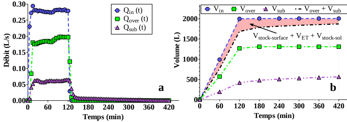
Figure 1.15. Représentation graphique des principaux flux au sein d'une noue. a. Hydrogrammes représentant les flux d'entrée et de sortie. b. Evolution temporelle des composantes volumiques
