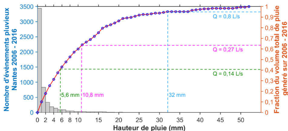
Figure 3.20. Représentativité des hauteurs de pluie des événements simulés par rapport aux pluies enregistrées à Nantes sur la période 2006 – 2016
