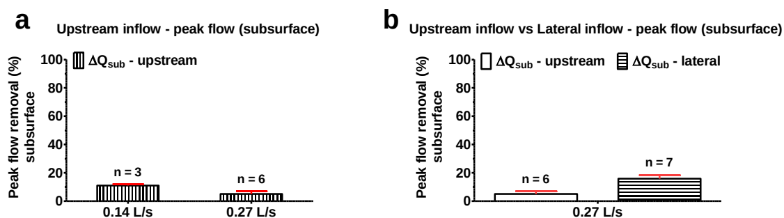
Figure 4.31. Abattements du débit de pointe en sortie de drains de la noue de filtration. a. Alimentation en tête. b. Comparaison des résultats pour des alimentations en tête et latérale
