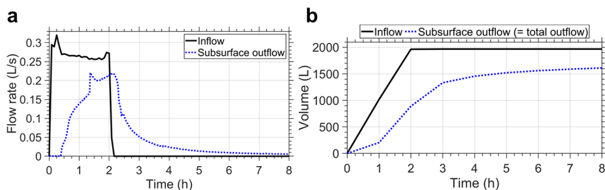
Figure 4.21. Réponses hydrauliques types de la noue de filtration observées suite à des alimentations latérales (a : hydrogrammes – b : volumes cumulés). a – b. Alimentation 0,27 L/s latérale (27/06/2018)
