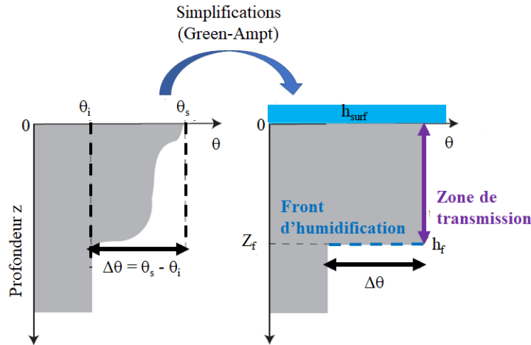
Figure 1.16. Schématisation de la simplification du processus d'infiltration proposée par Green and Ampt (1911) (figure adaptée de Rousseau (2012))
