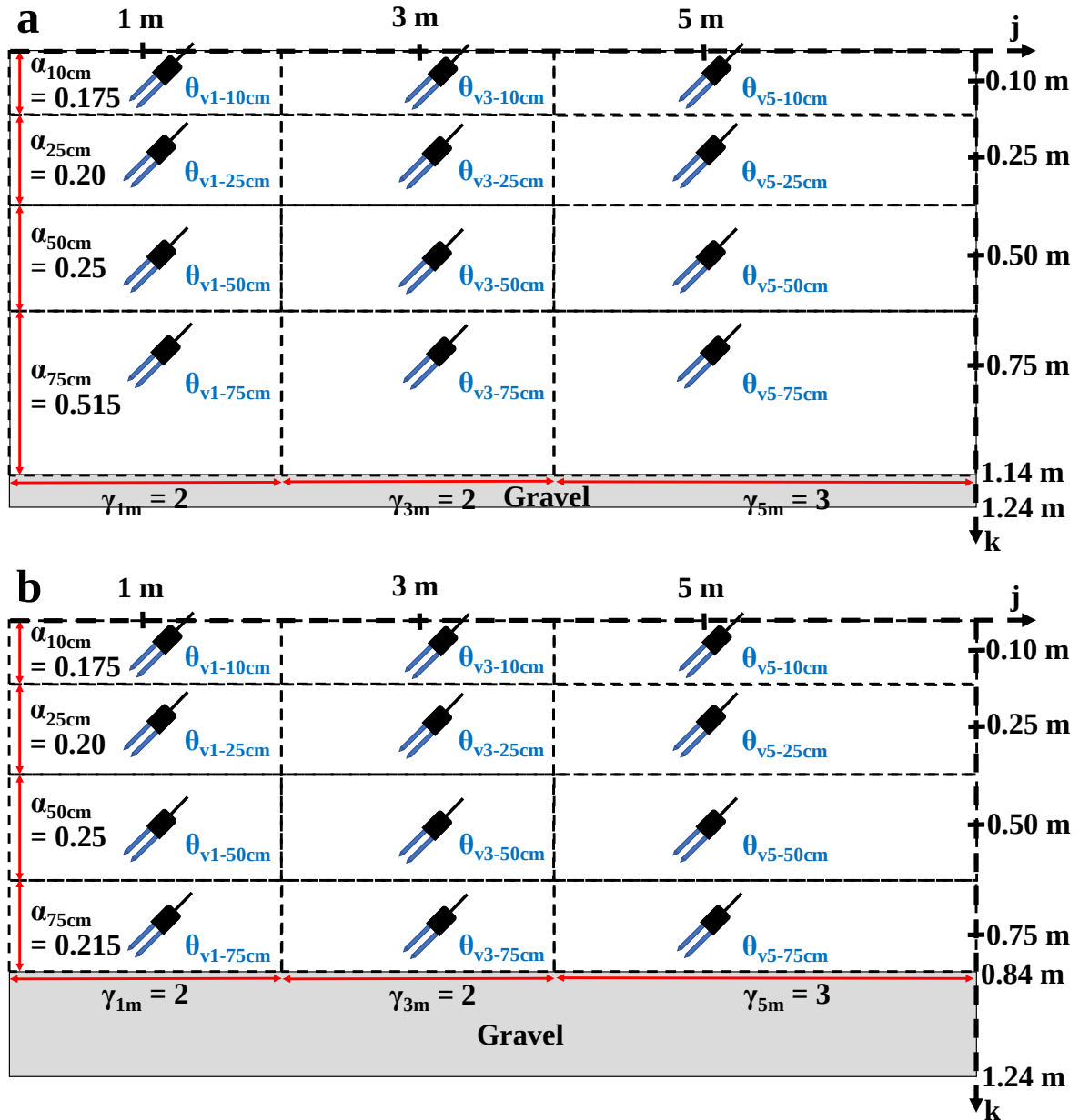
Figure 4.1. Dimensions des strates volumiques choisies et teneurs en eau volumiques associées pour estimer le degré de saturation de la partie centrale d'une noue pilote. a. Noue standard. b. Noue de filtration
