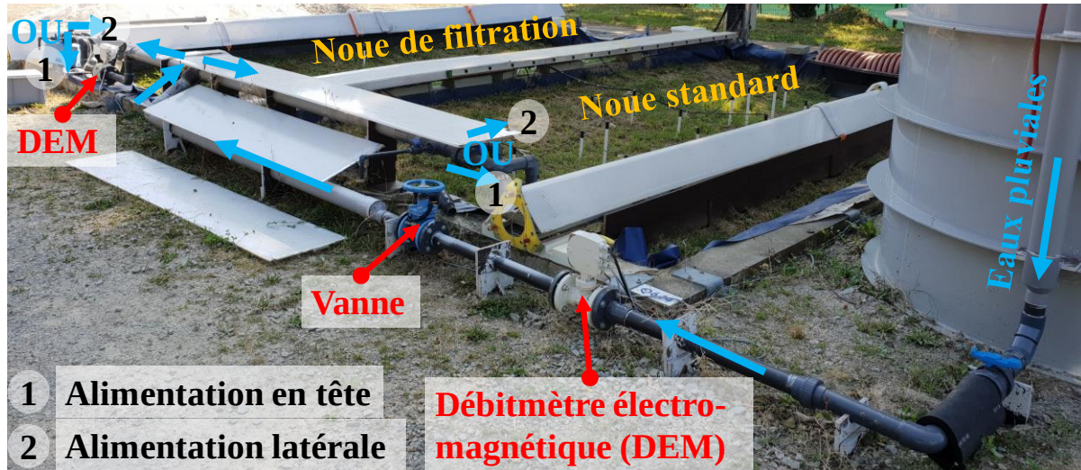
Figure 3.22. Simulateur de ruissellement installé sur le pilote
