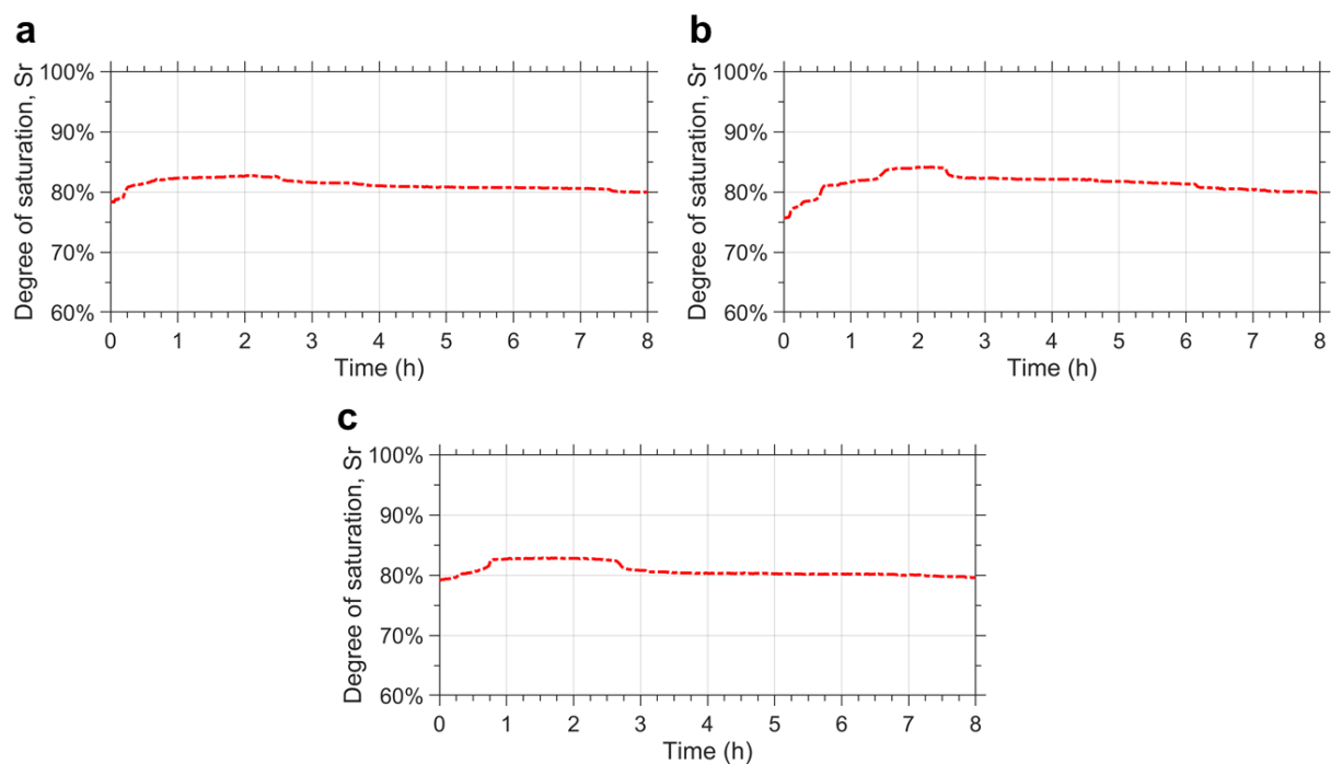
Figure 4.13. Evolutions types des S_r de la noue standard (alimentation en tête). a. 0,14 L/s. b. 0,27 L/s. c. 0,8 L/s
