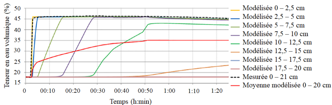
Figure 1.22. Comparaison des profils de teneur en eau volumique donnés par Mike SHE avec le profil mesuré par une sonde intégrant le volume de sol entre 0 et 21 cm de profondeur (modifiée de Rujner et al. (2018b))
