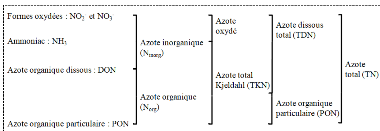
Figure 1.24. Formes de l'azote dans les eaux de ruissellement (adapté de Taylor et al. (2005))
