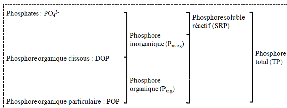
Figure 1.25. Formes du phosphore dans les eaux de ruissellement (Li and Davis, 2016)
