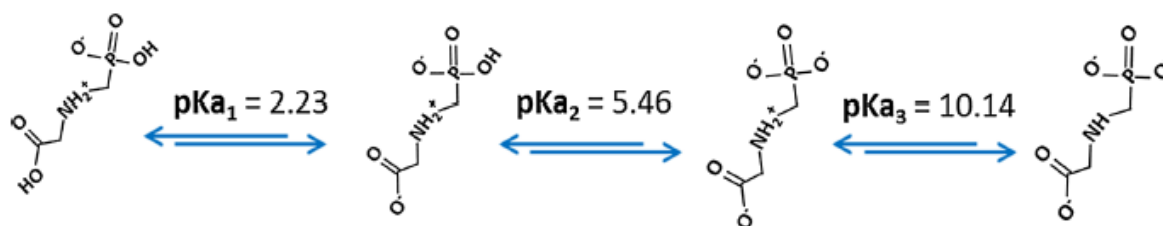
Figure 1.26. Formes du glyphosate en fonction du pH du milieu (extrait de Dollinger et al. (2015)). Les deux formes intermédiaires à un et deux niveaux de charges négatives nettes, sont les plus fréquentes dans les sols ou dans l'eau.
