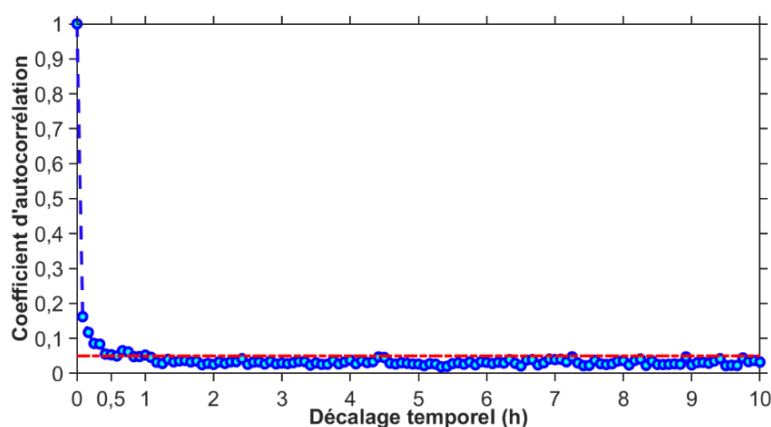
Figure 3.16. Evolution du coefficient d'autocorrélation en fonction du décalage temporel entre deux événements pluvieux successifs (Nantes, 2006-2016)
