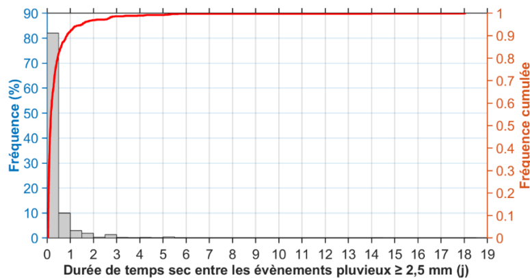
Figure 3.18. Distribution statistique des durées de temps sec observées entre deux évènements pluvieux générant au moins 2,5 mm d'eau (Nantes, 2006-2016)
