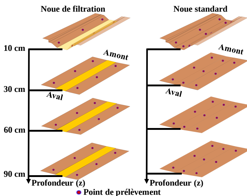
Figure 3.10. Schéma des emplacements des prélèvements de sol (loam limoneux) au sein des noues pilotes
