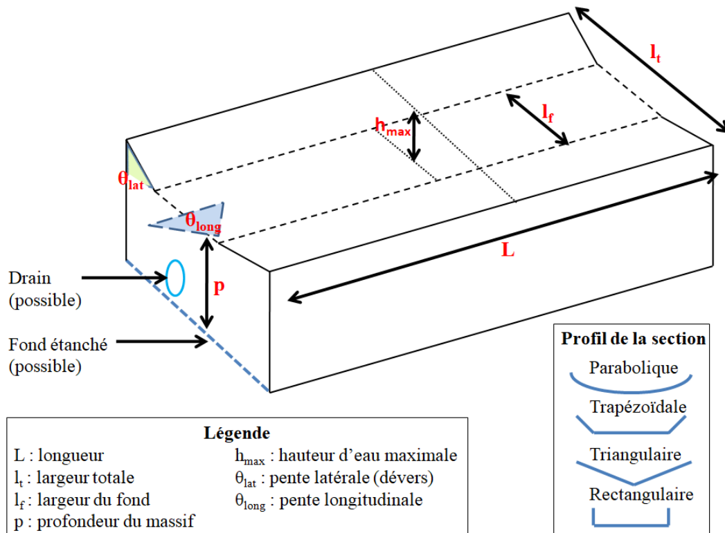
Figure 1.4. Schéma conceptuel d'une noue
