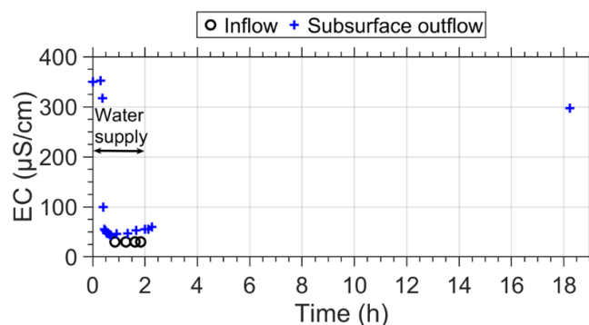
Figure 4.23. Evolution de la conductivité électrique EC à l'entrée et à la sortie de la noue de filtration (alimentation 0,27 L/s latérale)
