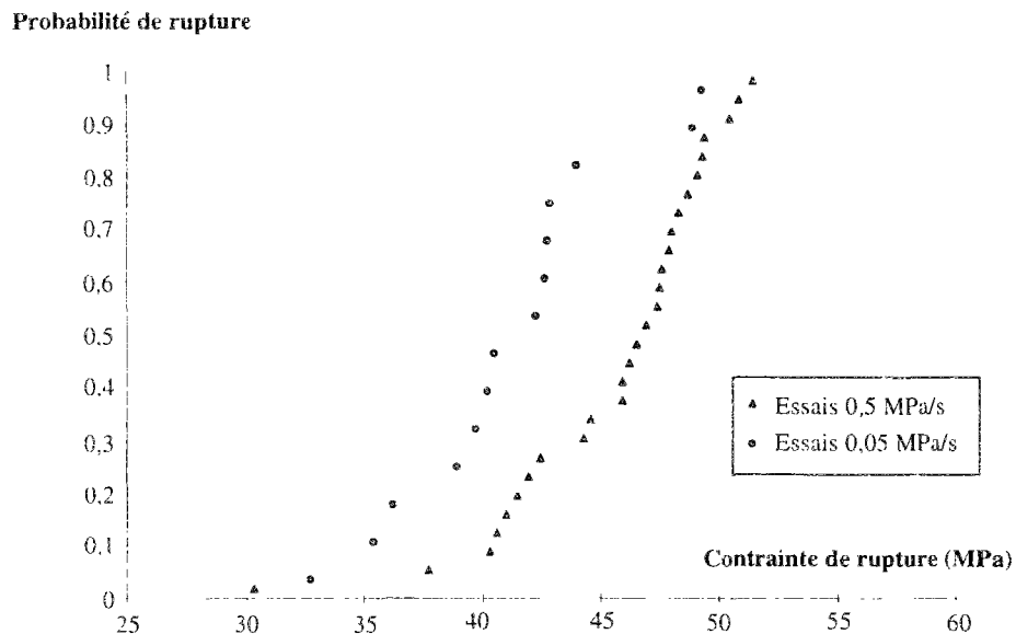
Figure C.21 : Superposition des courbes P_f/\sigma_{\text{rupture}} pour les deux vitesses de la première série
