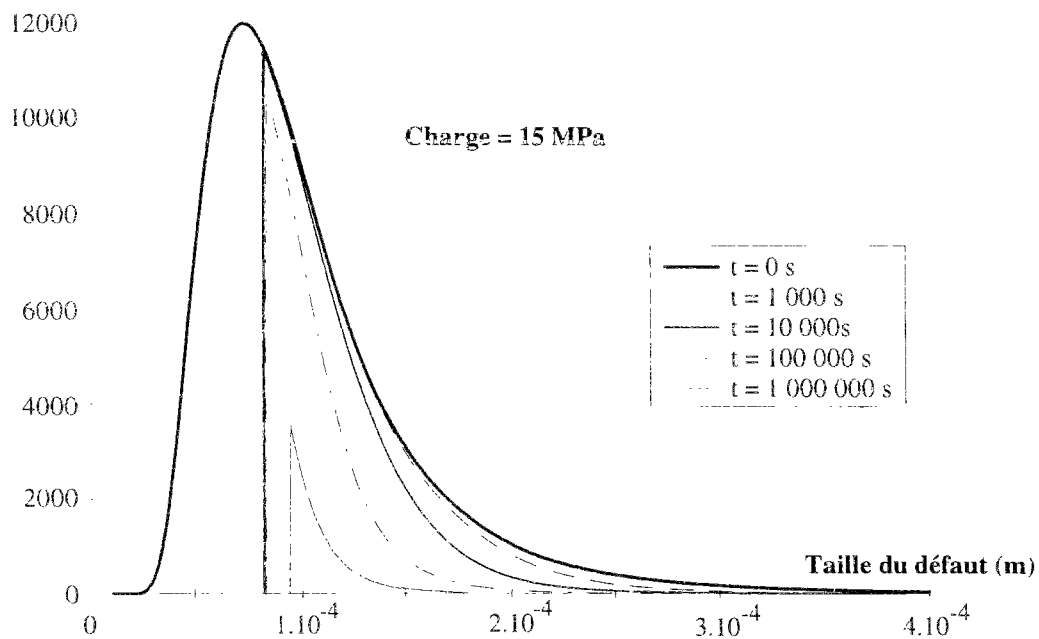
Figure C.26 : Evolution de la distribution des tailles de défauts ( \sigma_a = 15 \text{ MPa} , K_{Ith} = 0,20 \text{ MPa.m}^{1/2} )
