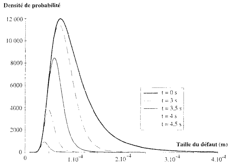
Figure C.29 : Evolution de la distribution des tailles de défauts ( \dot{\sigma} = 10 \text{ MPa/s} , K_{Ith} = 0,15 \text{ MPa.m}^{1/2} )
