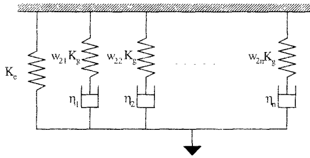
Figure B.3 : Représentation du modèle de Maxwell généralisé pour la partie volumique
