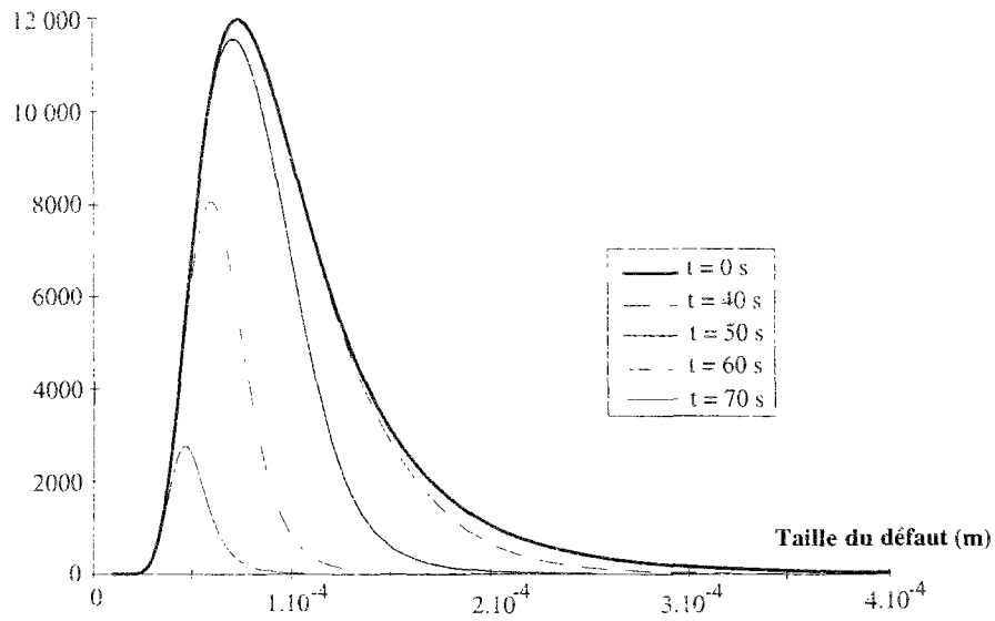
Figure C.30 : Evolution de la distribution des tailles de défauts ( \dot{\sigma} = 0,5 \text{ MPa/s} , K_{\text{Ith}} = 0,15 \text{ MPa} \cdot \text{m}^{1/2} )
