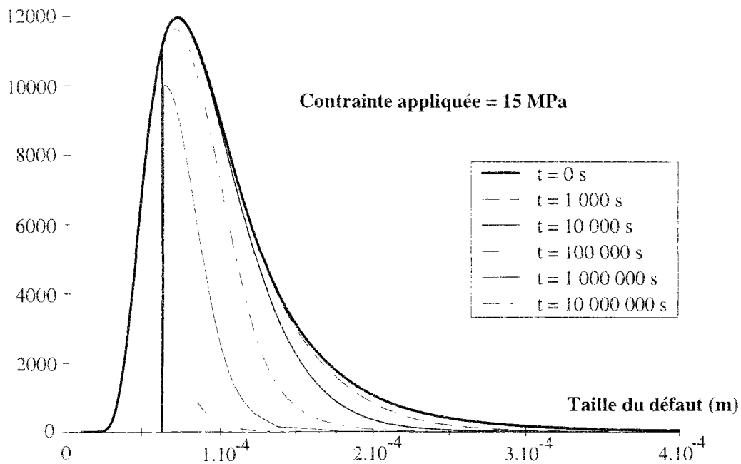
Figure C.25 : Evolution de la distribution des tailles de défauts ( \sigma_a = 15 \text{ MPa} , K_{Ith} = 0,15 \text{ MPa.m}^{1/2} )
