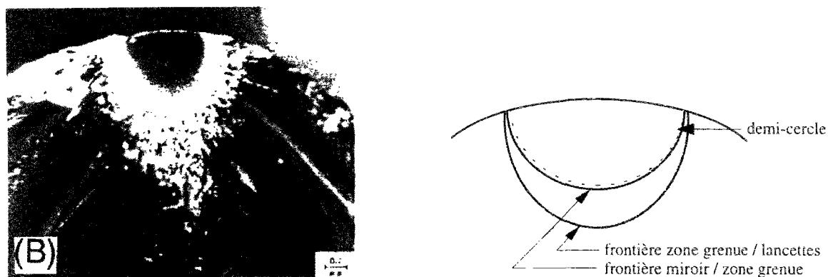
Figure A.11 : Faciès de rupture local pour un élément cylindrique
