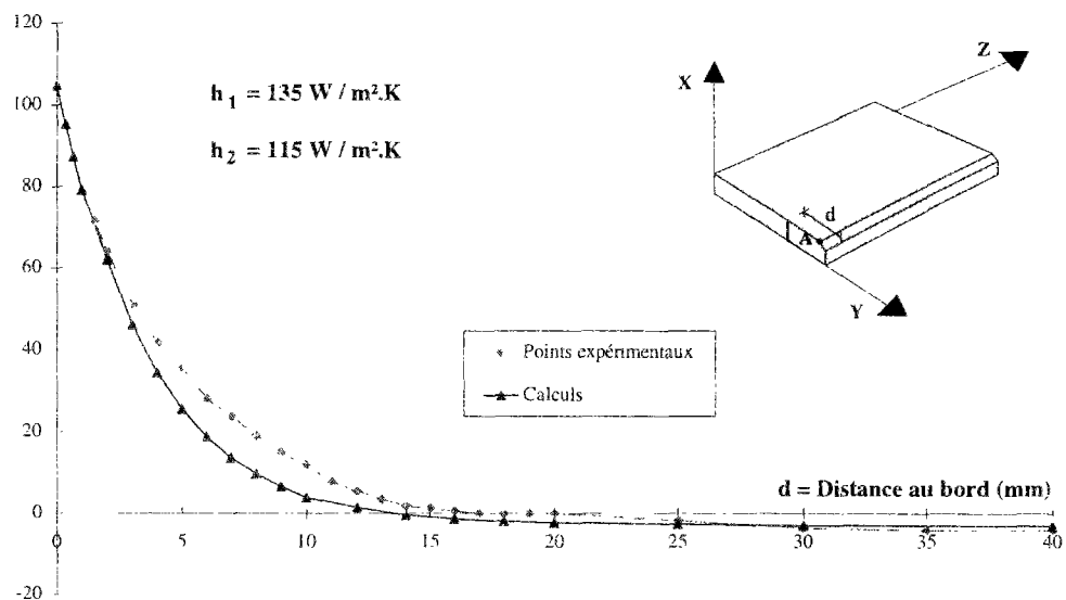
Figure B.37 : Variations de l'intégrale de la différence des contraintes principales en fonction de la distance au bord mesurées et calculées
