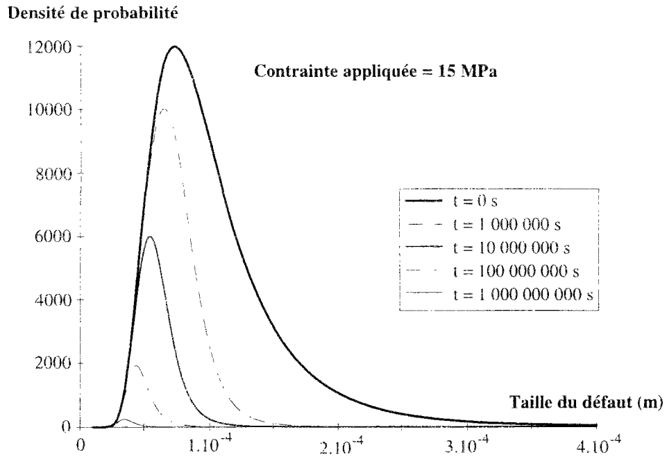
Figure C.23 : Evolution de la distribution des tailles de défauts avec le temps ( \sigma_{\text{appliquée}} = 15 MPa)
