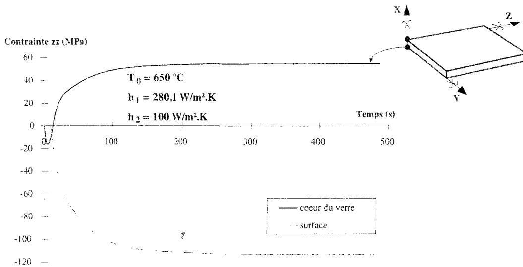
Figure B.17 : Variations des contraintes au cours du temps
