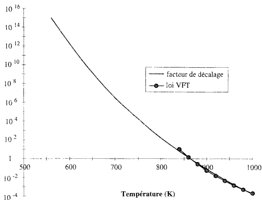
Rapport des temps de relaxation à T et T_{ref} en fonction de la température
