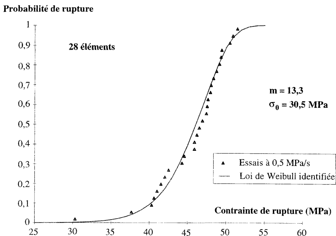
Figure C.15 : Probabilité de rupture en fonction de la contrainte de rupture (essais à 0,5 MPa/s)
