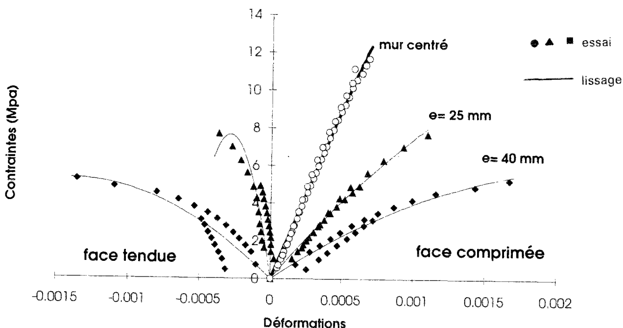
Figure 2.27- Courbes \sigma - \epsilon globale des trumeaux en bloc pour différentes excentricités.
