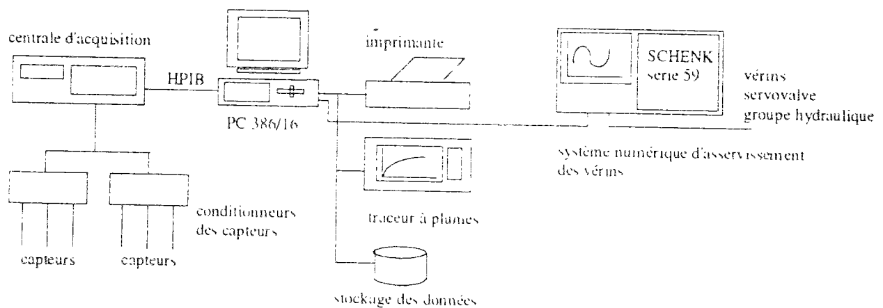
Figure 2.1- Schéma du système d'acquisition et de traitement des données.
