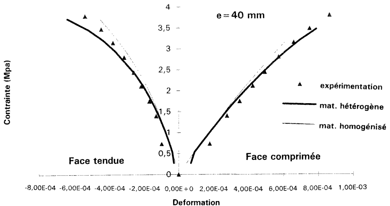
Figure 4.9- Courbes ( \sigma - \epsilon ) expérimentale et théorique des trumeaux sous charge excentrée ( e = 40 \text{ mm} ).
