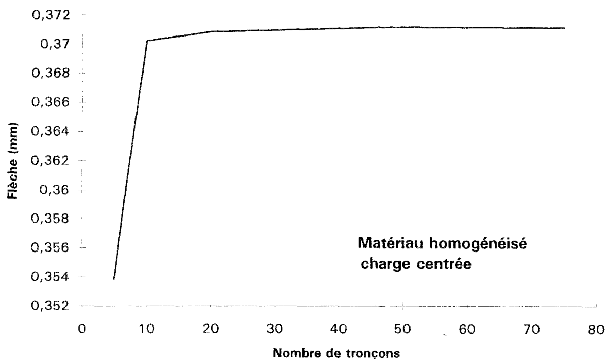
Figure 4.16- Influence du maillage sur la valeur de la flèche à mi-hauteur du mur.
