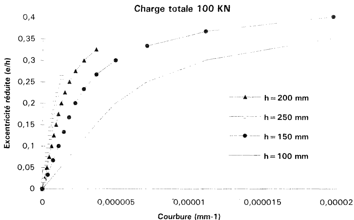
Figure 4.6- Influence de l'épaisseur des blocs sur les lois e(\frac{1}{r}, N) .
