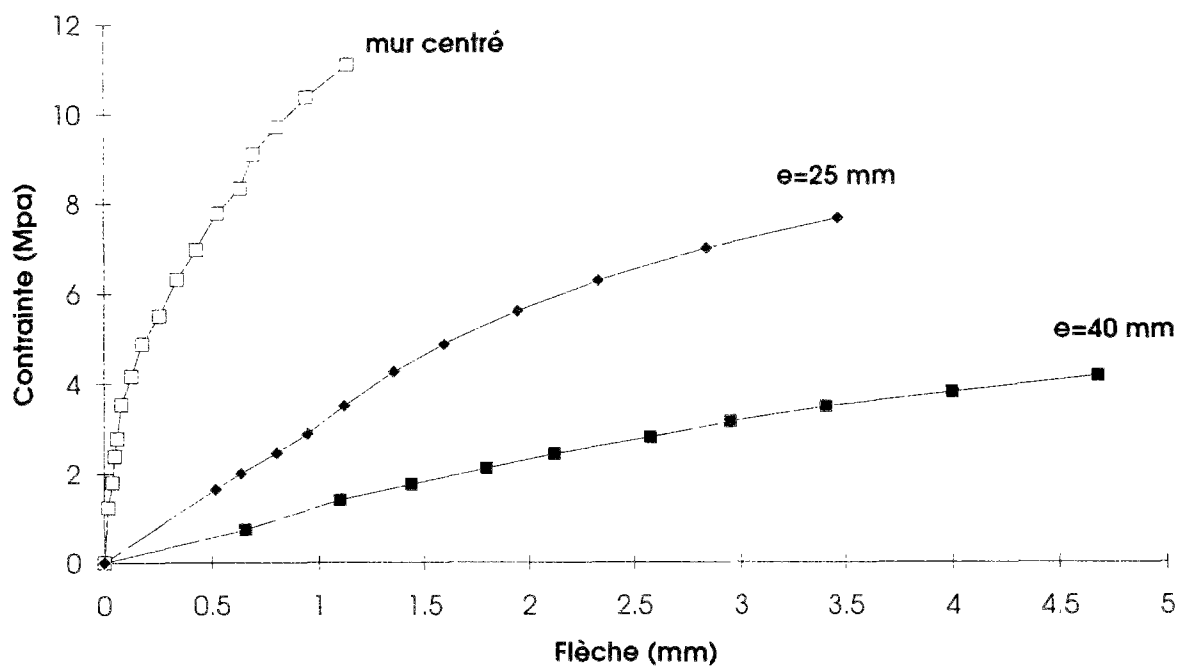
Figure 2.29- Variation de la flèche à mi-hauteur en fonction de la contrainte .
