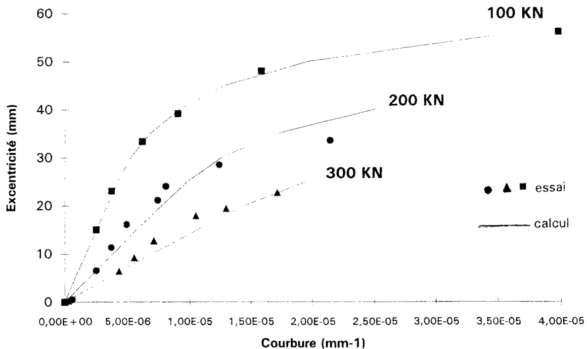
Figure 4.1- Courbes e(\frac{1}{r}, N) expérimentales et théoriques des assemblages de mortier M30.
