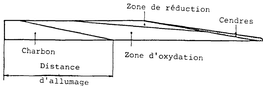
Figure 2-3 : Couche du charbon
