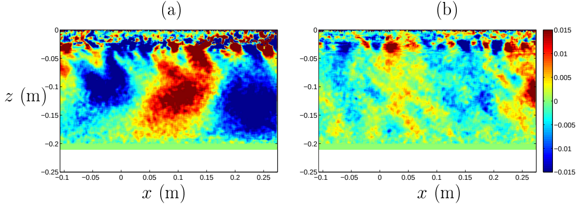
FIGURE 7.40 – Fr_h < 1 Champs instantanés \partial_x \rho à (a) t = 32 s et (b) t = 61 s, en \Delta N^2 (\text{rad s}^{-1})^2 .
