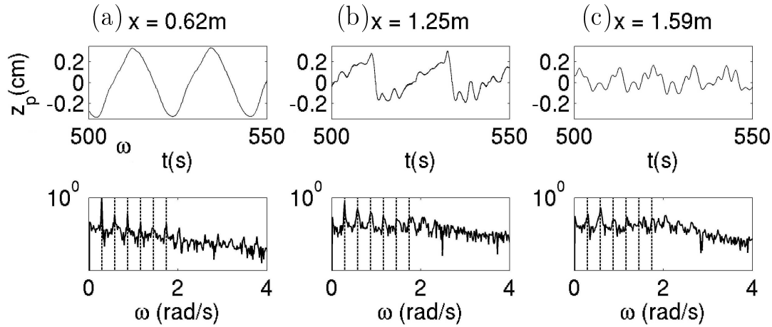
FIGURE 6.14 – Zooms sur trois sondes aux positions (a) x = 0.62\text{ m} , (b) x = 1.25\text{ m} et (c) x = 1.59\text{ m} , en régime établi, superposés aux spectres de Fourier associés à chacune des séries temporelles.
