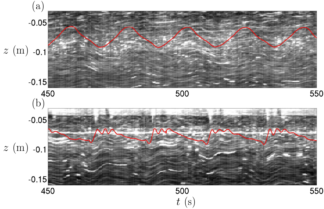
FIGURE 6.17 – Séries temporelles extraites en (a) x = 0.69 m et en (b) x = 1.20 m pour une expérience avec \omega = 0.29 rad s ^{-1} et \gamma = 0.17 . Les lignes rouges correspondent aux données issues des sondes à ultrasons (multipliées par un facteur 5), l'échelle de gris représentent l'intensité lumineuse associée aux images non-traitées de PIV, les zones blanches correspondent donc à des particules passant à la verticale de la position x fixée.
