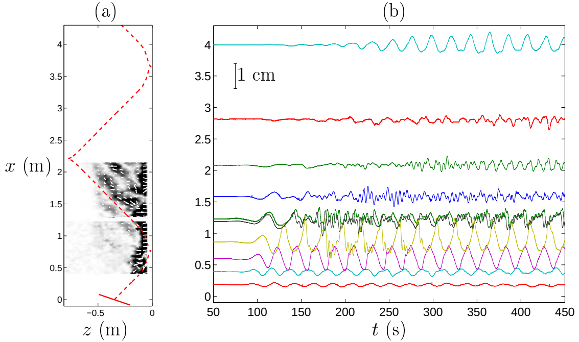
FIGURE 6.13 – (a) Vue tournée à 90^\circ d'un champ de vitesse instantané et (b) enregistrements des dix sondes à ultrasons pour une expérience avec \omega = 0.29 \text{ rad s}^{-1} et \gamma = 0.17 . Les pointillés rouges en (a) indiquent la propagation d'un rayon depuis le centre du générateur. Les enregistrements des sondes en (b) sont affichés au niveau de la position de la sonde selon l'axe ( Ox ), et l'amplitude réelle des oscillations est de l'ordre du centimètre comme indiqué par l'étalon.
