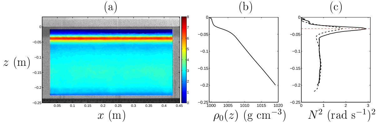
FIGURE 3.4 – (a) Image noir et blanc (acquise avec la caméra) sur laquelle est superposée le champ de déplacement vertical du motif (en pixel) obtenu à l’issu du calcul de l’algorithme CIVx avec comme image de référence un fluide homogène. (b) Profil de densité \rho_0(z) mesuré avec la sonde PME ©. (c) Comparaison des gradients verticaux de densité mesurés optiquement (ligne discontinue) et avec la sonde conductimétrique (ligne continue), le maximum du gradient mesuré optiquement étant repéré par les pointillés rouges.
