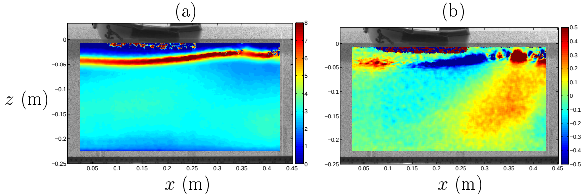
FIGURE 3.5 – Image noir et blanc acquise avec la caméra sur laquelle est superposée le champ de déplacement (a) vertical et (b) horizontal du motif (en pixel) obtenu à l’issu du calcul de l’algorithme CIVx avec comme image de référence un fluide homogène.
