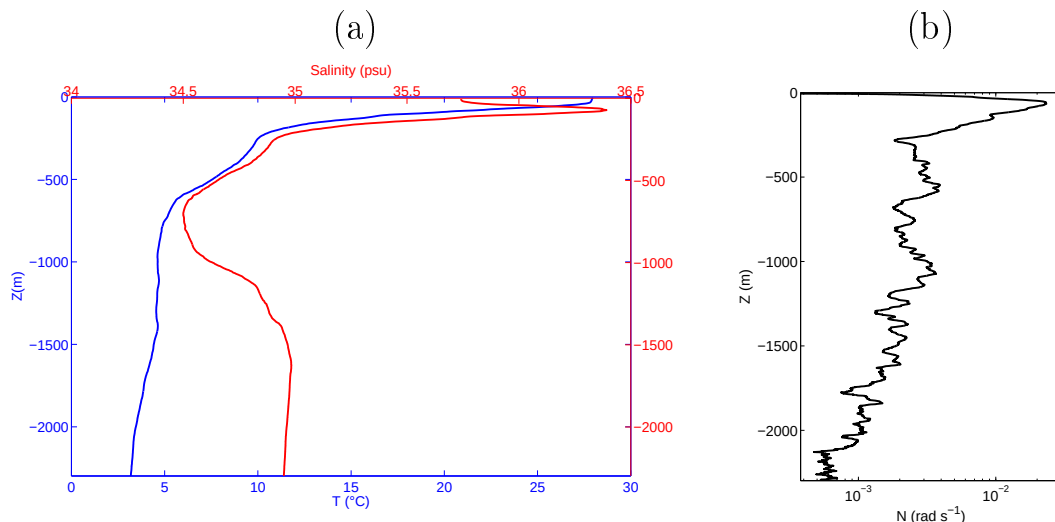
FIGURE 1.1 – (a) Profils de température et salinité et (b) profil N(z) associé, mesurés à bord du Pelagia (25/06/2009) dans le bassin Cêará ( 1^{\circ}23' \text{ N} , -38^{\circ}38' \text{ W} ) au large du Brésil.
