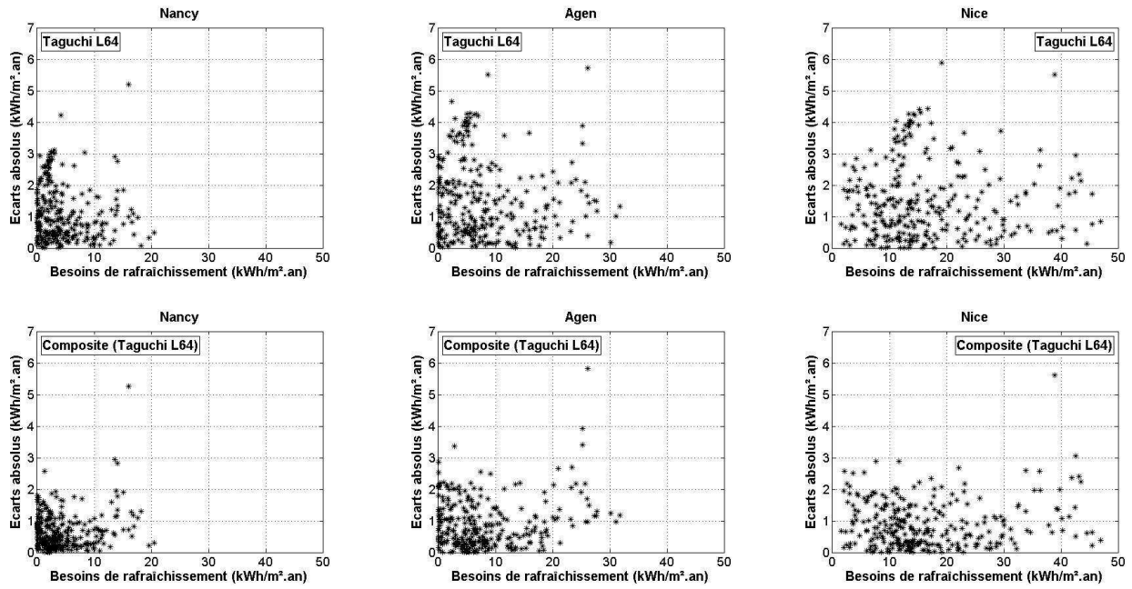
Figure 4.10 : Ecart absolu des besoins de rafraîchissement pour le plan composite L_{64}(2^{63}) les climats étudiés
