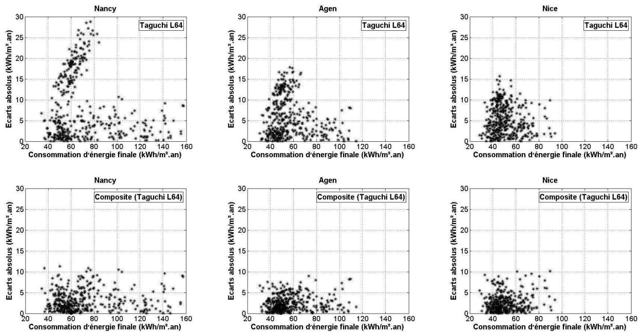
Figure 4.15 : Ecart absolu des besoins de la consommation d'énergie finale annuelle pour le plan composite L_{64}(2^{63}) pour les climats étudiés
