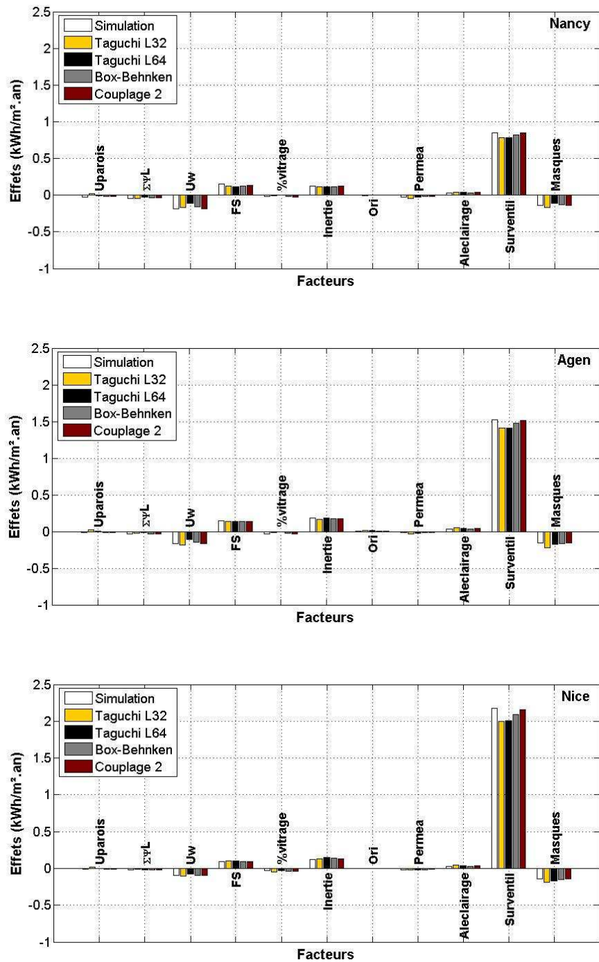
Figure 4.36 : Effets des facteurs sur la consommation d'énergie des auxiliaires de la surventilation mécanique nocturne pour Nancy, Agen et Nice
