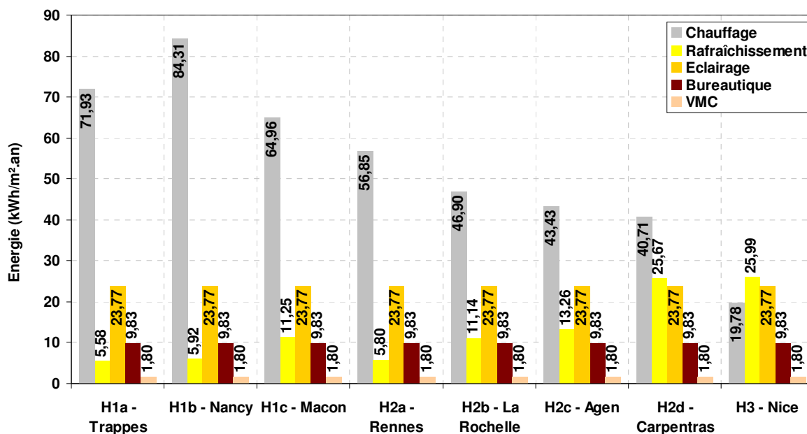
Figure 3.19 : Besoins et consommations énergétiques du bâtiment pour la configuration de référence pour les climats étudiés
