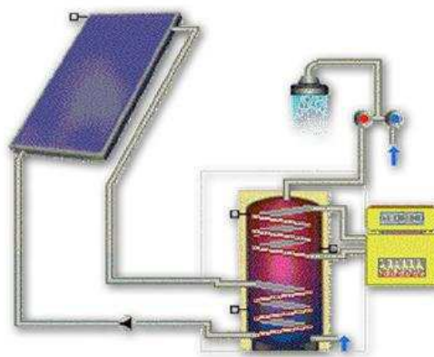
Figure 1.20 : Schéma de principe d'un CESA (Appoint chaudière) (ADEME, 2006a)
