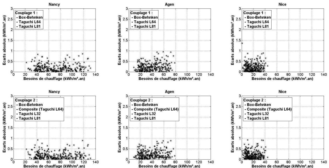
Figure 4.8 : Ecarts absolus des besoins de chauffage pour les plans d'expériences de couplage les climats étudiés
