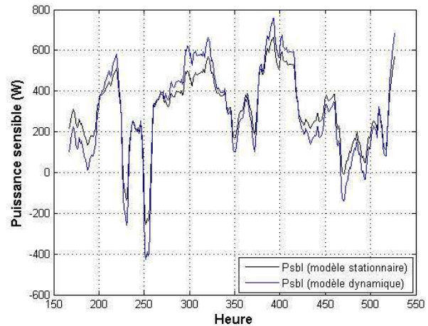
Figure 2.18 : Puissance sensible échangée entre l'air et le sol pour 10 jours
