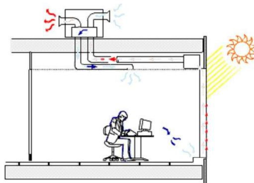
Figure 1.13 : Ventilation et récupération d'énergie pour une façade double peau (Permasteelisa, 2007)
