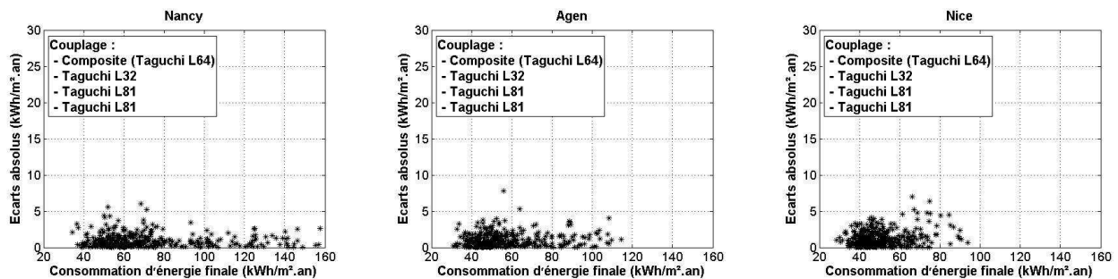
Figure 4.18 : Ecart absolu de la consommation d'énergie finale annuelle pour le plan de couplage pour les climats étudiés
