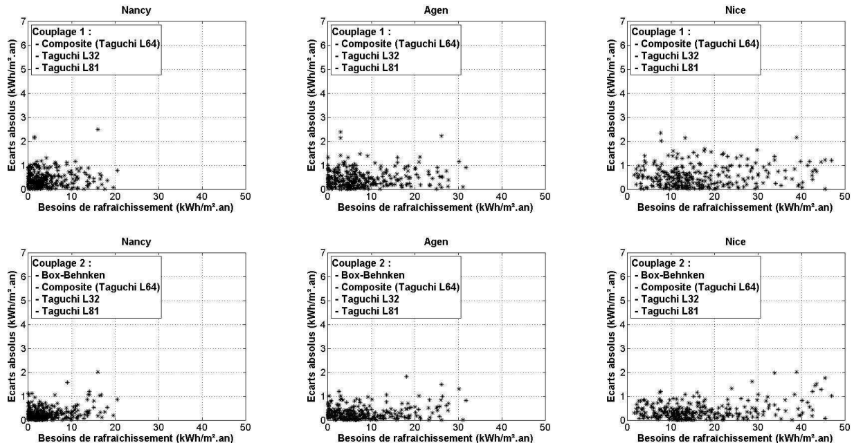
Figure 4.12 : Ecarts absolus des besoins de rafraîchissement pour les climats étudiés
