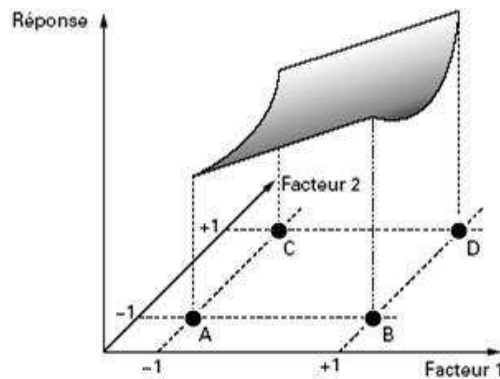
Figure 3.31 : Surface de réponse pour un plan à deux facteurs
