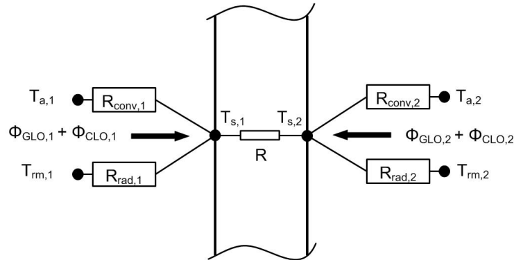
Figure 2.5 : Discrétisation nodale de la partie non protégée de la baie
