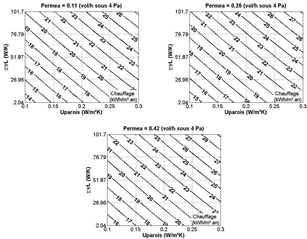
Figure 5.11 : Besoins de chauffage en fonction des facteurs U_{\text{parois}} , \Sigma\psi L et Permea avec une ventilation simple flux pour Agen
