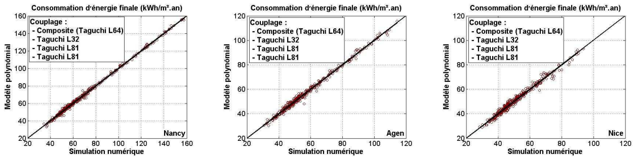
Figure 4.17 : Comparaison modèle polynômial / simulation numérique pour l'évaluation de la consommation d'énergie finale annuelle pour les trois climats étudiés
