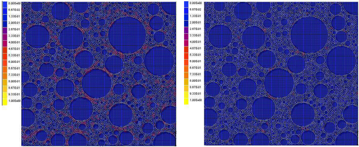
Figure 6.15 — Endommagement déviatorique localisé pour un chargement en traction de 20% de f_t à 200°C (gauche), et pour un chargement en traction de 40% de f_t à 140°C (droite).
