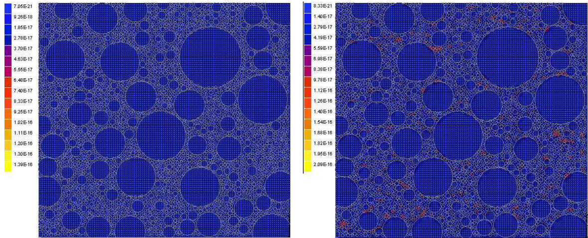
Figure 6.11 — Flux localisés sous un chargement en compression de 20% de f_c à 240^{\circ}C (gauche) et 260^{\circ}C (droite).
