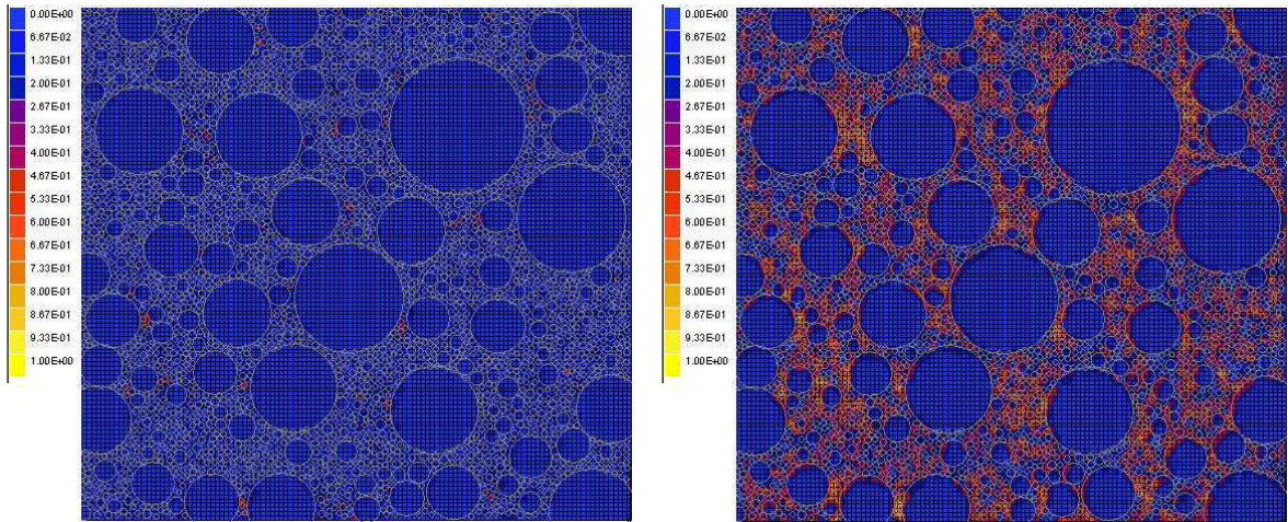
Figure 6.8 — Endommagement sphérique localisé sous un chargement en compression de 20% de f_c à 240°C (gauche) et 260°C (droite).
