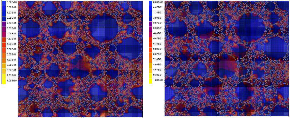
Figure 6.14 — Endommagement sphérique localisé pour un chargement en traction de 20% de f_t à 200°C (gauche), et pour un chargement en traction de 40% de f_t à 140°C (droite).
