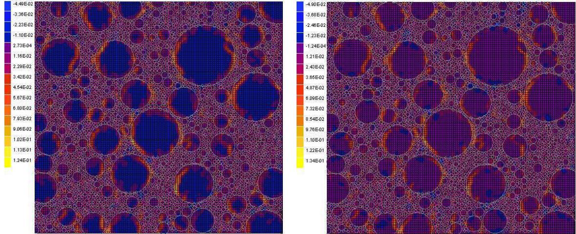
Figure 7.10 — Localisation des déformations dans le VER de béton à -22^{\circ}\text{C} durant le 1 er cycle de gel dégel (gauche) durant le 4 eme cycle (droite).
