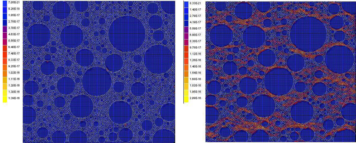
Figure 6.10 — Flux localisés pour un chargement nul à 240^{\circ}C (gauche) et 260^{\circ}C (droite).
