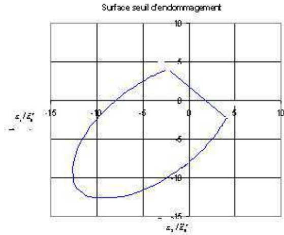
Figure 3.3 — Surface seuil d'endommagement
