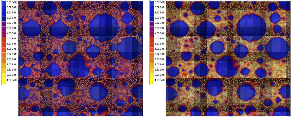
Figure 6.7 — Endommagement sphérique localisé sous un chargement en compression nul à 240°C (gauche) et 260°C (droite).
