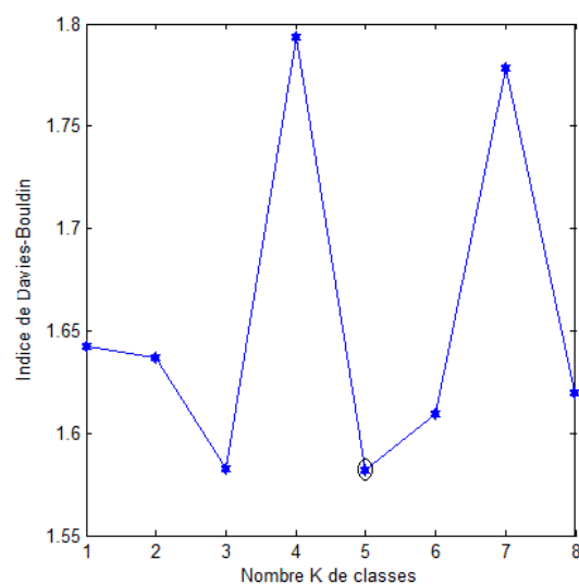
FIGURE 6.6 – Indice de Davies Bouldin pour K fixés
