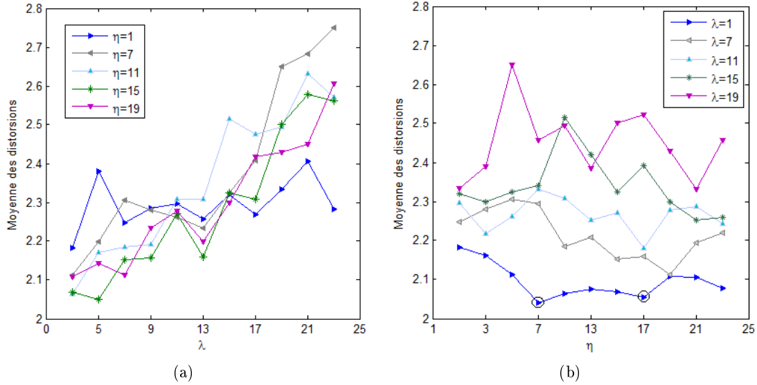
FIGURE 6.3 – Évolution de la moyenne de la mesure de distorsion pour les couples de paramètres \lambda et \eta
