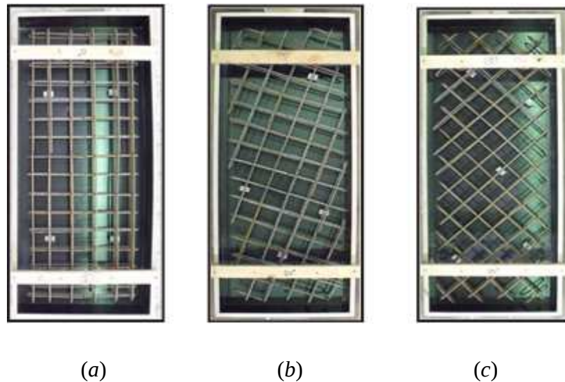
Figure 7.6. Coffrages et ferrillages des dalles pour des orientations du renforcement égales à : (a) 0^\circ , (b) 20^\circ , et (c) 45^\circ par rapport à l'axe longitudinal
