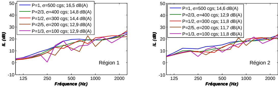
Figure 5.10. Perte par insertion en fonction de la fréquence d'un merlon acoustique de forme triangulaire pour différentes valeurs de P et \sigma . La valeur de la perte par insertion globale en dB(A) est donnée en légende pour chaque spectre.
