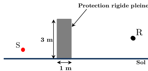
Figure 4.18. Deuxième protection rigide de référence d'une épaisseur de 1 m utilisée pour le calcul de l'efficacité de la protection innovante (écran+cristal sonique).
