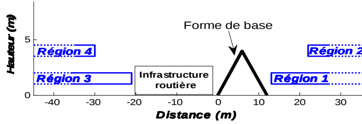
Figure 5.20. Configuration géométrique utilisée pour l'optimisation multiobjectif des merlons acoustiques : positions du merlon à optimiser, de l'infrastructure routière et des régions de récepteurs.
