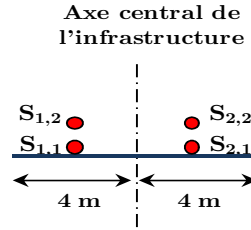
Figure 5.26. Positions des sources de roulement et de moteur pour une infrastructure d'une route à deux voies
