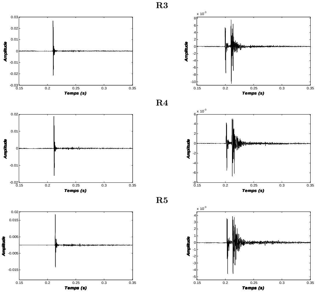
Figure B.2. Mesures en réflexion : réponses impulsionnelles obtenues pour la configuration en présence de l'écran en gabions (à gauche) et celles obtenues pour la configuration de référence (à droite) pour les cinq points récepteurs.
