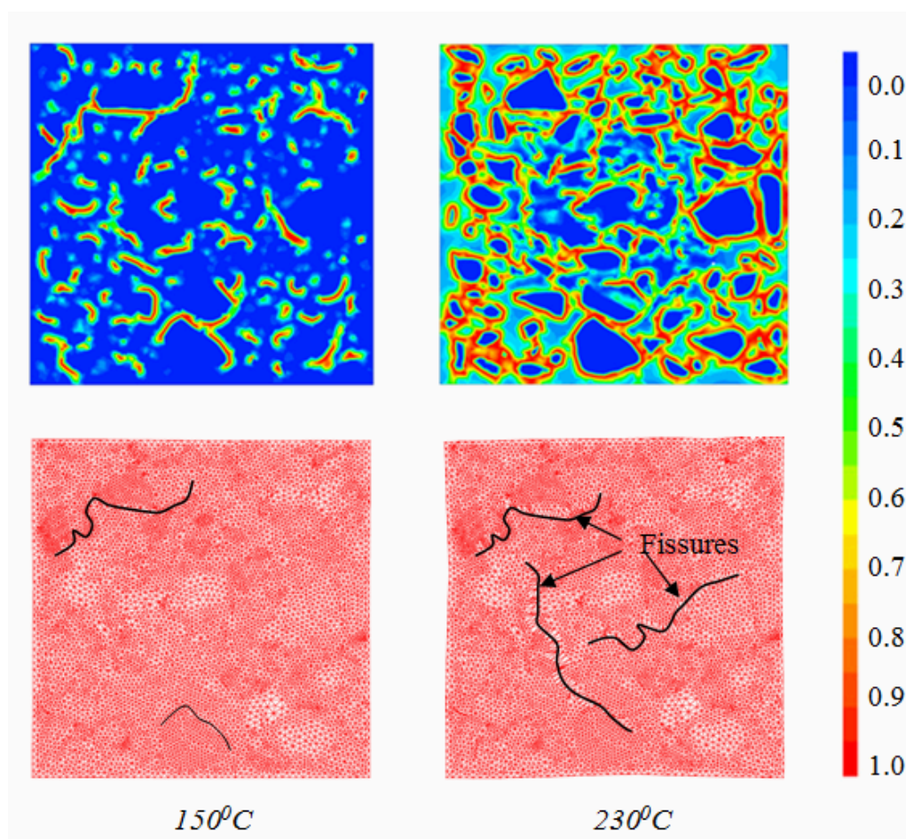
Figure 3.20 — Eprouvette 1— Réelle : Profil d'endommagement (en haut), déformée (en bas) - Chauffage 1^\circ\text{C}/\text{min} .
