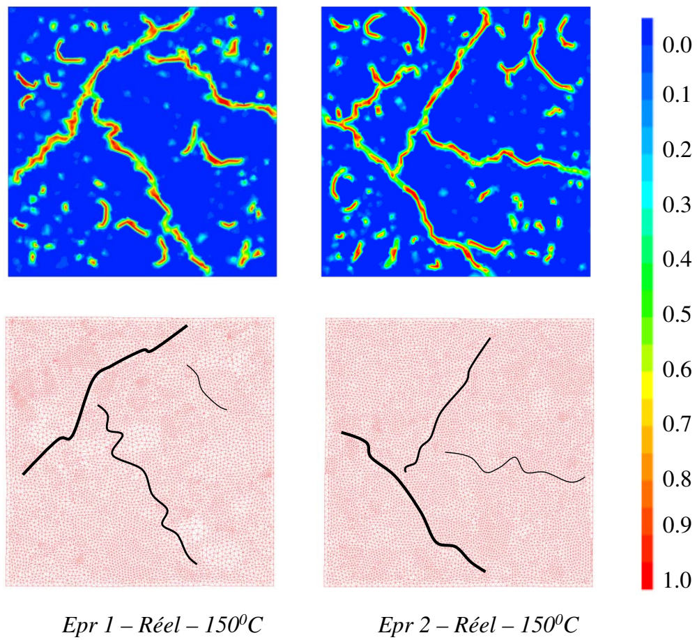
Figure 3.23 — Eprouvette 1 et 2 - Réelle : Profil d'endommagement (en haut), déformée (en bas) quand la température au bord est égale à 150^{\circ}\text{C} - Chauffage 5^{\circ}\text{C}/\text{min} .
