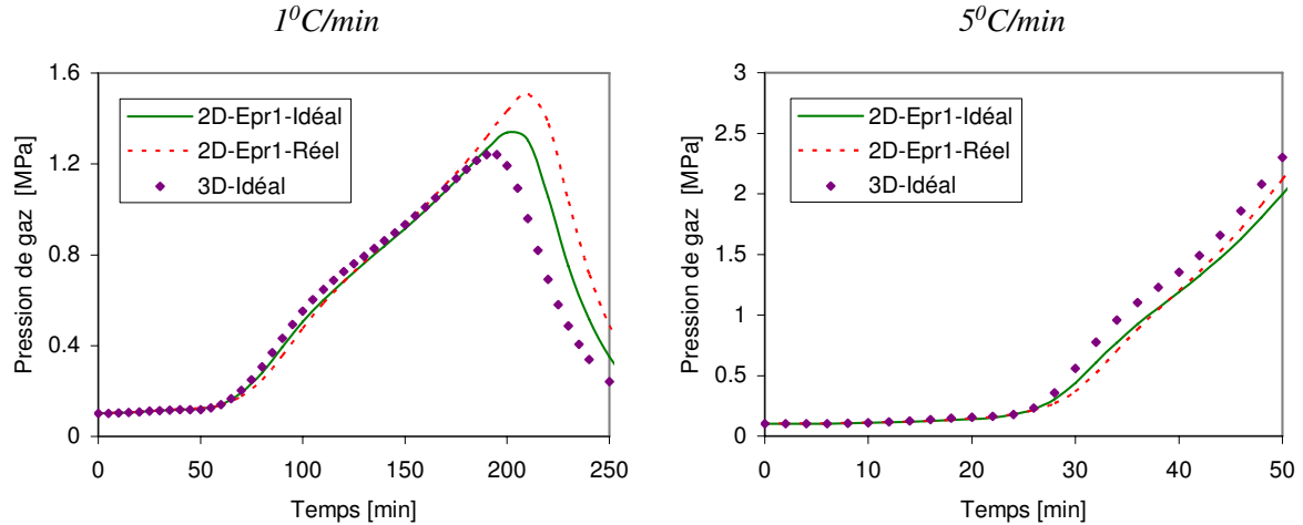
Figure 3.31 — Evolution dans le temps de la pression de gaz au centre du VER 3D ainsi que sa comparaison avec celle des VER 2D : Chauffage 1^\circ\text{C}/\text{min} (gauche) - Chauffage 5^\circ\text{C}/\text{min} (droite).
