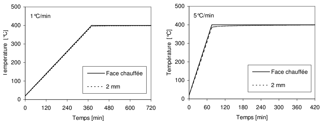
Figure 5.6 — Comparaison par simulation des évolutions de la température à la surface chauffée et à 2 mm : écart limité à 1.27% pour le chauffage à 1^{\circ}\text{C}/\text{min} et de 3.52% pour le chauffage à 5^{\circ}\text{C}/\text{min} .
