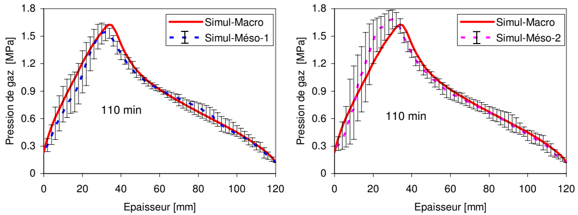
Figure 4.16 — Profil de la pression de gaz selon la profondeur    110 min de chauffage.
