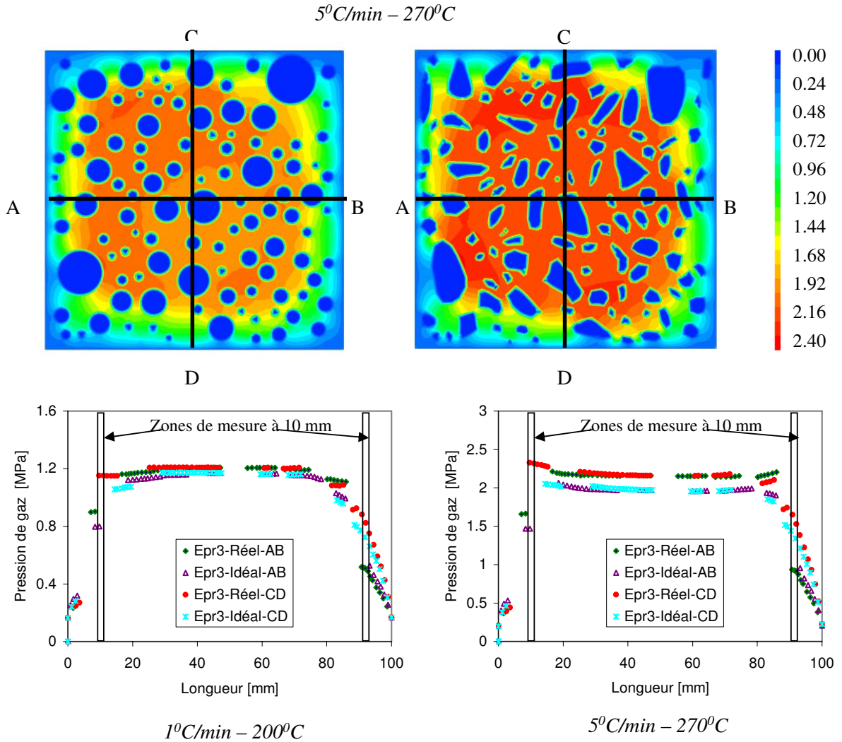
Figure 3.19 — Evolution de la pression de gaz selon l'épaisseur de l'éprouvette 3 réelle et idéalisée : Chauffage 1^\circ\text{C}/\text{min} (gauche) - Chauffage 5^\circ\text{C}/\text{min} (droite).
