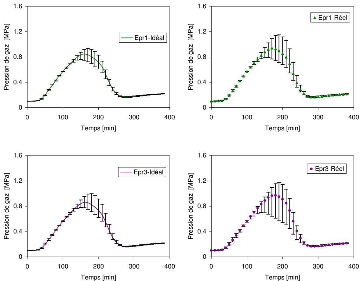
Figure 3.17 — Evolution dans le temps de la pression de gaz dans les zones de mesure à 10 mm du bord chauffé : Chauffage 1^\circ\text{C}/\text{min} .
