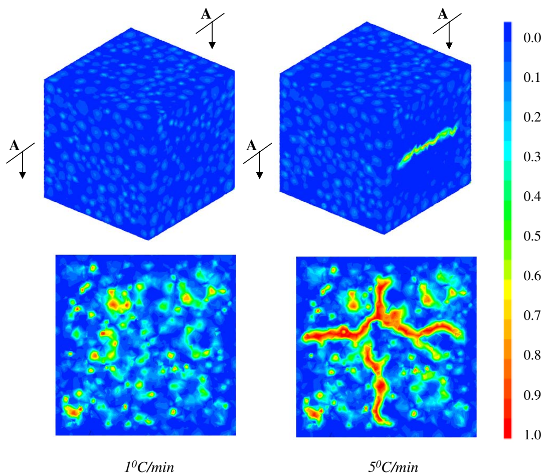
Figure 3.35 — Iso-valeurs de l'endommagement du VER 3D et d'une coupe courante dans le plan de chauffage quand la température au bord est égale à 150^\circ\text{C} : Chauffage 1^\circ\text{C}/\text{min} (gauche) - Chauffage 5^\circ\text{C}/\text{min} (droite).
