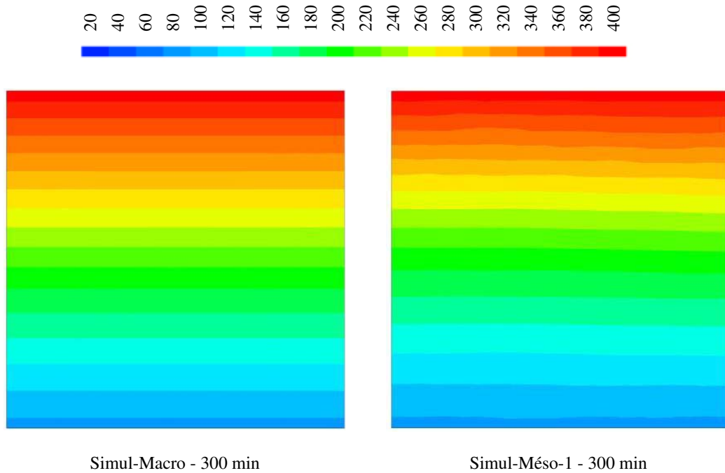
Figure 4.8 — Iso-valeurs de la température [ ^{\circ}\text{C} ] après 300 min de chauffage obtenues par la simulation macroscopique et mésoscopique.
