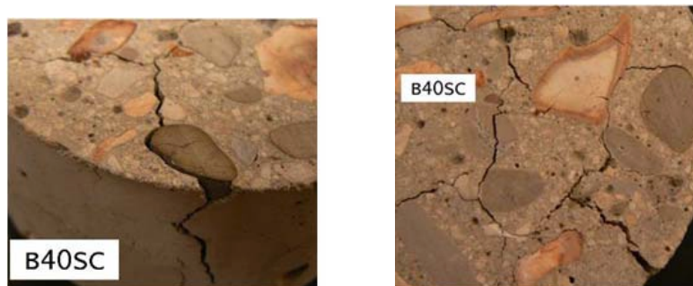
Figure 3.24 — Observations visuelles de l'éprouvette B40SC à 400^{\circ}\text{C} [96].
