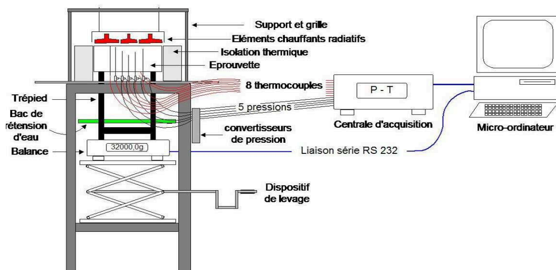
Figure 5.1 — Vue d'ensemble du dispositif "PTM" de caractérisation thermohydraulique des bétons.
