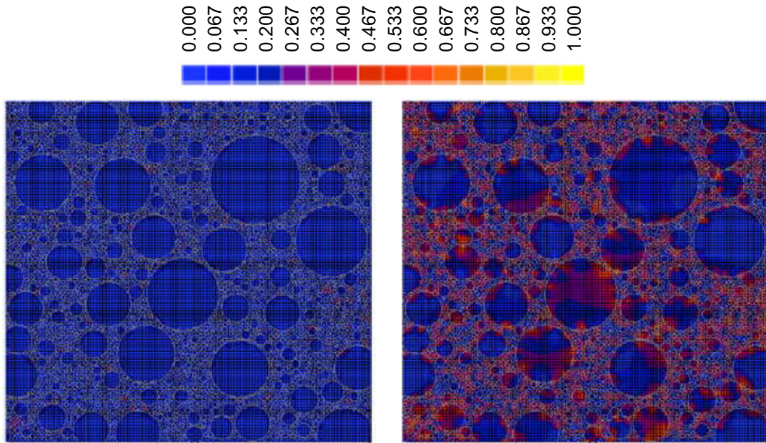
Figure 1.36 — Localisation de l'endommagement dans le béton à 100^{\circ}\text{C} et 140^{\circ}\text{C} [55].
