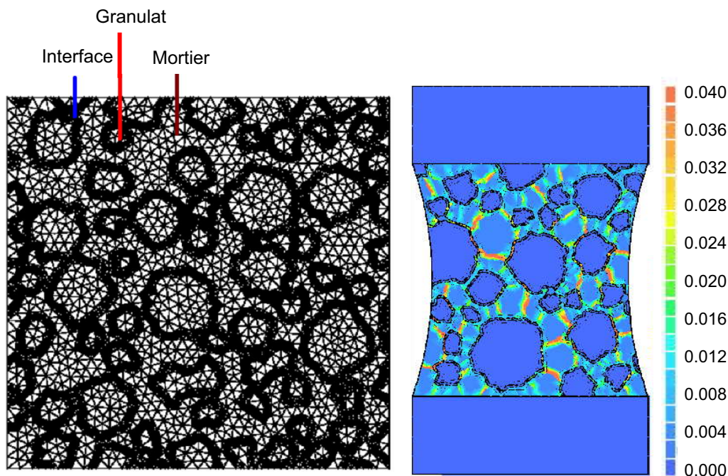
Figure 1.37 — A gauche, exemple de génération des phases (Modèle Delft TNO). A droite, déformation plastique dans la direction principale (matériau chauffé à 400^{\circ}\text{C} ) [25].
