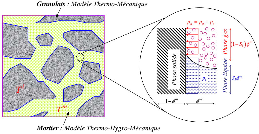
Figure 2.2 — Modèles de comportement des constituants du béton.
