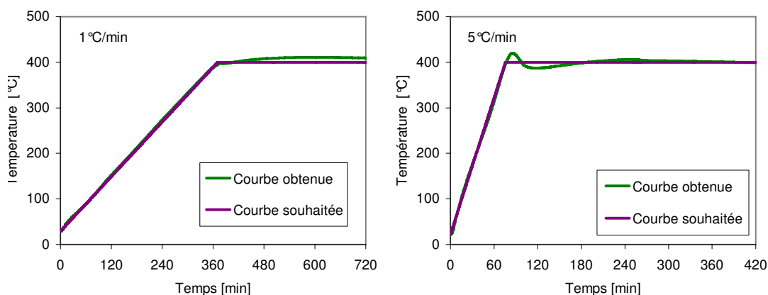
Figure 5.7 — Profil des températures souhaitée et obtenue à 2 mm de la surface chauffée pour le chauffage à 1^{\circ}\text{C}/\text{min} (gauche) et à 5^{\circ}\text{C}/\text{min} (droite).
