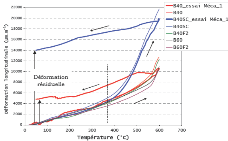
Figure 1.24 — Déformation thermique libre des bétons de l'étude de Mindeguia [96]. La phase de refroidissement a été enregistrée pour le B40 et le B40SC.
