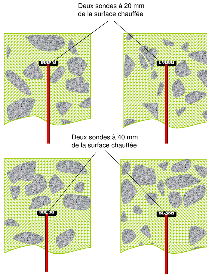
Figure 5.13 — Découpe de l'éprouvette B40C 20 \times 40 à des positions des sondes.
