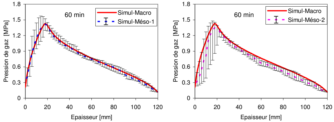
Figure 4.15 — Profil de la pression de gaz selon la profondeur    60 min de chauffage.
