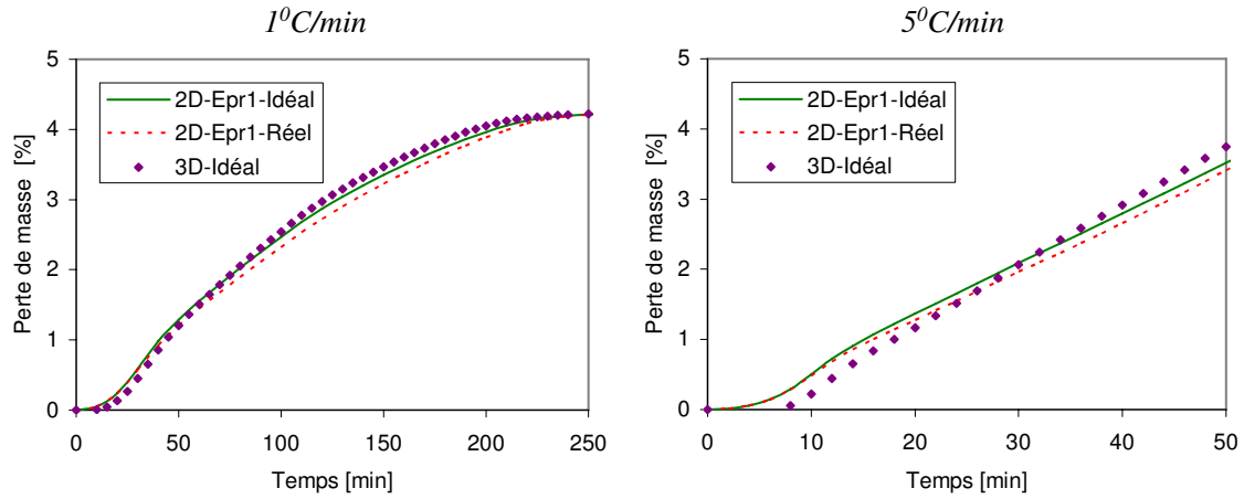
Figure 3.28 — Comparaison des évolutions de la perte de masse globale du VER 3D avec deux VER 2D de l'éprouvette 1 réelle et idéalisée : Chauffage 1^{\circ}\text{C/min} (gauche) - Chauffage 5^{\circ}\text{C/min} (droite).
