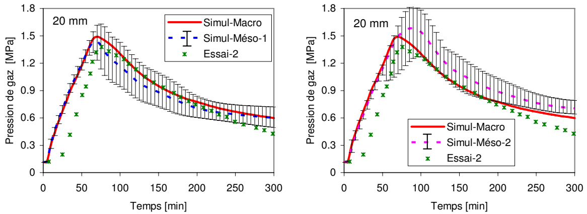
Figure 4.18 —  volution de la pression de gaz en fonction du temps   20 mm de la surface chauff e.
