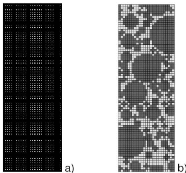
Figure 1.40 — Maillages aux éléments finis : a) Béton considéré homogène, b) Béton considéré hétérogène [32].
