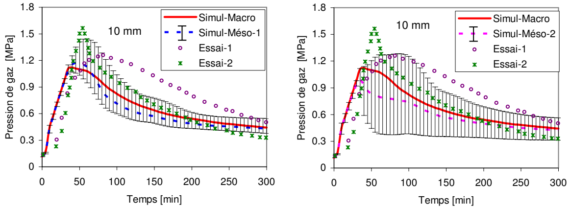
Figure 4.17 —  volution de la pression de gaz en fonction du temps   10 mm de la surface chauff e.
