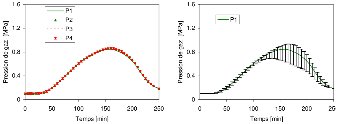
Figure 3.33 — Evolution dans le temps de la pression de gaz à 10 mm par rapport à la surface chauffée du VER pour le chauffage 1^{\circ}\text{C}/\text{min} : valeurs moyennes des quatres prismes (gauche) - Evolution dans le prisme P1 (droite).
