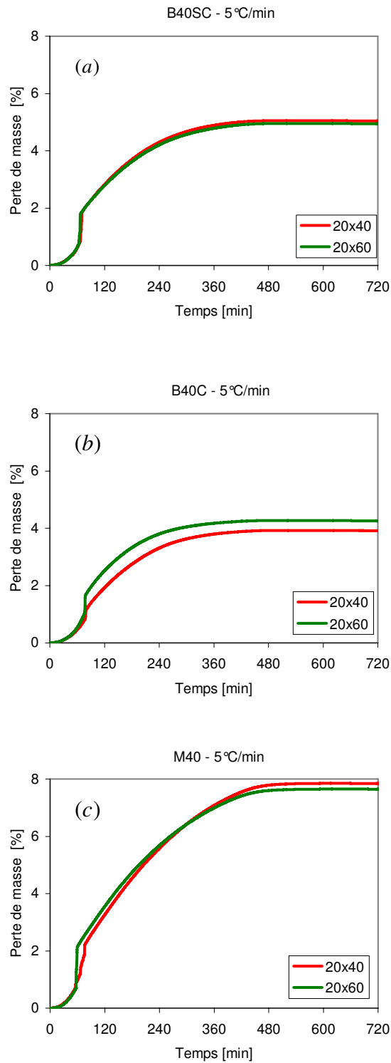
Figure 5.16 — Evolutions de la perte de masse en fonction du temps pour le chauffage à 5^{\circ}\text{C}/\text{min} : (a) - Pour le béton B40SC, (b) - Pour le béton B40C et (c) - Pour le mortier M40.
