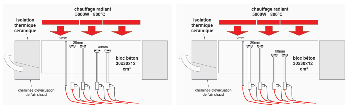
Figure 5.2 — Disposition des sondes dans l'éprouvette.
