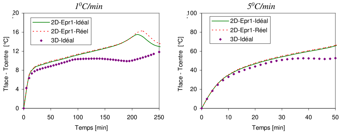
Figure 3.29 — Evolution dans le temps de la différence entre la température à la surface chauffée et celle au centre du VER 3D ainsi que sa comparaison avec les VER 2D : Chauffage 1^{\circ}\text{C/min} (gauche) - Chauffage 5^{\circ}\text{C/min} (droite).
