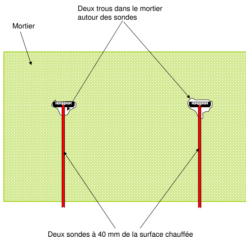
Figure 5.12 — Découpe de l'éprouvette M40 20 × 40 à la position des deux sondes à 40 mm.
