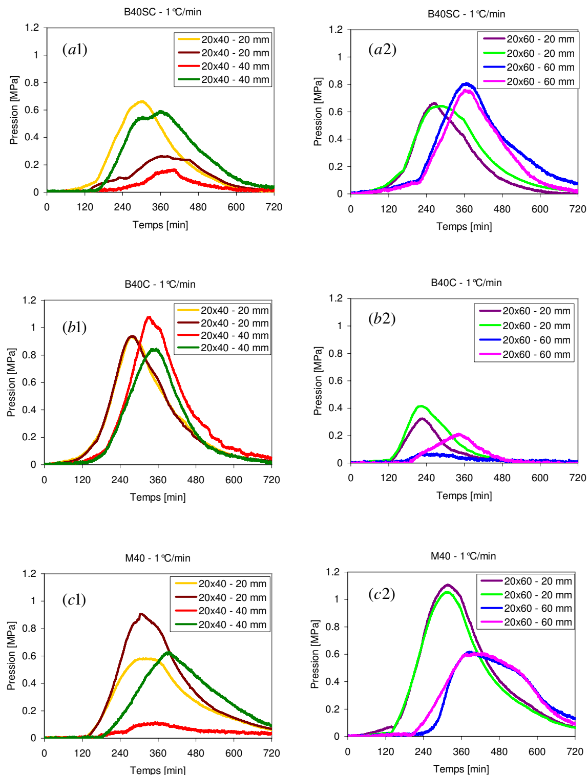
Figure 5.11 — Evolutions de la pression en fonction du temps pour le chauffage à 1°C/min : (a1) - Eprouvette B40SC avec les sondes à 20 mm et 40 mm, (a2) - Eprouvette B40SC avec les sondes à 20 mm et 60 mm, (b1) - Eprouvette B40C avec les sondes à 20 mm et 40 mm, (b2) - Eprouvette B40C avec les sondes à 20 mm et 60 mm, (c1) - Eprouvette M40 avec les sondes à 20 mm et 40 mm, (c2) - Eprouvette M40 avec les sondes à 20 mm et 60 mm.
