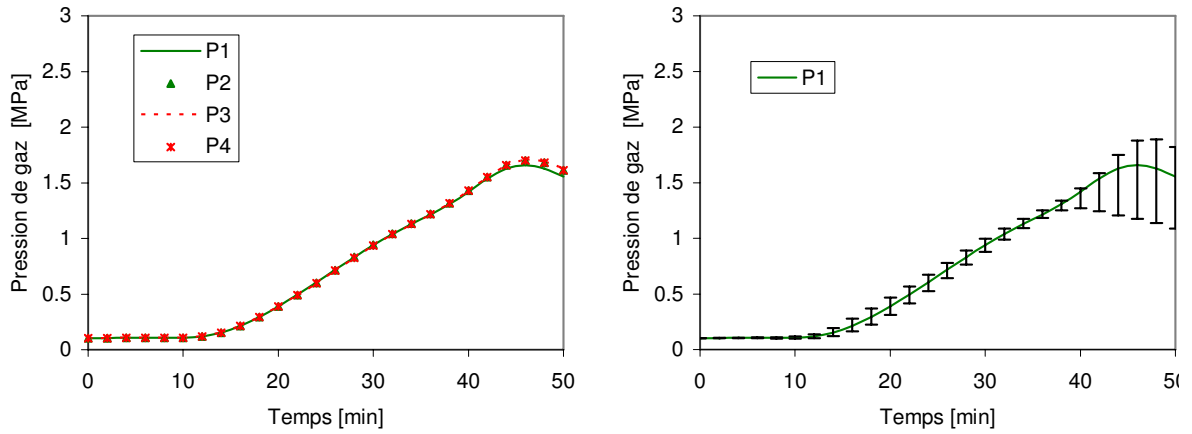
Figure 3.34 — Evolution dans le temps de la pression de gaz à 10 mm par rapport à la surface chauffée du VER pour le chauffage 5^{\circ}\text{C}/\text{min} : valeurs moyennes des quatres prismes (gauche) - Evolution dans le prisme P1 (droite).
