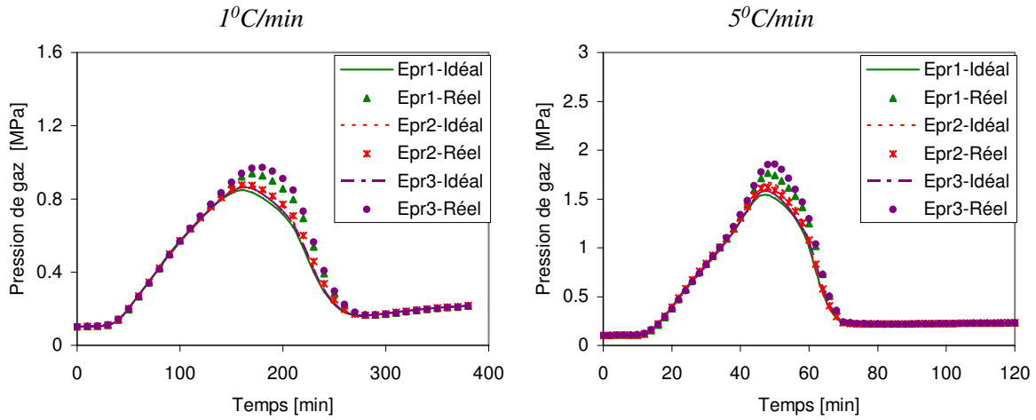
Figure 3.16 — Evolution dans le temps de la pression de gaz moyenne à 10 mm par rapport au bord chauffé : Chauffage 1^{\circ}\text{C}/\text{min} (gauche) - Chauffage 5^{\circ}\text{C}/\text{min} (droite).
