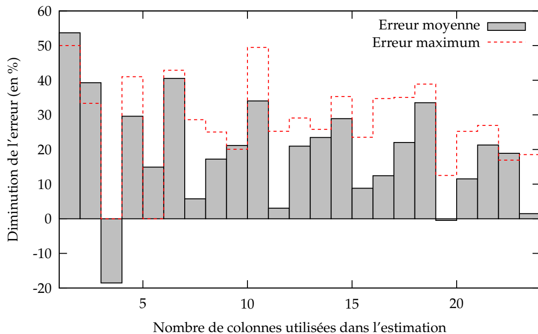
Figure 1.15 Diminution de l'erreur en % en fonction du nombre de colonnes implantées dans l'estimation, en utilisant un opérateur hybride par rapport à un tri des produits partiels seul, pour un argument de 16 bits élevé à la puissance 4
