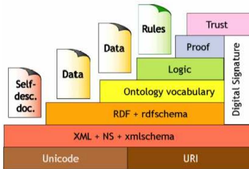
Figure 3 Les couches du Web Sémantique
