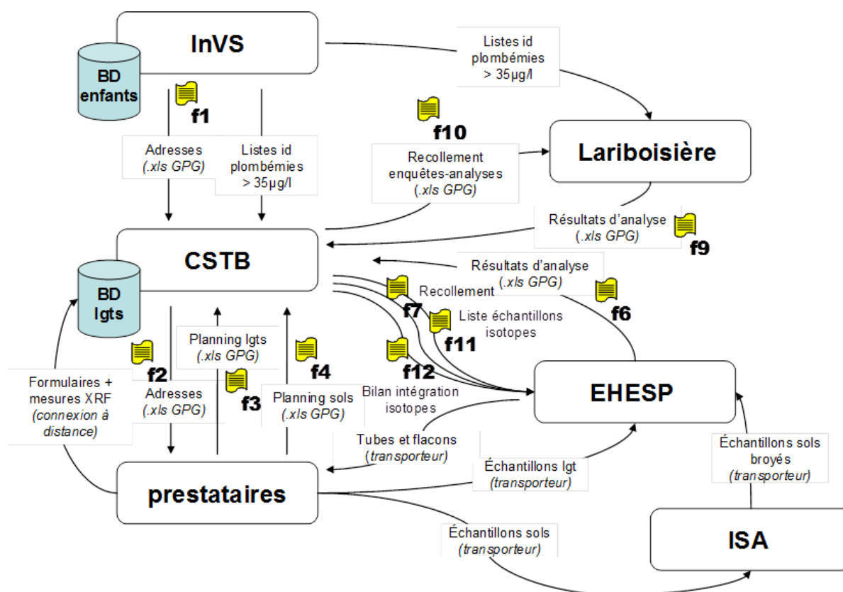
FIGURE 17 – Flux des données entre les différents partenaires de l'enquête Plomb-Habitat
