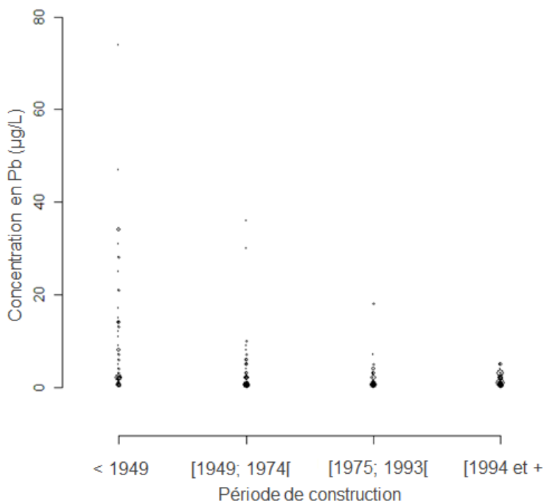
FIGURE 24 – Concentrations en plomb dans l’eau du robinet selon la période de construction.
