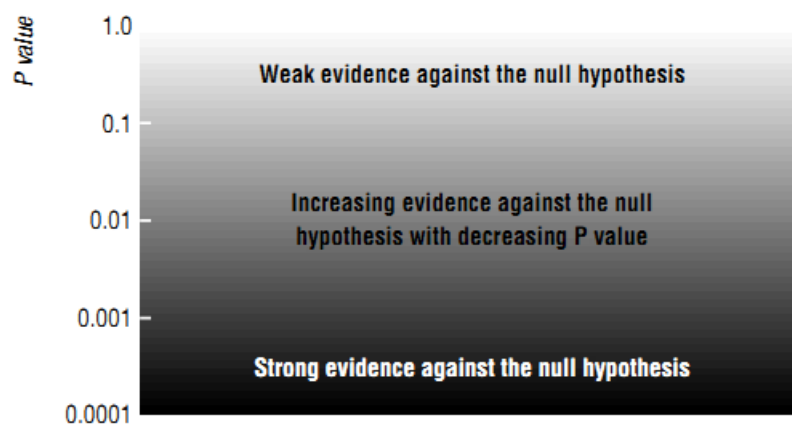
FIGURE 33 – Suggestion d'interprétation de la p-value proposée dans l'article [Sterne & Davey Smith, 2001].
