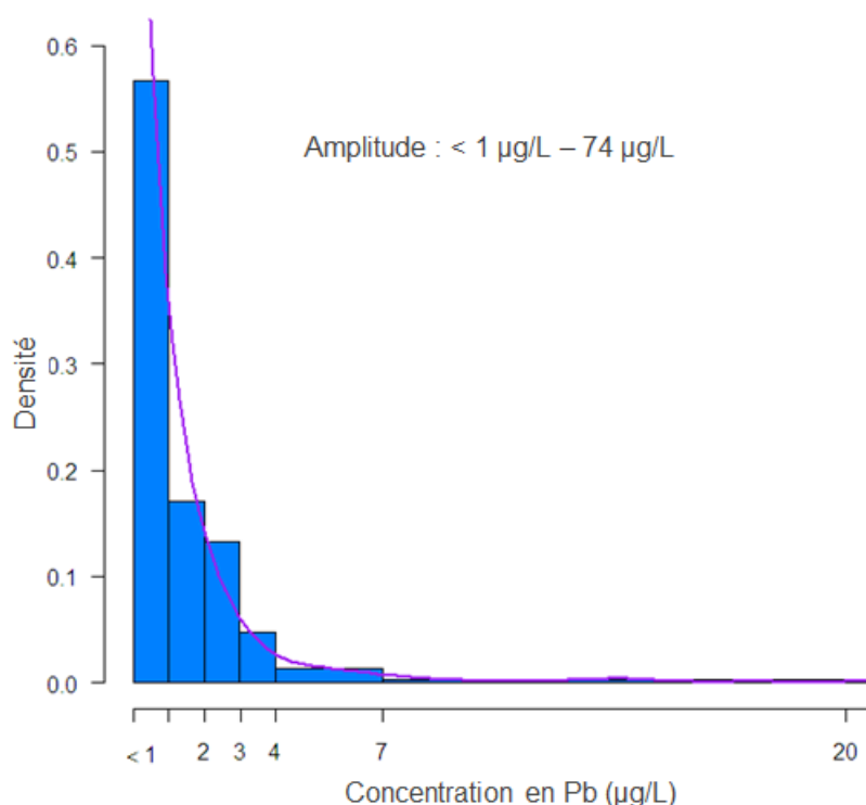
FIGURE 23 – Distribution des concentrations en plomb dans l’eau du robinet.
