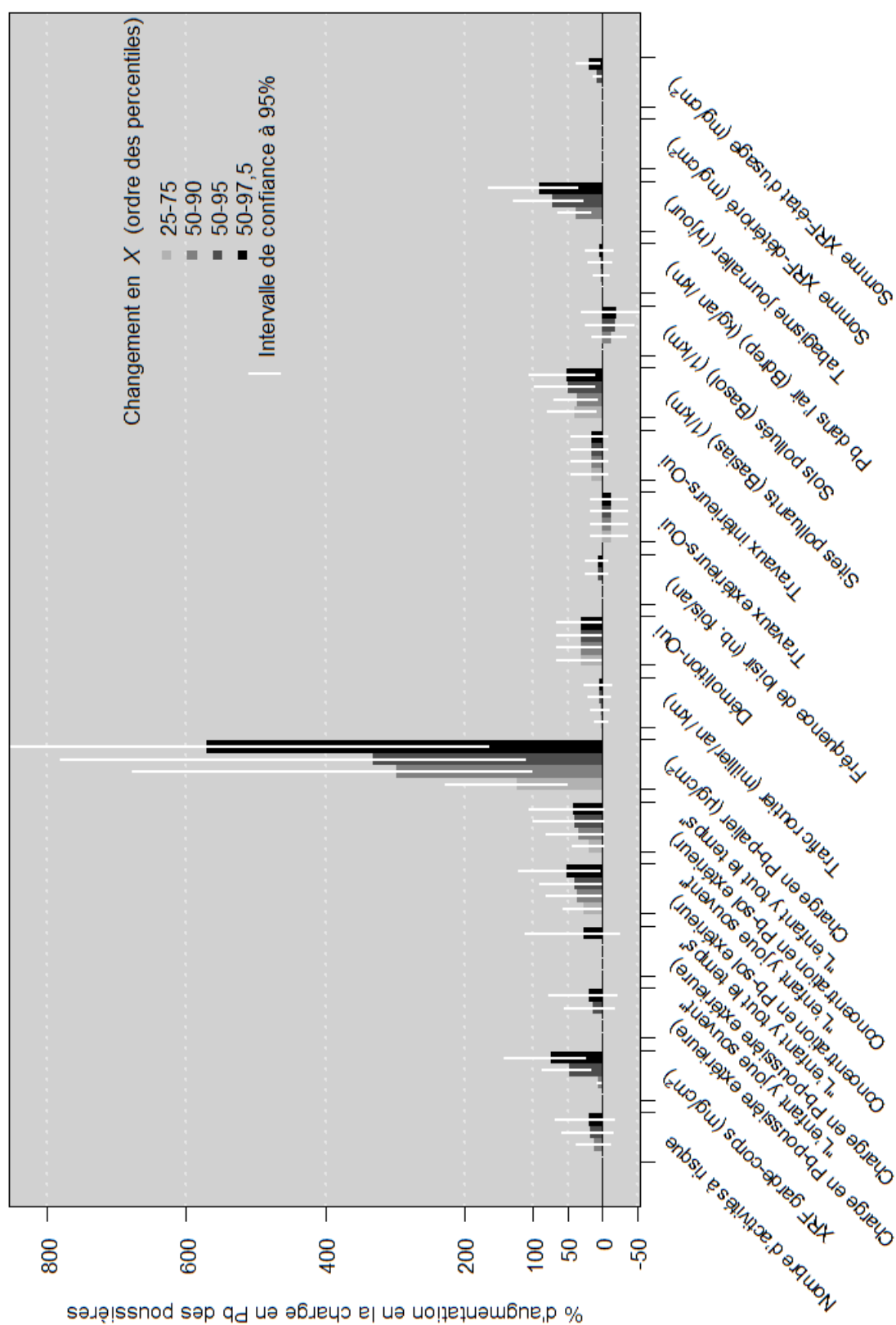
FIGURE 35 – Contribution de chaque source X exprimée en % d'augmentation en la charge en plomb des poussières ( \mu\text{g}/\text{m}^2 ), calculée à partir des données imputées. Plomb total
