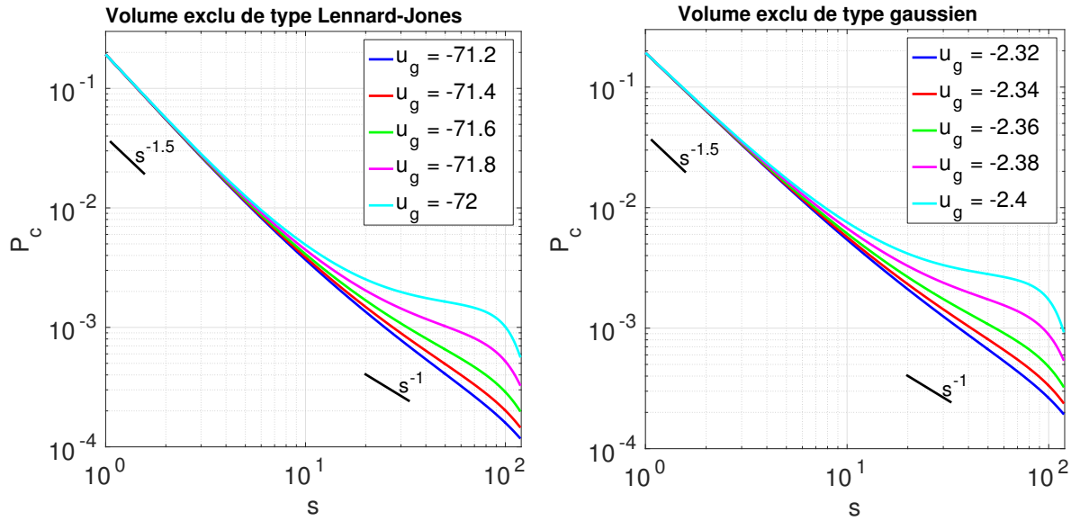
FIGURE 4.2.5 – Détermination du champ générique U_g par optimisation d'un paramètre u_g . Les deux graphes (à gauche si le volume exclu est modélisé par un potentiel de type Lennard-Jones, à droite s'il l'est par un potentiel gaussien) présentent la probabilité de contact, P_c , en fonction de la distance génomique s en bin pour un homopolymère auto-évitant de 120 monomères auquel on ajoute un champ de crumpling uniforme d'intensité en k_B T donnée en légende. Dans les deux cas, la pente de la droite en échelle log dépend de l'intensité du champ générique ajouté. La pente est globalement la plus proche de -1 dans le cas de la courbe verte, correspondant à u_g = -71.6k_B T à gauche et u_g = -2.36k_B T à droite.
