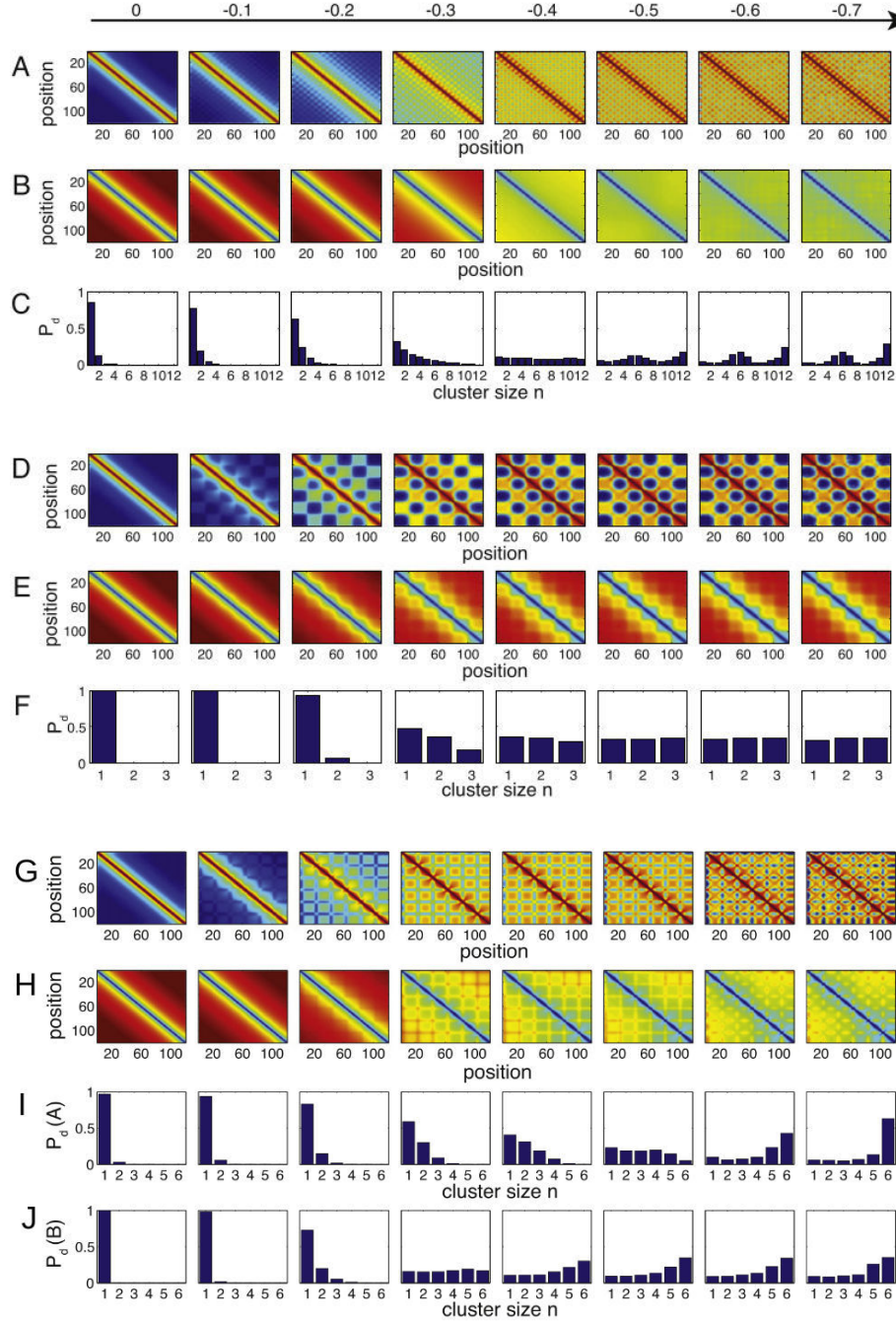
FIGURE 4.3.4 – Propriétés structurales d'un copolymère en fonction du paramètre u_e et en fonction de la taille de ses domaines. Les lignes A, B et C présentent le copolymère (A_5B_5)_{12} , les lignes D, E et F s'intéressent à (A_{20}B_{20})_3 et enfin les lignes G, H, I et J correspondent au copolymère asymétrique (A_5B_{15})_6 . (A,D,G) Matrice de contact avec la même échelle de couleur que figure 4.3.3(A). (B,E,H) Matrice des distances quadratiques moyennes avec la même échelle de couleur que figure 4.3.3(C). (C,F,I,J) Probabilité P_d(n) pour un domaine dans un certain état épigénomique (A ou B) d'appartenir à un groupe composé de n domaines du même état.
