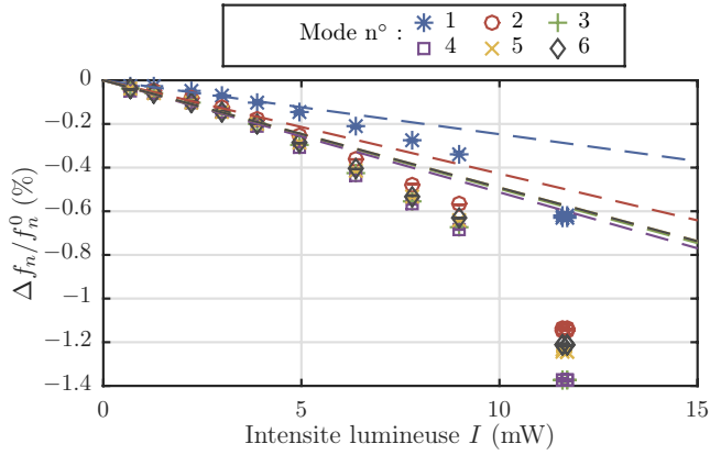
FIGURE 3.1 – Micro-levier C100 : Décalage relatif en fréquence \Delta f_n/f_n^0 en fonction de l'intensité lumineuse I dans le vide ( P = 4 \text{ Pa} ). Les courbes en pointillés représentent les régressions linéaires à faible intensité lumineuse ( I < 7 \text{ mW} ). Il existe un aspect non linéaire pour des intensités lumineuses supérieures à 5 \text{ mW} .
