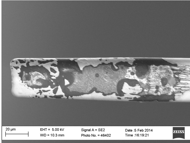
FIGURE 3.14 – Image par microscopie électronique à balayage d'un levier avec revêtement en or après chauffage. On voit nettement ici le revêtement en or qui a fondu laissant apparaître le silicium et la couche d'accroche en chrome.
