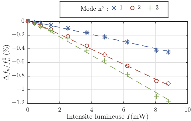
FIGURE 3.2 – Micro-levier C30 : Décalage fréquentiel relatif \Delta f_n/f_n en fonction de l'intensité lumineuse I dans le vide ( P = 10 \text{ Pa} ). Les courbes en pointillés représentent les régressions linéaires.
