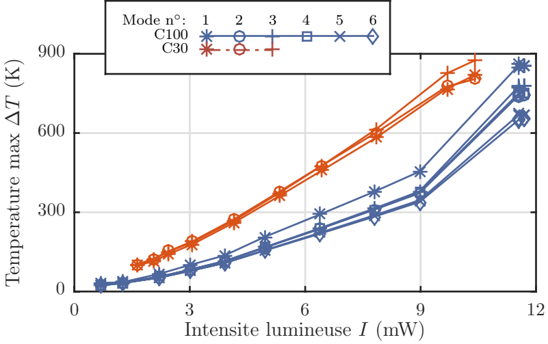
FIGURE 3.4 — Température à l'extrémité libre du levier estimée grâce au décalage fréquentiel dans le vide, en supposant un profil de température linéaire. Cette approximation tend à devenir fausse pour de fortes intensités lumineuses, zone pour laquelle les non-linéarités sont importantes et l'estimation de \Delta T des différents modes est plus dispersée. Nous remarquons cependant qu'un fort gradient de température est déjà présent pour de faibles intensités lumineuses (quelques mW)
