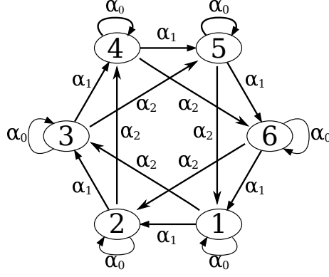
FIGURE 7.1 – Grphe de transition. Exemple pour d = 6 et \mathcal{E} = \alpha_0 \text{Id} + \alpha_1 J_d + \alpha_2 J_d^2 ( \alpha_0 + \alpha_1 + \alpha_2 = 1 ) où J_d est une matrice de saut circulaire (cf. Eq. (III.53))
