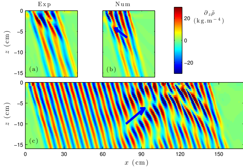
FIGURE 5.4 – Gradient de densité vertical pour les expériences III et IV ( \omega_0/N = 0.74 , \ell_0 = 66 \text{ m}^{-1} , \psi_0/\nu = 33 ). (a) Champ expérimental avec W = 3\lambda_0 . (b) Champ numérique avec W = 3\lambda_0 . (c) Champ numérique avec W = 20\lambda_0 . Les deux flèches bleues représentent la direction de la vitesse de groupe de l'onde secondaire la plus visible.
