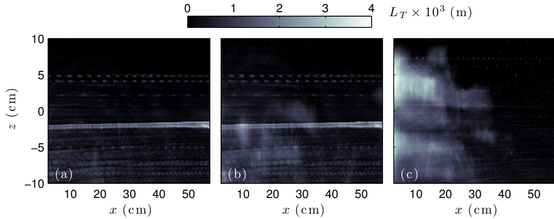
FIGURE 7.14 – (a) Évolution spatiale de la moyenne temporelle de l'échelle de Thorpe pour un mode-1 stable. (b) Évolution spatiale de la moyenne temporelle de l'échelle de Thorpe pour une expérience présentant de la PSI mais sans mélange significatif. (c) Évolution spatiale de la moyenne temporelle de l'échelle de Thorpe pour une expérience présentant de la PSI et du mélange.
