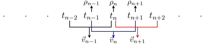
FIGURE 7.3 – Calcul des champs de vitesse et de densité dans le cas où les deux caméras ont la même fréquence d'acquisition.
