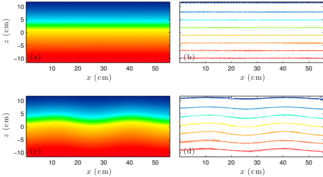
FIGURE 6.8 – (a) Image corrigée de la stratification initiale. (b) Représentation de quelques isopycnas de l'image (a). (c) Image corrigée à un instant t pendant la propagation d'un mode-1. (d) Représentation de quelques isopycnas de l'image (c).
