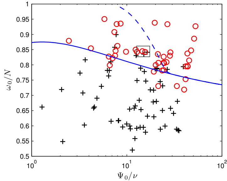
FIGURE 5.1 – Représentation des expériences effectuées en fonction de la pulsation de l'onde mère \omega_0 , normalisée par la pulsation de flottabilité N , et de l'amplitude de la fonction courant de l'onde mère \Psi_0 , normalisée par la viscosité \nu . La ligne continue représente pour chaque amplitude la transition entre le cas où les ondes secondaires sont sélectionnées sur la partie extérieure de l'espace des solutions et le cas où les ondes secondaires sont sélectionnées sur la partie centrale. La ligne en pointillé représente la pulsation seuil en dessous de laquelle le transfert d'énergie vers les grandes échelles est possible. Les cercles rouges représentent les expériences présentant de la PSI, les croix noirs des expériences stables.
