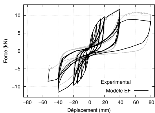
(c) OSB9 E5 C1
