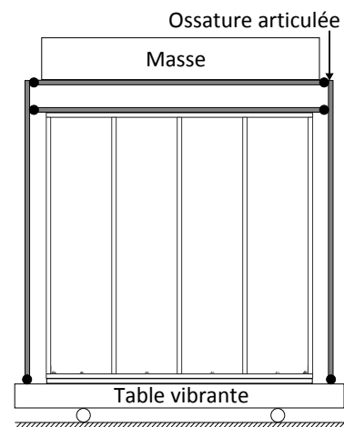
Figure 4.5: Essais dynamiques avec ossature articulée
