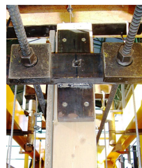
(c) Entretoise opposée
