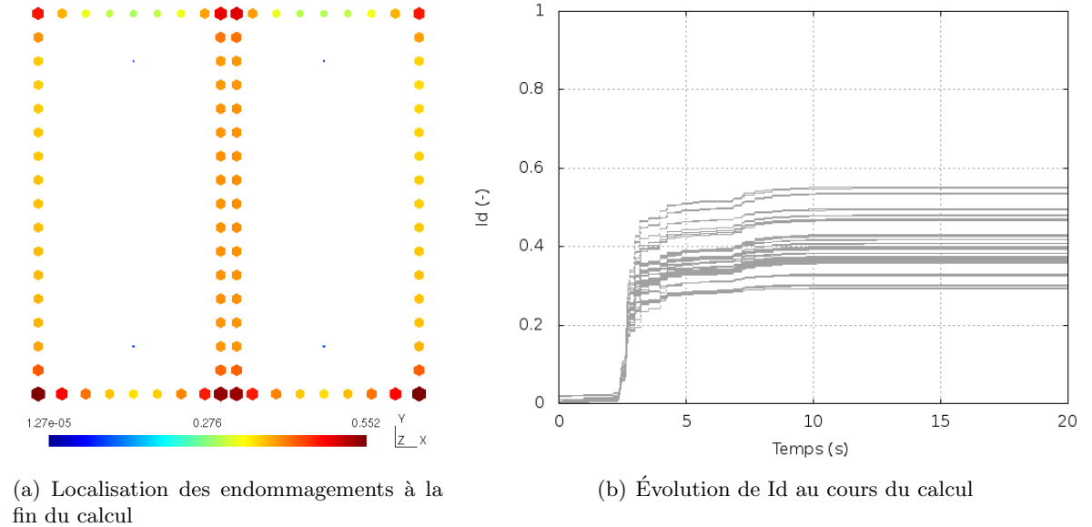
Figure 6.22: Localisation de l'endommagement dans un mur
