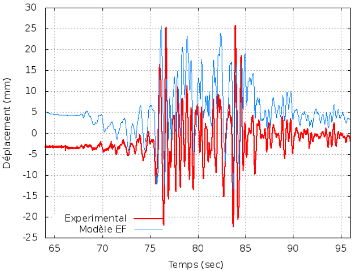
OSB12 AH 1500kg Guadeloupe Modifié #3 0,33 g
