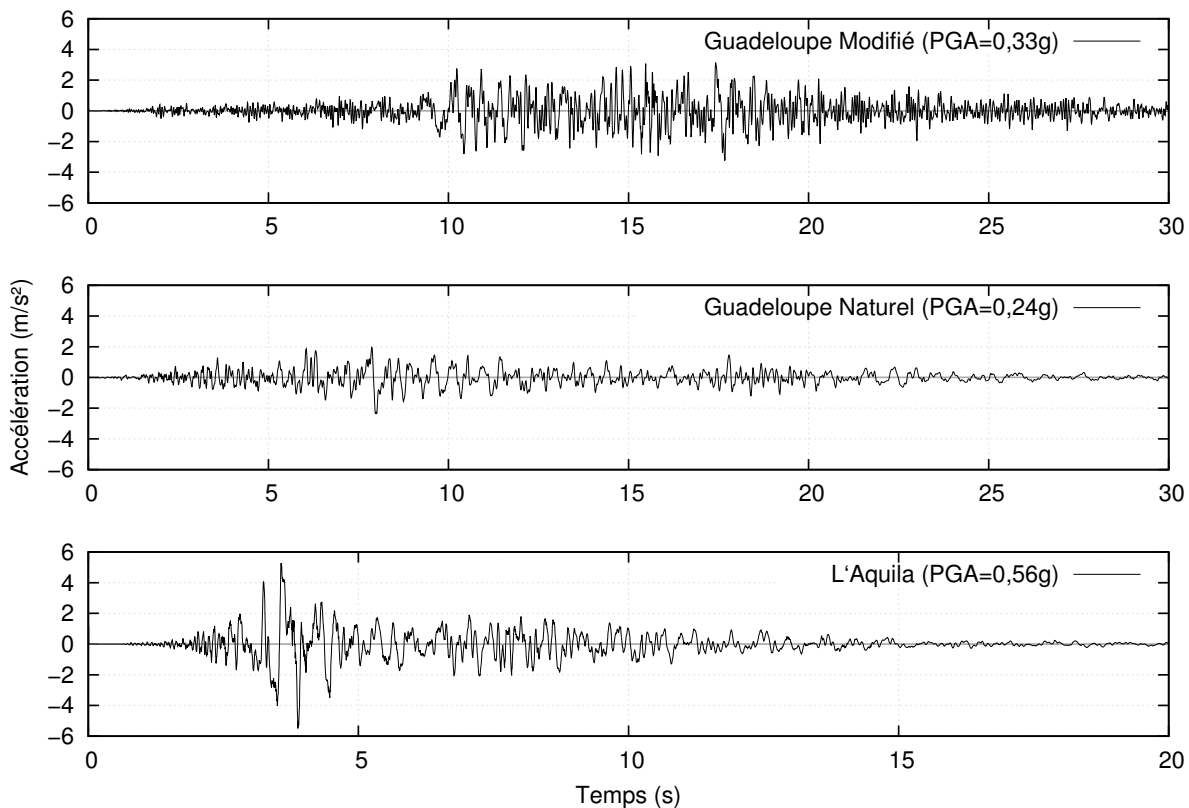
Figure 6.8: Accélérographes sélectionnés pour les essais dynamiques
