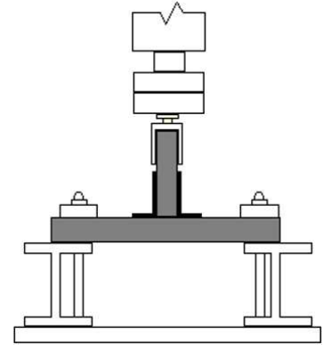
Figure 5.6: Banc d'essais (installation pour essai en Z)
