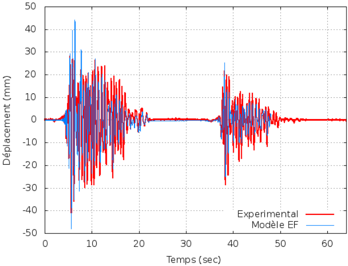
P16 AH 1500kg l'Aquila
