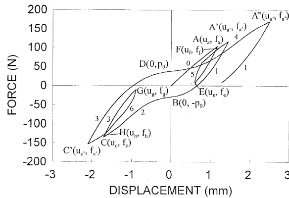
Figure B.7: Modèle de Kasal
