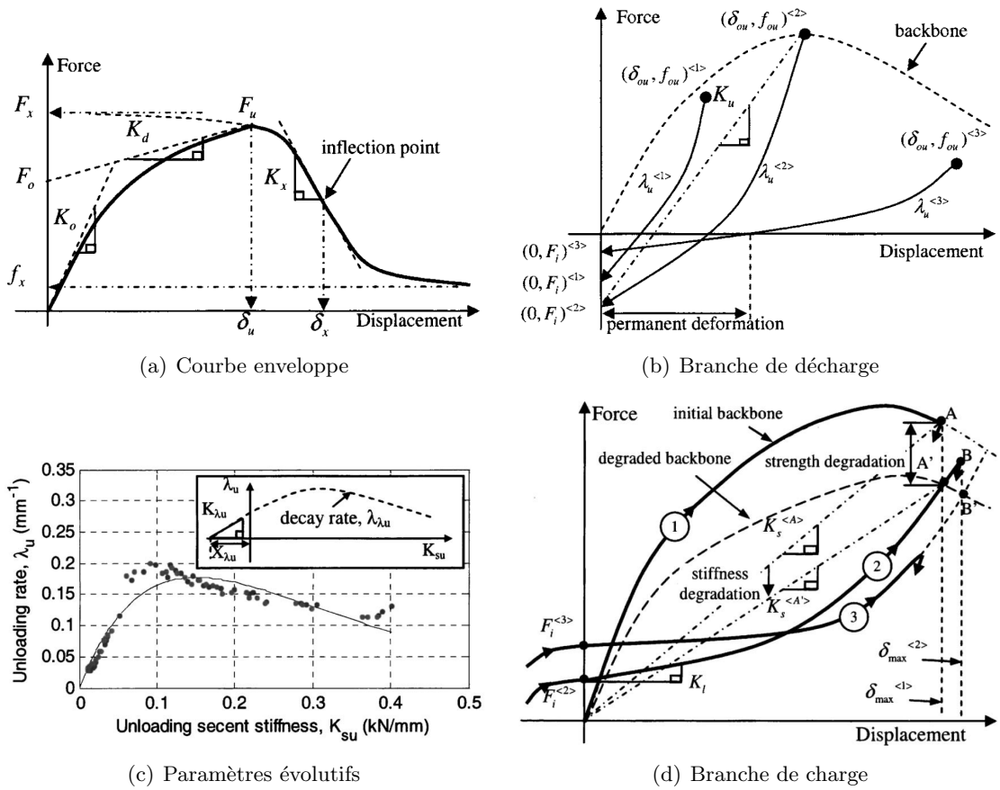
Figure B.16: Modèle EPHM
