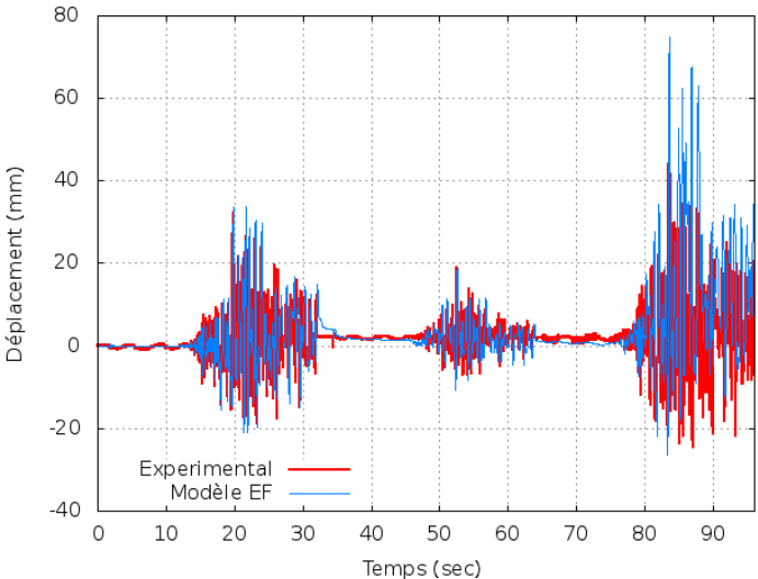
OSB12 AH 1500kg Guadeloupe Naturel
