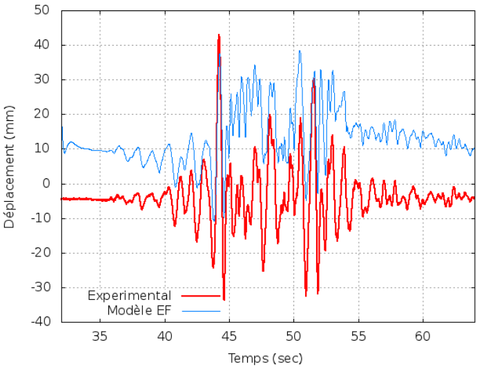
OSB12 AH 2000kg Guadeloupe Modifié 0,33 g
