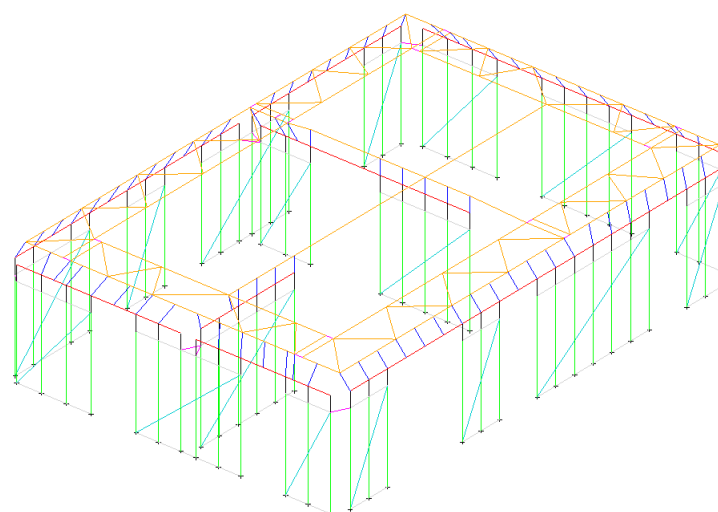
Figure 7.13: Maillage de la maison 8 \times 12 m
