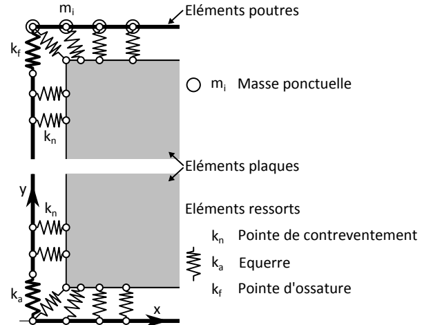
Figure 6.14: Représentation éclatée du modèle EF détaillé
