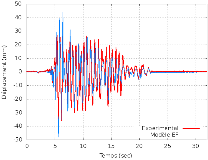
P16 AH 1500kg l'Aquila 1,8 g
