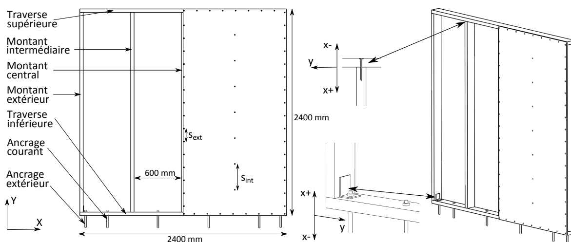
Figure 6.2: Schéma de principe des murs de contreventement
