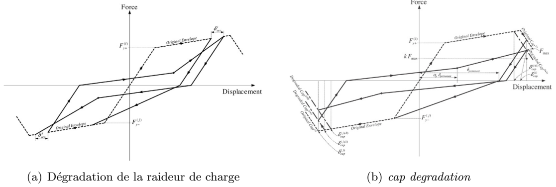
Figure B.15: Modèle de Ayoub (2ème partie)
