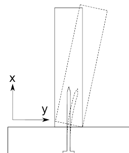
Figure 6.15: Rotation selon DRZ d'un assemblage entre éléments d'ossature
