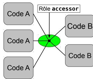
FIGURE 5.2 – Utilisation d'un connecteur pour décrire une interaction par partage de mémoire. Le connecteur possède un rôle accessor rempli par les ports de tous les composants qui accèdent à la mémoire dans le cas représenté de deux codes parallèles de degré 3 et 2.
