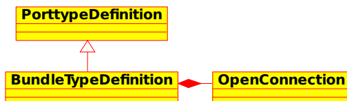
FIGURE 5.16 – Présentation de la modélisation du concept de bundle.
