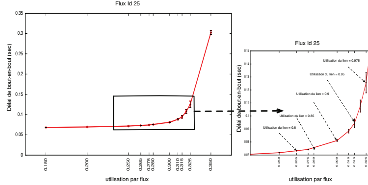
FIGURE 5.3 – Calcul du délai moyen de bout-en-bout du flux Id 25 en fonction du taux d'utilisation.
