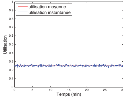
FIGURE 4.2 – Evolution du taux d'utilisation en fonction du temps pour une source Poisson.
