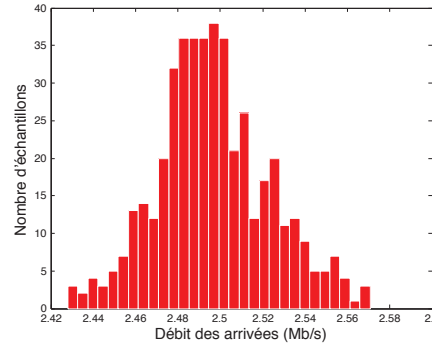
FIGURE 4.3 – Répartition des débits des arrivées pour une source Poisson.
