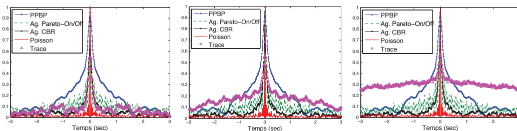
FIGURE 4.13 – Fonctions d'autocorrélations pour une trace réelle (Trace 2), pour une source Poisson, pour une source PPBP, pour une superposition de 100 flux CBR indépendants et pour une superposition de 20 flux On/Off Pareto sur différents intervalles de temps.
