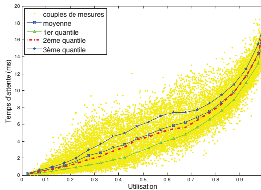
FIGURE 3.1 – Evolution du délai d'attente moyen des paquets dans le buffer du lien en fonction du taux d'utilisation.
