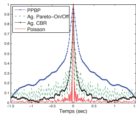
FIGURE 4.5 – Fonction d'autocorrélation pour une source Poisson, pour une source PPBP, pour une superposition de 100 flux CBR indépendants et pour une superposition de 20 flux On/Off Pareto.
