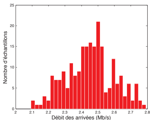
FIGURE 4.11 – Répartition des débits des arrivées pour une trace réelle (Trace 1).
