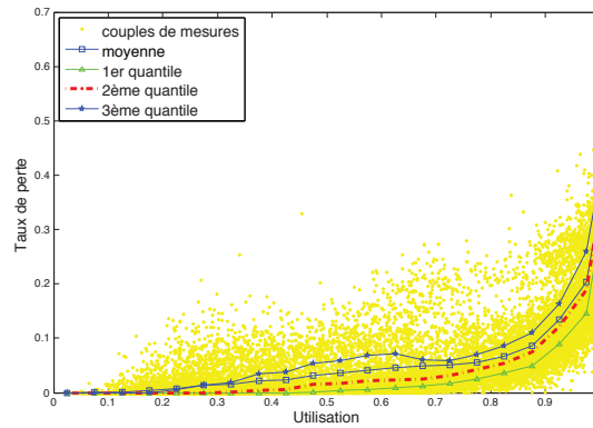
FIGURE 3.2 – Evolution du taux de perte moyen de paquets dans le buffer du lien en fonction du taux d'utilisation.
