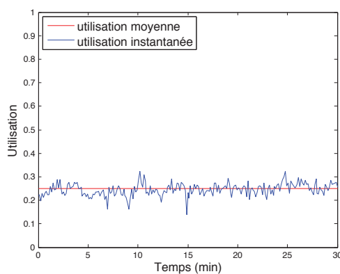
FIGURE 4.10 – Evolution du taux d'utilisation en fonction du temps pour une trace réelle (Trace 1).
