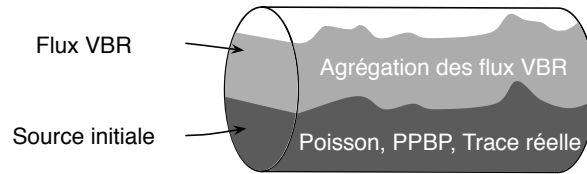
FIGURE 4.1 – Trafic transitant sur un lien de communication, modélisé par une source initiale et des flux VBR.
